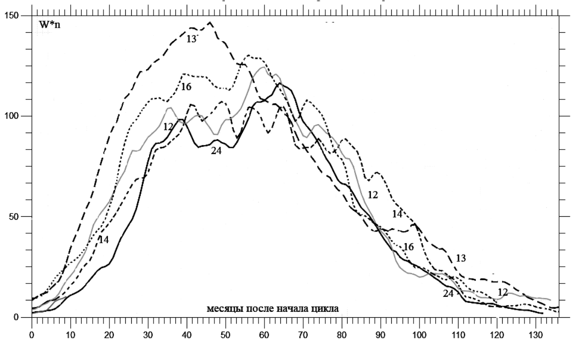
Рис. 2 – Развитие СЦ 24 в сравнении с низкими (12–серый, 14, 16) и средним (13) СЦ в сглаженных относительных числах пятен ( W^*n - в новой системе V2)
