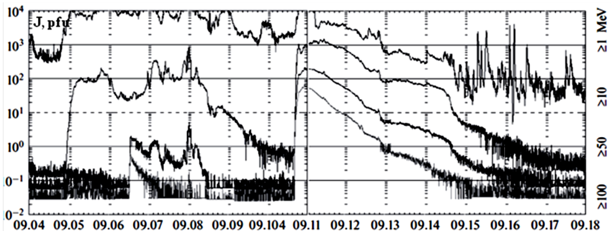
Рис. 5. Поток солнечных высокоэнергичных протонов в сентябре 2017 г. от больших солнечных вспышек в AR12673 по данным геостационарного спутника GOES-11. ( http://www.swpc.noaa.gov )
