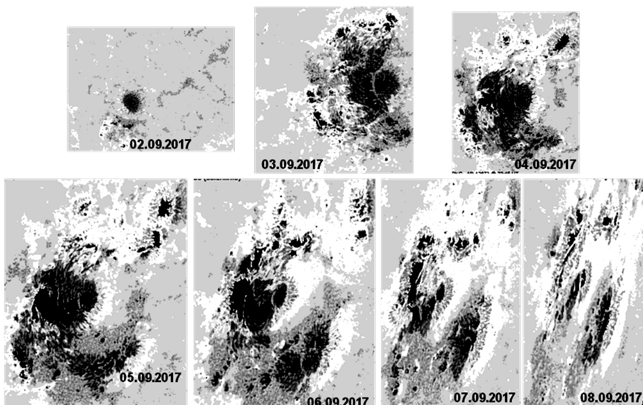
Рис. 4 – Вид группы пятен AR12673 и динамика её развития по наблюдениям космической солнечной обсерватории SDO в непрерывном спектре (4500 Å) с наложенным магнитным полем (белое "+" полярность) за 2 – 8.09.2017 г. Преобразованный рисунок из http://www.solen.info/solar/ .
