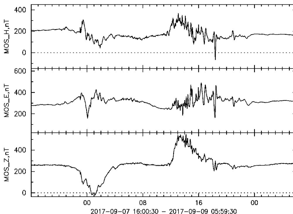
Рис. 6. Очень большая магнитная буря (G4) 7 – 8.09.2017 г. по данным геомагнитной обсерватории Москва (ИЗМИРАН). По вертикальной оси приводится развитие магнитной бури в компонентах геомагнитного поля H, E, Z
