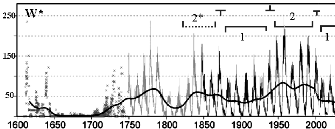
Рис. 1 – Полный ряд наблюдений сглаженных ( W^* ) относительных чисел солнечных пятен. Достоверный ряд ( W^*1 ) с 1849 г. (чёрный) с границами структурных эпох пониженной (1) и повышенной (2) СА с переходными циклами между ними ( \top – к пониженной; \perp – к повышенной). В первом периоде повышенной СА (2*), включающей СЦ 10 – 6 циклы 6 и 7 включены условно. Вероятный ход развития 25 СЦ (последний справа). Восстановленный ряд ( W^*2 ) – серый, предполагаемый – крестики. Преобразованный рисунок из Википедии http://en.wikipedia.org/wiki/Sunspot
