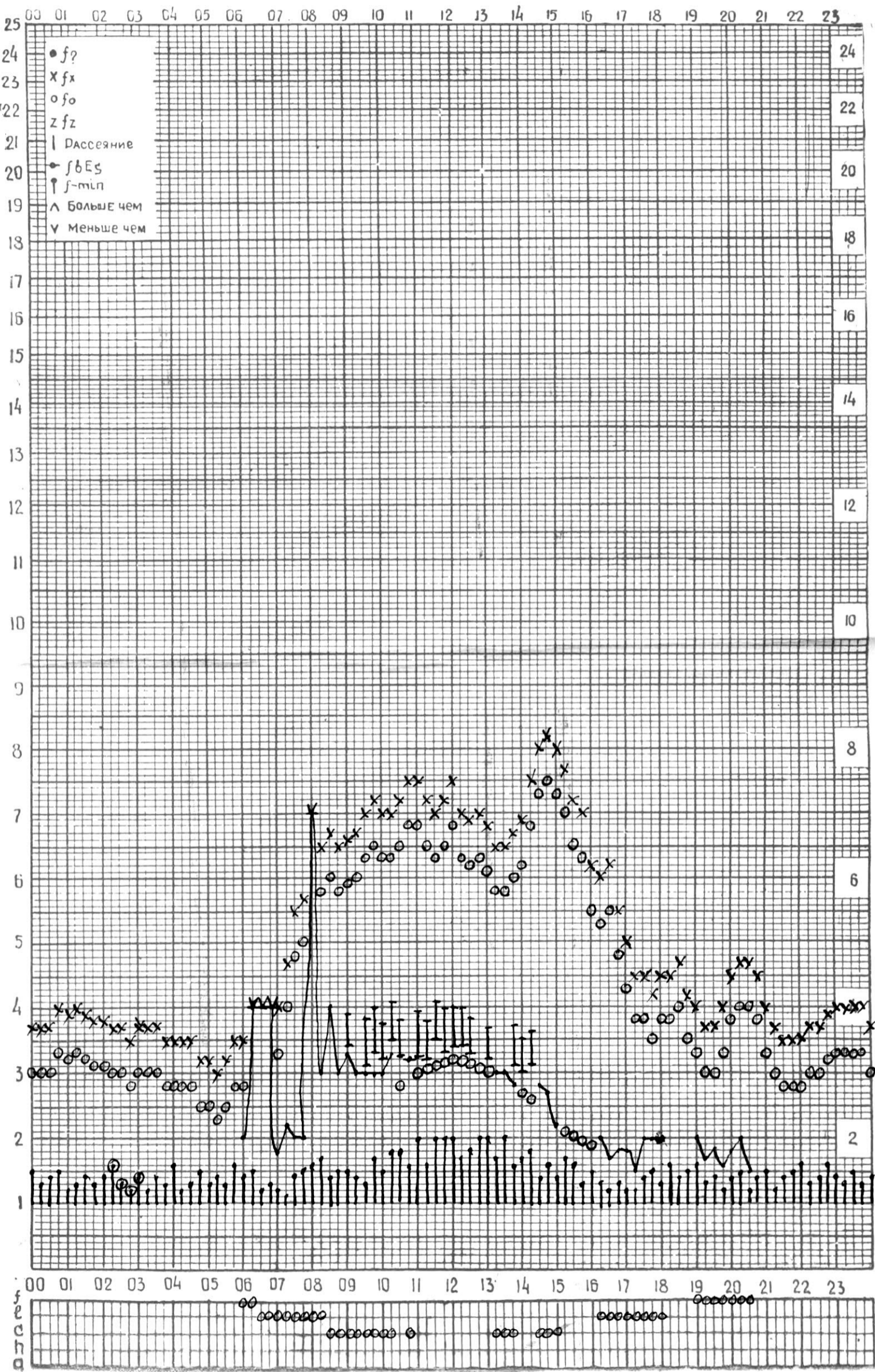
СТАНЦИЯ ТБИЛИСИ F-ГРАФИК ИОНОСФЕРНЫХ ДАННЫХ, ДАТА 10 ДЕКАБРЯ, 1974
