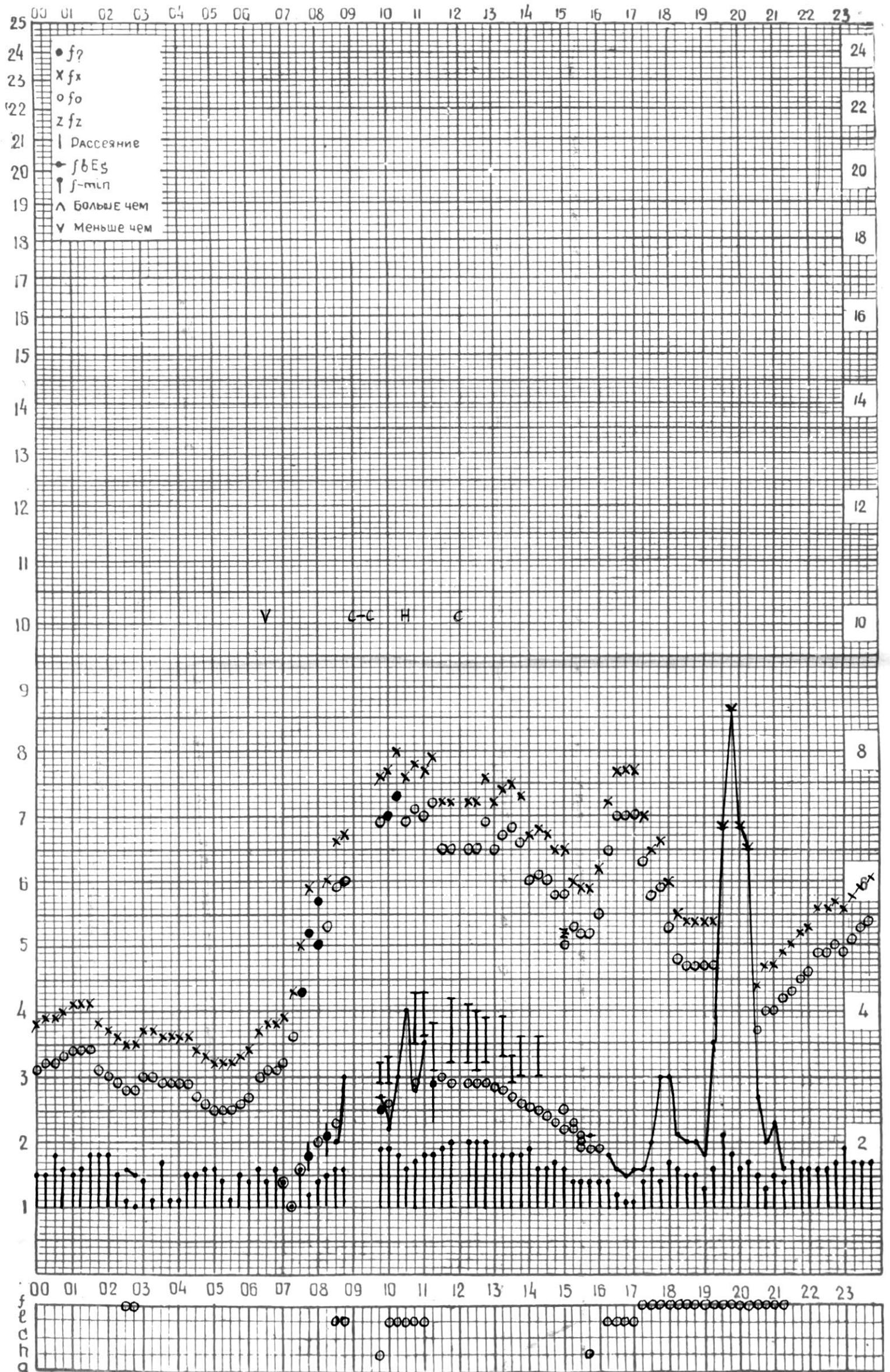
СТАНЦИЯ ТБИЛИСИ F-ГРАФИК ИОНОСФЕРНЫХ ДАННЫХ, ДАТА 29 ДЕКАБРЯ, 1974
