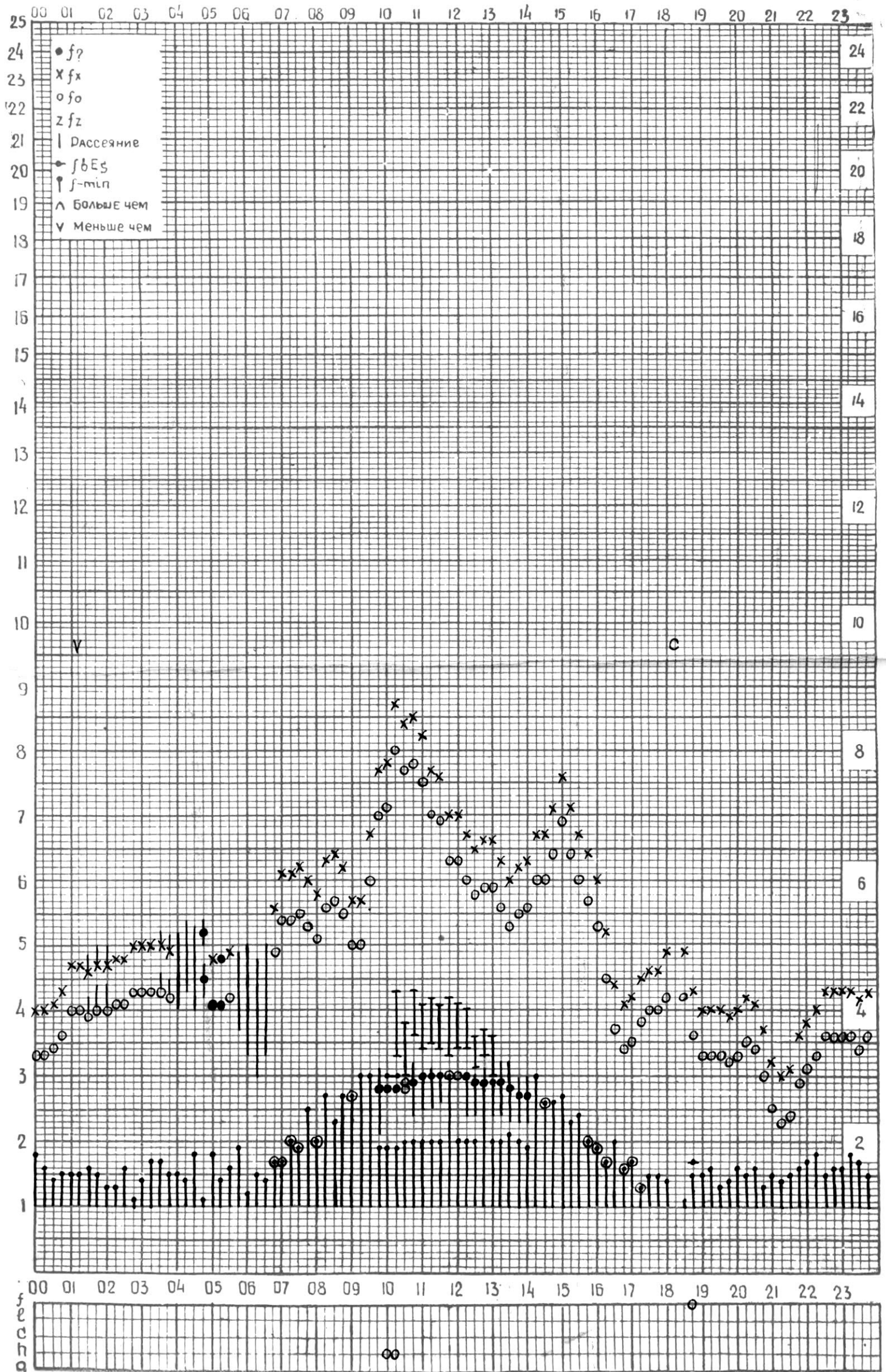
СТАНЦИЯ ТБИЛИСИ F-ГРАФИК ИОНОСФЕРНЫХ ДАННЫХ, ДАТА 5 ДЕКАБРЯ, 1974
