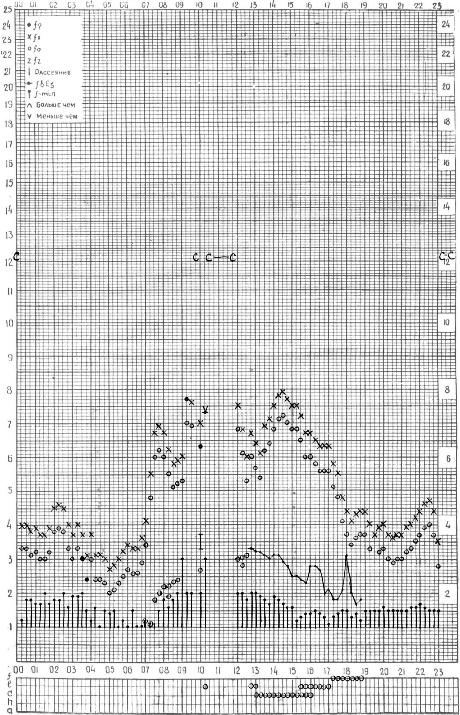
СТАНЦИЯ ТБИЛИСИ F-ГРАФИК ИОНОСФЕРНЫХ ДАННЫХ, ДАТА 19 ДЕКАБРЯ 1974
