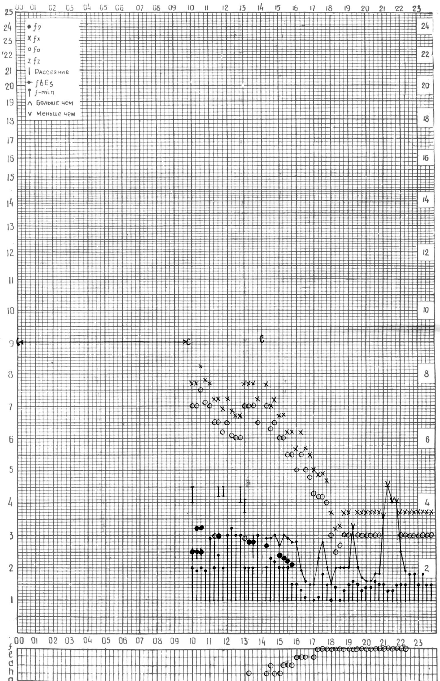
СТАНЦИЯ ТБИЛИСИ F-ГРАФИК ИОНОСФЕРНЫХ ДАННЫХ, ДАТА 16 ДЕКАБРЯ, 1974
