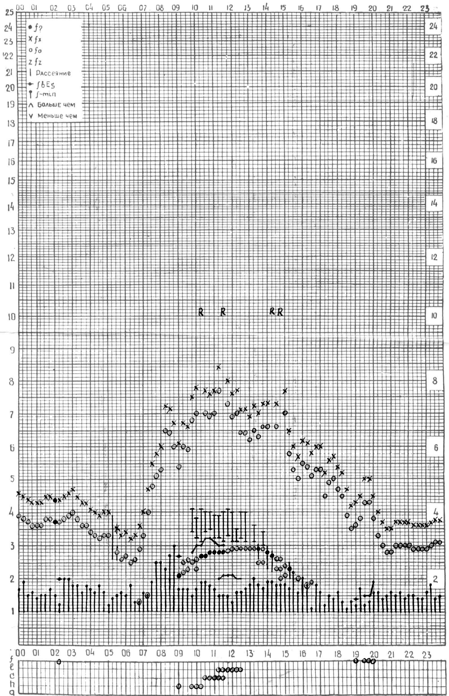
СТАНЦИЯ ТБИЛИСИ F-ГРАФИК ИОНОСФЕРНЫХ ДАННЫХ, ДАТА 9 ДЕКАБРЯ, 1974
