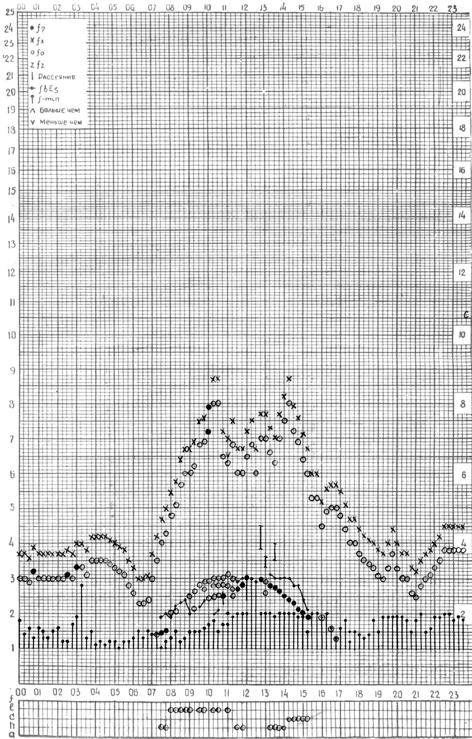
СТАНЦИЯ ТБИЛИСИ F-ГРАФИК ИОНОСФЕРНЫХ ДАННЫХ, ДАТА 12 ДЕКАБРЯ, 1974
