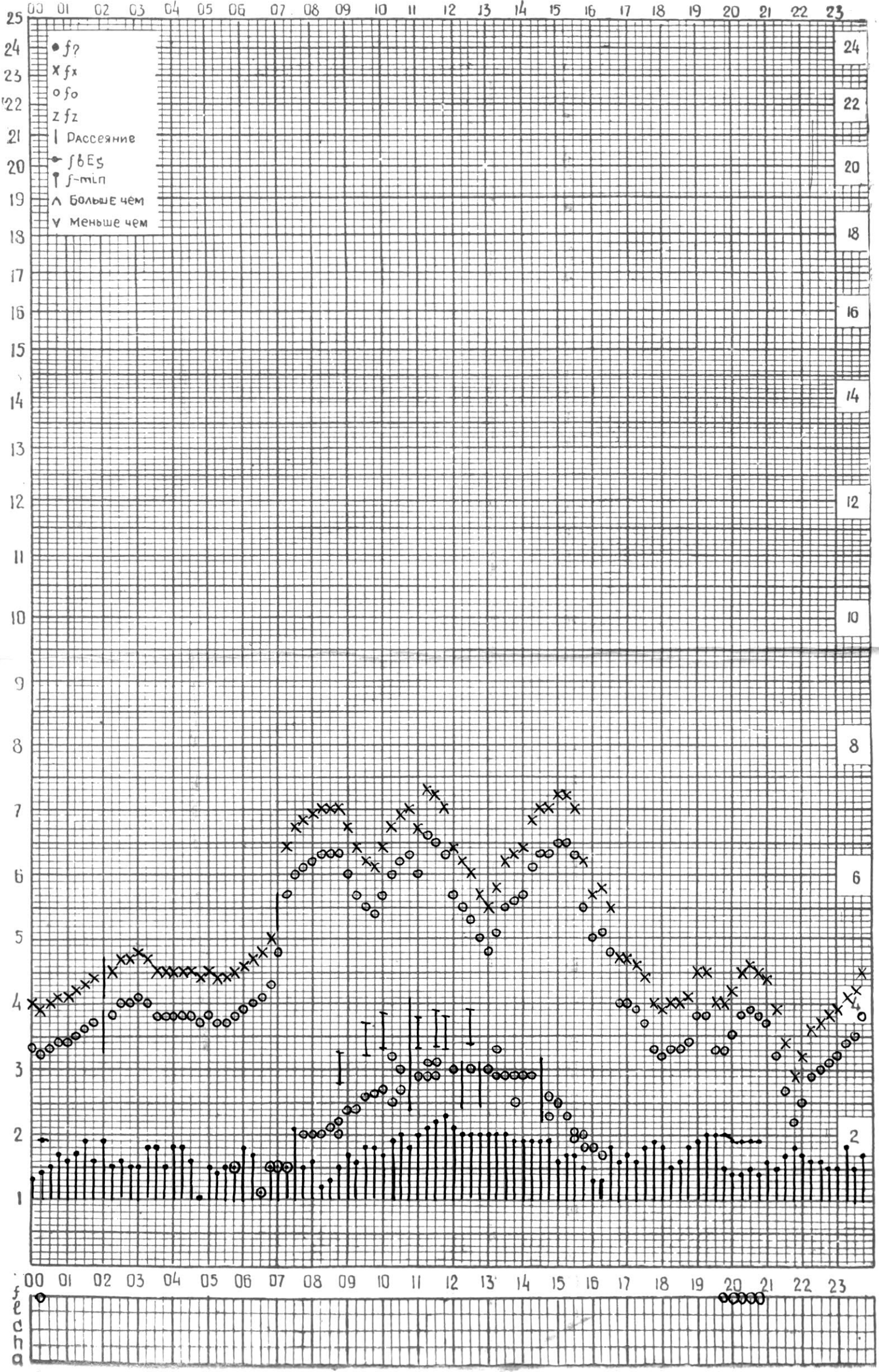
СТАНЦИЯ ТБИЛИСИ F-ГРАФИК ИОНОСФЕРНЫХ ДАННЫХ, ДАТА 7 ДЕКАБРЯ, 1974
