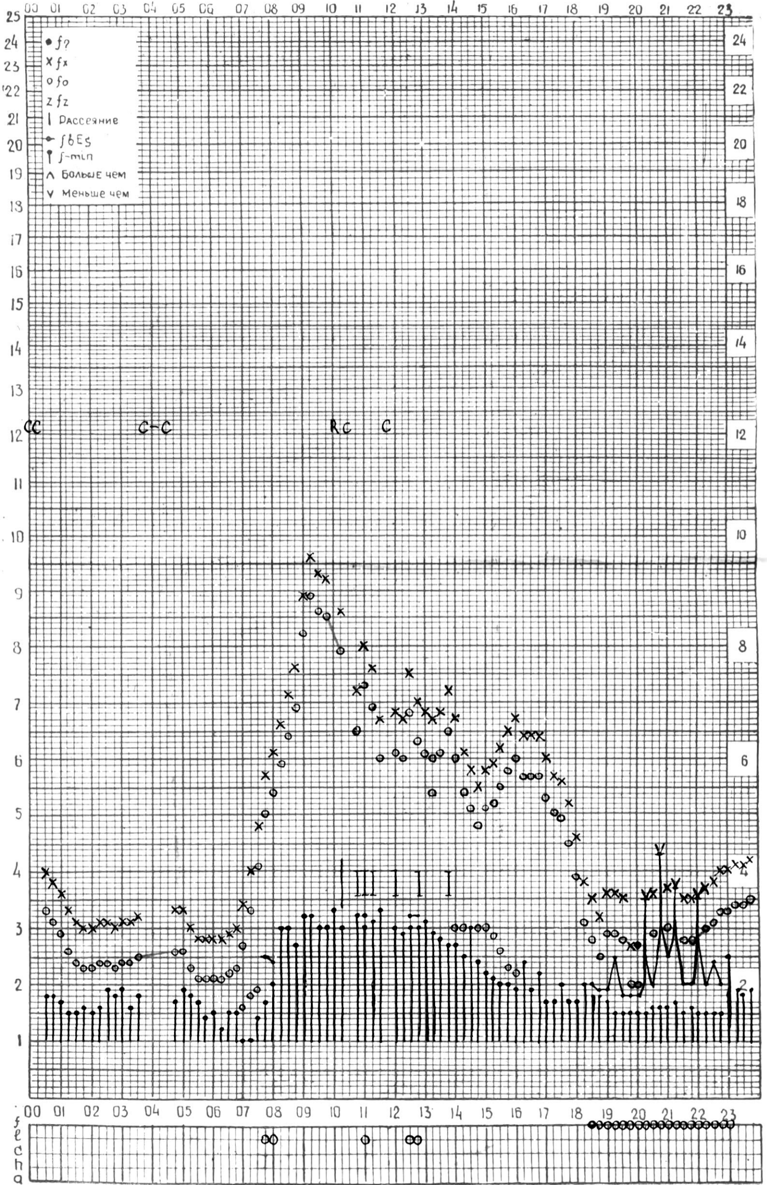
СТАНЦИЯ ТБИЛИСИ F-ГРАФИК ИОНОСФЕРНЫХ ДАННЫХ, ДАТА 31 ДЕКАБРЯ 1974
