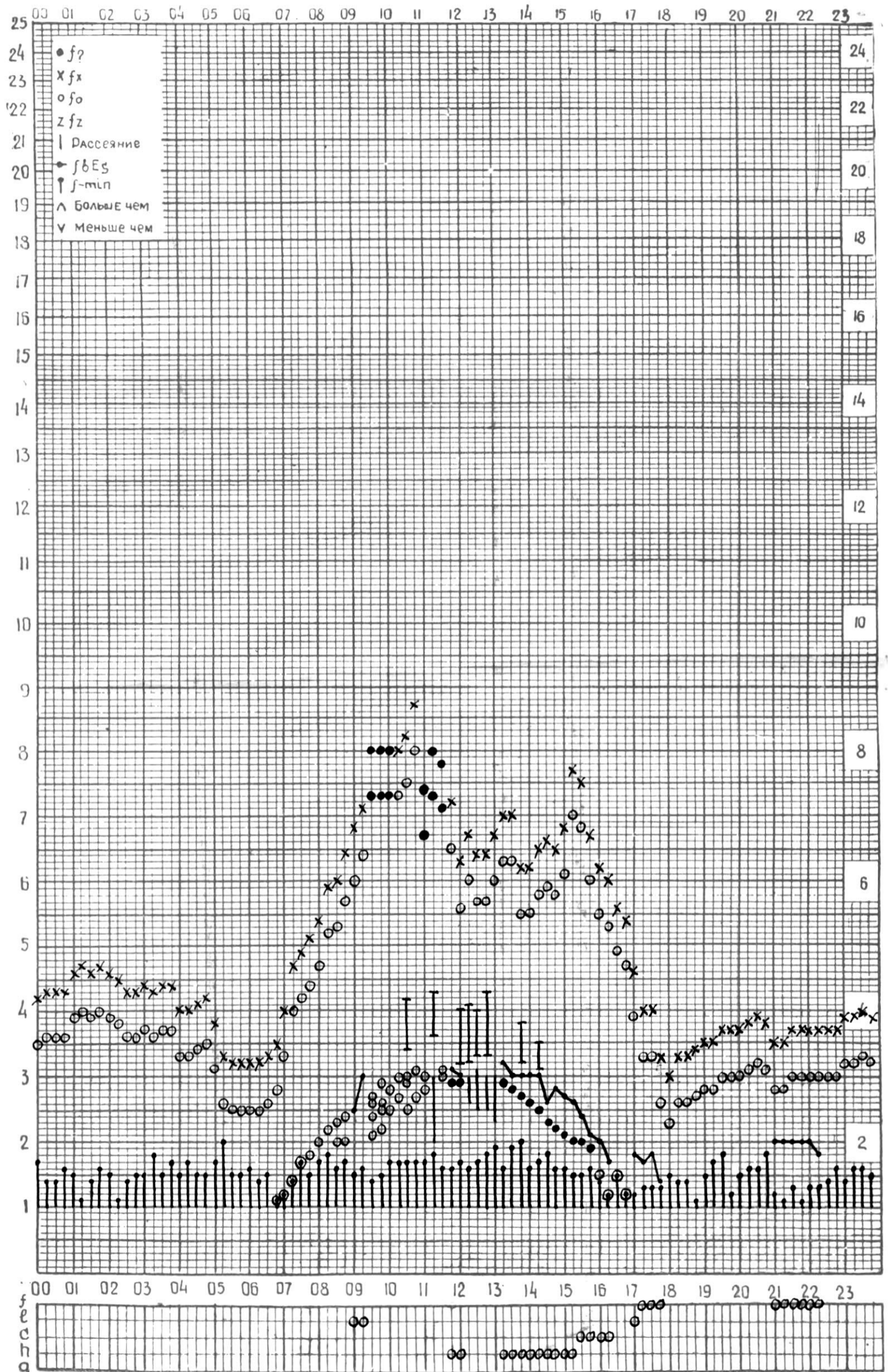
СТАНЦИЯ ТБИЛИСИ F-ГРАФИК ИОНОСФЕРНЫХ ДАННЫХ, ДАТА 13 ДЕКАБРЯ, 1974
