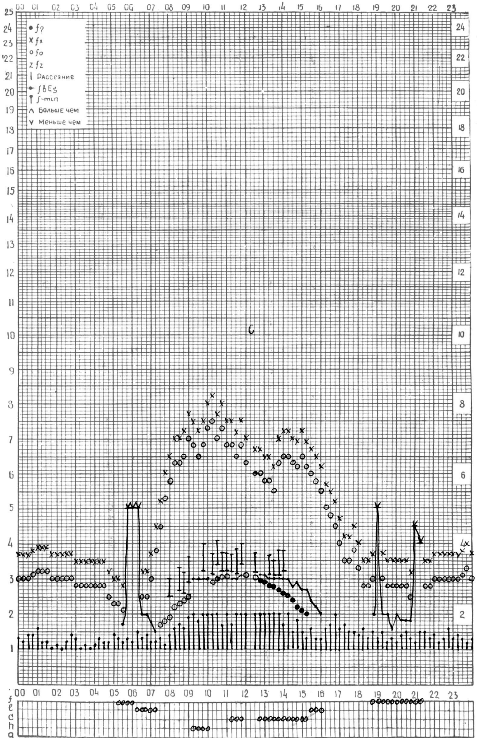
СТАНЦИЯ ТБИЛИСИ F-ГРАФИК ИОНОСФЕРНЫХ ДАННЫХ, ДАТА 26 ДЕКАБРЯ, 1974
