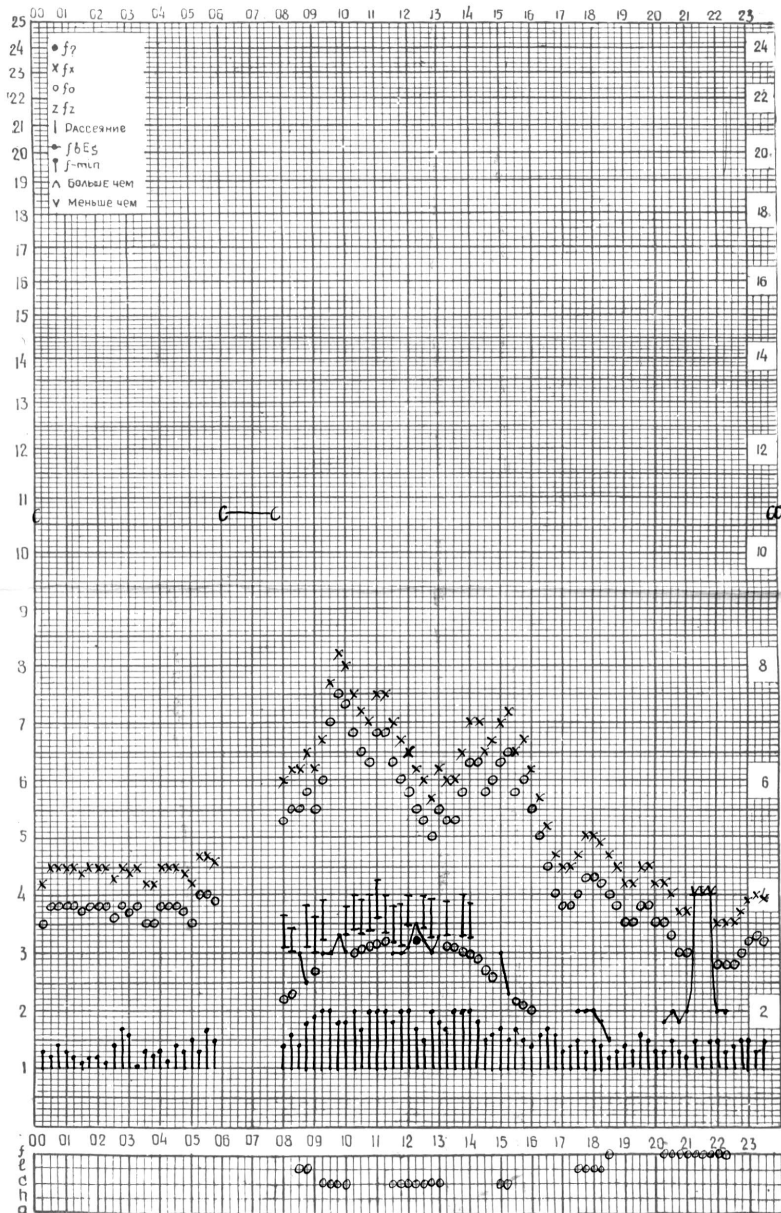
СТАНЦИЯ ТБИЛИСИ F-ГРАФИК ИОНОСФЕРНЫХ ДАННЫХ, ДАТА 6 ДЕКАБРЯ, 1974
