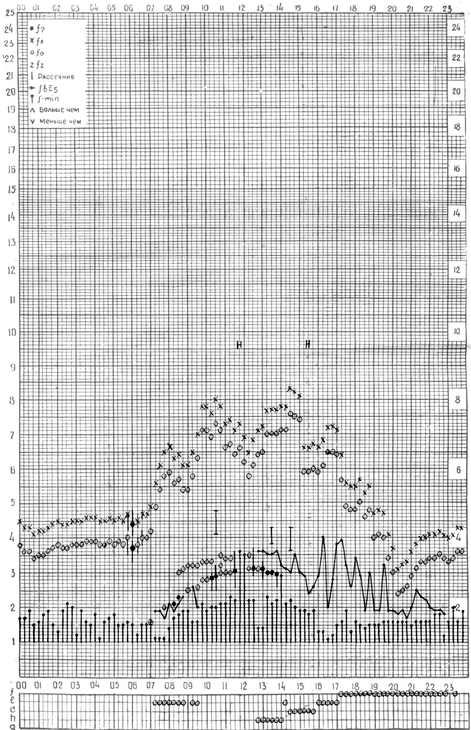
СТАНЦИЯ ТБИЛИСИ F-ГРАФИК ИОНОСФЕРНЫХ ДАННЫХ, ДАТА 17 ДЕКАБРЯ, 1974
