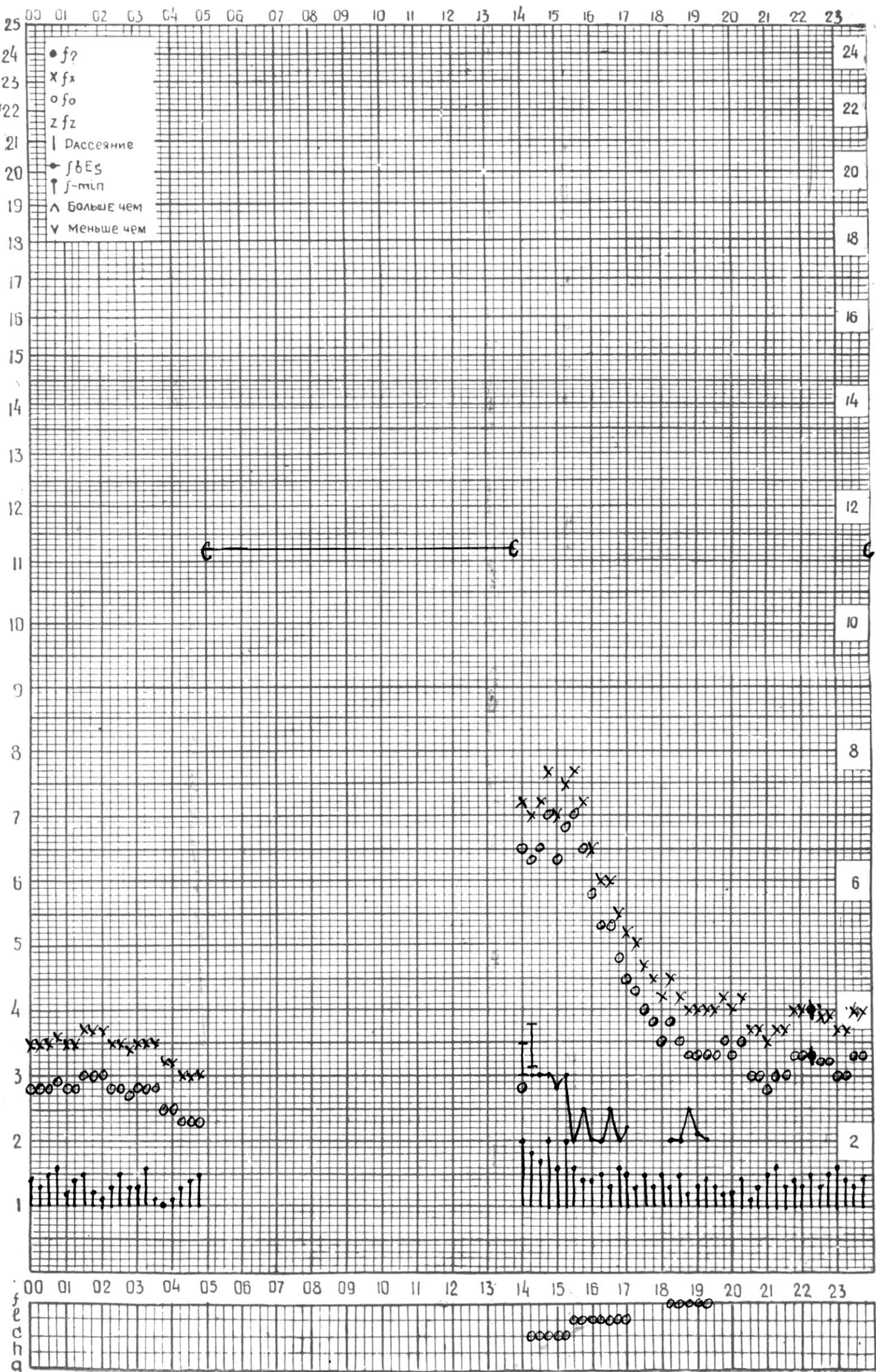
СТАНЦИЯ ТБИЛИСИ F-ГРАФИК ИОНОСФЕРНЫХ ДАННЫХ, ДАТА 14 ДЕКАБРЯ, 1974
