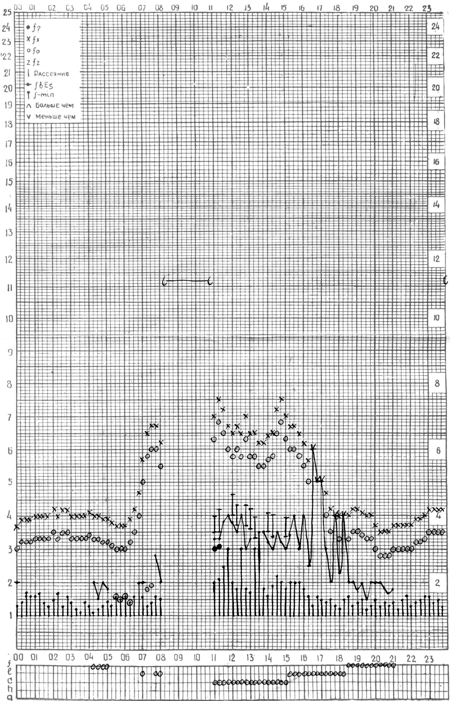
СТАНЦИЯ ТБИЛИСИ F-ГРАФИК ИОНОСФЕРНЫХ ДАННЫХ, ДАТА 1 ДЕКАБРЯ, 1974.
