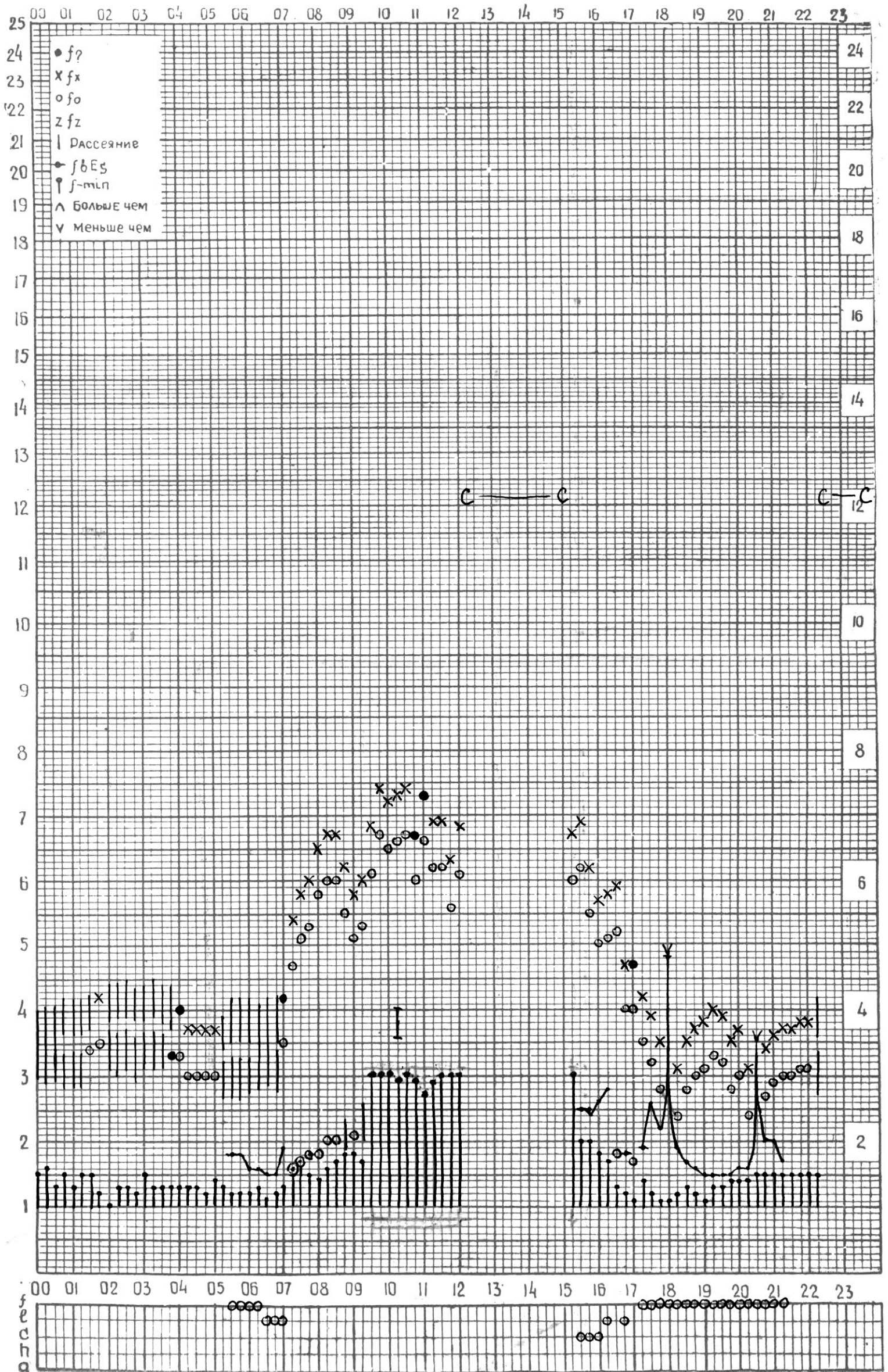
СТАНЦИЯ ТБИЛИСИ F-ГРАФИК ИОНОСФЕРНЫХ ДАННЫХ, ДАТА 15 ДЕКАБРЯ, 1974
