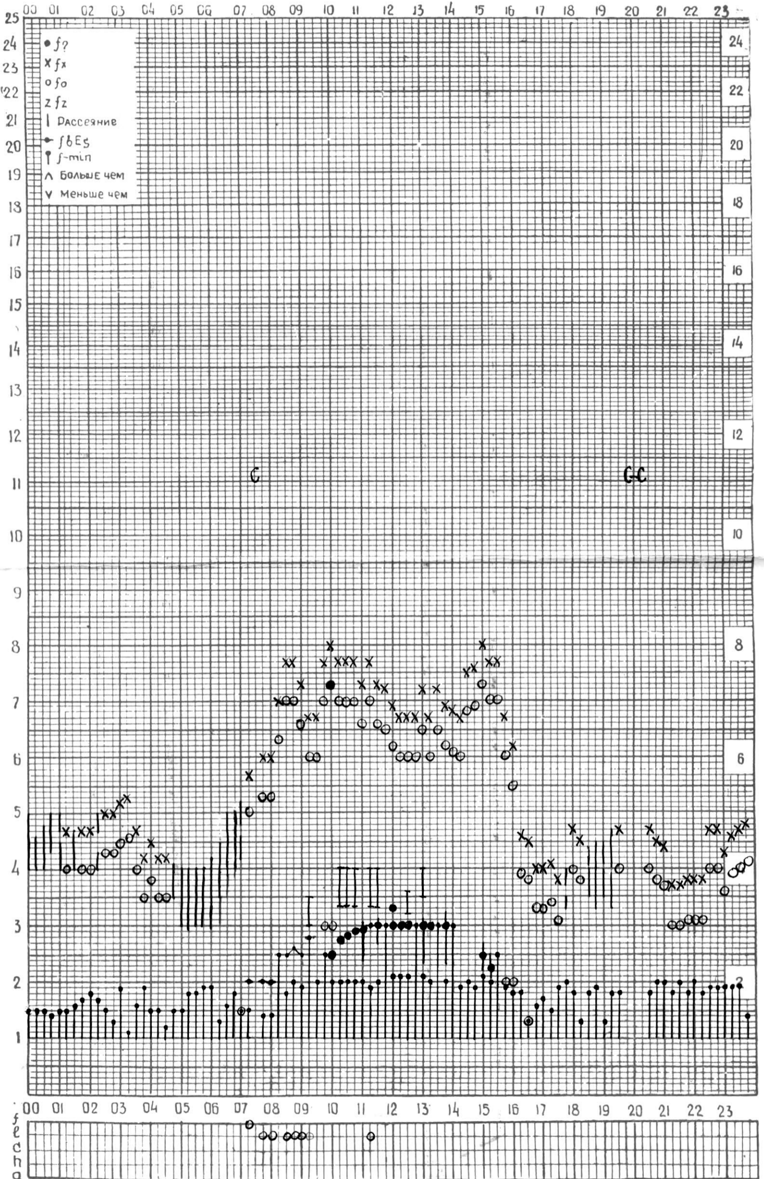
СТАНЦИЯ ТБИЛИСИ F-ГРАФИК ИОНОСФЕРНЫХ ДАННЫХ, ДАТА 4 ДЕКАБРЯ, 1974
