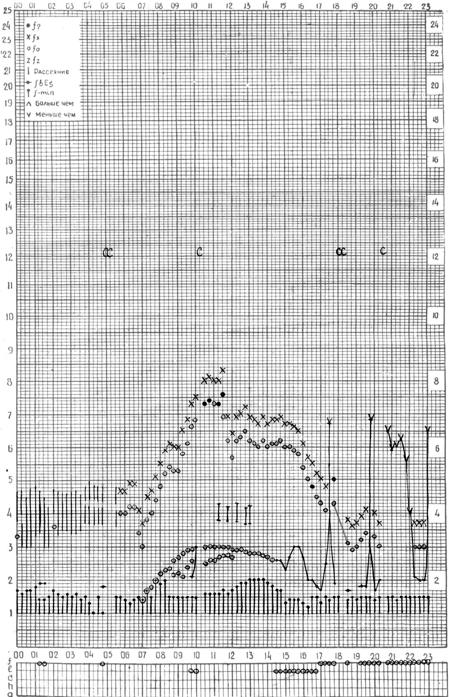
СТАНЦИЯ ТБИЛИСИ F-ГРАФИК ИОНОСФЕРНЫХ ДАННЫХ, ДАТА 23 ДЕКАБРЯ, 1974
