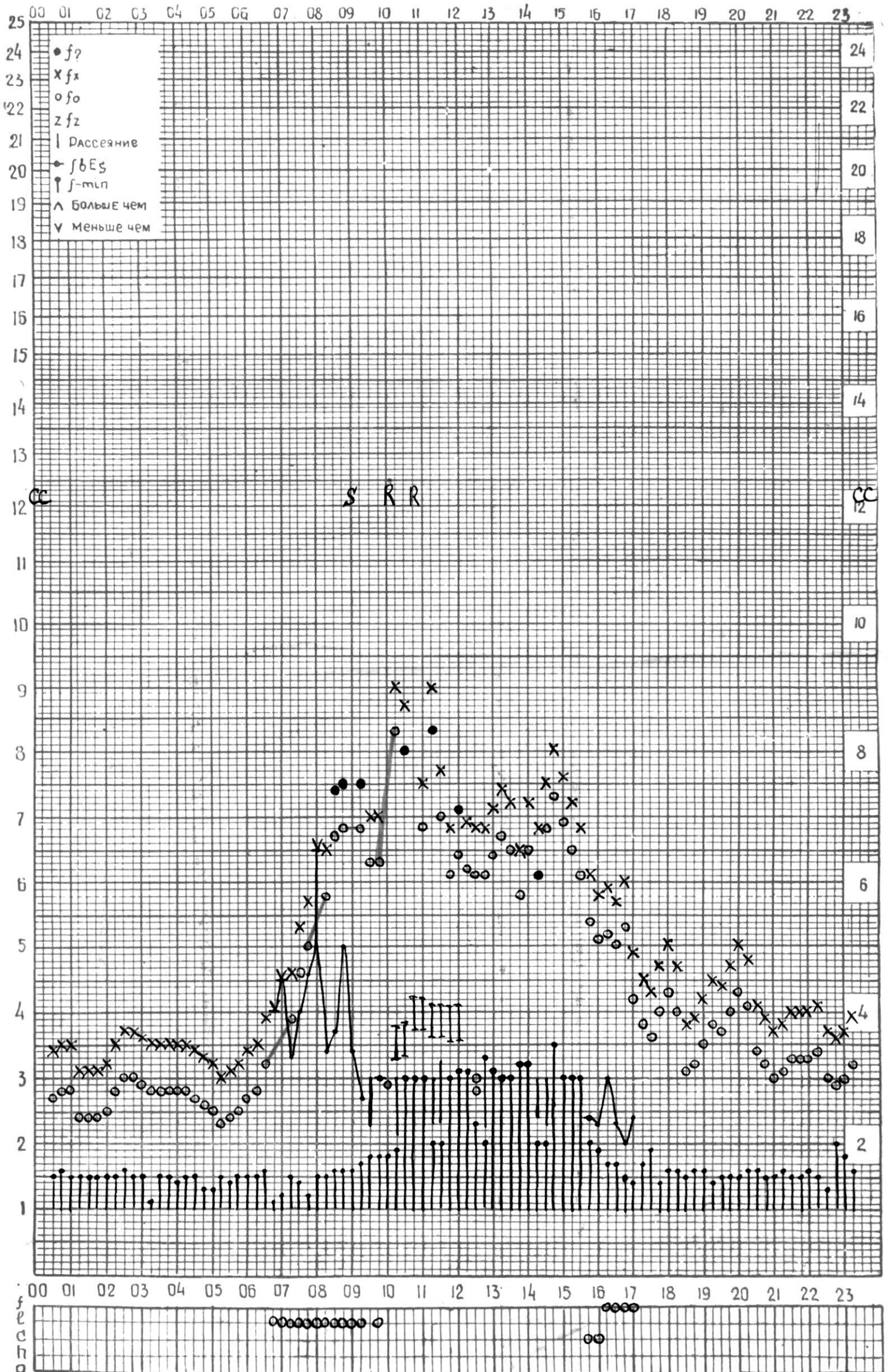
СТАНЦИЯ ТБИЛИСИ F-ГРАФИК ИОНОСФЕРНЫХ ДАННЫХ, ДАТА 27 ДЕКАБРЯ 1974
