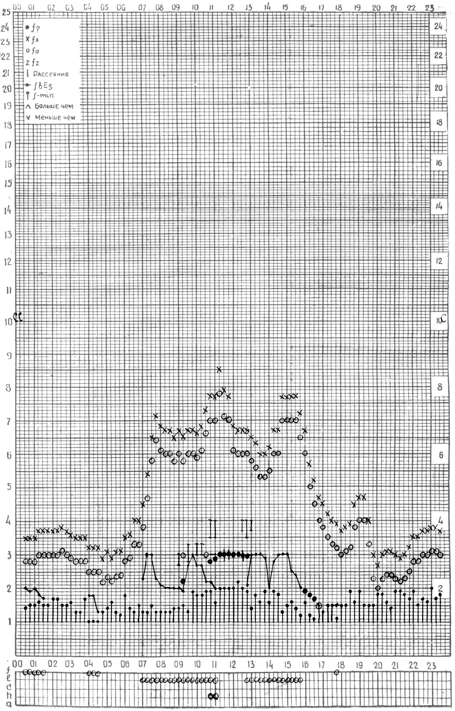
СТАНЦИЯ ТБИЛИСИ F-ГРАФИК ИОНОСФЕРНЫХ ДАННЫХ, ДАТА 24 ДЕКАБРЯ, 1974
