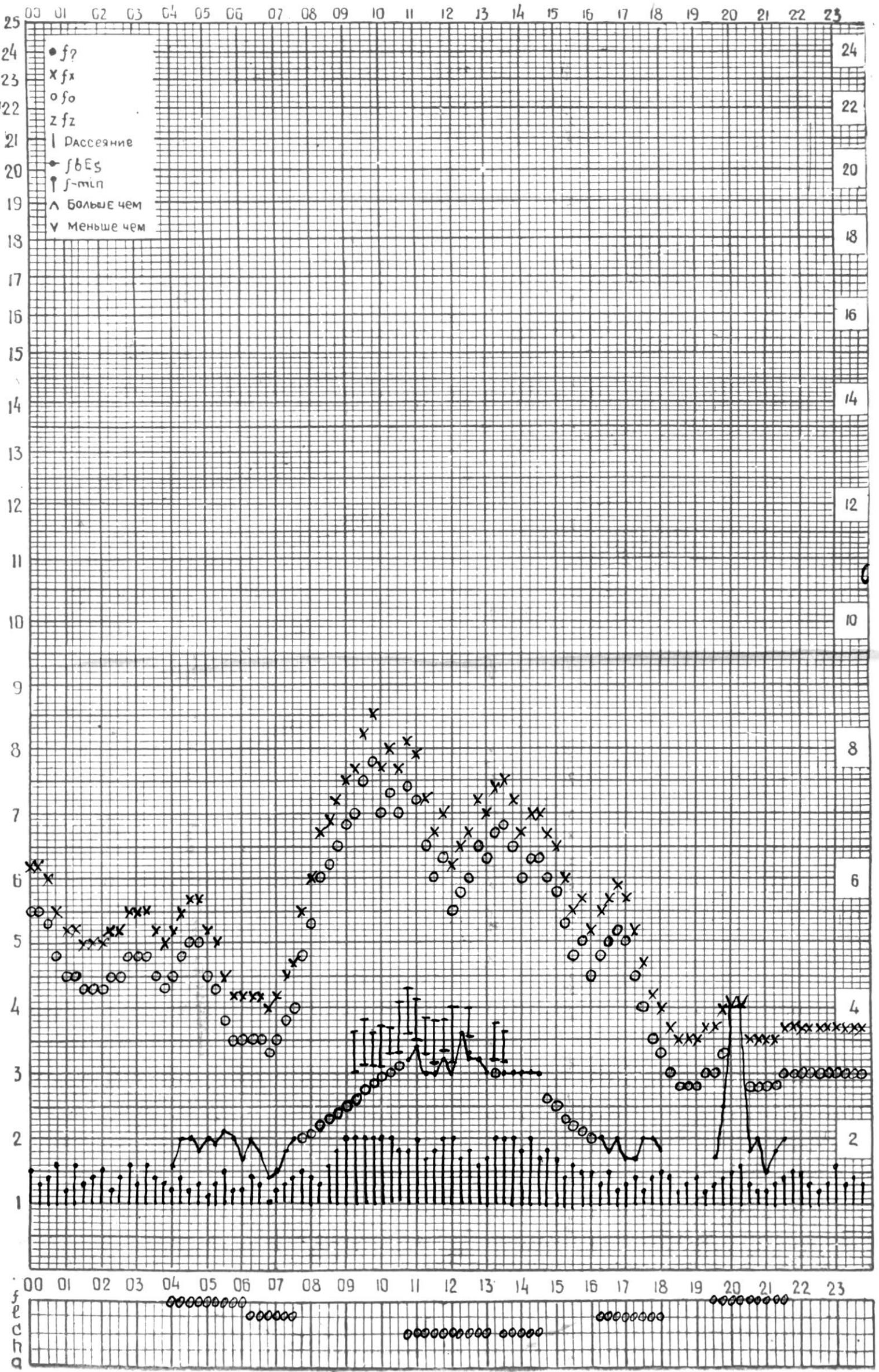
СТАНЦИЯ ТБИЛИСИ F-ГРАФИК ИОНОСФЕРНЫХ ДАННЫХ, ДАТА 30 ДЕКАБРЯ, 1974
