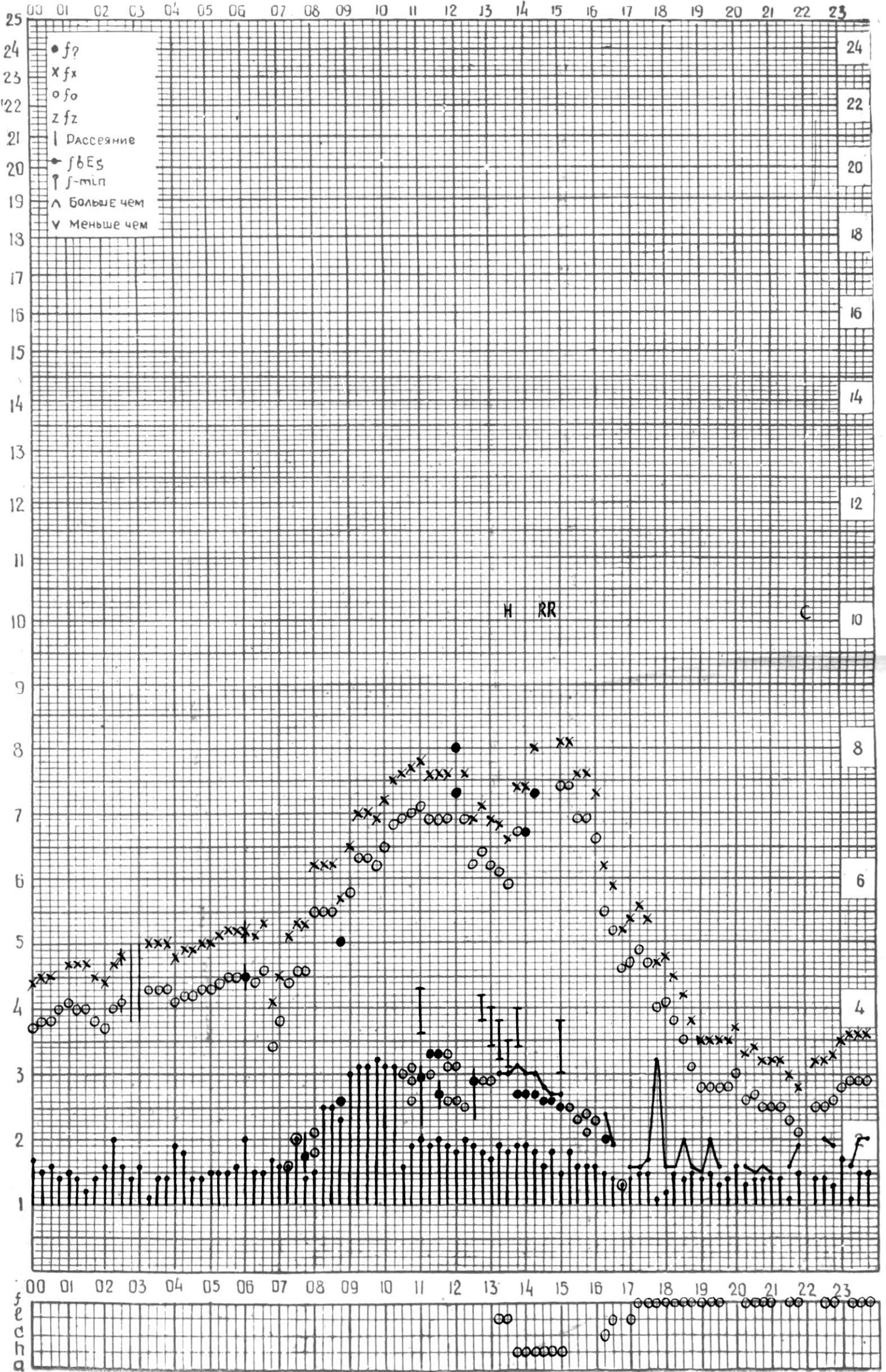
СТАНЦИЯ ТБИЛИСИ F-ГРАФИК ИОНОСФЕРНЫХ ДАННЫХ, ДАТА 21 ДЕКАБРЯ, 1974
