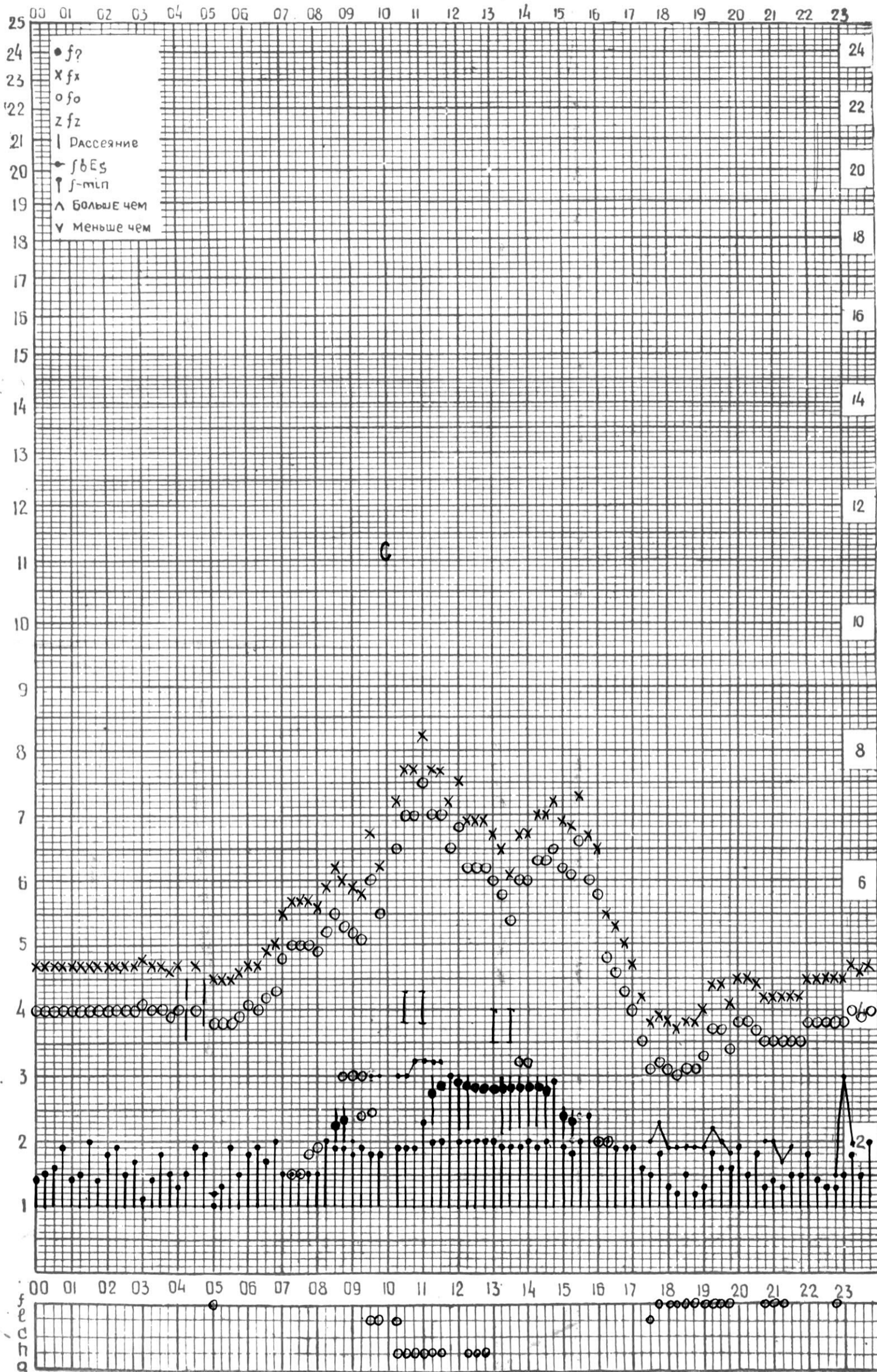
СТАНЦИЯ ТБИЛИСИ F-ГРАФИК ИОНОСФЕРНЫХ ДАННЫХ, ДАТА 8 ДЕКАБРЯ, 1974
