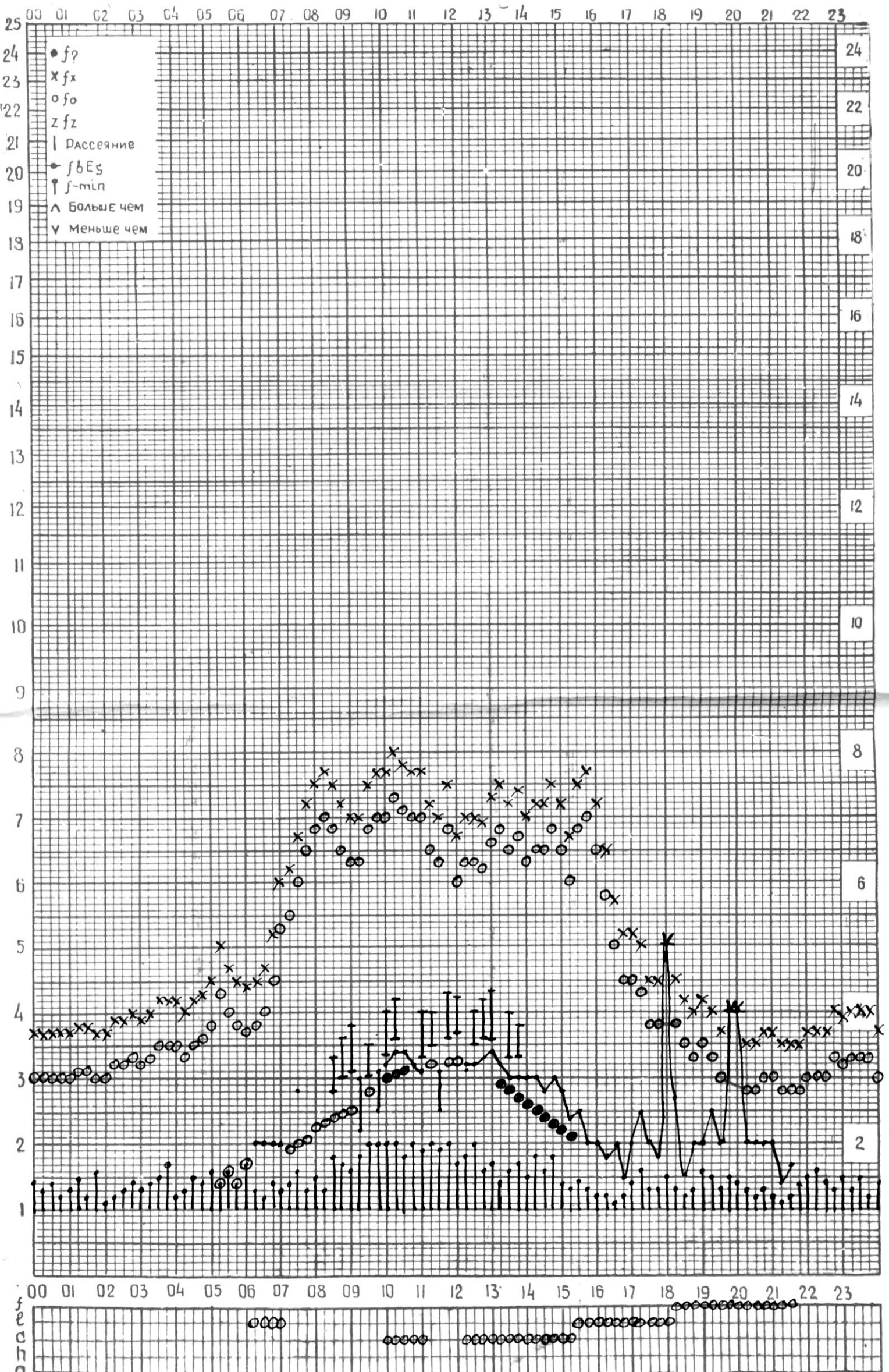
СТАНЦИЯ ТБИЛИСИ F-ГРАФИК ИОНОСФЕРНЫХ ДАННЫХ, ДАТА 27 НОЯБРЯ, 1974
