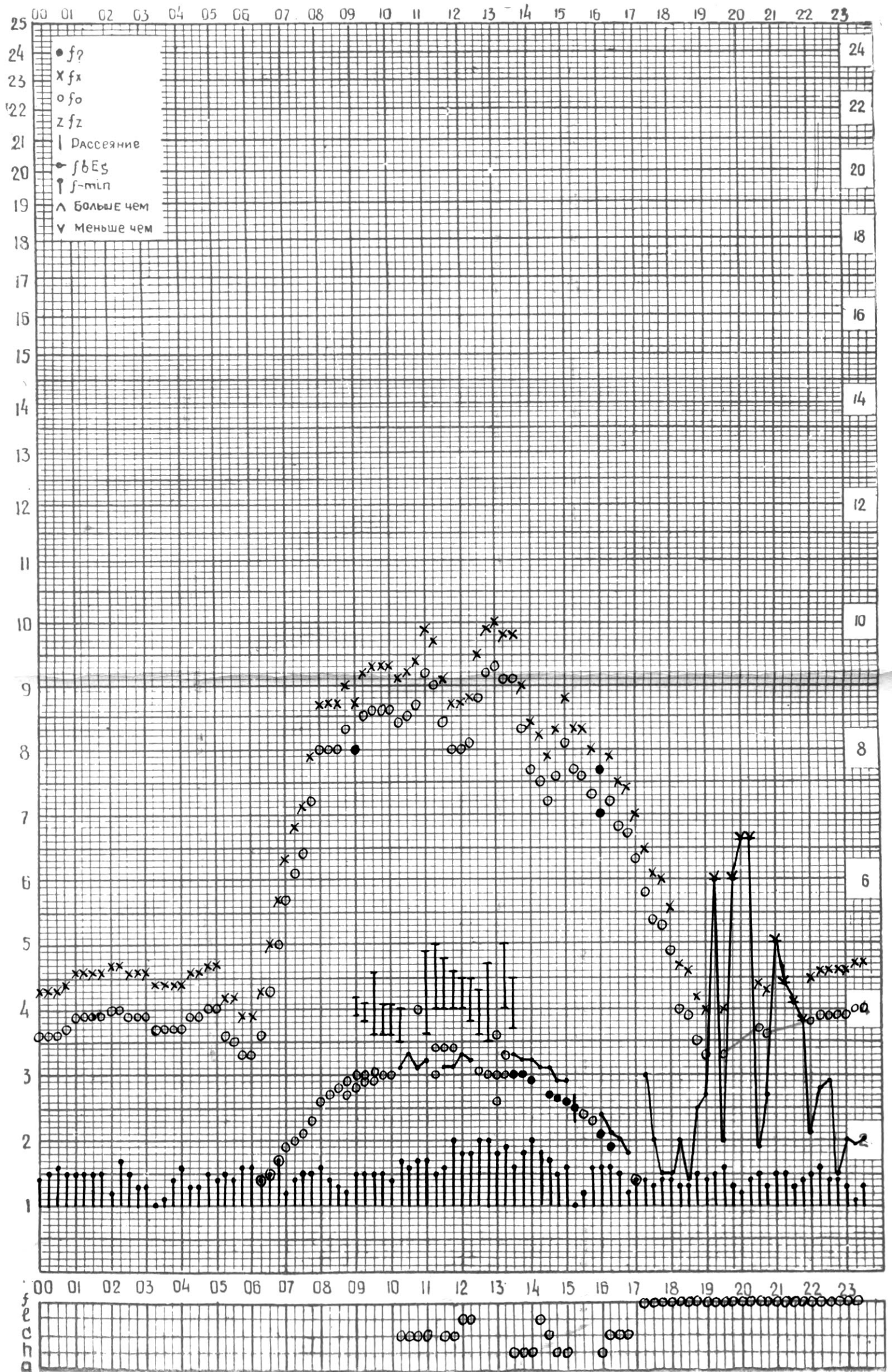
СТАНЦИЯ ТБИЛИСИ F-ГРАФИК ИОНОСФЕРНЫХ ДАННЫХ, ДАТА 3 НОЯБРЯ, 1974
