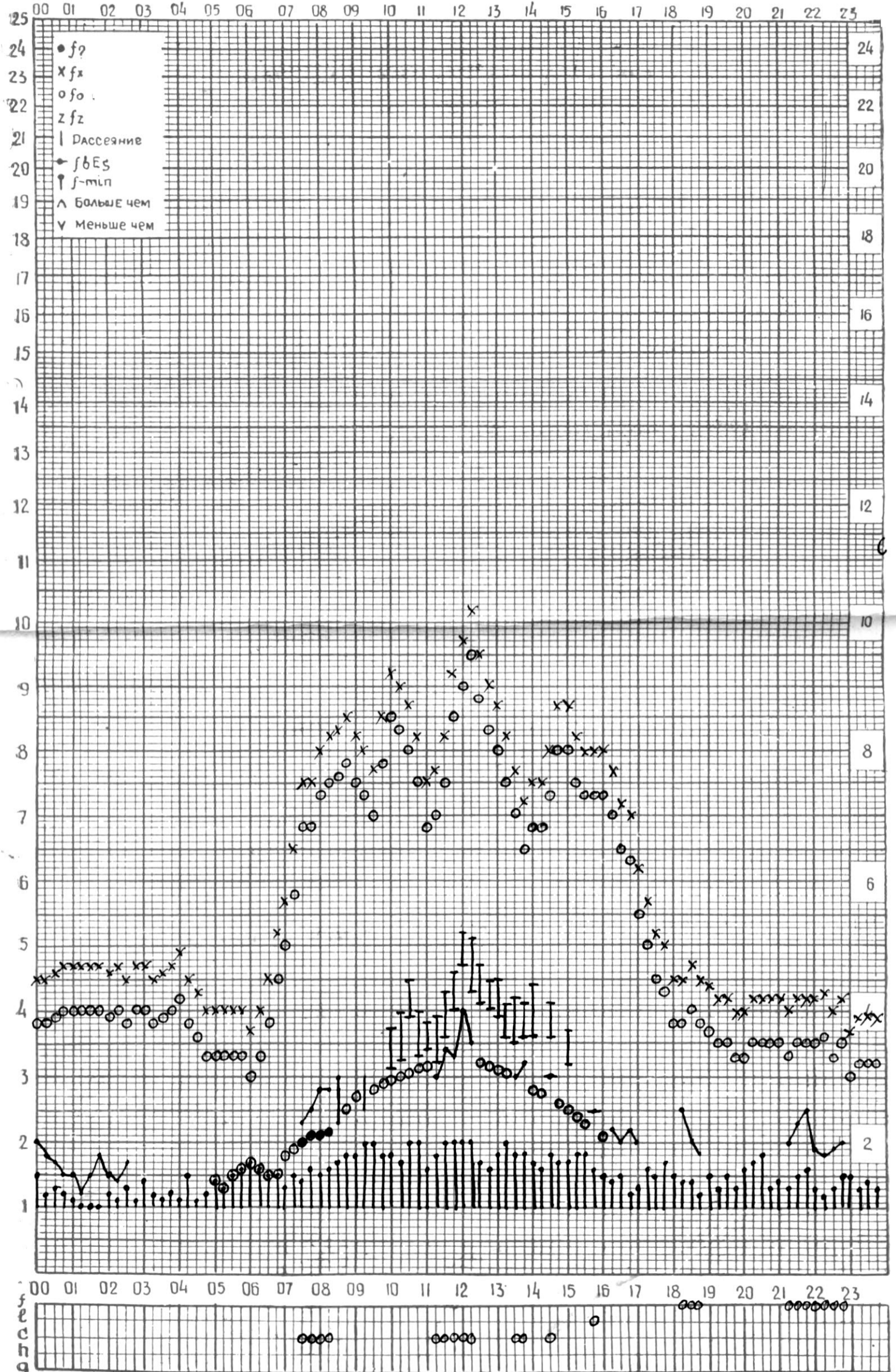
СТАНЦИЯ ТБИЛИСИ F-ГРАФИК ИОНОСФЕРНЫХ ДАННЫХ, ДАТА 8 НОЯБРЯ, 1974
