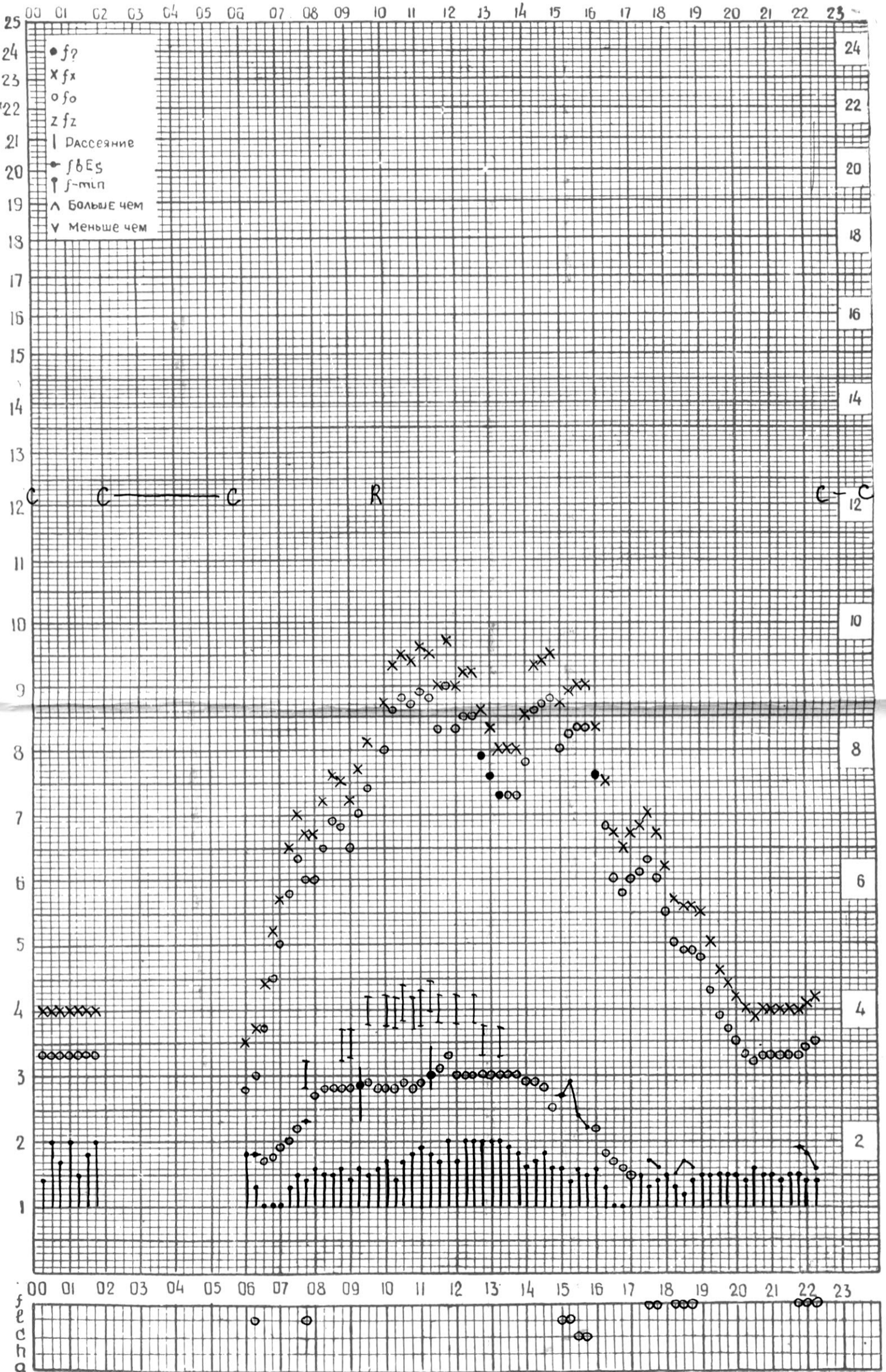
СТАНЦИЯ ТБИЛИСИ F-ГРАФИК ИОНОСФЕРНЫХ ДАННЫХ, ДАТА 9 НОЯБРЯ, 1974
