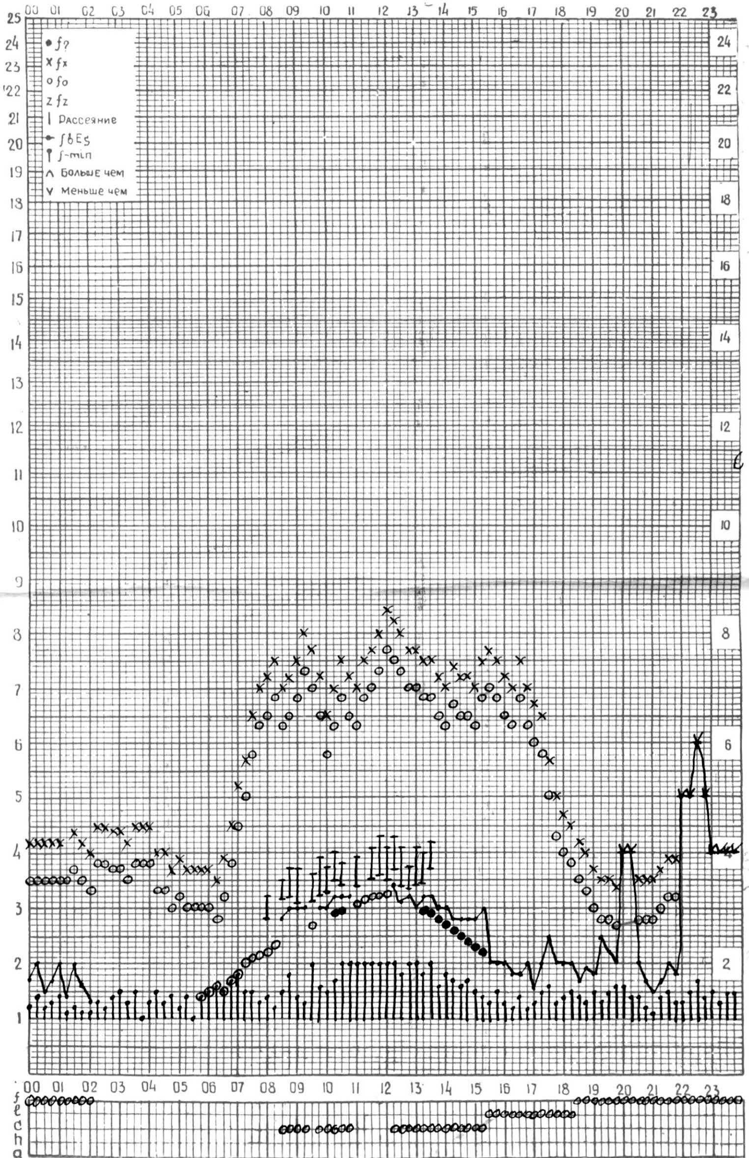
СТАНЦИЯ ТБИЛИСИ F-ГРАФИК ИОНОСФЕРНЫХ ДАННЫХ, ДАТА 20 НОЯБРЯ, 1974
