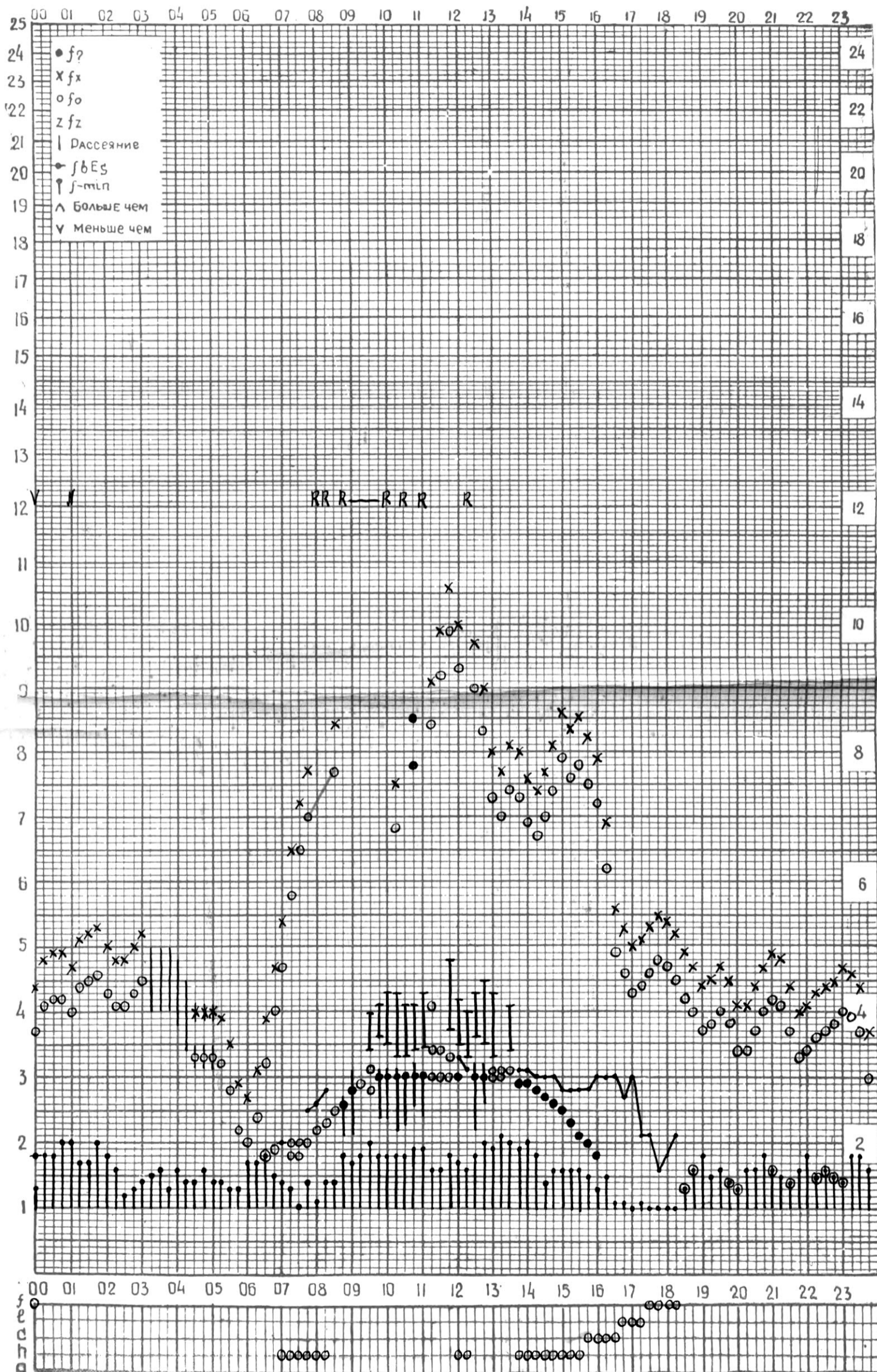
СТАНЦИЯ ТБИЛИСИ F-ГРАФИК ИОНОСФЕРНЫХ ДАННЫХ, ДАТА 11 НОЯБРЯ, 1974
