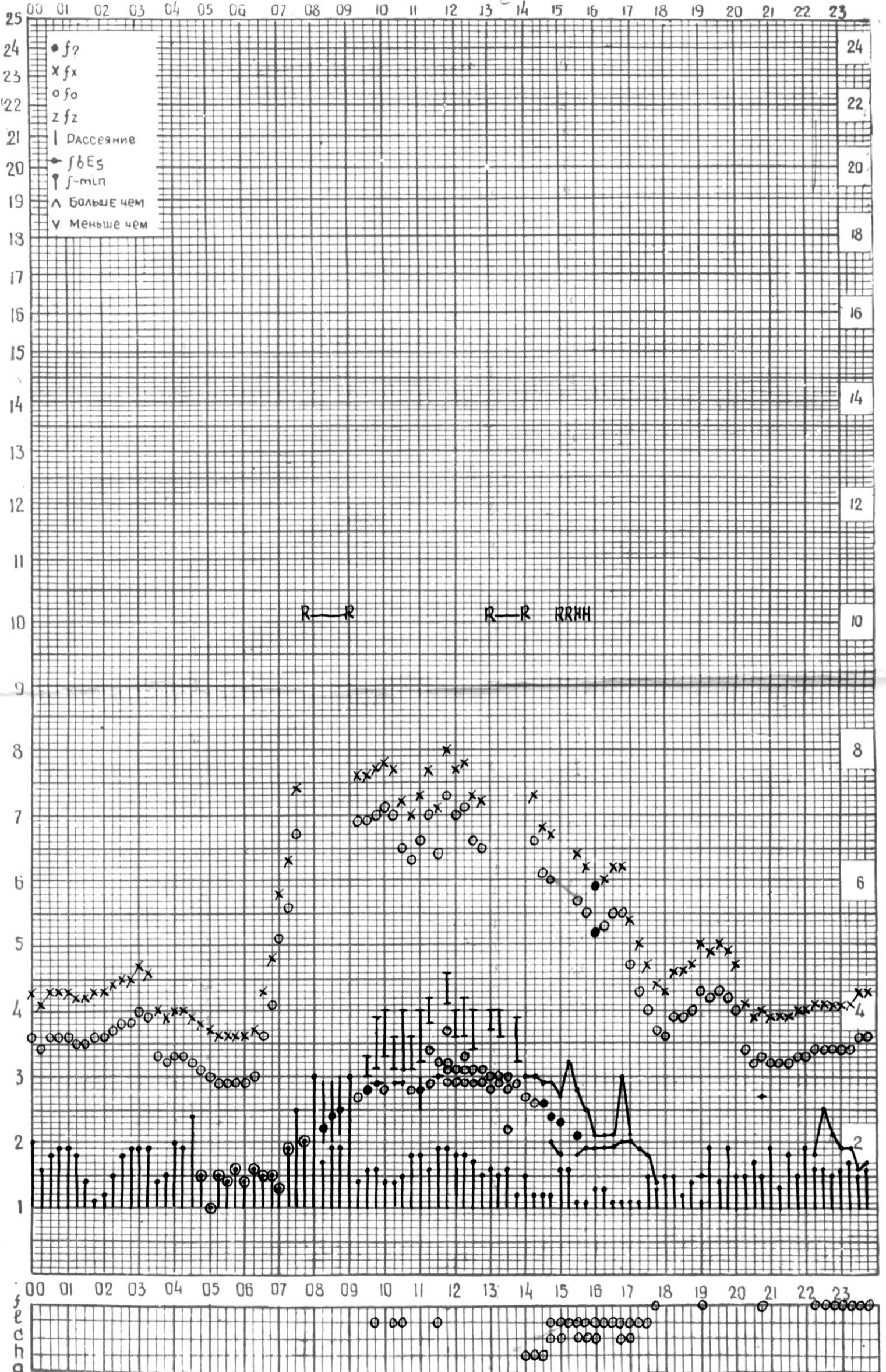
СТАНЦИЯ ТБИЛИСИ F-ГРАФИК ИОНОСФЕРНЫХ ДАННЫХ, ДАТА 19 НОЯБРЯ, 1974
