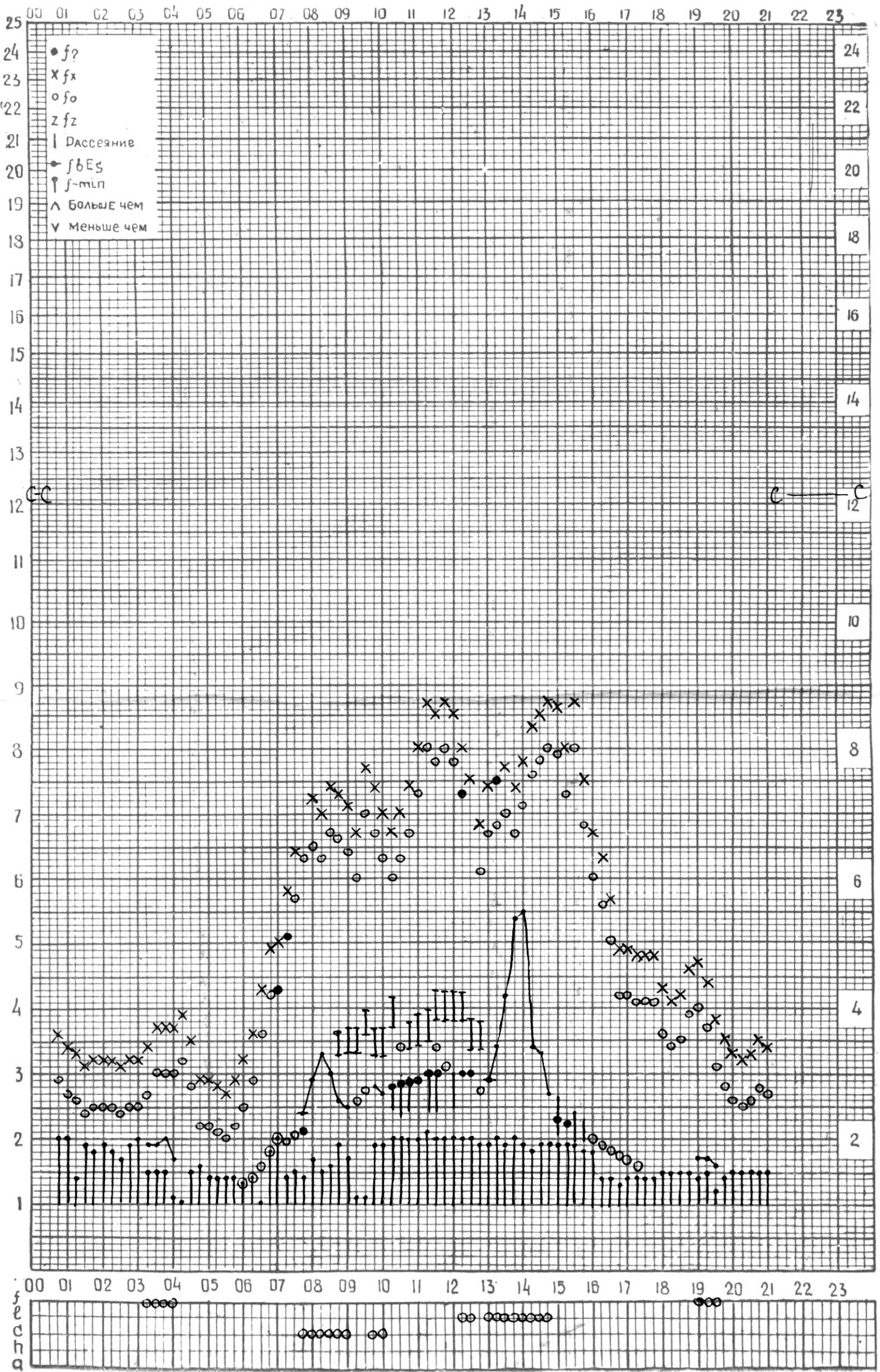
СТАНЦИЯ ТБИЛИСИ F-ГРАФИК ИОНОСФЕРНЫХ ДАННЫХ, ДАТА 13 НОЯБРЯ, 1974
