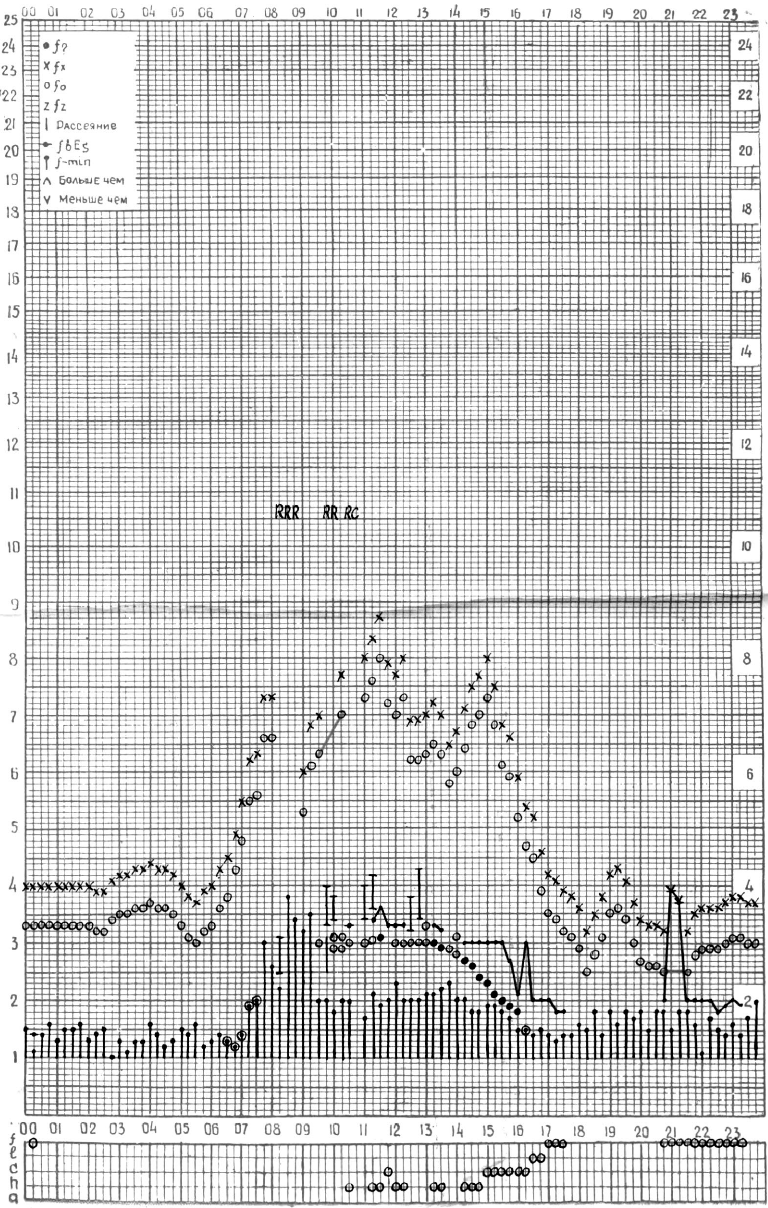
СТАНЦИЯ ТБИЛИСИ F-ГРАФИК ИОНОСФЕРНЫХ ДАННЫХ, ДАТА 28 НОЯБРЯ, 1974
