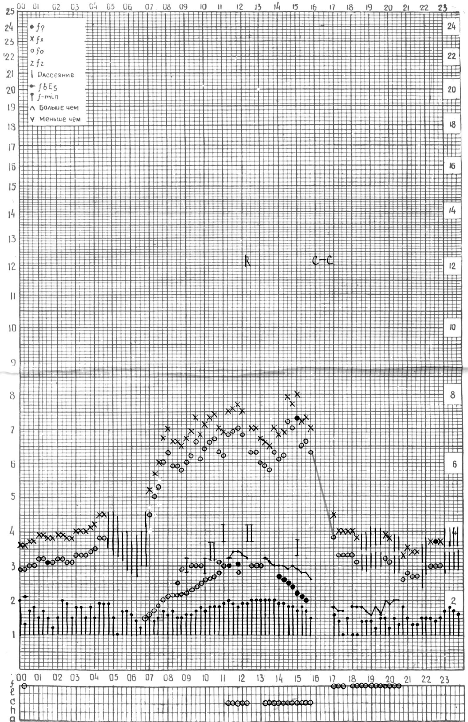
СТАНЦИЯ ТБИЛИСИ F-ГРАФИК ИОНОСФЕРНЫХ ДАННЫХ, ДАТА 29 НОЯБРЯ, 1974
