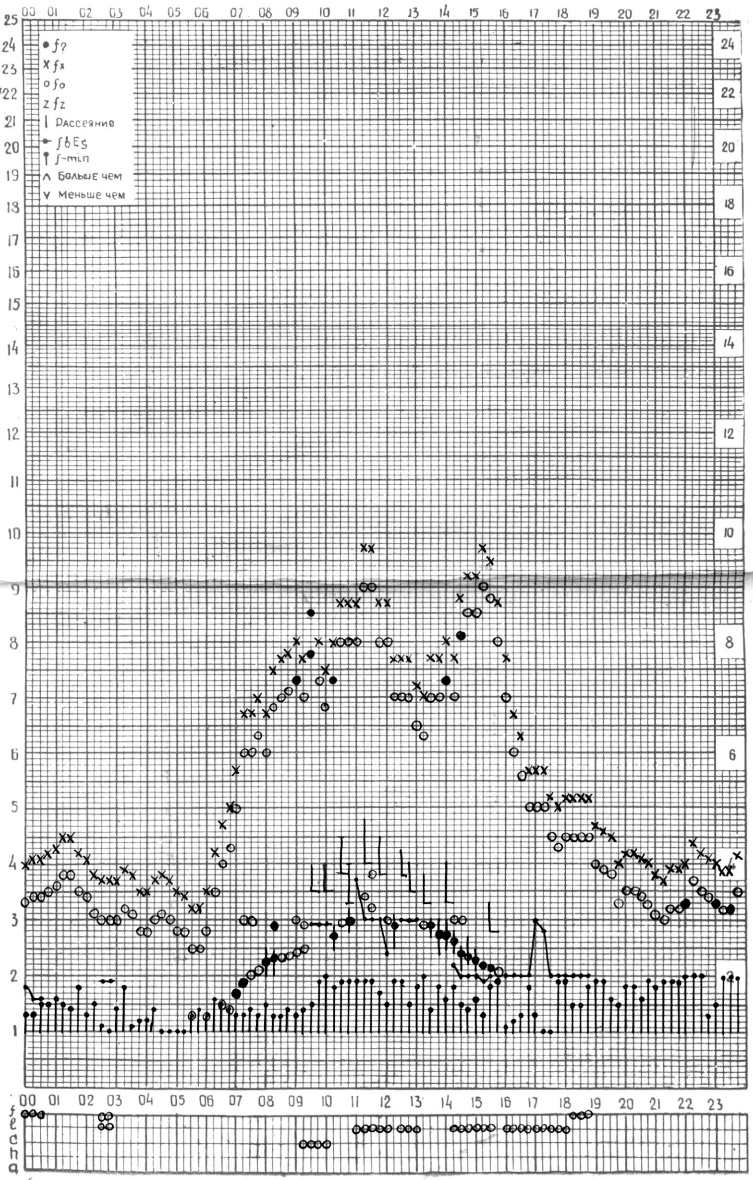
СТАНЦИЯ ТБИЛИСИ, F-ГРАФИК ИОНОСФЕРНЫХ ДАННЫХ, ДАТА 10 НОЯБРЯ, 1974
