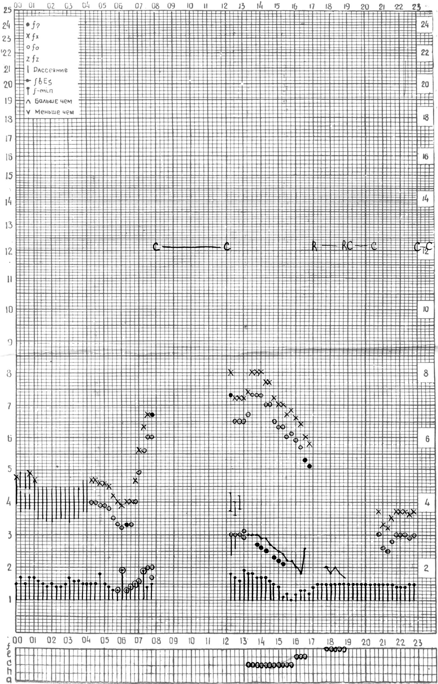
СТАНЦИЯ ТБИЛИСИ F-ГРАФИК ИОНОСФЕРНЫХ ДАННЫХ, ДАТА 25 НОЯБРЯ, 1974
