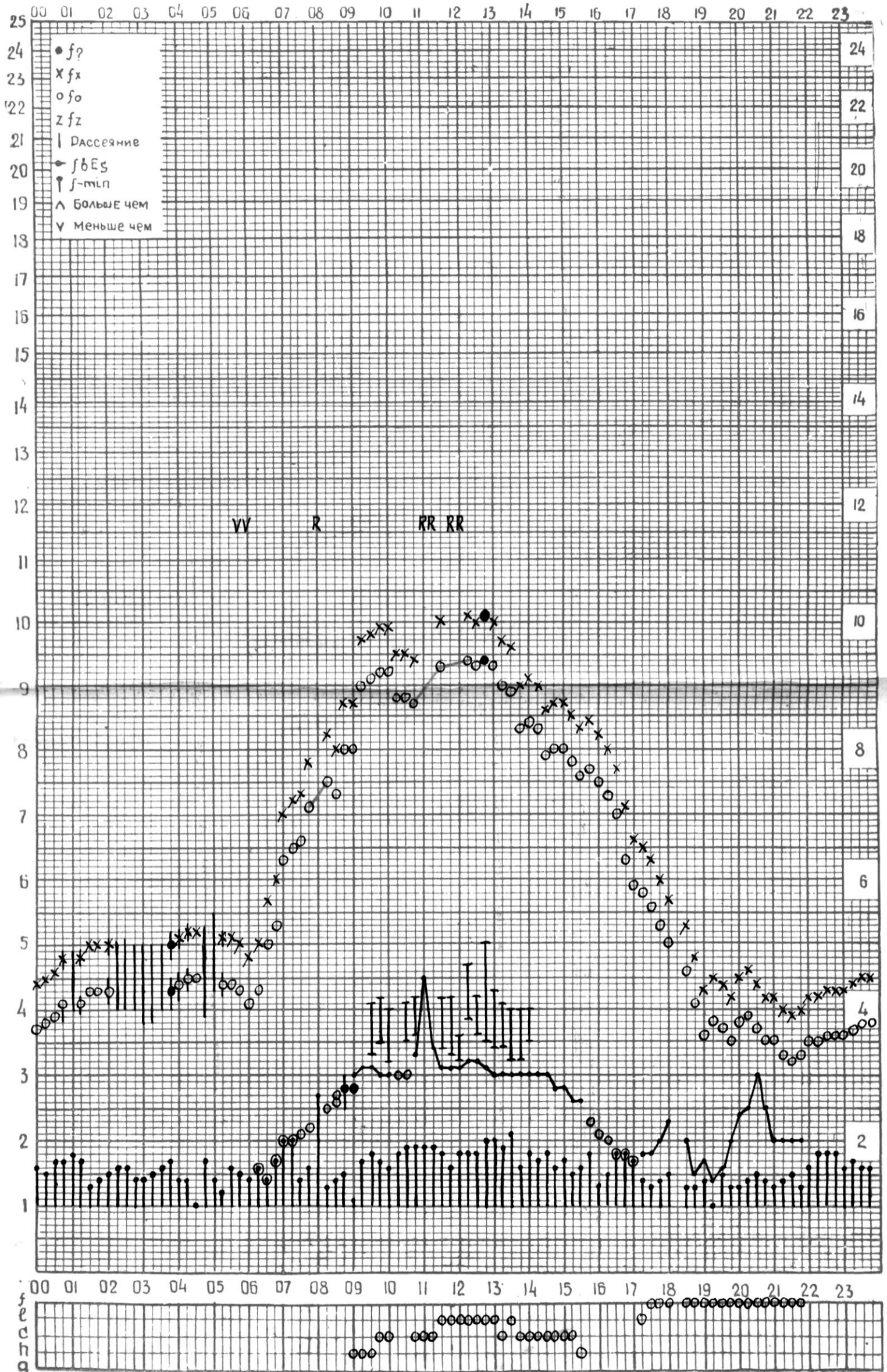
СТАНЦИЯ ТБИЛИСИ F-ГРАФИК ИОНОСФЕРНЫХ ДАННЫХ, ДАТА 7 НОЯБРЯ, 1974
