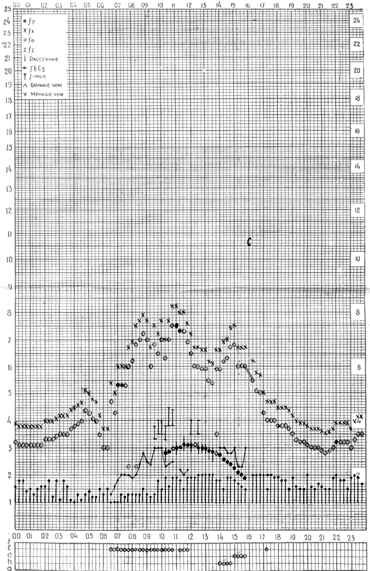
СТАНЦИЯ ТБИЛИСИ F-ГРАФИК ИОНОСФЕРНЫХ ДАННЫХ, ДАТА 18 НОЯБРЯ, 1974
