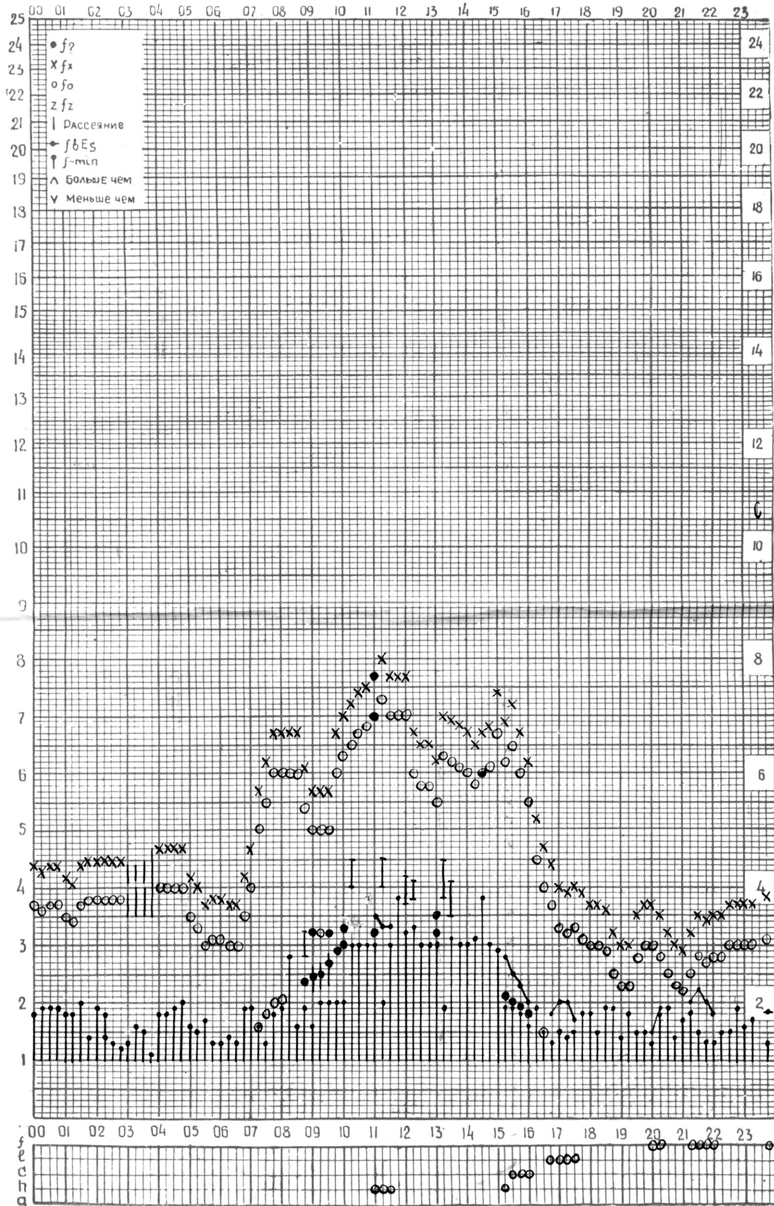
СТАНЦИЯ ТБИЛИСИ F-ГРАФИК ИОНОСФЕРНЫХ ДАННЫХ, ДАТА 30 НОЯБРЯ, 1974
