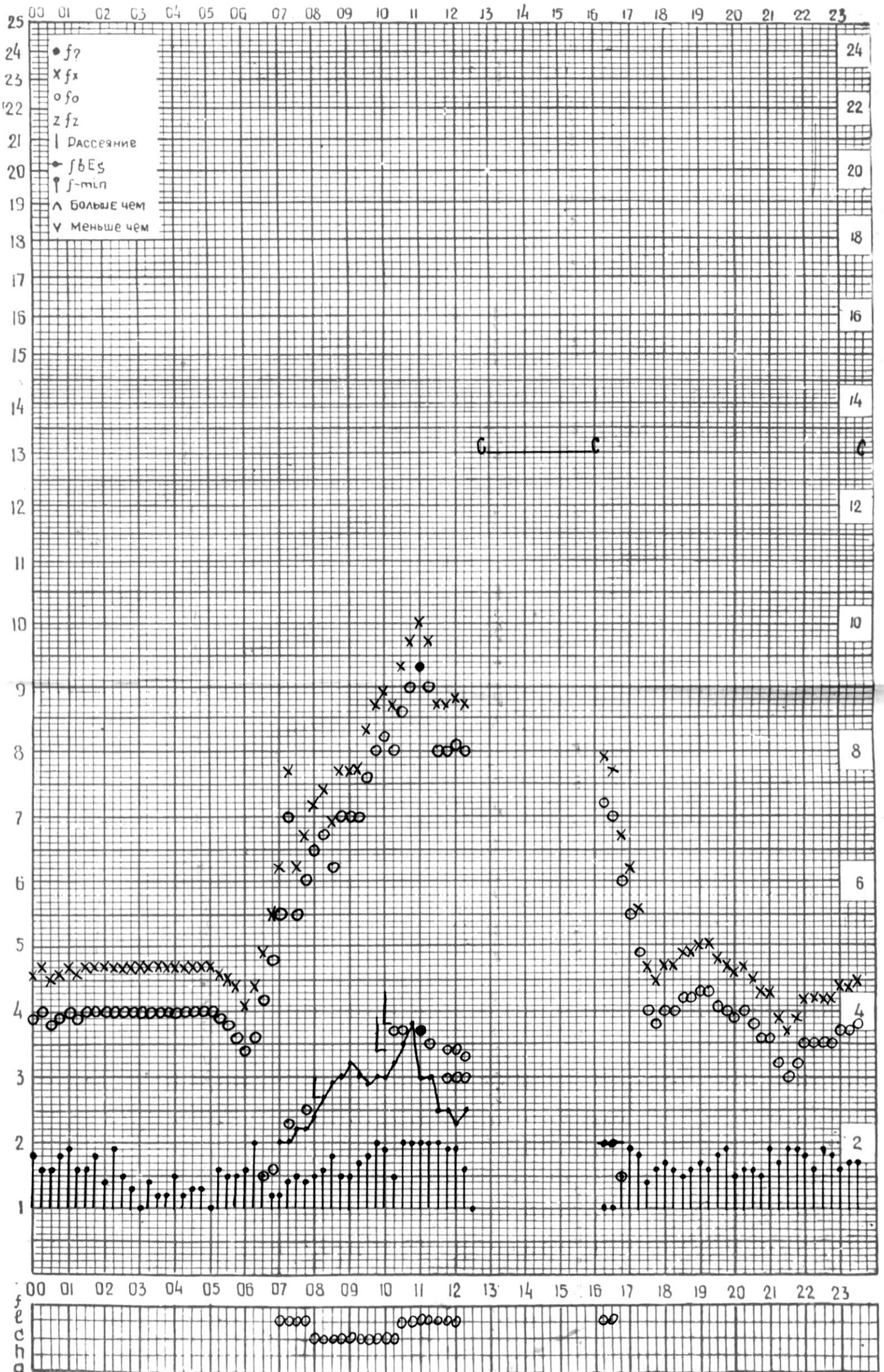
СТАНЦИЯ ТБИЛИСИ F-ГРАФИК ИОНОСФЕРНЫХ ДАННЫХ, ДАТА 2 НОЯБРЯ, 1974
