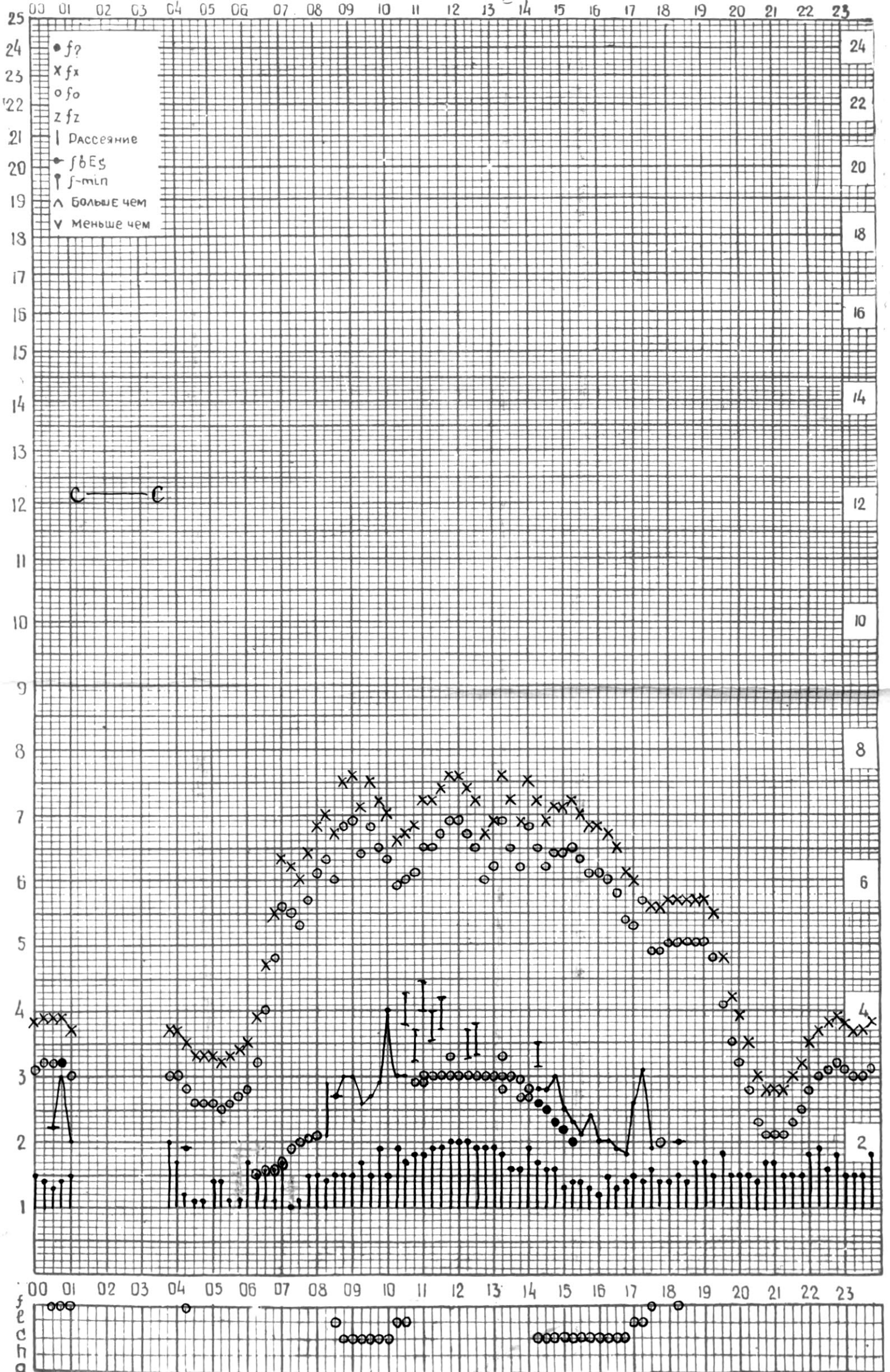
СТАНЦИЯ ТБИЛИСИ F-ГРАФИК ИОНОСФЕРНЫХ ДАННЫХ, ДАТА 17 НОЯБРЯ, 1974
