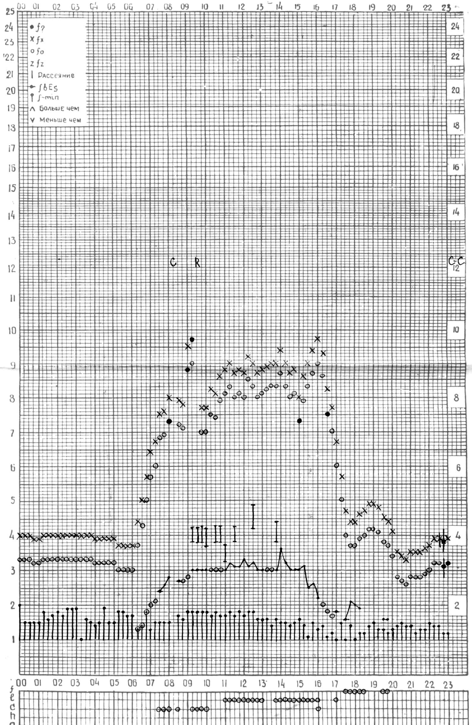
СТАНЦИЯ ТБИЛИСИ F-ГРАФИК ИОНОСФЕРНЫХ ДАННЫХ, ДАТА 5 НОЯБРЯ, 1974
