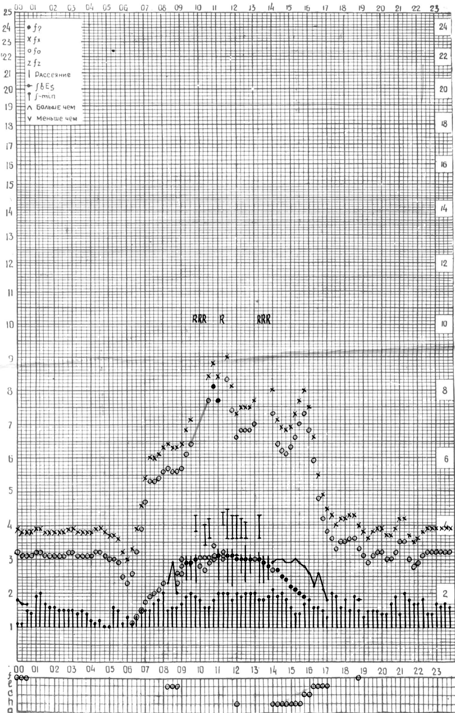
СТАНЦИЯ ТБИЛИСИ F-ГРАФИК ИОНОСФЕРНЫХ ДАННЫХ, ДАТА 23 НОЯБРЯ, 1974
