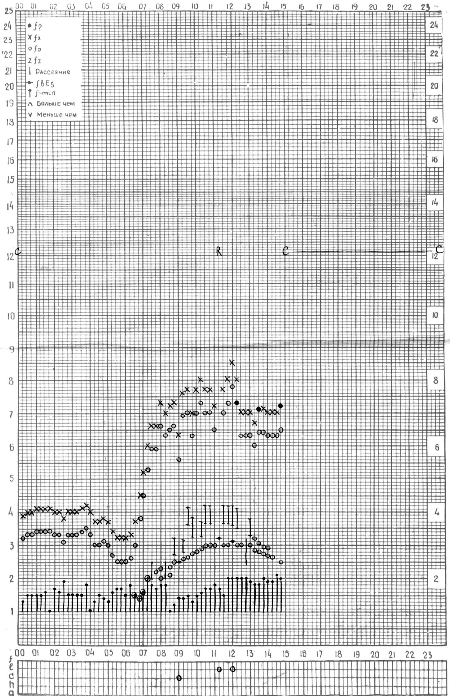
СТАНЦИЯ ТБИЛИСИ F-ГРАФИК ИОНОСФЕРНЫХ ДАННЫХ, ДАТА 21 НОЯБРЯ, 1974
