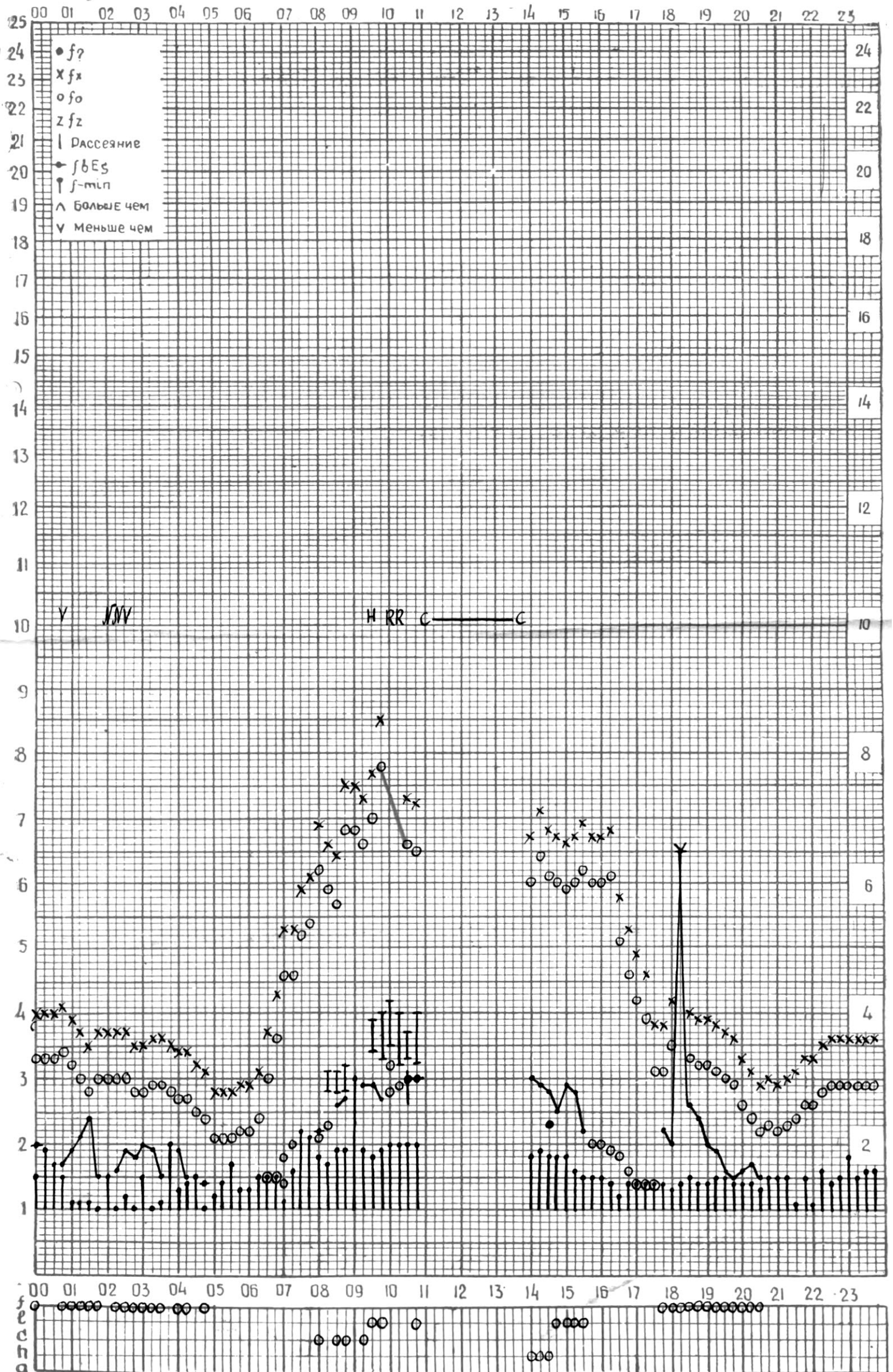
СТАНЦИЯ ТБИЛИСИ F-ГРАФИК ИОНОСФЕРНЫХ ДАННЫХ, ДАТА 15 НОЯБРЯ, 1974
