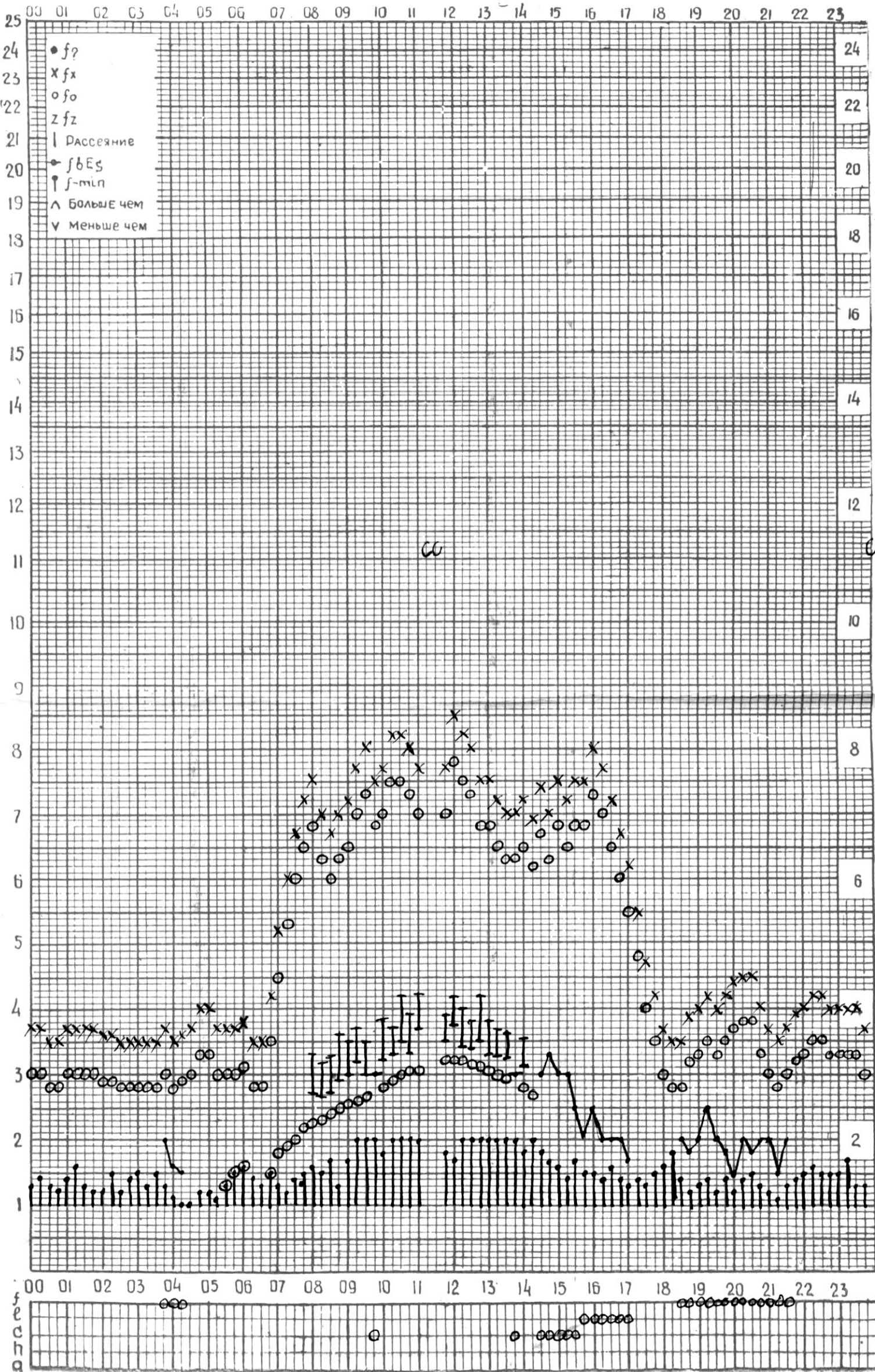
СТАНЦИЯ ТБИЛИСИ F-ГРАФИК ИОНОСФЕРНЫХ ДАННЫХ, ДАТА 16 НОЯБРЯ, 1974
