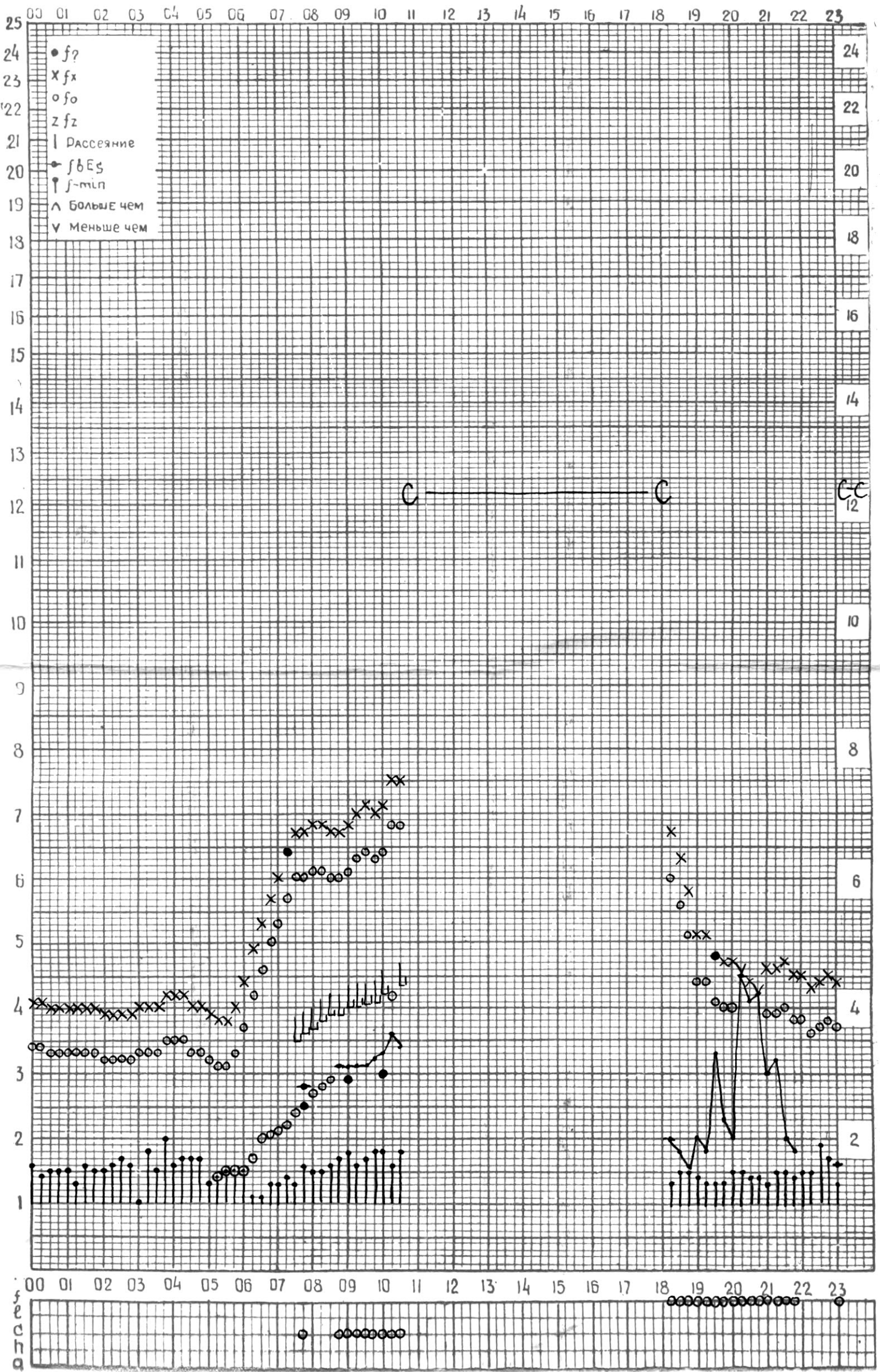
СТАНЦИЯ ТБИЛИСИ F-ГРАФИК ИОНОСФЕРНЫХ ДАННЫХ, ДАТА 4 ОКТЯБРЯ, 1974
