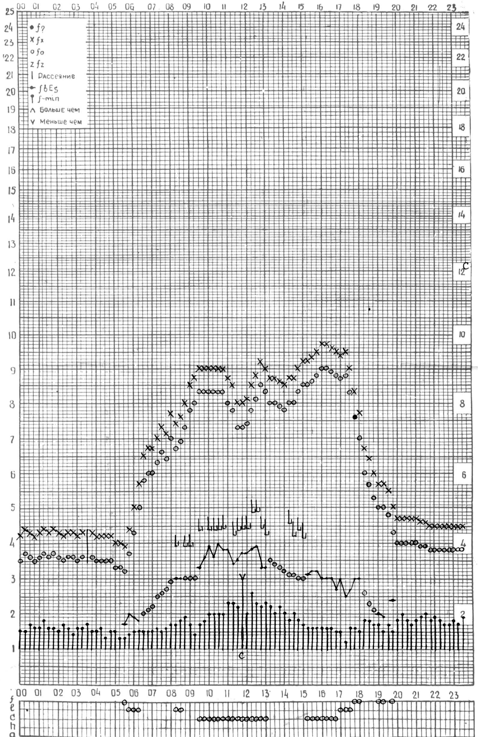
СТАНЦИЯ ТБИЛИСИ F-ГРАФИК ИОНОСФЕРНЫХ ДАННЫХ, ДАТА 8 ОКТЯБРЯ, 1974
