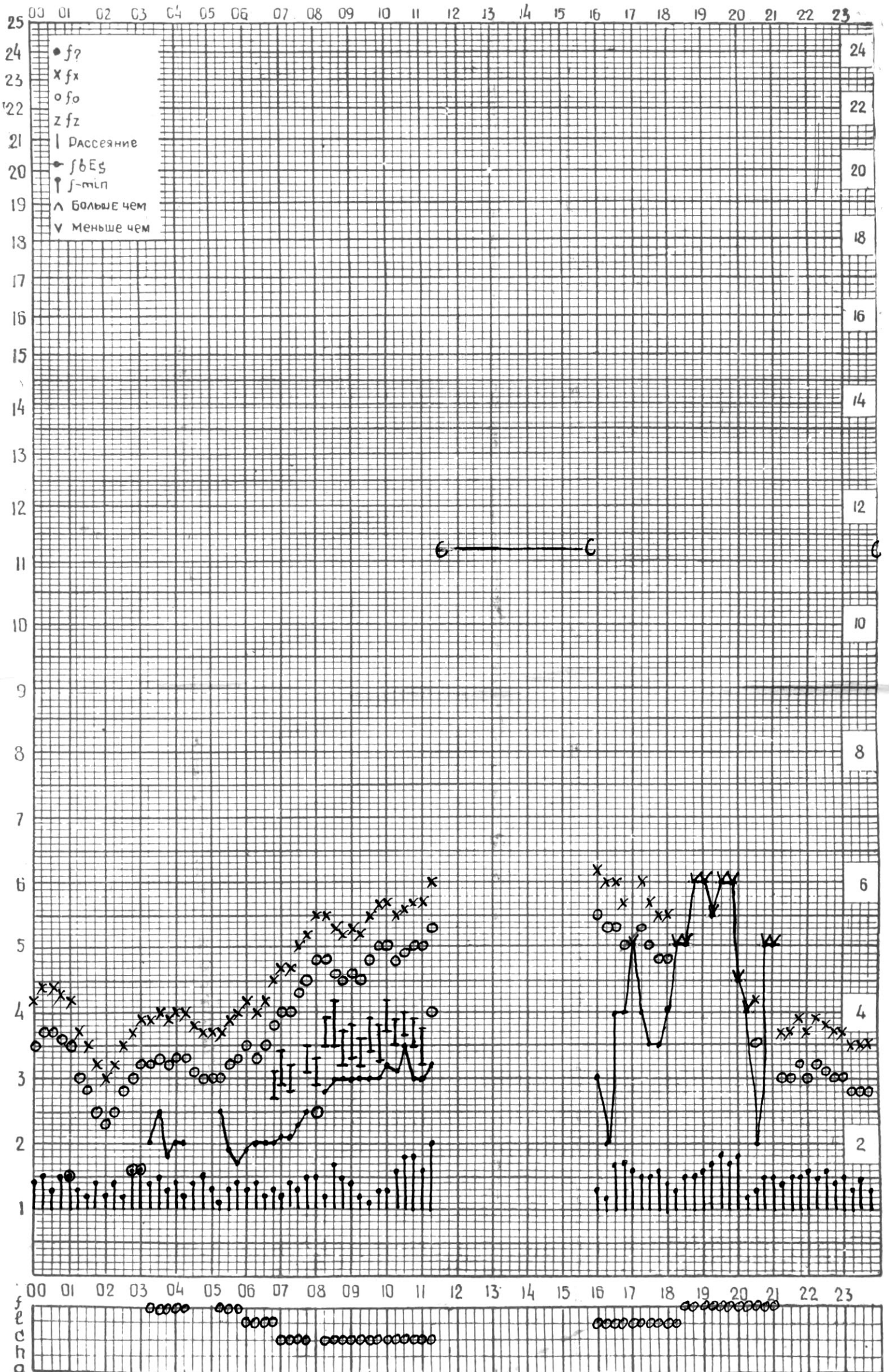
СТАНЦИЯ ТБИЛИСИ F-ГРАФИК ИОНОСФЕРНЫХ ДАННЫХ, ДАТА 15 ОКТЯБРЯ, 1974
