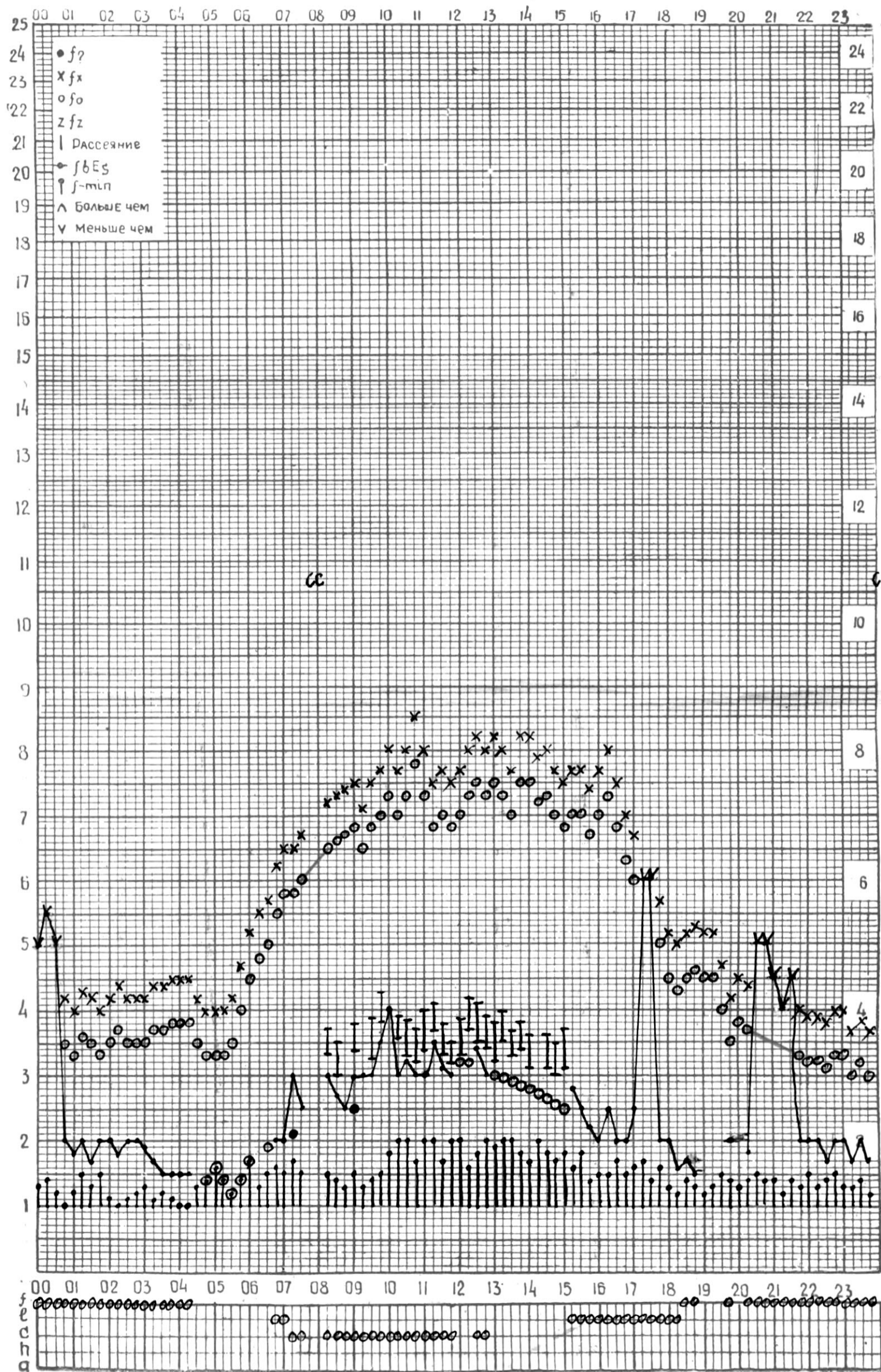
СТАНЦИЯ ТБИЛИСИ F-ГРАФИК ИОНОСФЕРНЫХ ДАННЫХ, ДАТА 23 ОКТЯБРЯ, 1974
