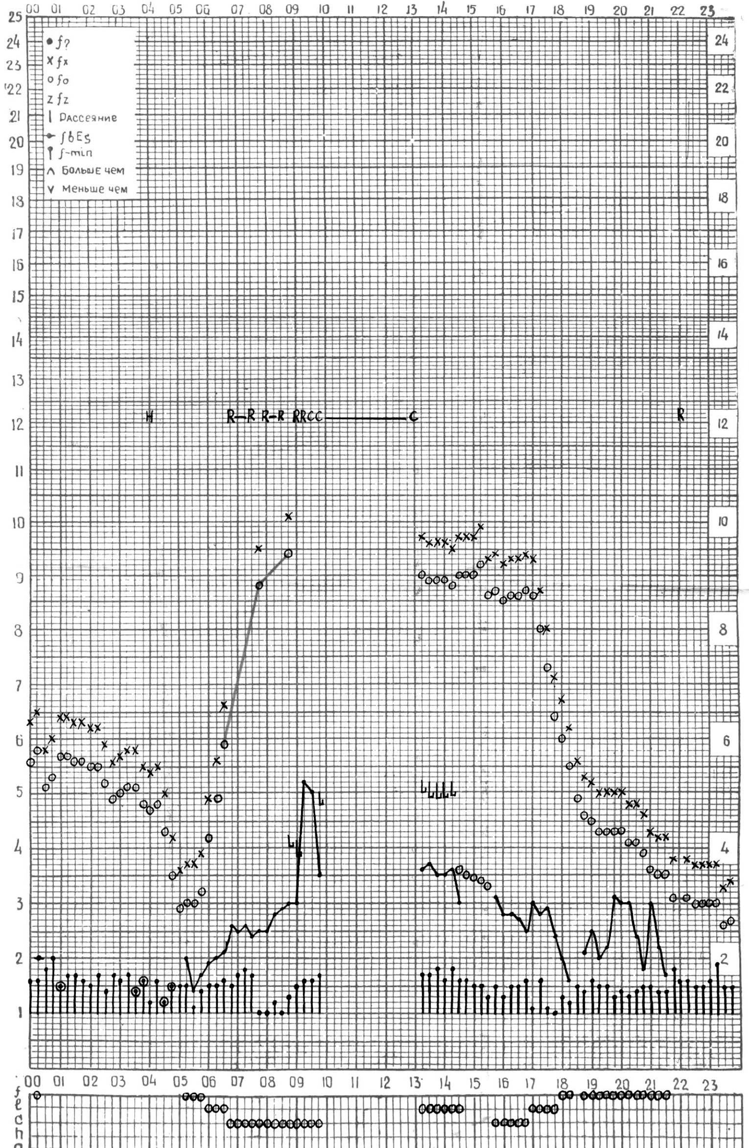
СТАНЦИЯ ТБИЛИСИ F-ГРАФИК ИОНОСФЕРНЫХ ДАННЫХ, ДАТА 14 ОКТЯБРЯ, 1974
