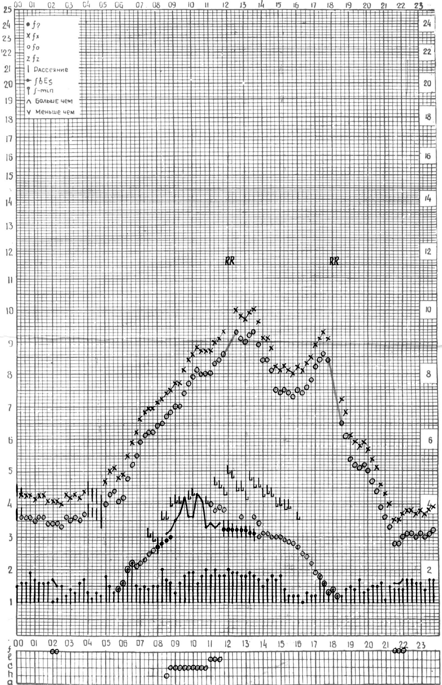
СТАНЦИЯ ТБИЛИСИ F-ГРАФИК ИОНОСФЕРНЫХ ДАННЫХ, ДАТА 6 ОКТЯБРЯ, 1974
