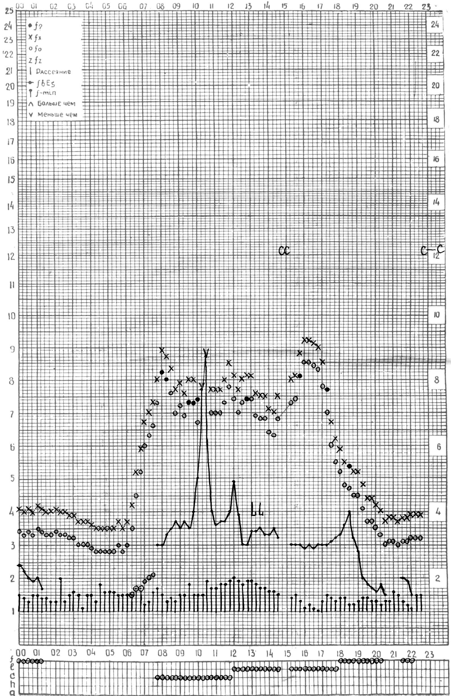
СТАНЦИЯ ТБИЛИСИ F-ГРАФИК ИОНОСФЕРНЫХ ДАННЫХ, ДАТА 28 ОКТЯБРЯ, 1974
