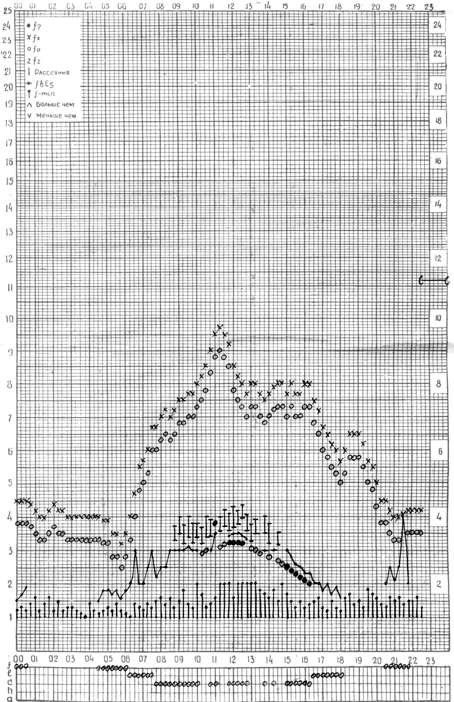
СТАНЦИЯ ТБИЛИСИ F-ГРАФИК ИОНОСФЕРНЫХ ДАННЫХ, ДАТА 27 ОКТЯБРЯ, 1974
