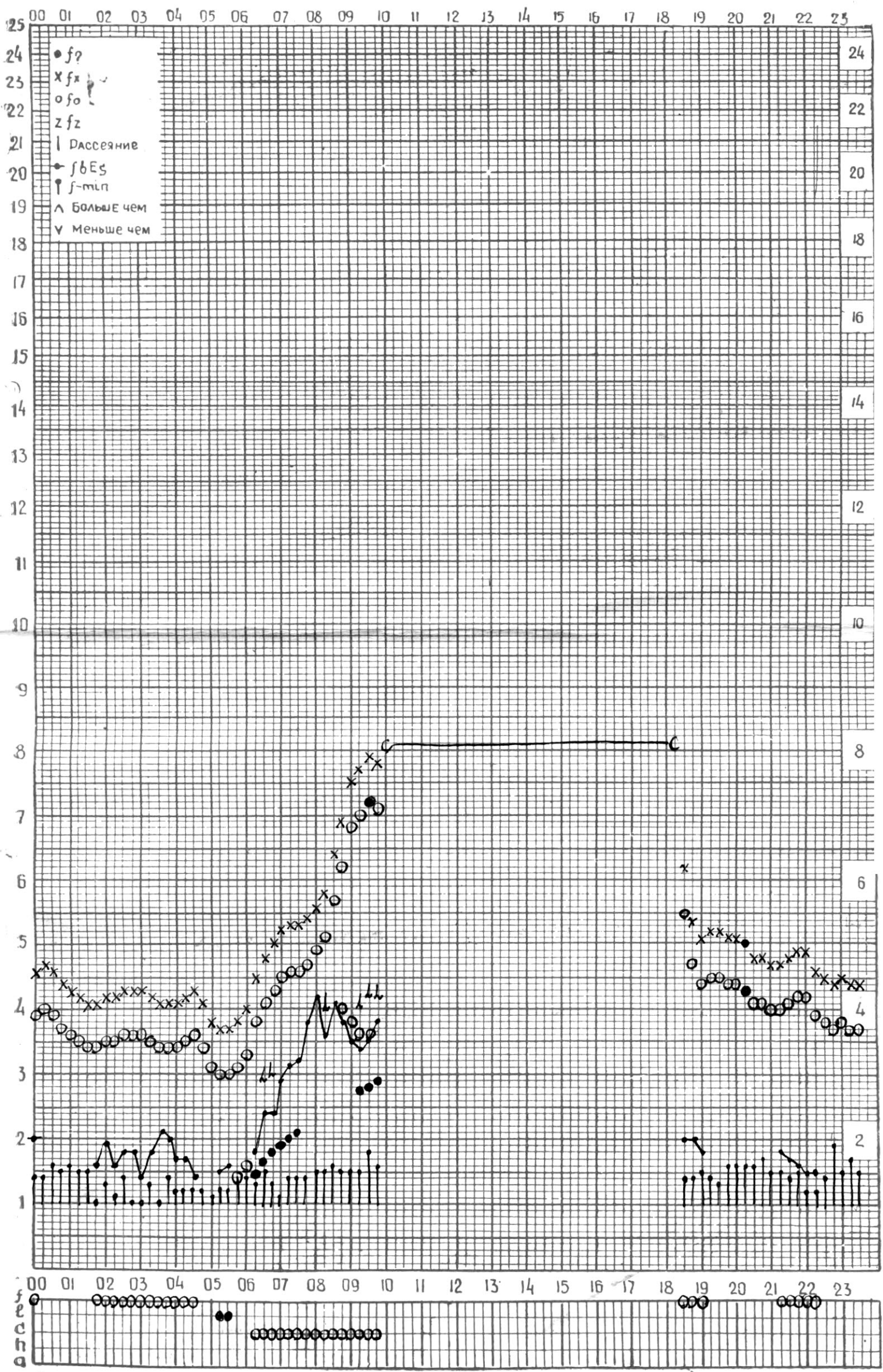
СТАНЦИЯ ТБИЛИСИ F—ГРАФИК ИОНОСФЕРНЫХ ДАННЫХ, ДАТА 3 ОКТЯБРЯ 1974
