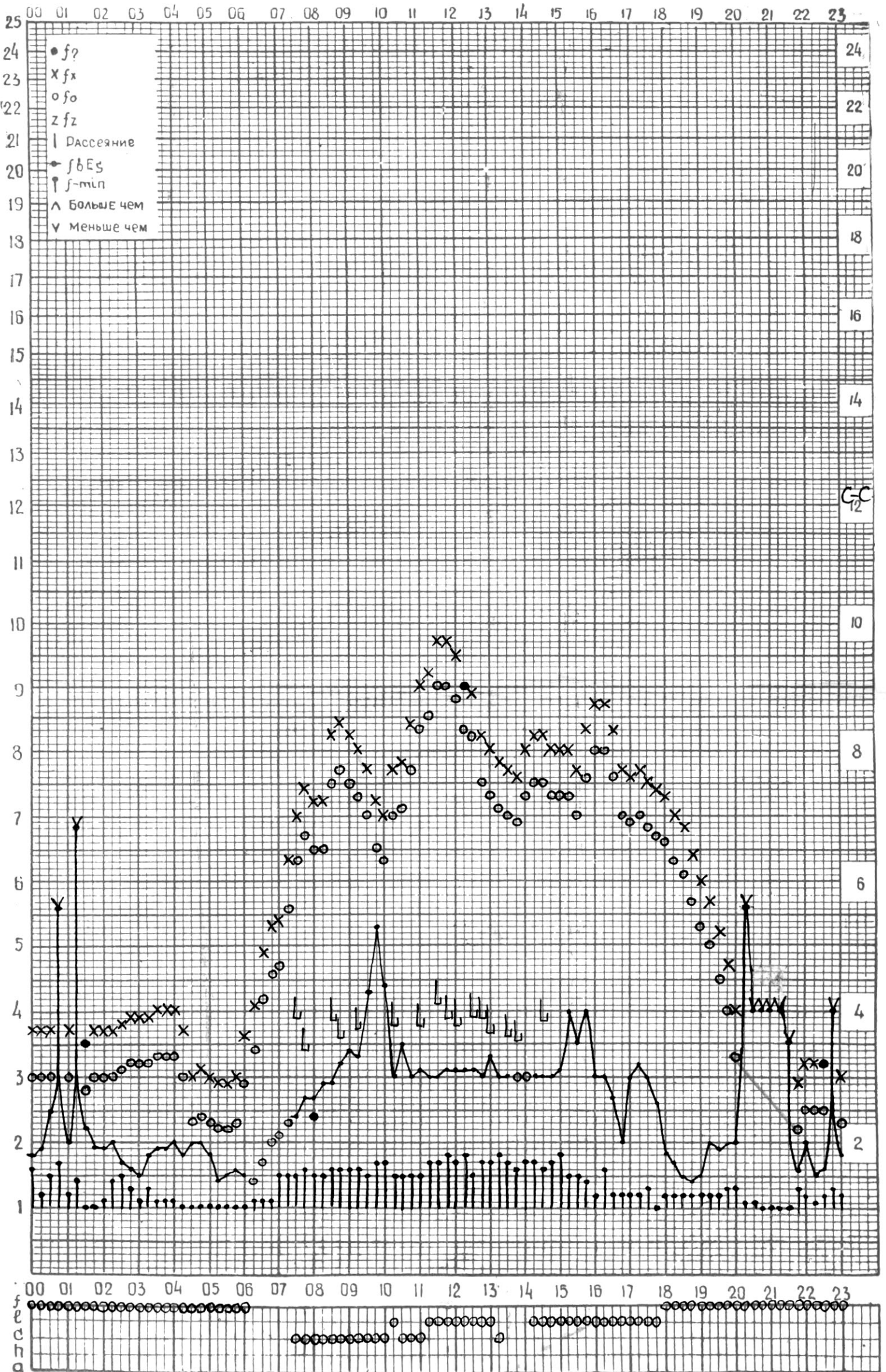
СТАНЦИЯ ТБИЛИСИ F-ГРАФИК ИОНОСФЕРНЫХ ДАННЫХ, ДАТА 19 ОКТЯБРЯ, 1974
