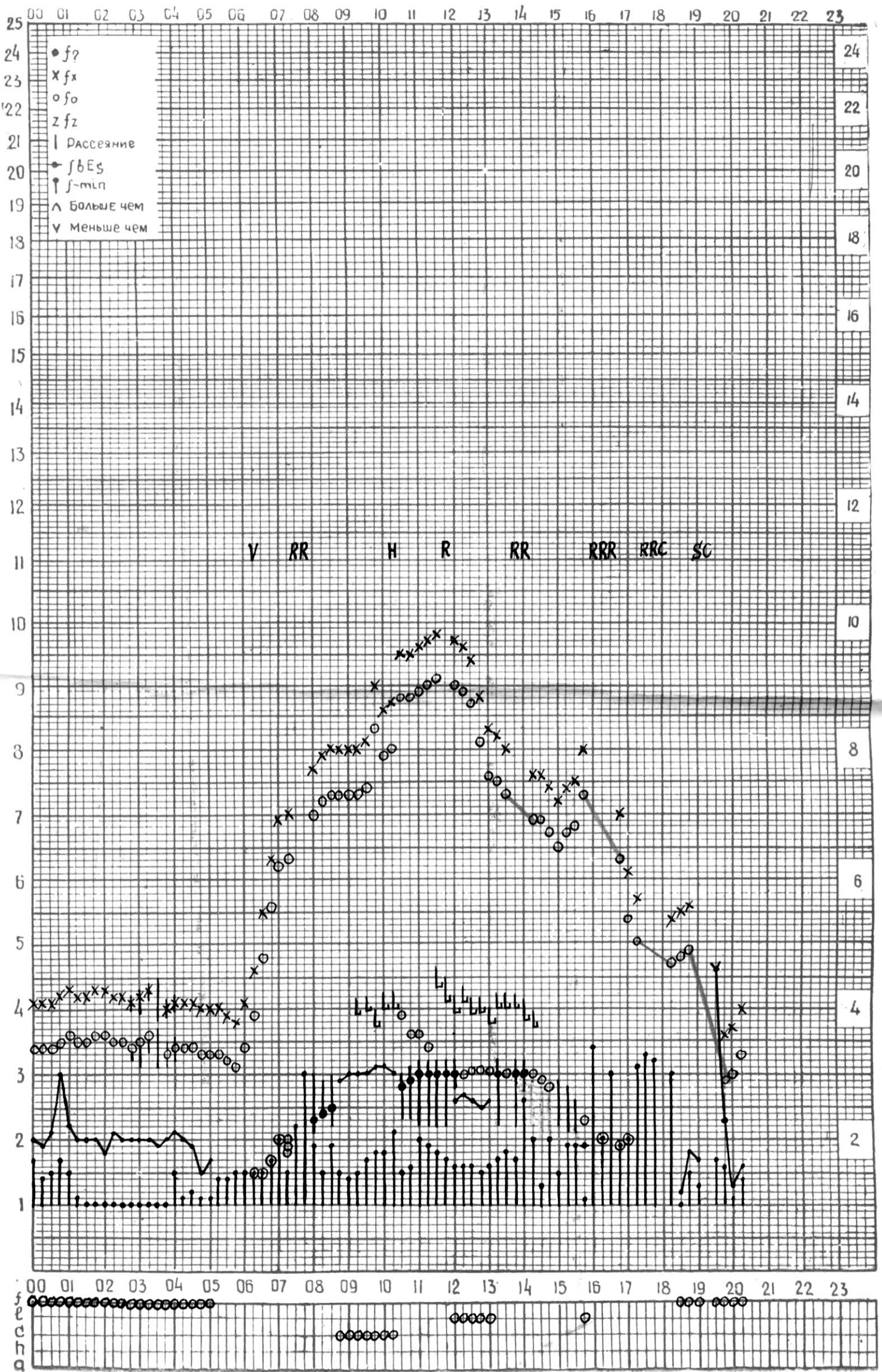
СТАНЦИЯ ТБИЛИСИ F-ГРАФИК ИОНОСФЕРНЫХ ДАННЫХ, ДАТА 30 ОКТЯБРЯ, 1974
