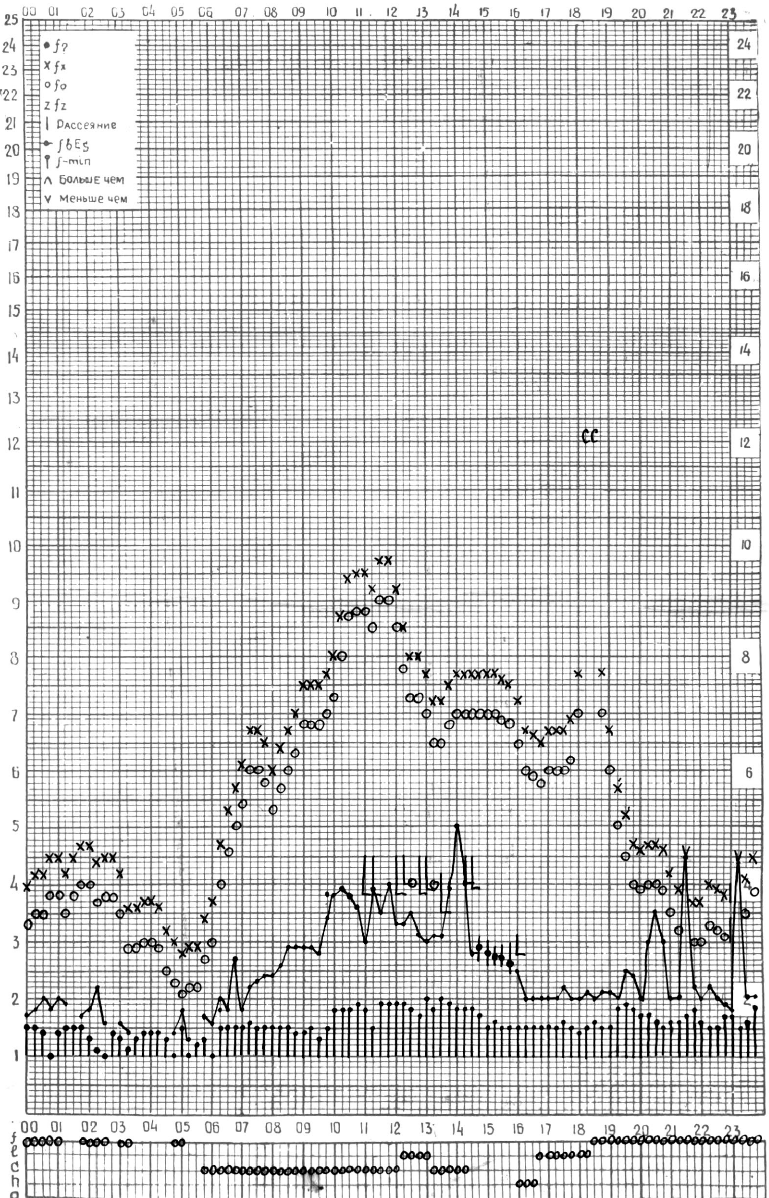
СТАНЦИЯ ТБИЛИСИ F-ГРАФИК ИОНОСФЕРНЫХ ДАННЫХ, ДАТА 17 ОКТЯБРЯ, 1974
