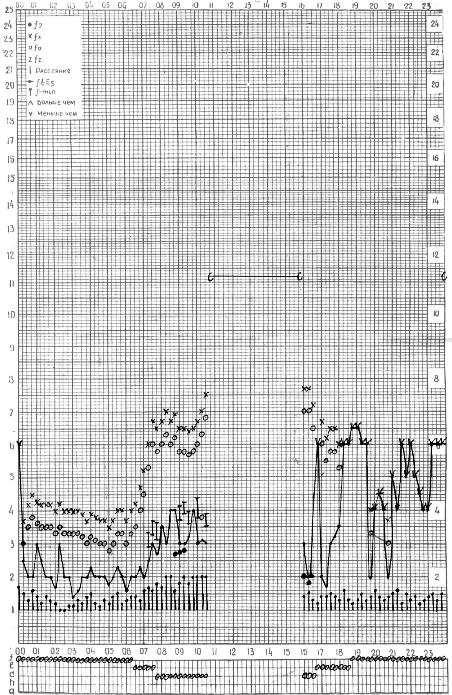
СТАНЦИЯ ТБИЛИСИ F-ГРАФИК ИОНОСФЕРНЫХ ДАННЫХ, ДАТА 18 ОКТЯБРЯ, 1974
