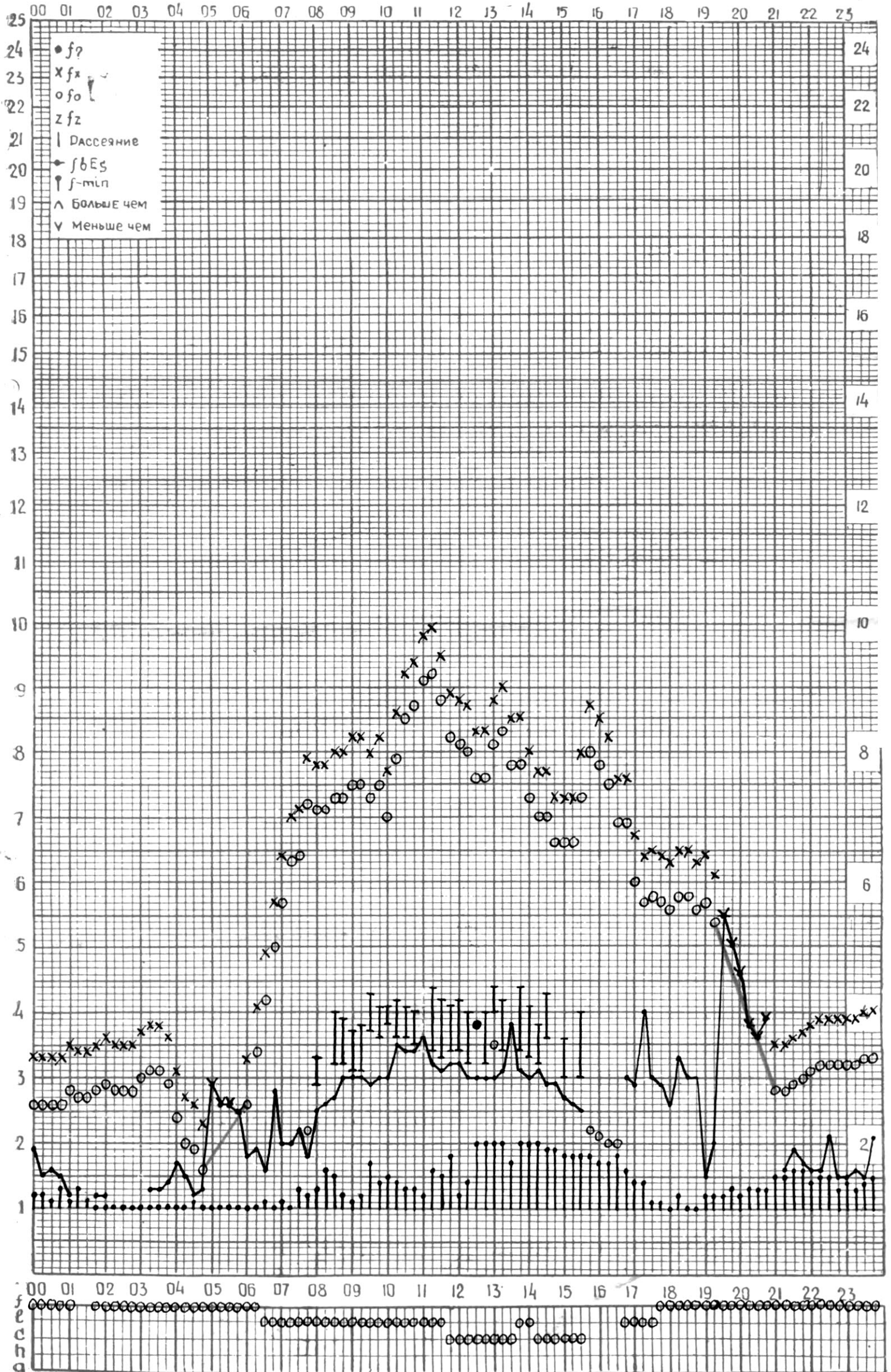
СТАНЦИЯ ТБИЛИСИ F-ГРАФИК ИОНОСФЕРНЫХ ДАННЫХ, ДАТА 20 ОКТЯБРЯ, 1974
