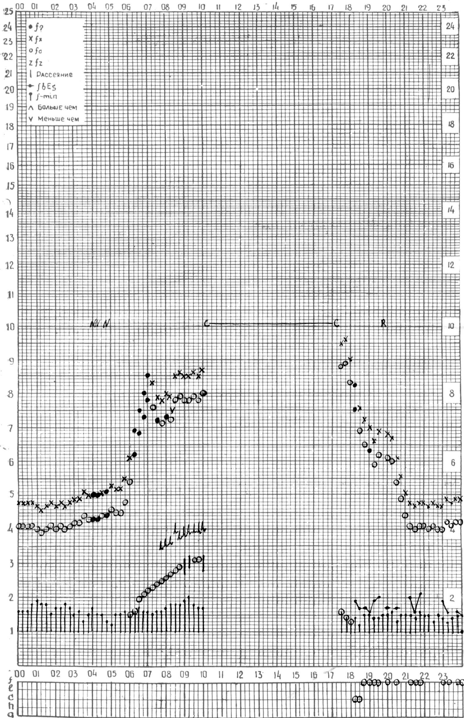
СТАНЦИЯ ТБИЛИСИ F-ГРАФИК ИОНОСФЕРНЫХ ДАННЫХ, ДАТА 11 ОКТЯБРЯ, 1974
