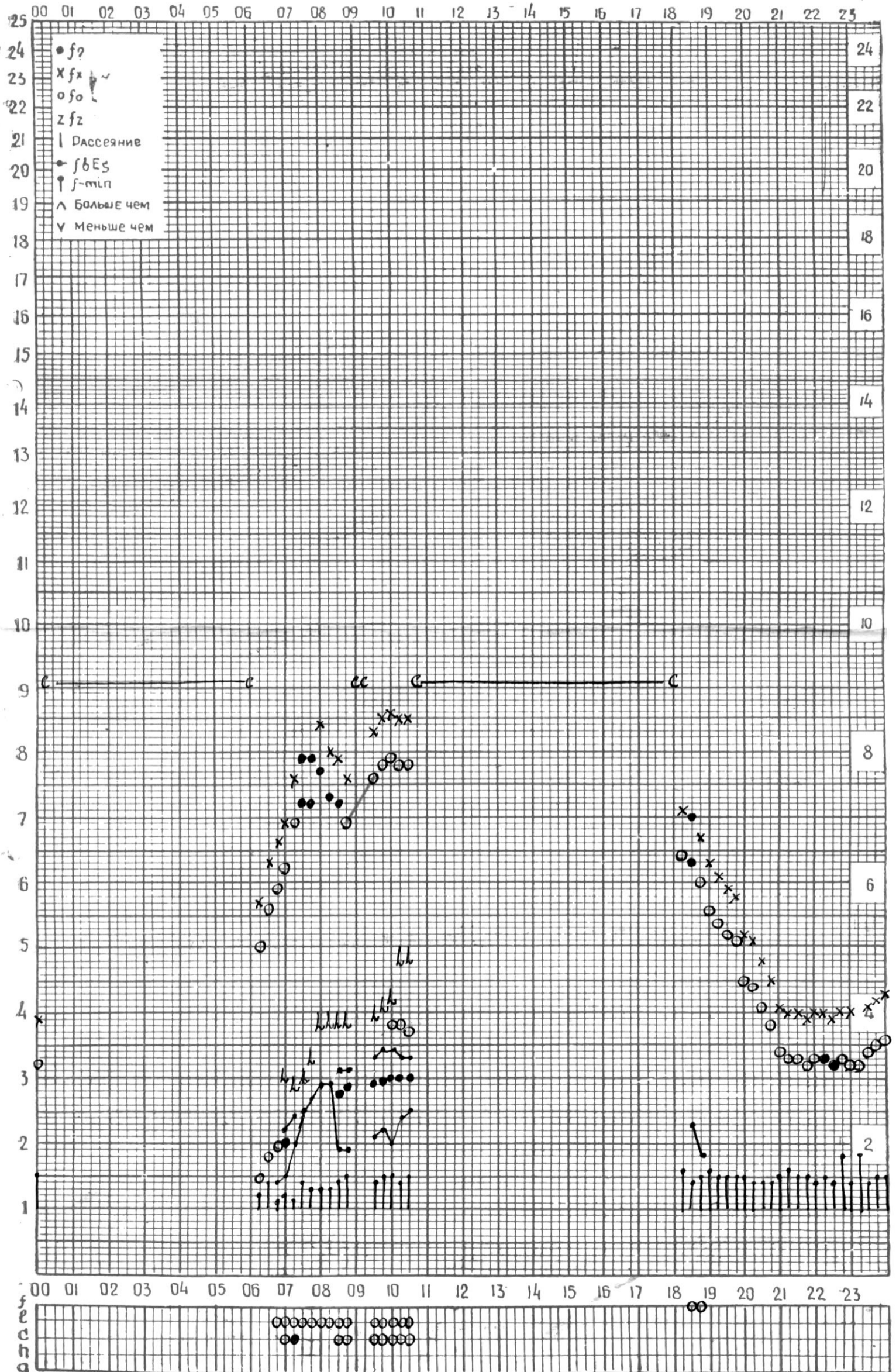
СТАНЦИЯ ТБИЛИСИ F-ГРАФИК ИОНОСФЕРНЫХ ДАННЫХ, ДАТА 7 ОКТЯБРЯ, 1974
