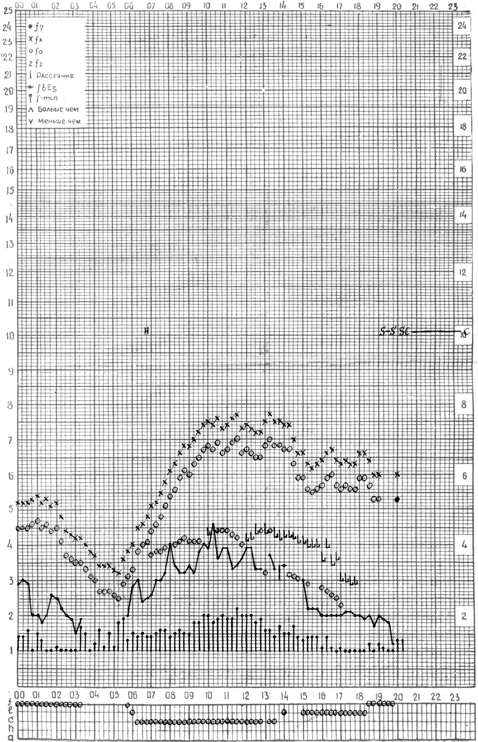
СТАНЦИЯ ТБИЛИСИ F-ГРАФИК ИОНОСФЕРНЫХ ДАННЫХ, ДАТА 4 СЕНТЯБРЯ 1974
