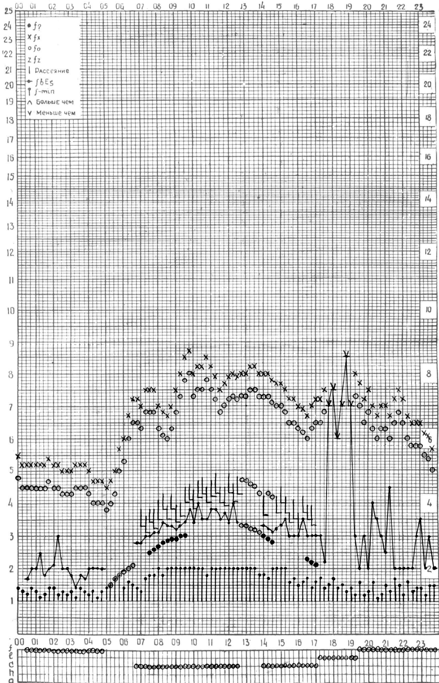
СТАНЦИЯ ТБИЛИСИ F-ГРАФИК ИОНОСФЕРНЫХ ДАННЫХ, ДАТА 11 СЕНТЯБРЯ, 1974
