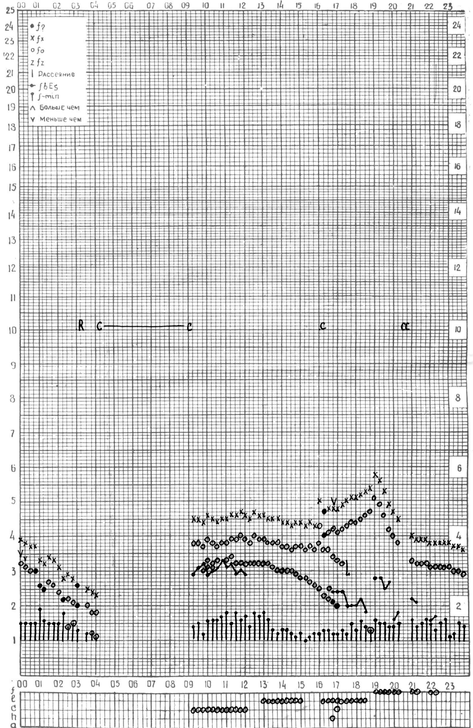
СТАНЦИЯ ТБИЛИСИ F-ГРАФИК ИОНОСФЕРНЫХ ДАННЫХ, ДАТА 16 СЕНТЯБРЯ, 1974
