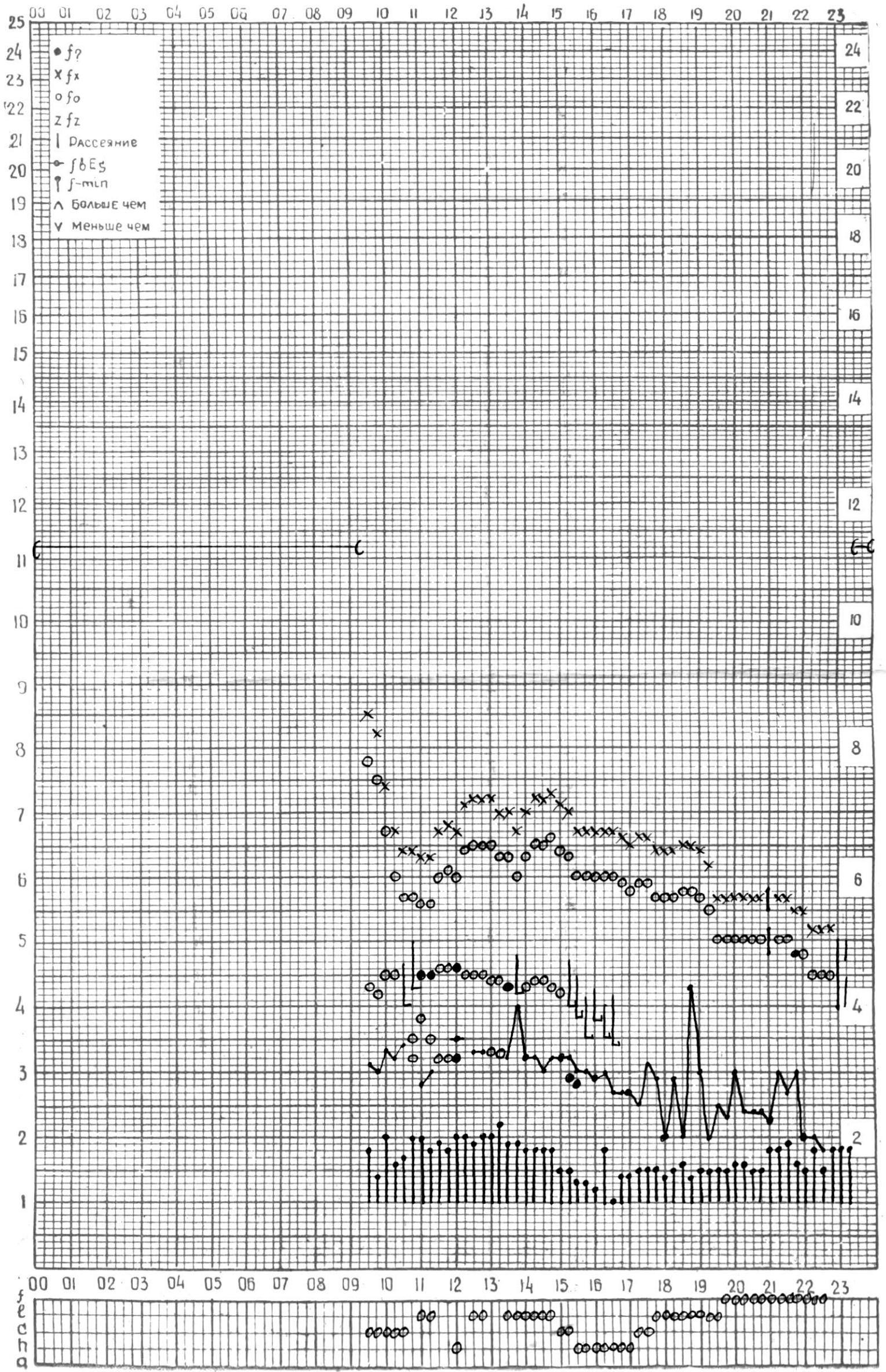
СТАНЦИЯ ТБИЛИСИ F-ГРАФИК ИОНОСФЕРНЫХ ДАННЫХ, ДАТА 6 СЕНТЯБРЯ, 1974
