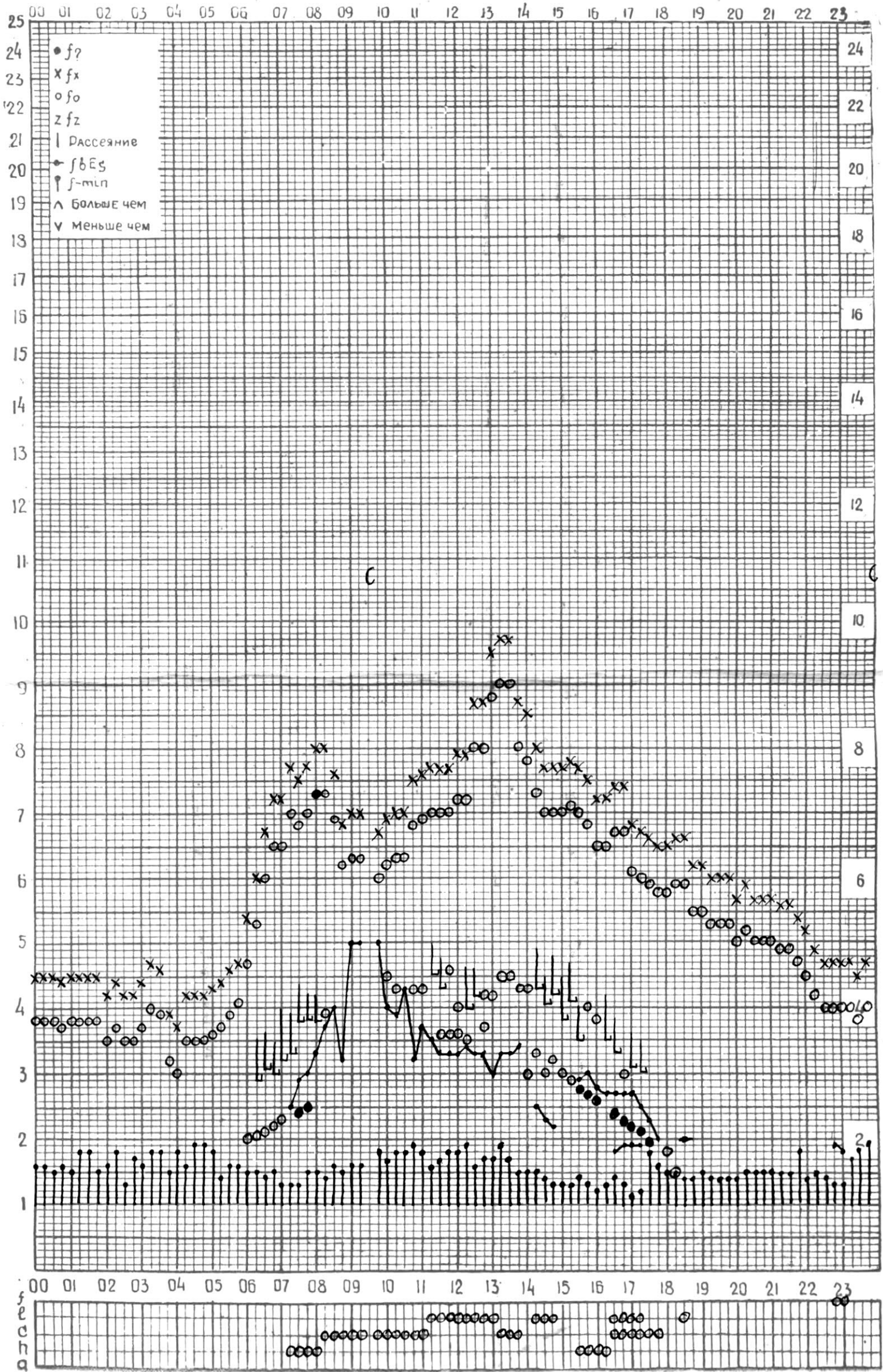
СТАНЦИЯ ТБИЛИСИ F-ГРАФИК ИОНОСФЕРНЫХ ДАННЫХ, ДАТА 2 СЕНТЯБРЯ, 1974
