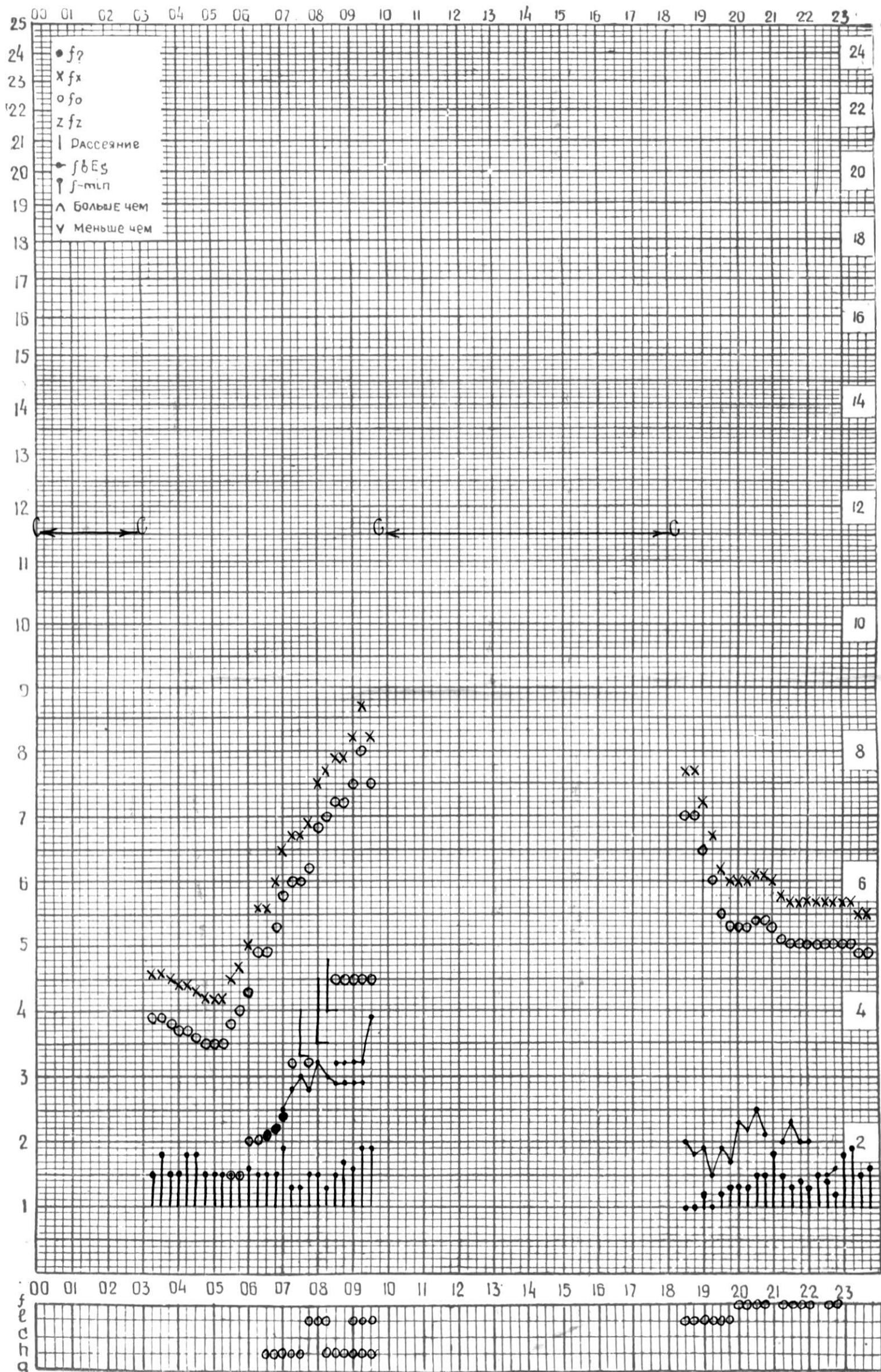
СТАНЦИЯ ТБИЛИСИ F-ГРАФИК ИОНОСФЕРНЫХ ДАННЫХ, ДАТА 10 СЕНТЯБРЯ, 1974
