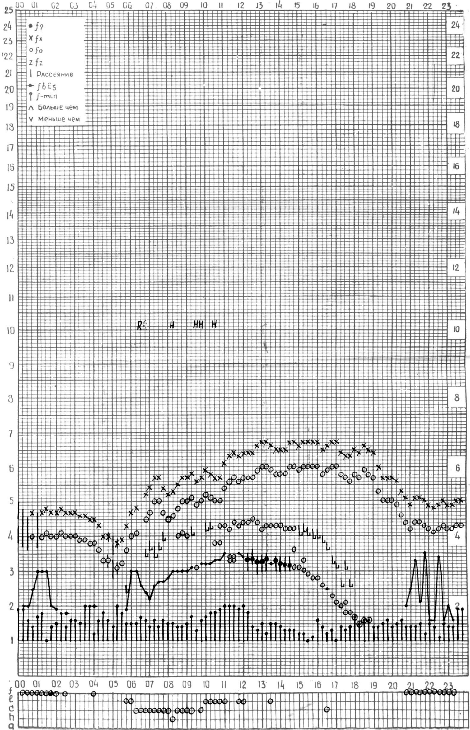
СТАНЦИЯ ТБИЛИСИ F-ГРАФИК ИОНОСФЕРНЫХ ДАННЫХ, ДАТА 7 СЕНТЯБРЯ, 1974
