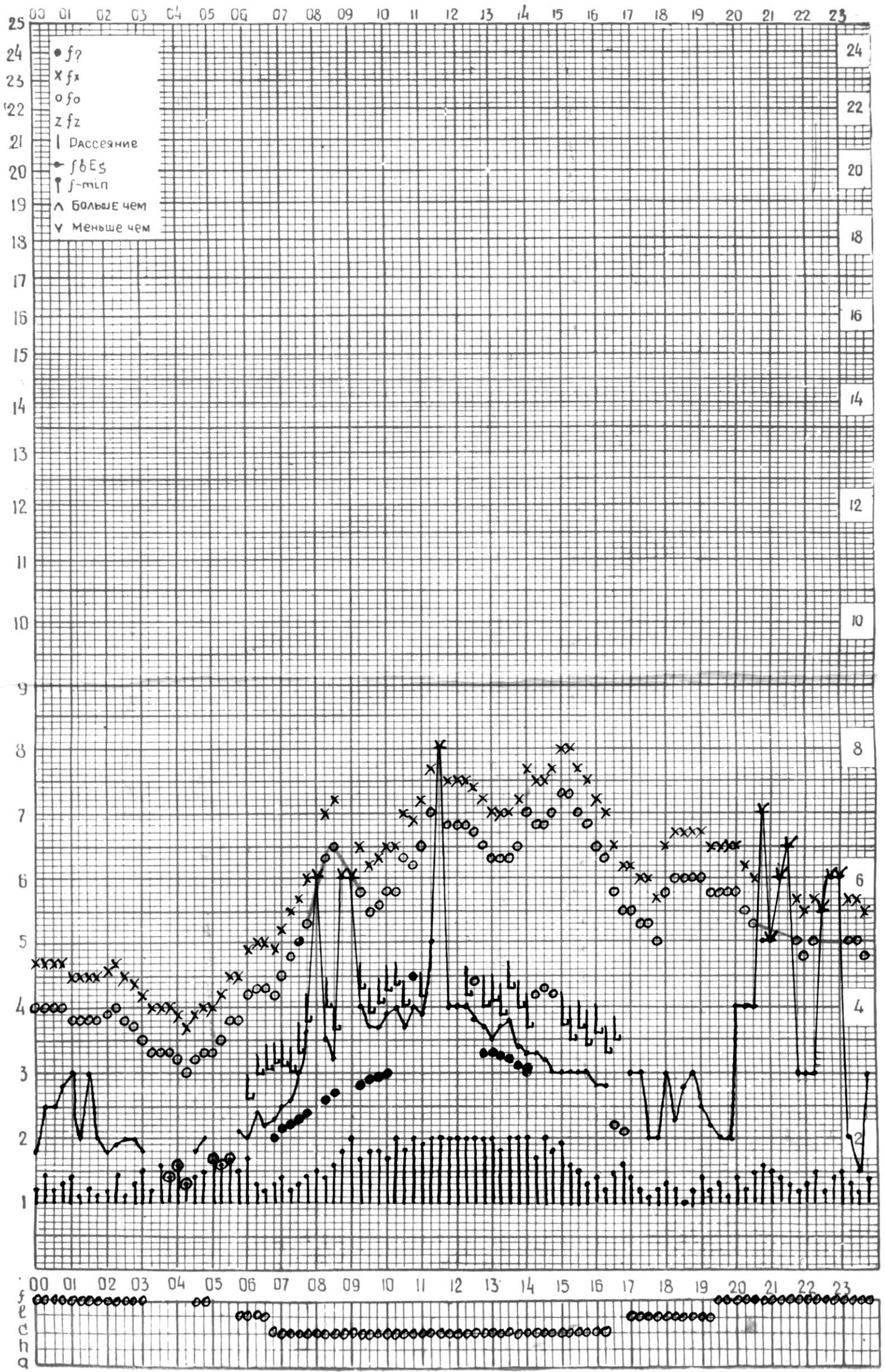
СТАНЦИЯ ТБИЛИСИ F-ГРАФИК ИОНОСФЕРНЫХ ДАННЫХ, ДАТА 3 СЕНТЯБРЯ, 1974
