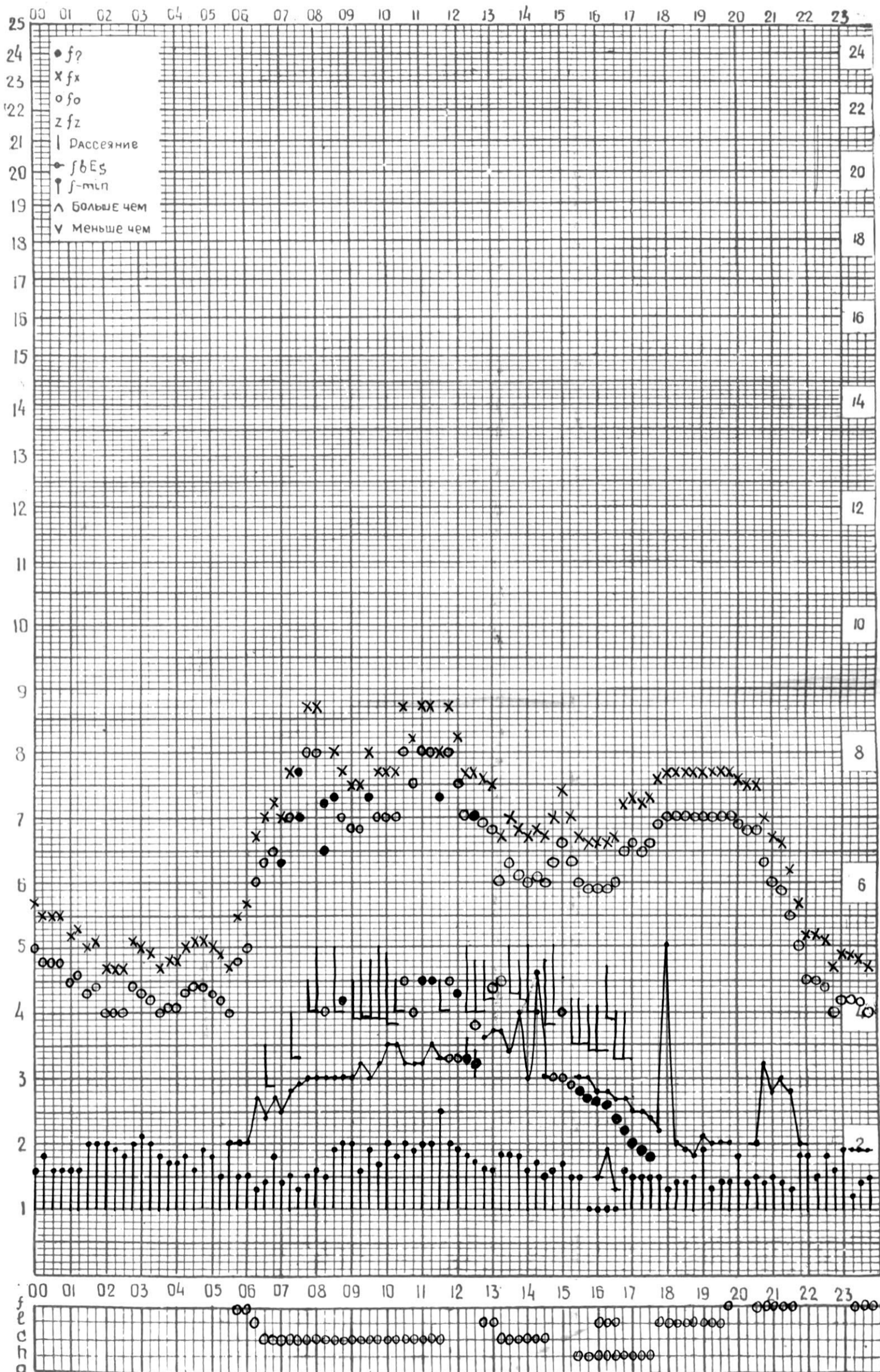
СТАНЦИЯ ТБИЛИСИ F-ГРАФИК ИОНОСФЕРНЫХ ДАННЫХ, ДАТА 14 СЕНТЯБРЯ, 1974
