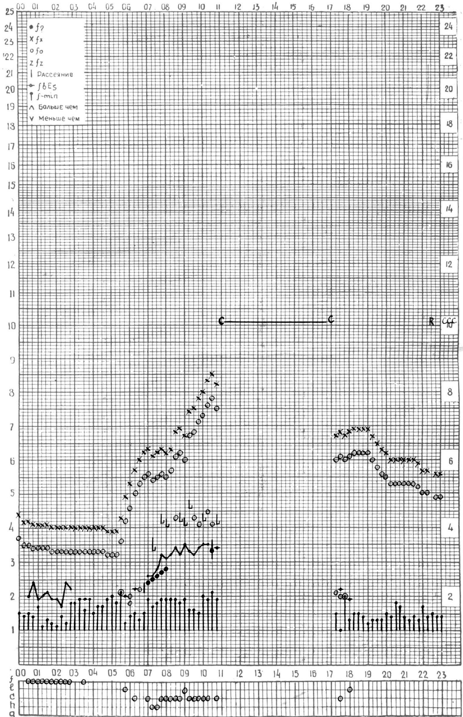
СТАНЦИЯ ТБИЛИСИ F-ГРАФИК ИОНОСФЕРНЫХ ДАННЫХ, ДАТА 12 СЕНТЯБРЯ, 1974
