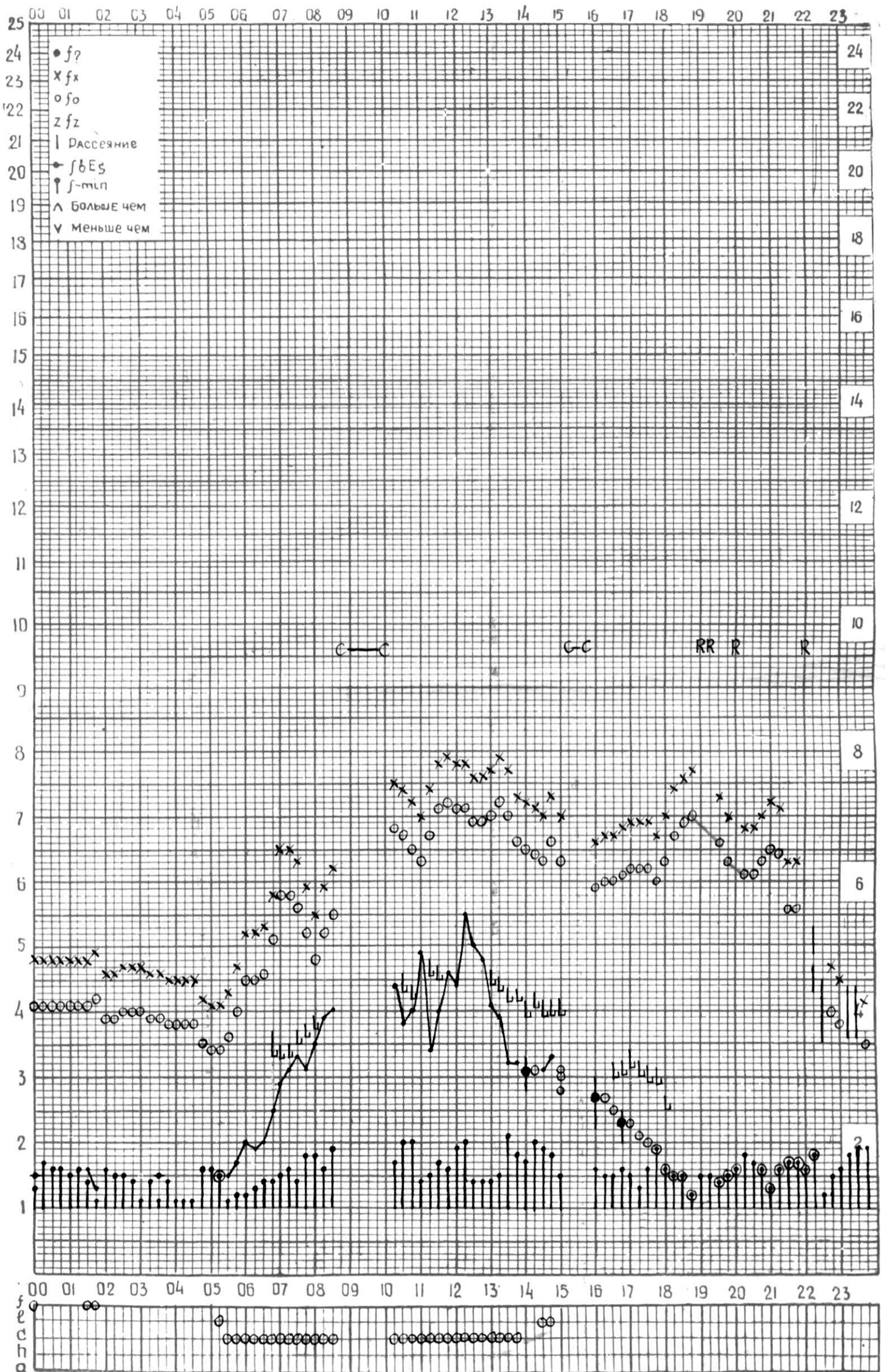
СТАНЦИЯ ТБИЛИСИ F-ГРАФИК ИОНОСФЕРНЫХ ДАННЫХ, ДАТА 15 СЕНТЯБРЯ, 1974
