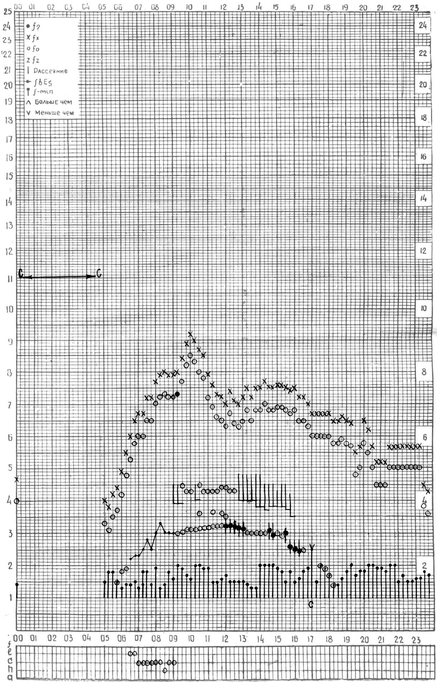
СТАНЦИЯ ТБИЛИСИ F-ГРАФИК ИОНОСФЕРНЫХ ДАННЫХ, ДАТА 18 СЕНТЯБРЯ, 1974
