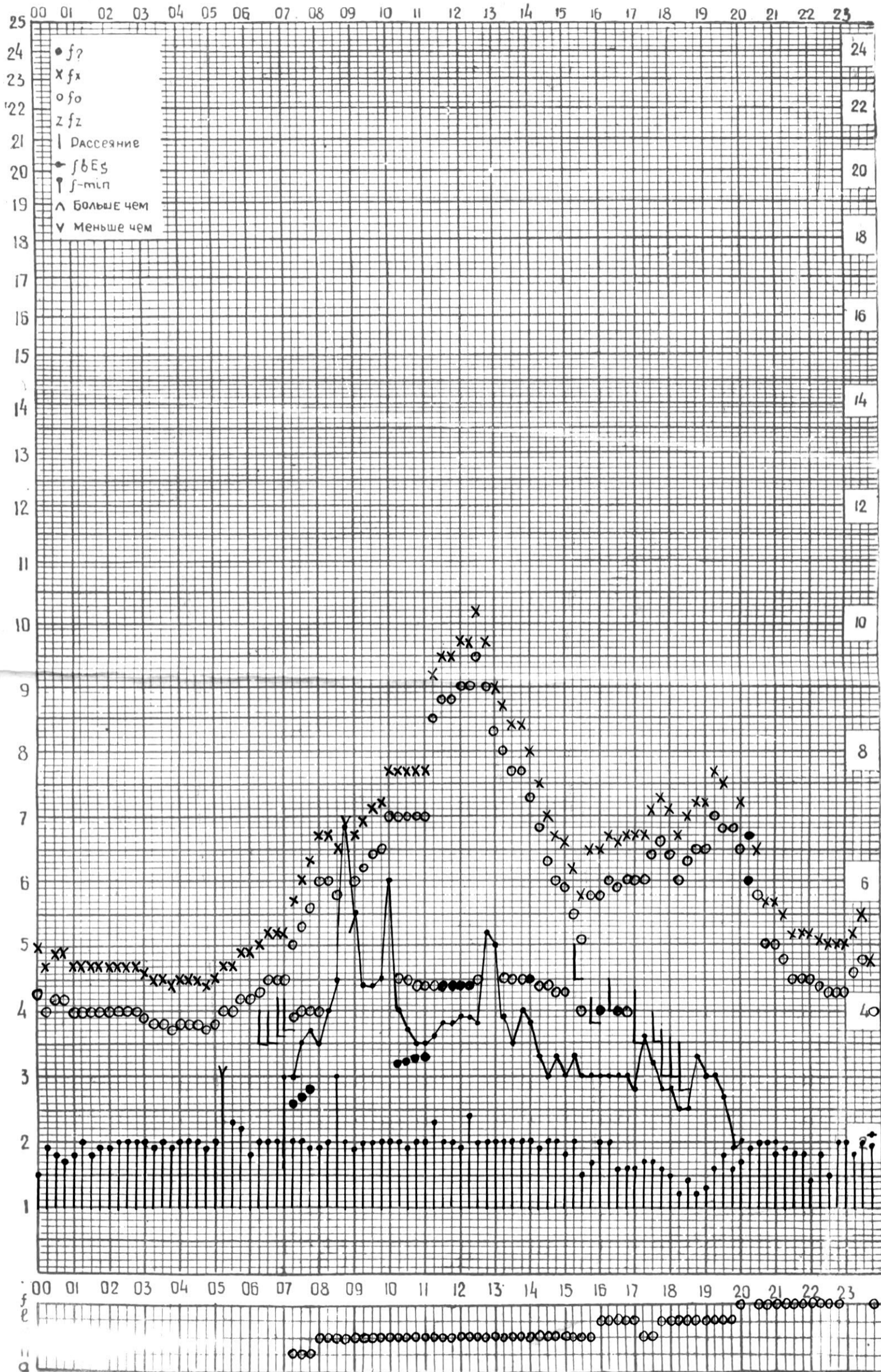
СТАНЦИЯ ТБИЛИСИ F—ГРАФИК ИОНОСФЕРНЫХ ДАННЫХ, ДАТА 9 АВГУСТА, 1974
