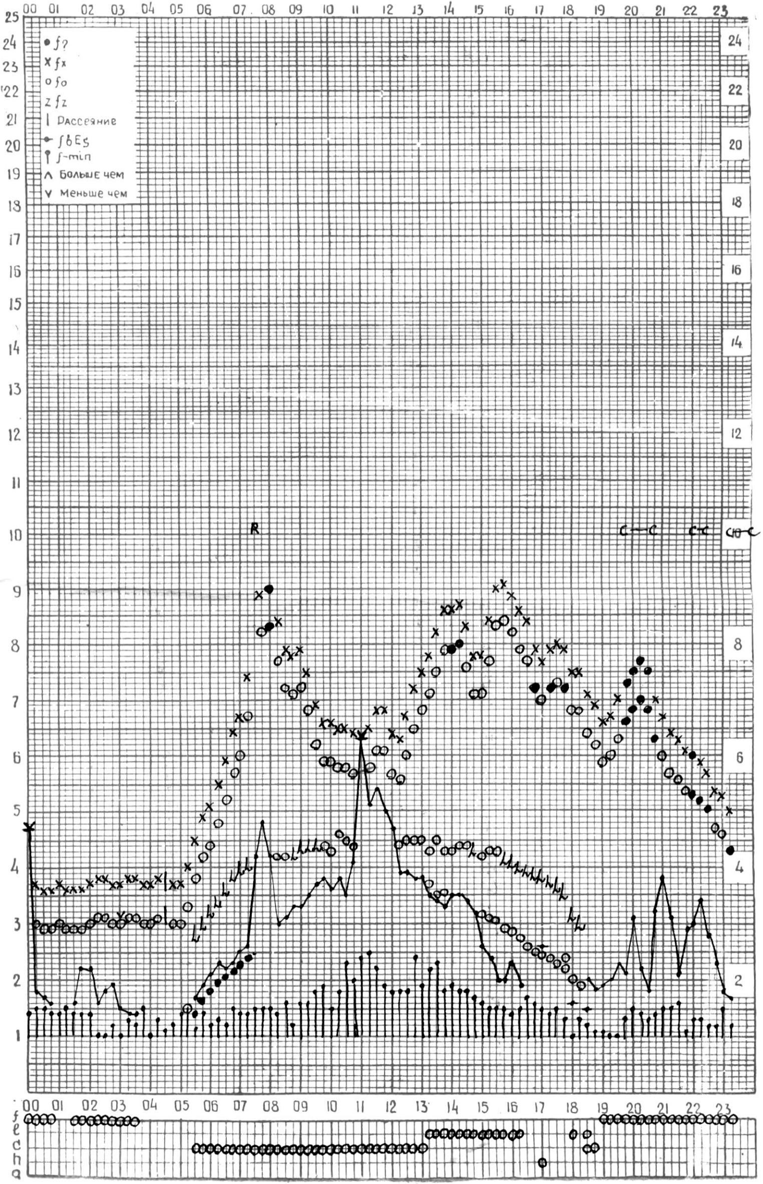
СТАНЦИЯ ТБИЛИСИ F-ГРАФИК ИОНОСФЕРНЫХ ДАННЫХ, ДАТА 19 АВГУСТА, 1974
