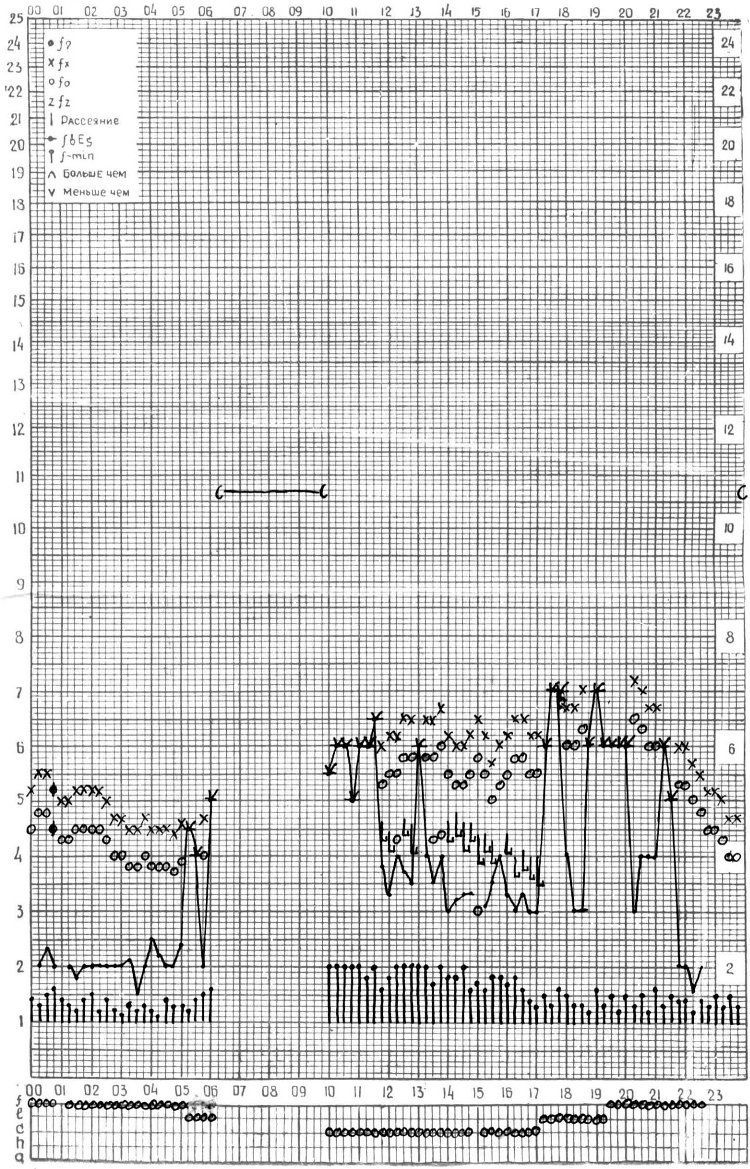
СТАНЦИЯ ТБИЛИСИ F-ГРАФИК ИОНОСФЕРНЫХ ДАННЫХ, ДАТА 10 АВГУСТА, 1974
