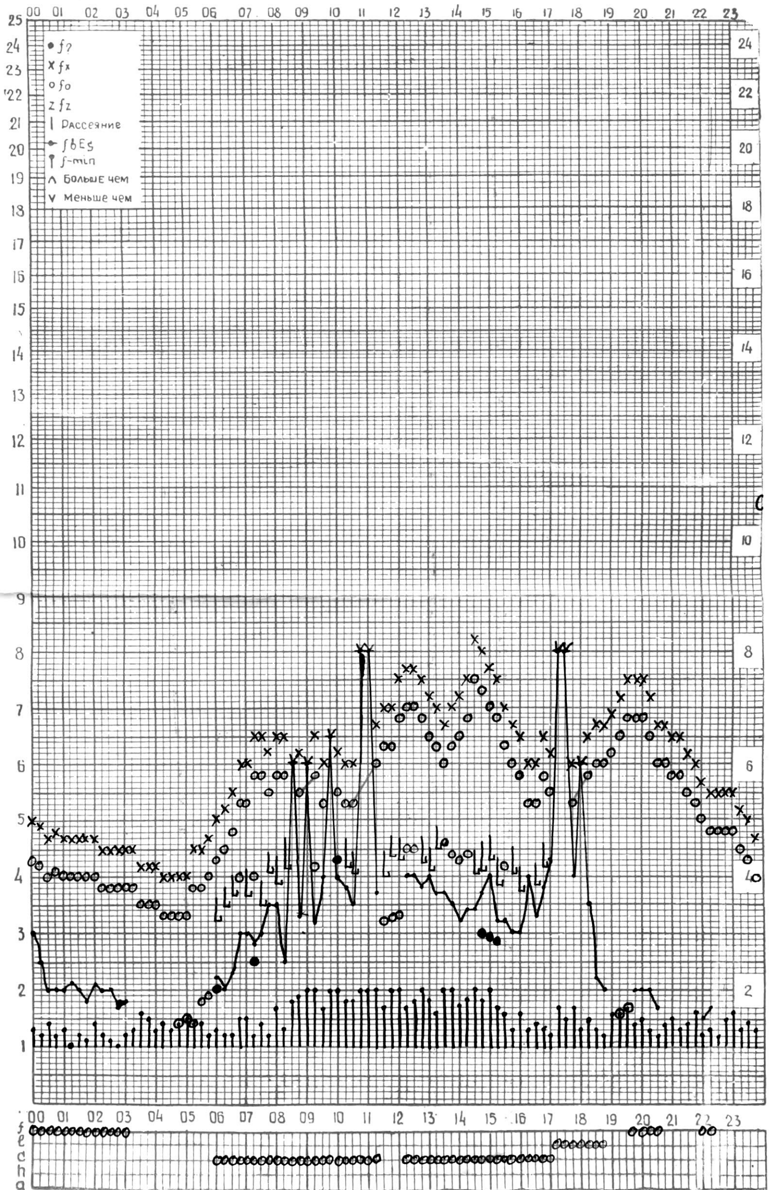
СТАНЦИЯ ТБИЛИСИ F-ГРАФИК ИОНОСФЕРНЫХ ДАННЫХ, ДАТА 6 АВГУСТА, 1974
