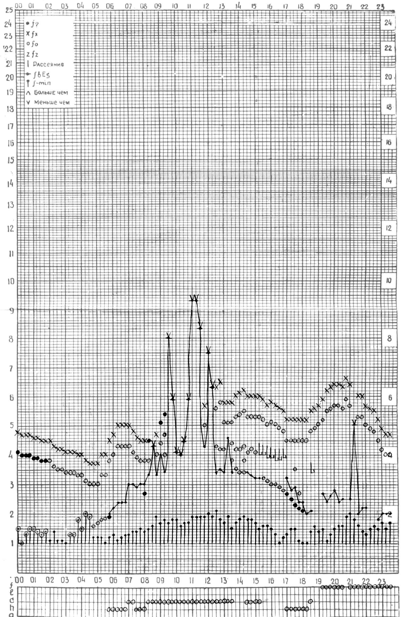
СТАНЦИЯ ТБИЛИСИ F-ГРАФИК ИОНОСФЕРНЫХ ДАННЫХ, ДАТА 4 АВГУСТА, 1974
