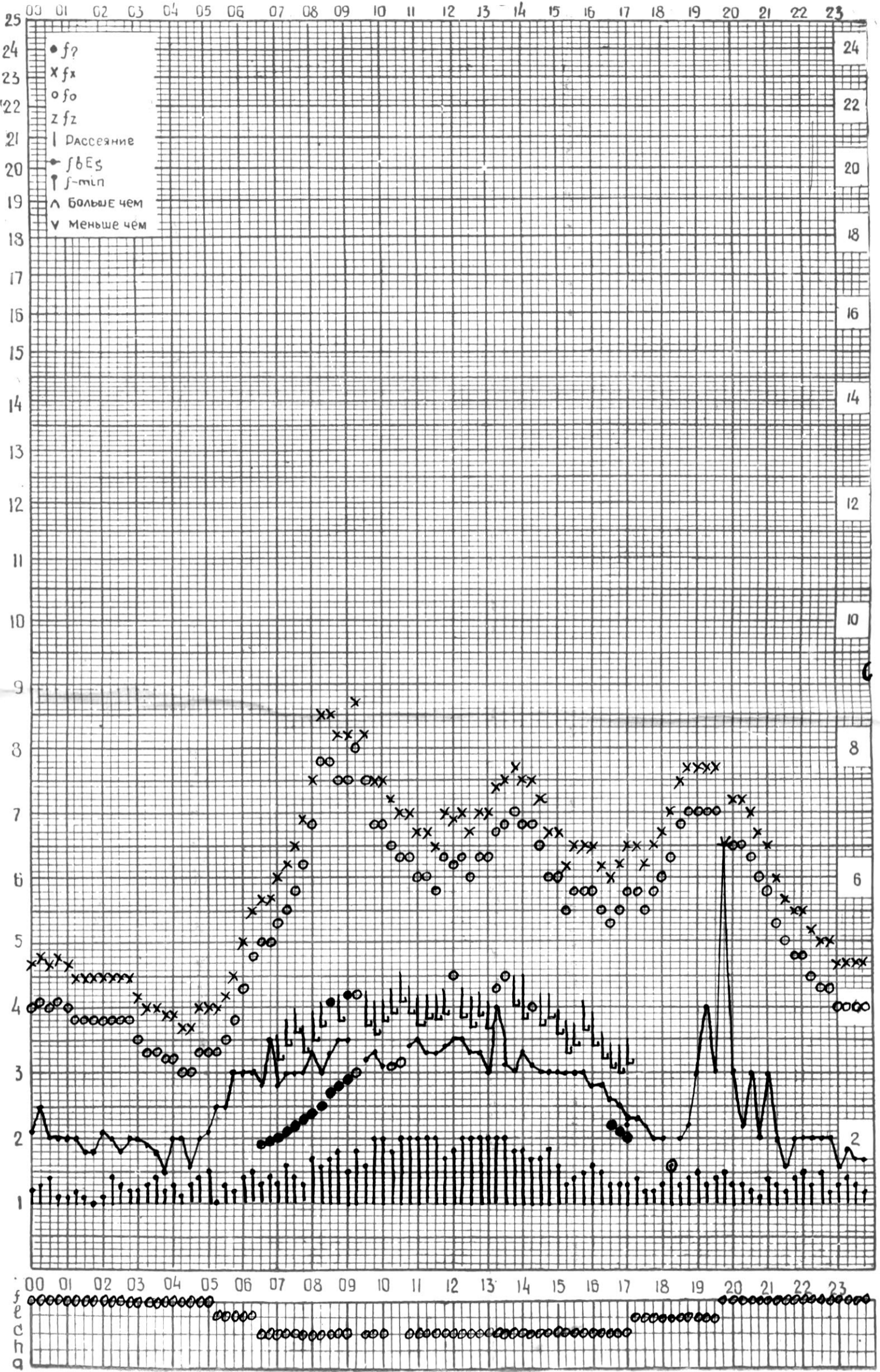
СТАНЦИЯ ТБИЛИСИ F-ГРАФИК ИОНОСФЕРНЫХ ДАННЫХ, ДАТА 30 АВГУСТА, 1974
