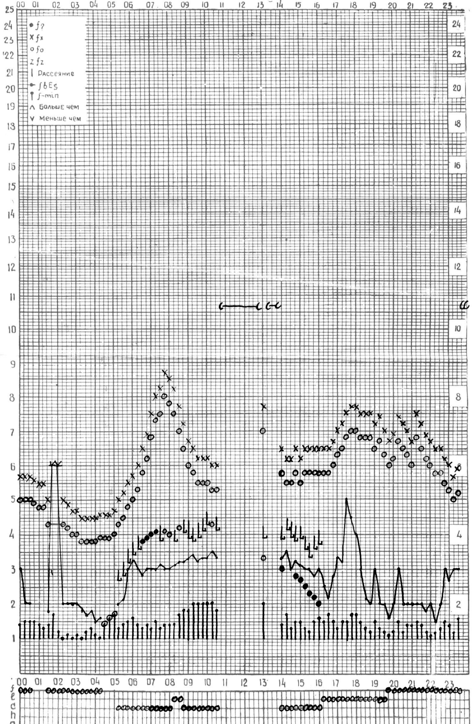
СТАНЦИЯ ТБИЛИСИ F-ГРАФИК ИОНОСФЕРНЫХ ДАННЫХ, ДАТА 2 АВГУСТА, 1974
