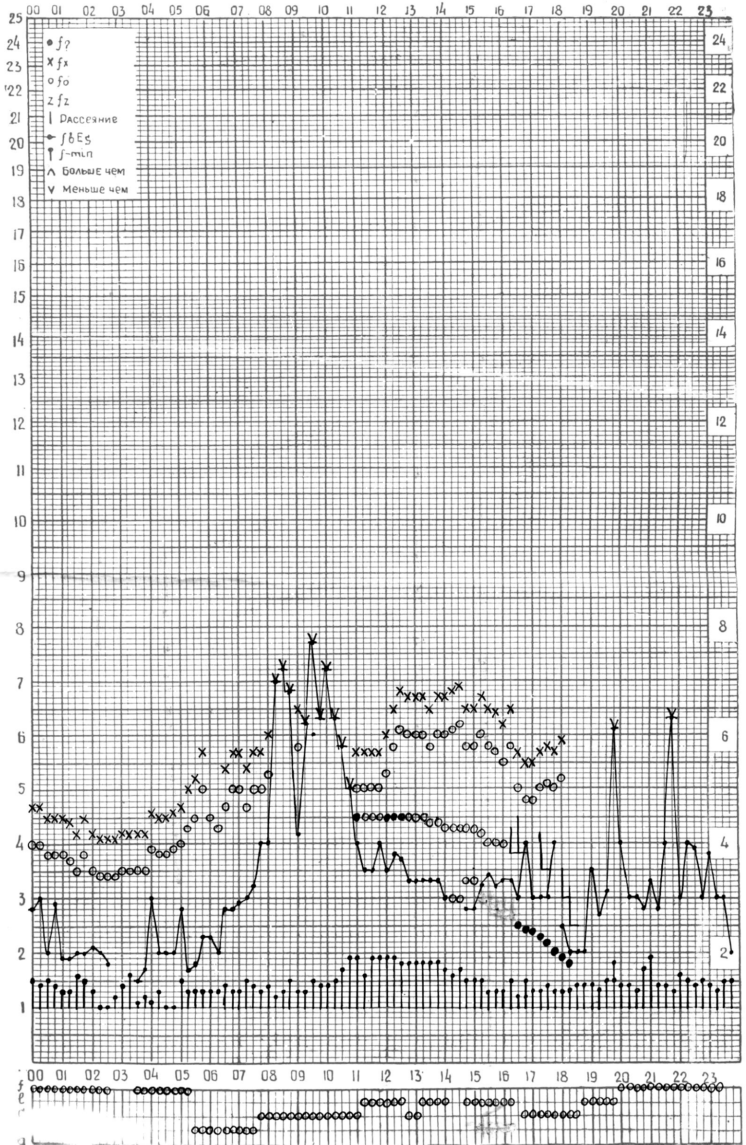
СТАНЦИЯ ТБИЛИСИ F-ГРАФИК ИОНОСФЕРНЫХ ДАННЫХ, ДАТА 21 АВГУСТА, 1974
