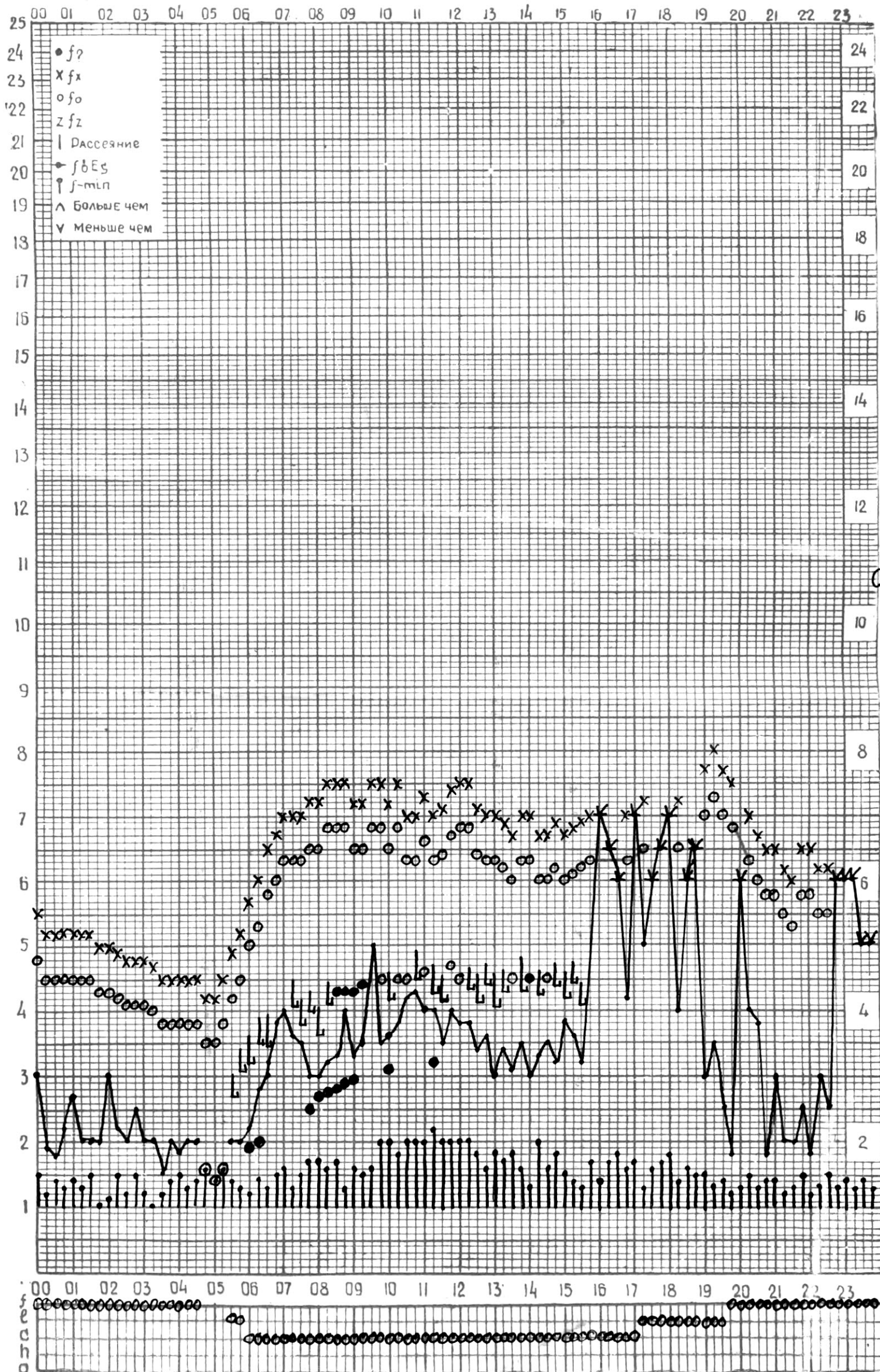
СТАНЦИЯ ТБИЛИСИ F-ГРАФИК ИОНОСФЕРНЫХ ДАННЫХ, ДАТА 14 АВГУСТА, 1974
