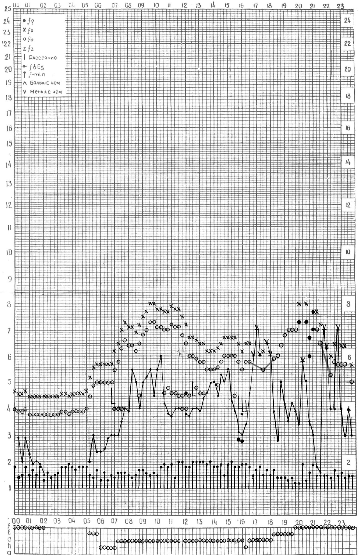
СТАНЦИЯ ТБИЛИСИ F-ГРАФИК ИОНОСФЕРНЫХ ДАННЫХ, ДАТА 17 АВГУСТА, 1974
