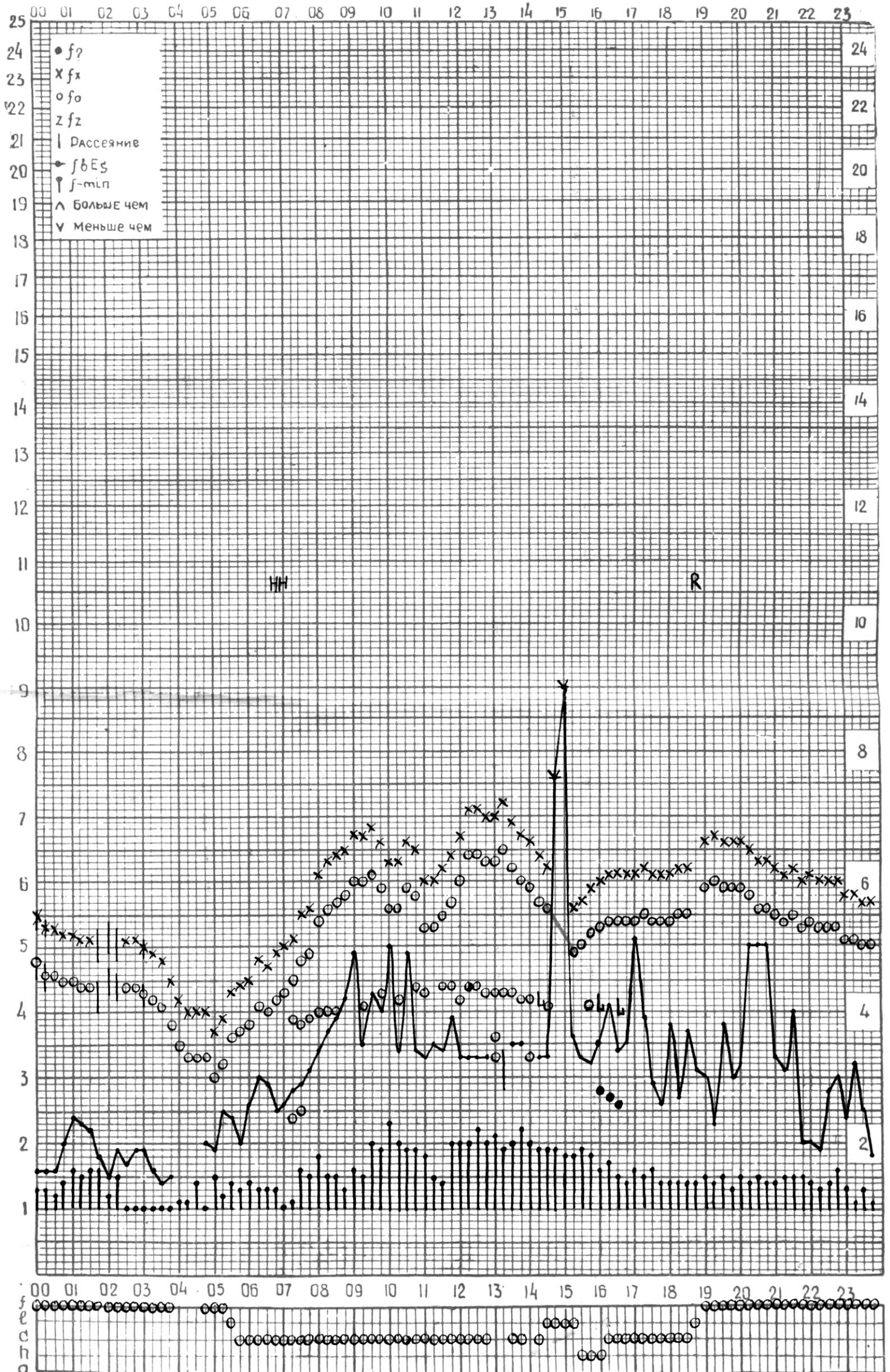
СТАНЦИЯ ТБИЛИСИ F—ГРАФИК ИОНОСФЕРНЫХ ДАННЫХ, ДАТА 23 АВГУСТА 1974
