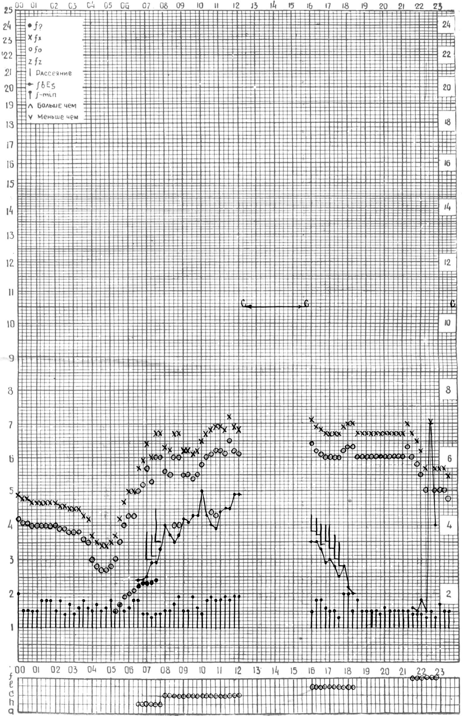
СТАНЦИЯ ТБИЛИСИ F-ГРАФИК ИОНОСФЕРНЫХ ДАННЫХ, ДАТА 25 АВГУСТА, 1974
