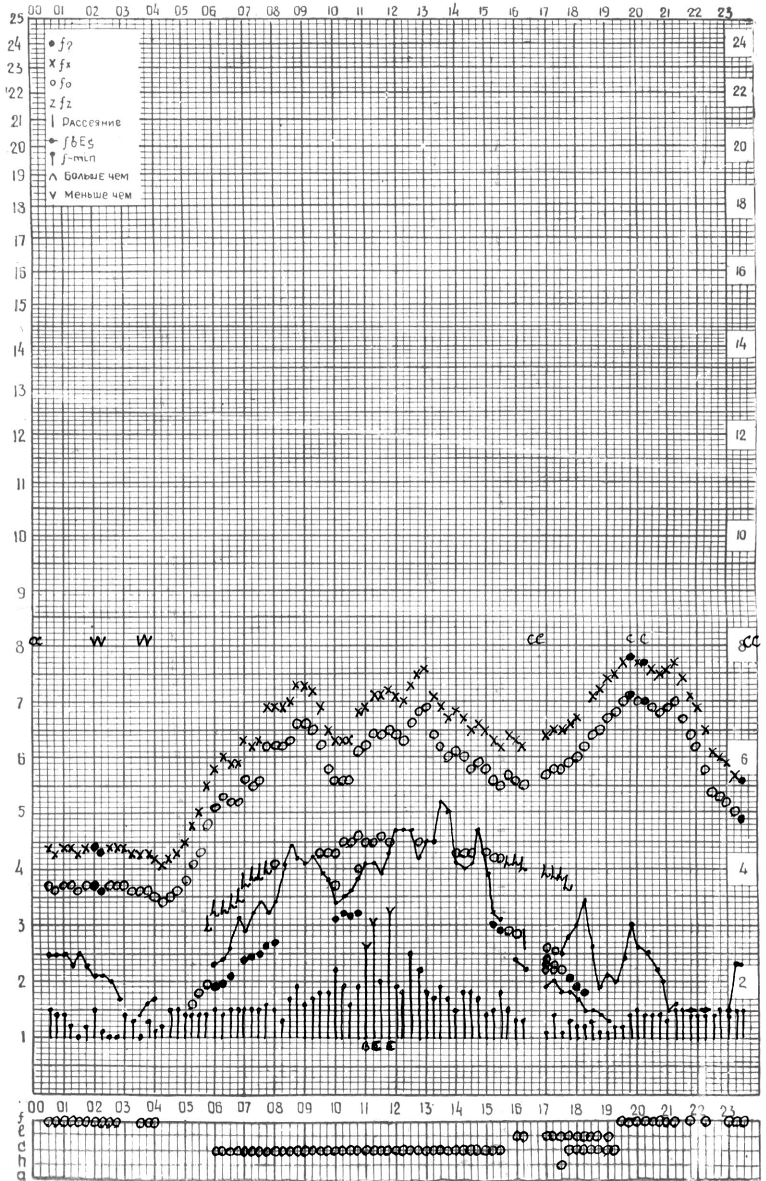
СТАНЦИЯ ТБИЛИСИ F-ГРАФИК ИОНОСФЕРНЫХ ДАННЫХ, ДАТА 15 АВГУСТА, 1974
