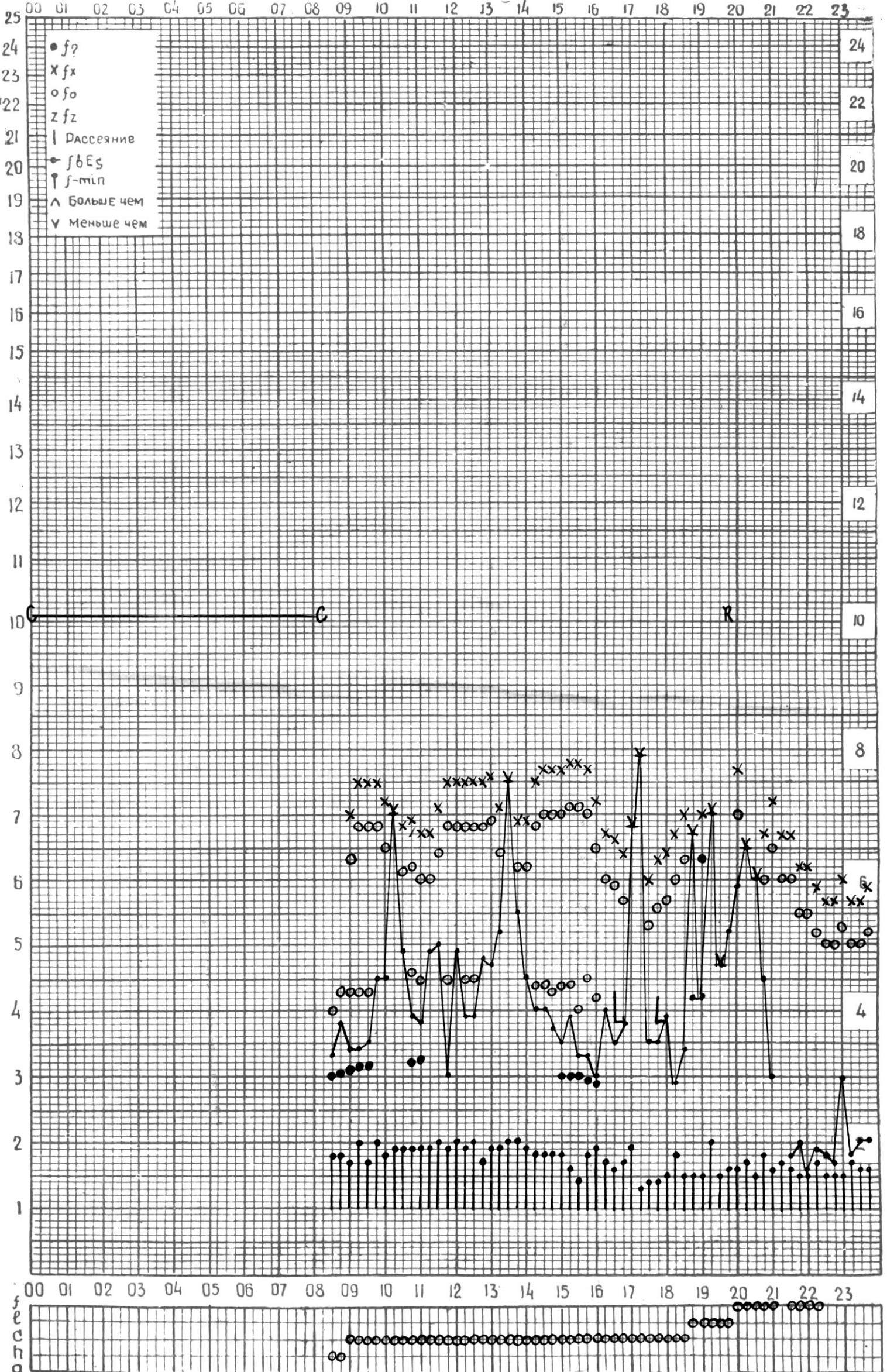
СТАНЦИЯ ТБИЛИСИ F-ГРАФИК ИОНОСФЕРНЫХ ДАННЫХ, ДАТА 24 ИЮЛЯ, 1974
