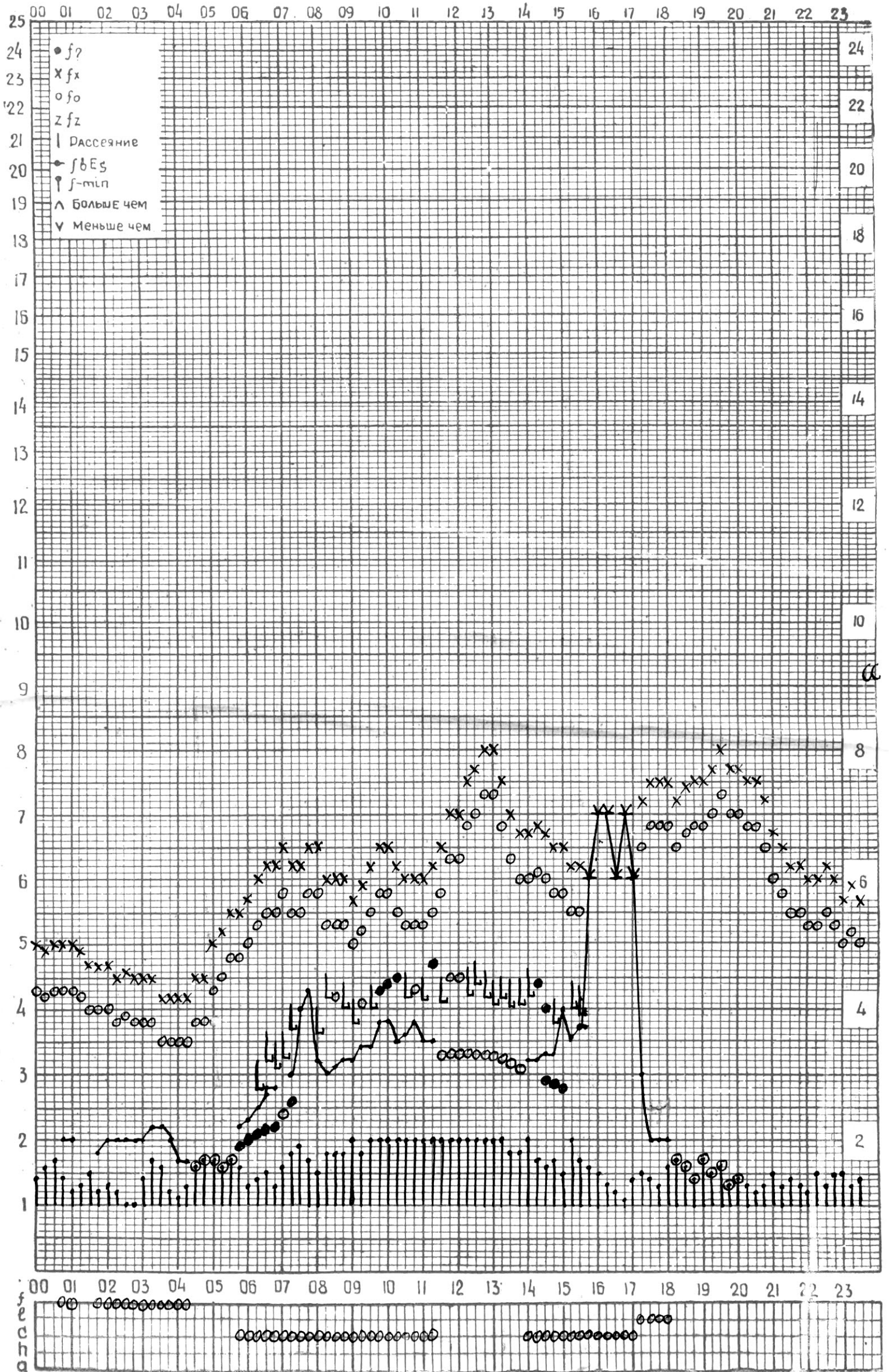
СТАНЦИЯ ТБИЛИСИ F-ГРАФИК ИОНОСФЕРНЫХ ДАННЫХ, ДАТА 29 ИЮЛЯ, 1974
