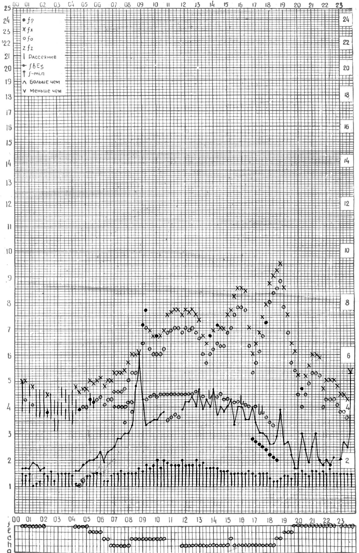
СТАНЦИЯ ТБИЛИСИ F-ГРАФИК ИОНОСФЕРНЫХ ДАННЫХ, ДАТА 23 ИЮЛЯ, 1974
