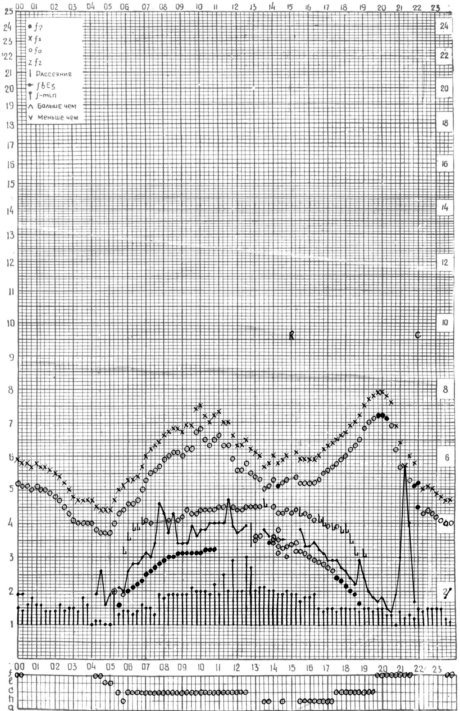
СТАНЦИЯ ТБИЛИСИ F—ГРАФИК ИОНОСФЕРНЫХ ДАННЫХ, ДАТА 26 ИЮЛЯ, 1974
