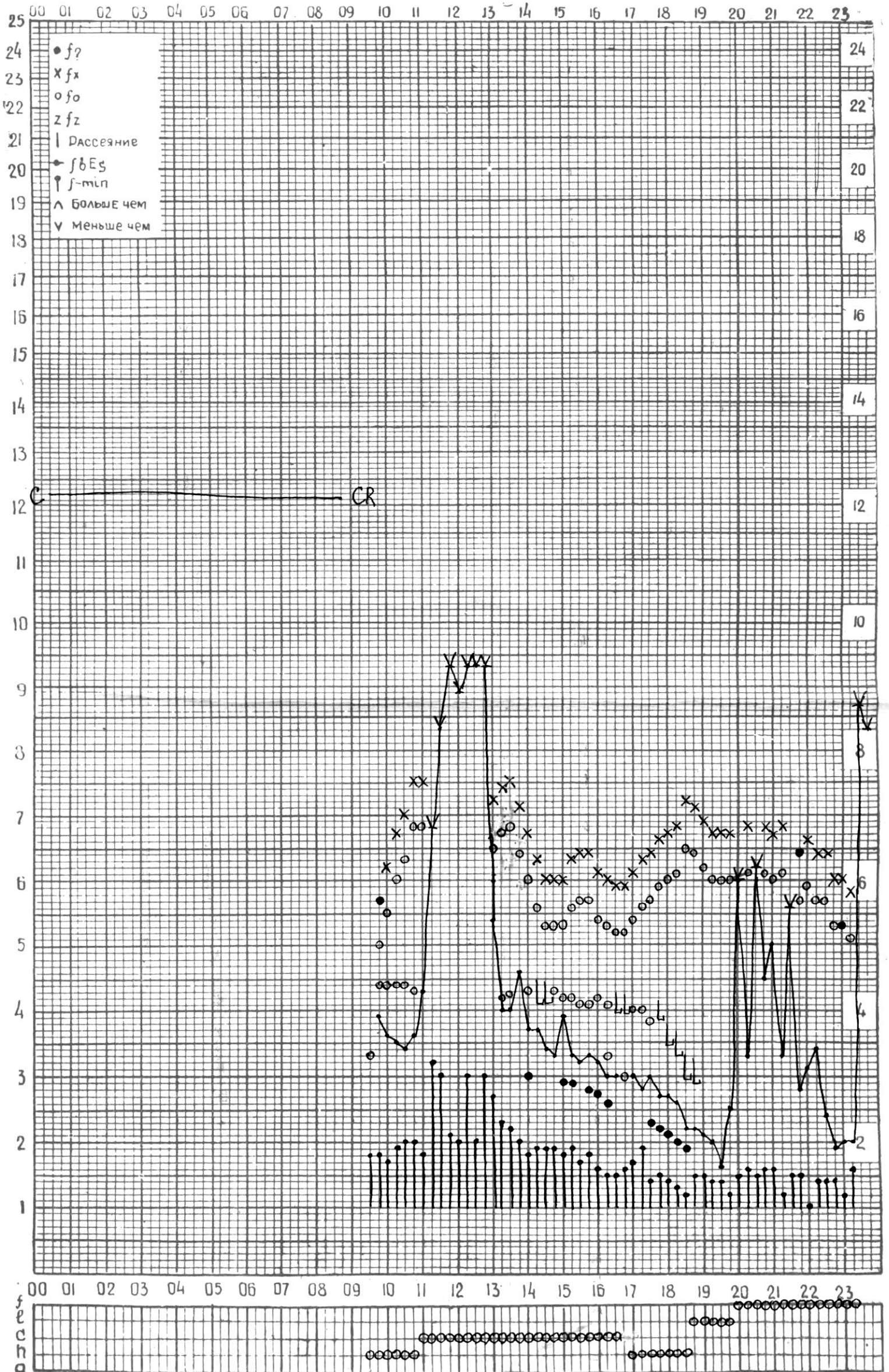
СТАНЦИЯ ТБИЛИСИ F—ГРАФИК ИОНОСФЕРНЫХ ДАННЫХ, ДАТА 11 ИЮЛЯ, 1974
