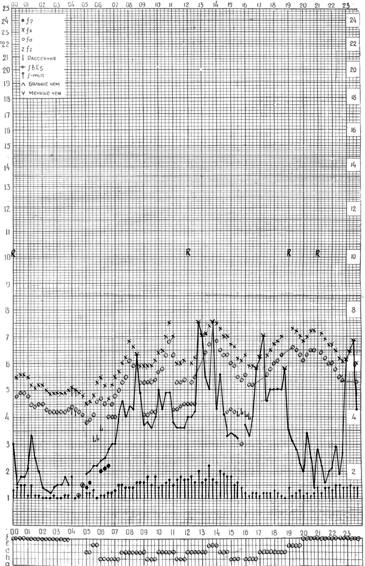
СТАНЦИЯ ТБИЛИСИ F-ГРАФИК ИОНОСФЕРНЫХ ДАННЫХ, ДАТА 14 ИЮЛЯ, 1974
