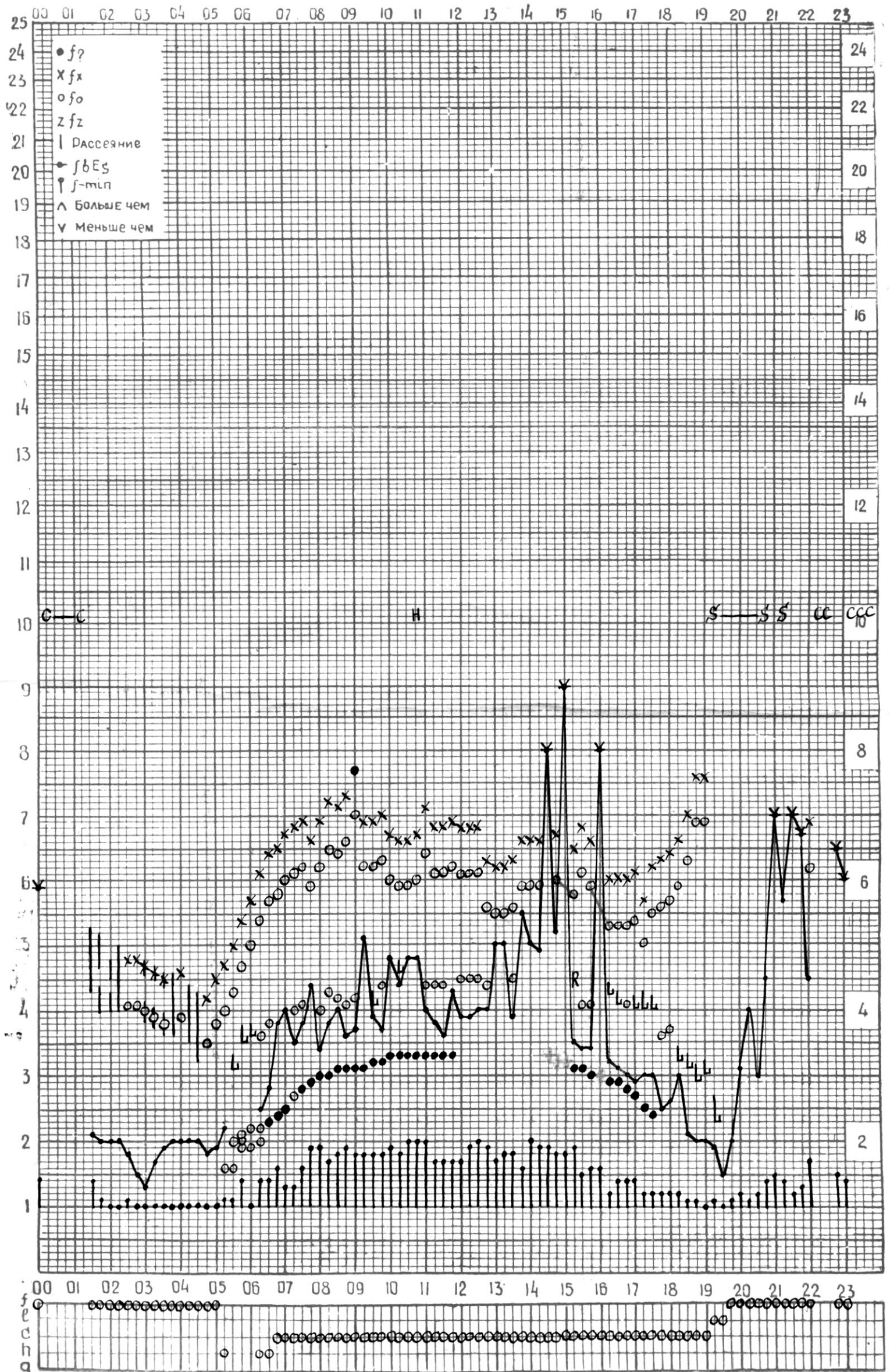
СТАНЦИЯ ТБИЛИСИ F—ГРАФИК ИОНОСФЕРНЫХ ДАННЫХ, ДАТА 18 ИЮЛЯ, 1974
