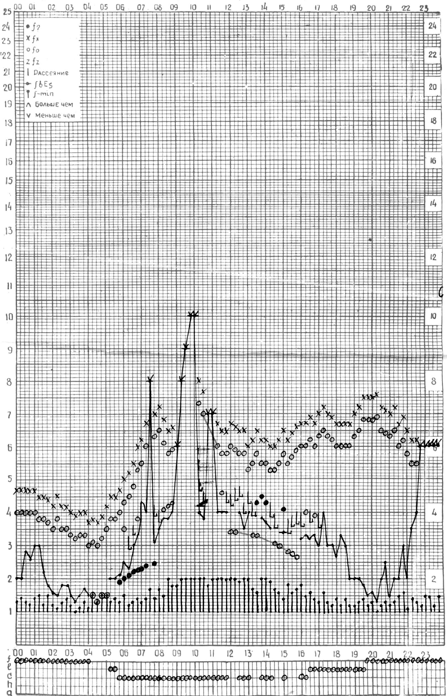
СТАНЦИЯ ТБИЛИСИ F-ГРАФИК ИОНОСФЕРНЫХ ДАННЫХ, ДАТА 17 ИЮЛЯ, 1974
