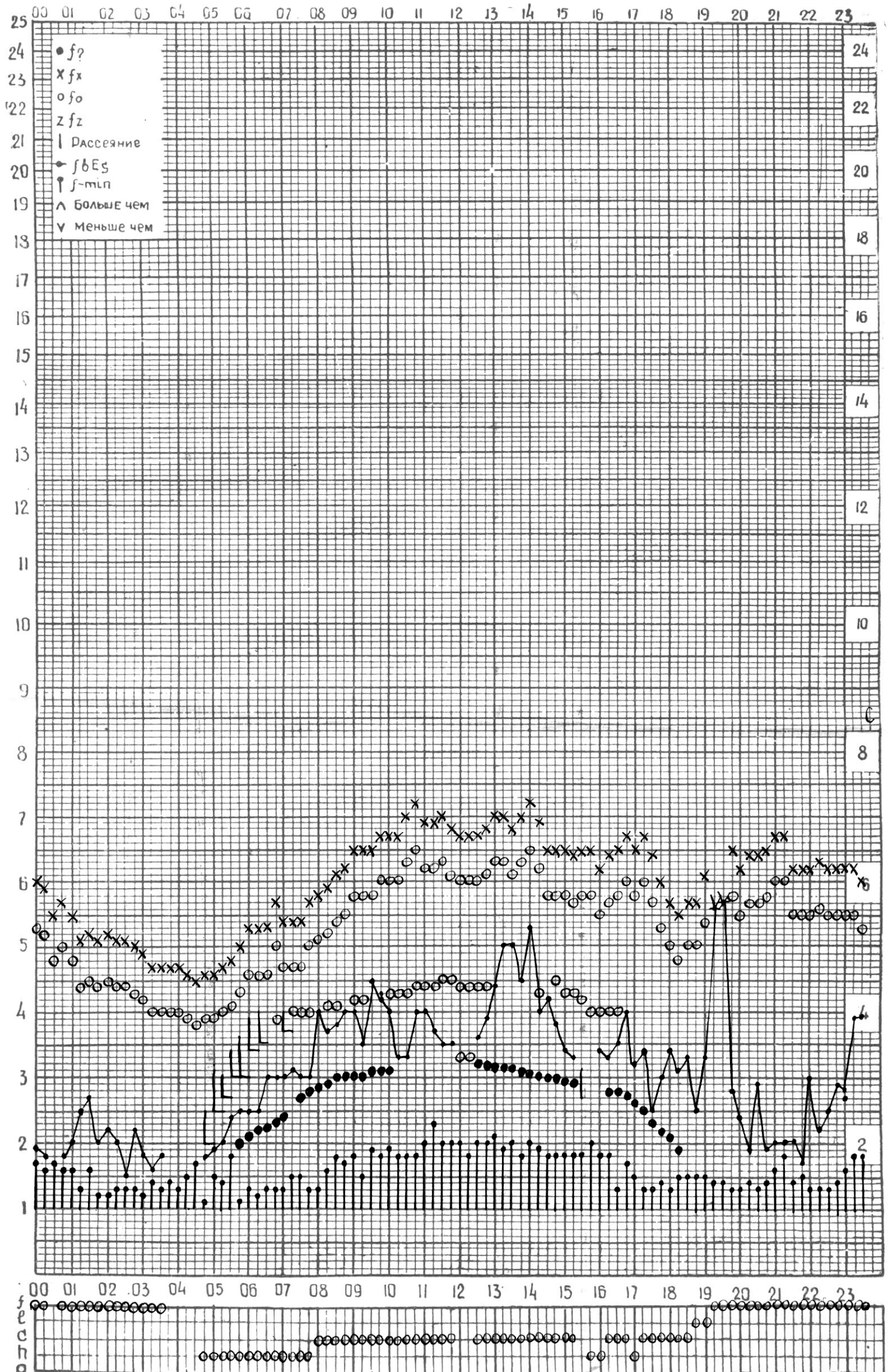
СТАНЦИЯ ТБИЛИСИ F-ГРАФИК ИОНОСФЕРНЫХ ДАННЫХ, ДАТА 20 ИЮЛЯ, 1974
