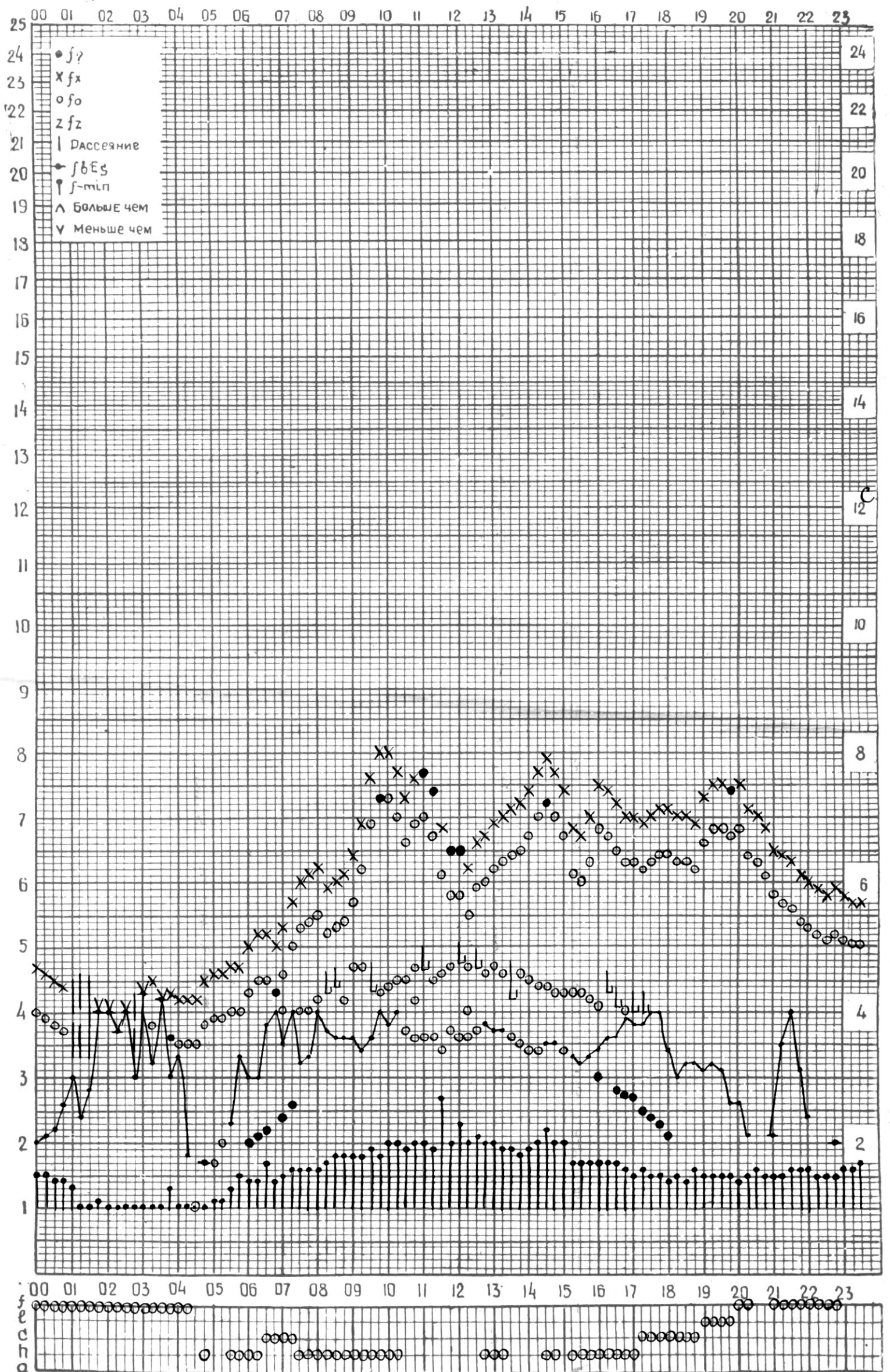
СТАНЦИЯ ТБИЛИСИ F-ГРАФИК ИОНОСФЕРНЫХ ДАННЫХ, ДАТА 27 ИЮЛЯ, 1974
