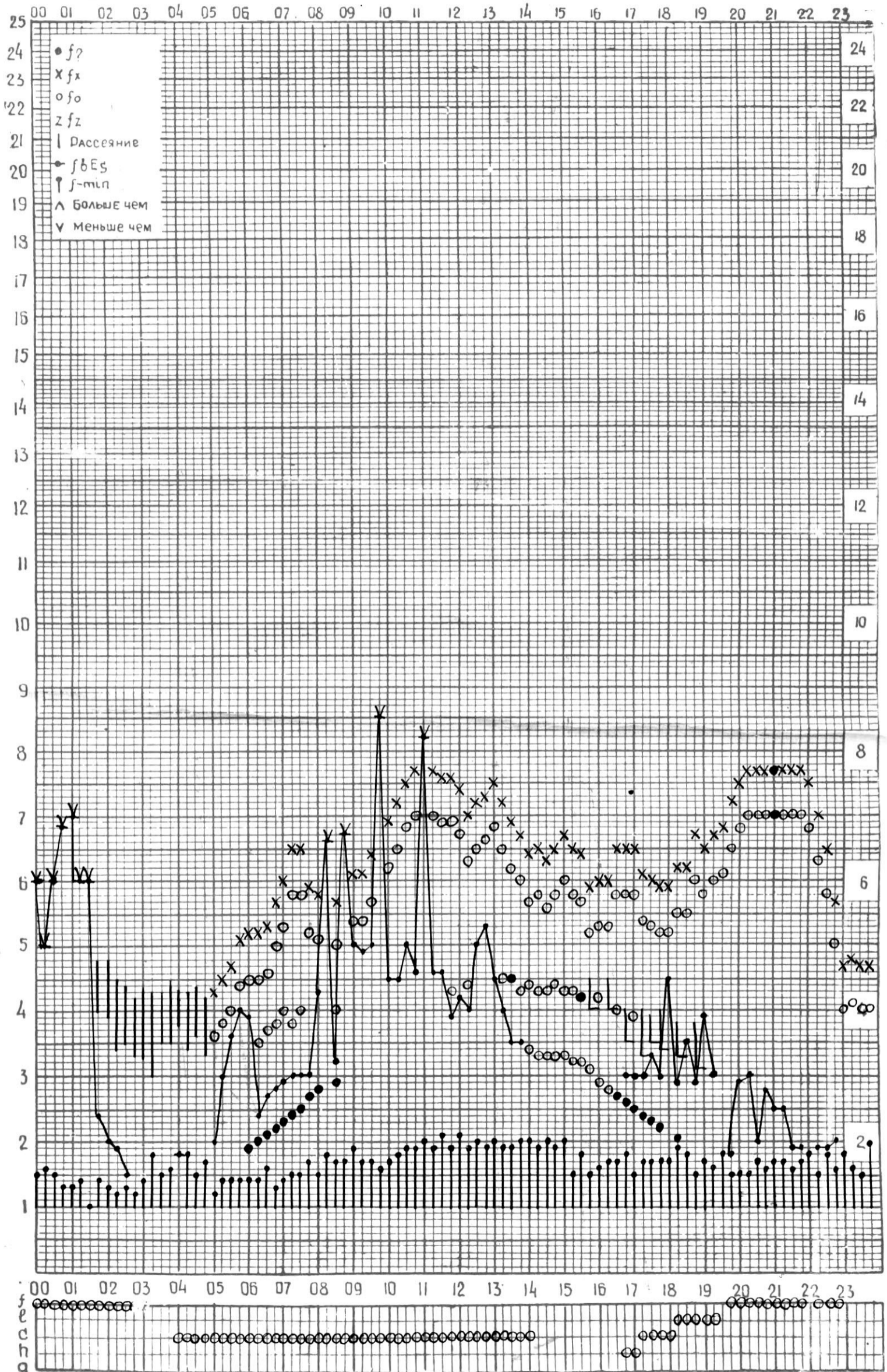
СТАНЦИЯ ТБИЛИСИ F—ГРАФИК ИОНОСФЕРНЫХ ДАННЫХ, ДАТА 16 ИЮЛЯ, 1974
