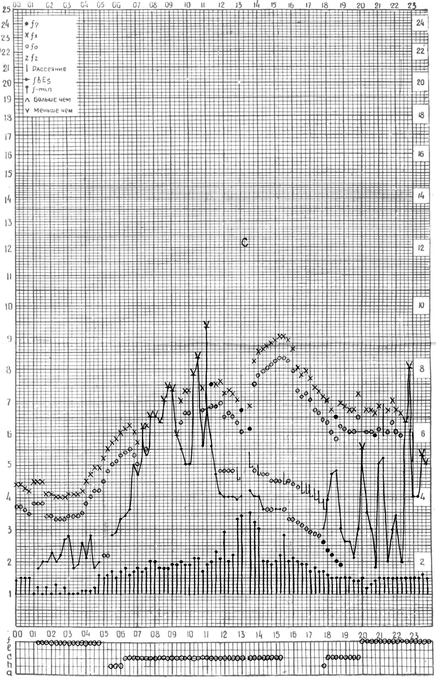
СТАНЦИЯ ТБИЛИСИ F-ГРАФИК ИОНОСФЕРНЫХ ДАННЫХ, ДАТА 7 ИЮЛЯ, 1974
