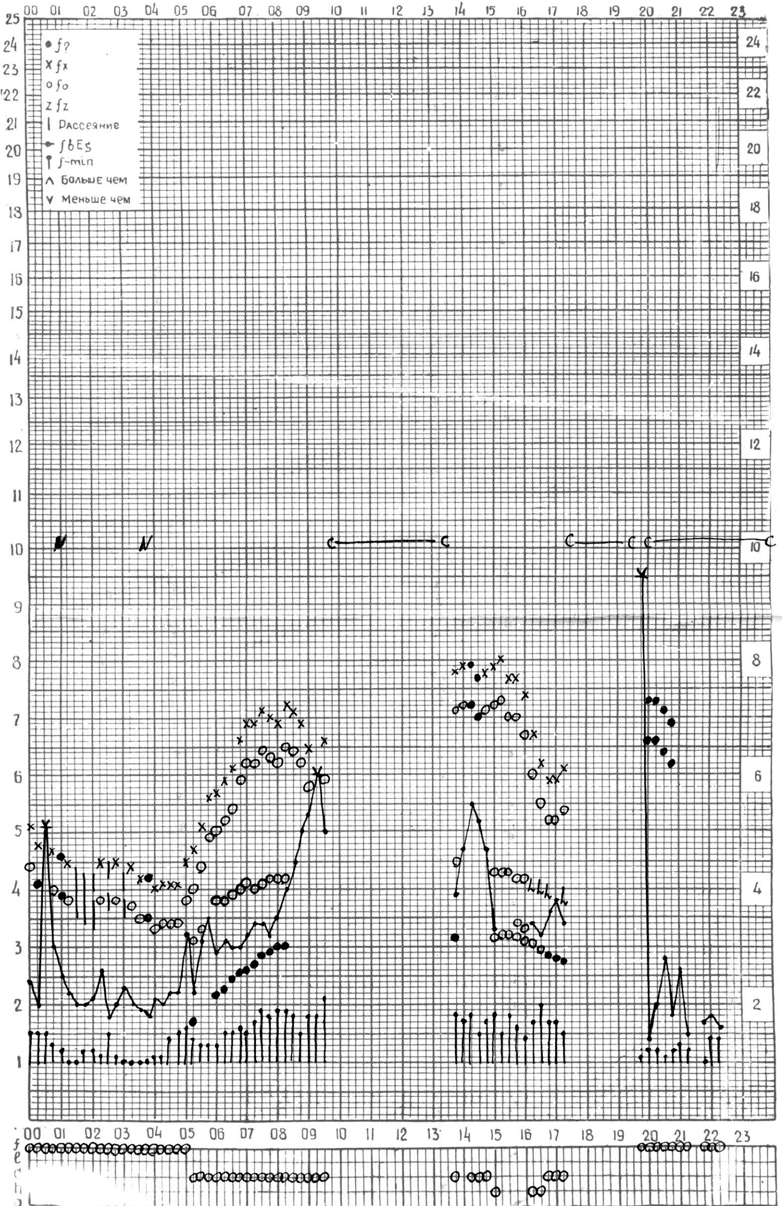
СТАНЦИЯ ТБИЛИСИ F-ГРАФИК ИОНОСФЕРНЫХ ДАННЫХ, ДАТА 2 ИЮЛЯ, 1974
