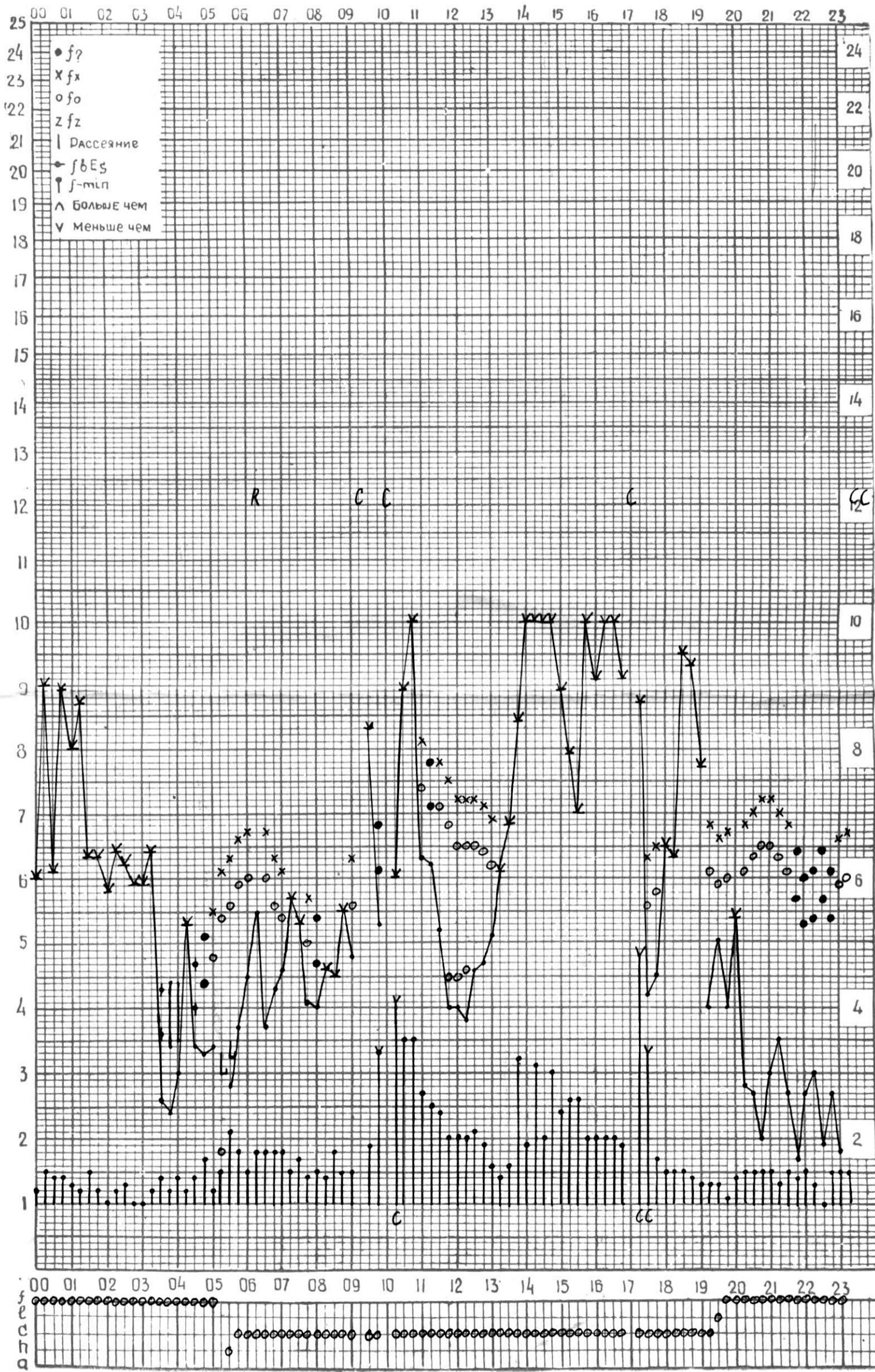
СТАНЦИЯ ТБИЛИСИ F-ГРАФИК ИОНОСФЕРНЫХ ДАННЫХ, ДАТА 4 ИЮЛЯ, 1974
