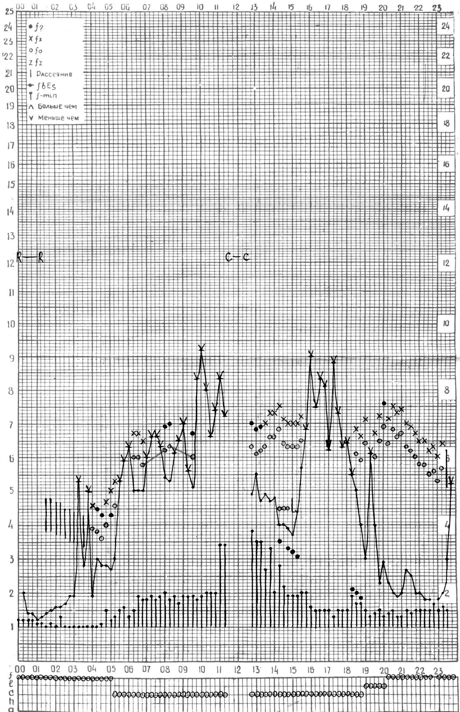
СТАНЦИЯ ТБИЛИСИ F-ГРАФИК ИОНОСФЕРНЫХ ДАННЫХ, ДАТА 3 ИЮЛЯ, 1974
