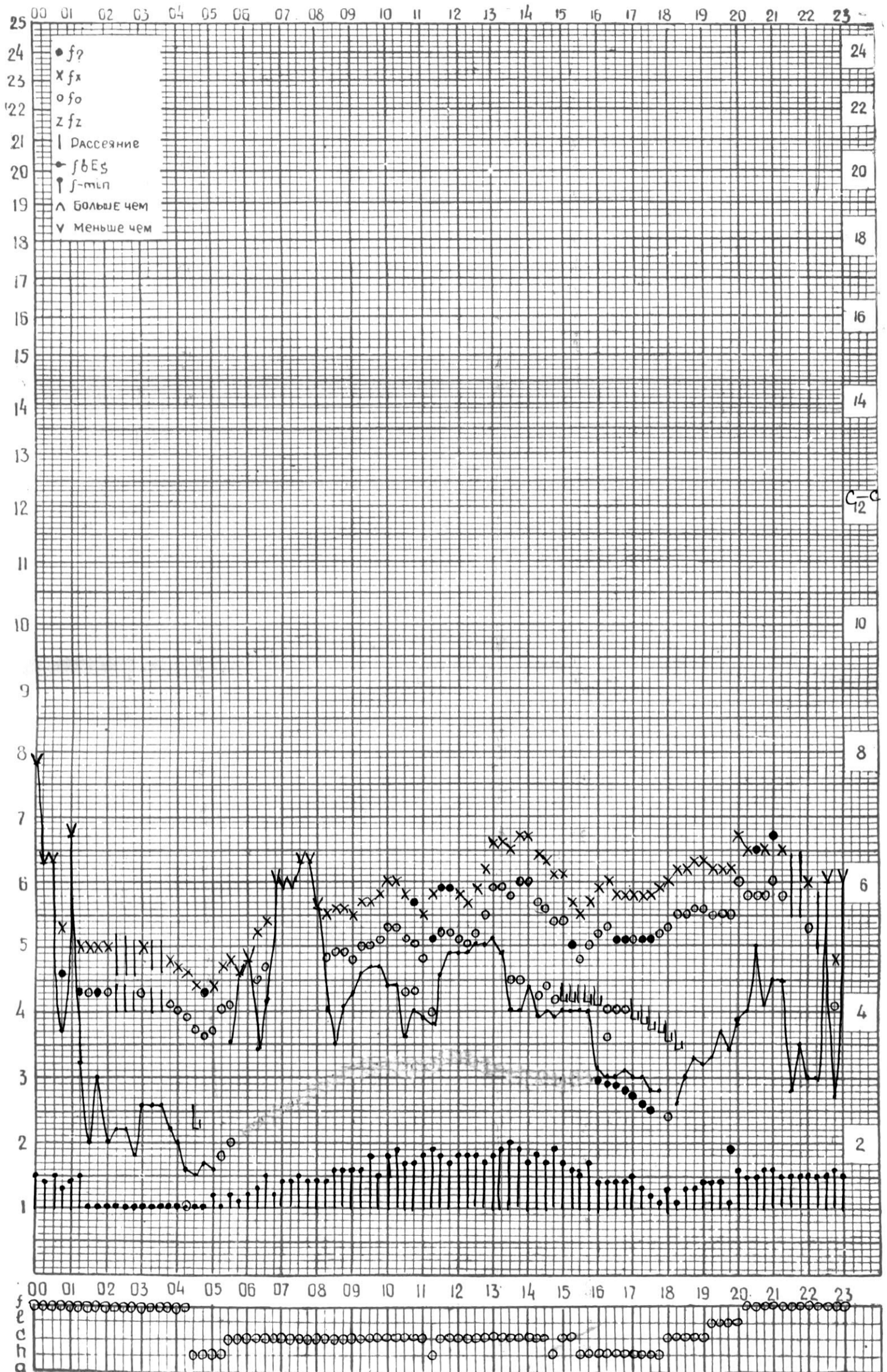
СТАНЦИЯ ТБИЛИСИ F-ГРАФИК ИОНОСФЕРНЫХ ДАННЫХ, ДАТА 21 ИЮНЯ, 1974
