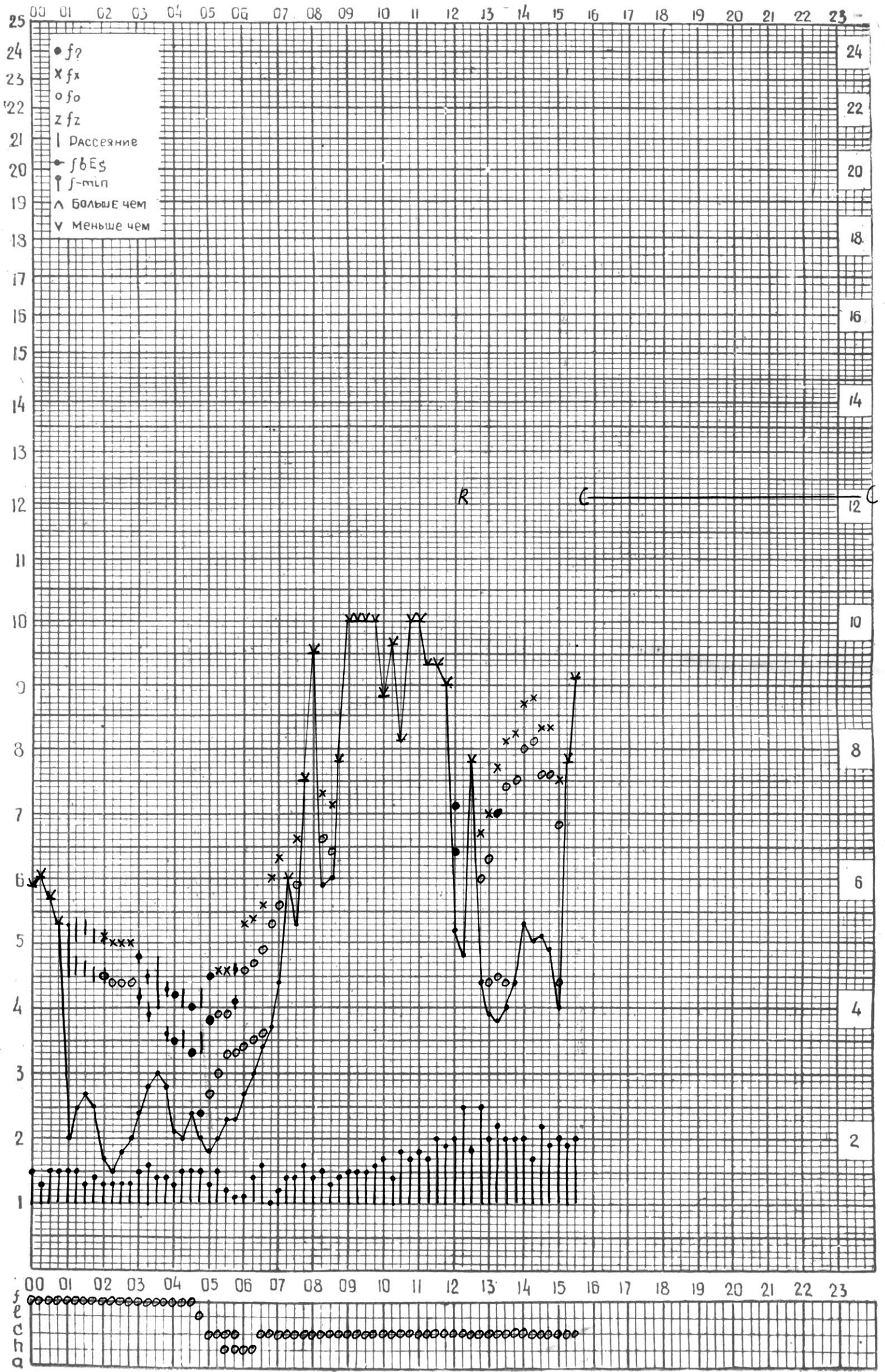
СТАНЦИЯ ТБИЛИСИ F—ГРАФИК ИОНОСФЕРНЫХ ДАННЫХ, ДАТА 26 ИЮНЯ, 1974
