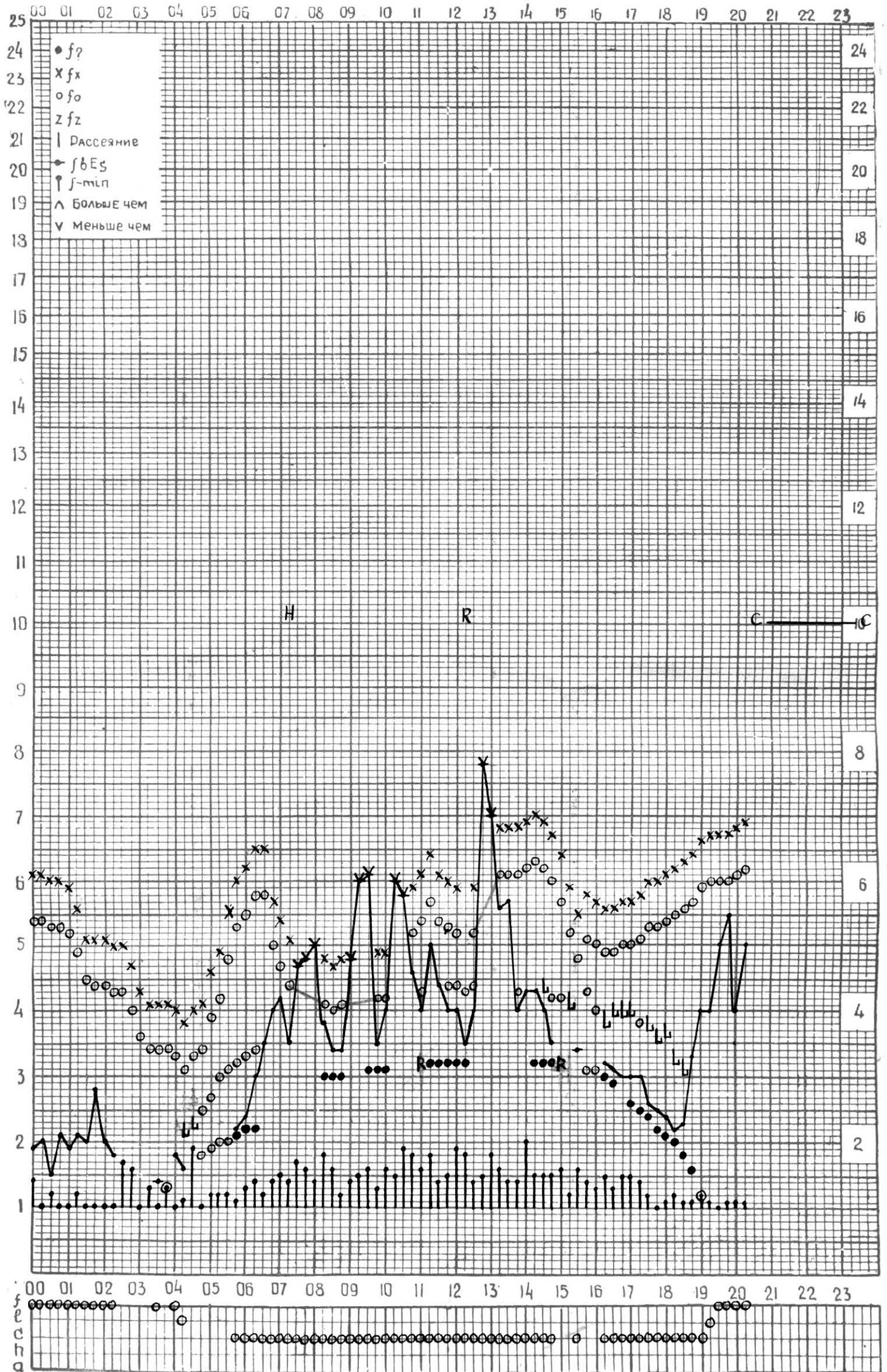
СТАНЦИЯ ТБИЛИСИ F-ГРАФИК ИОНОСФЕРНЫХ ДАННЫХ, ДАТА 16 ИЮНЯ, 1974
