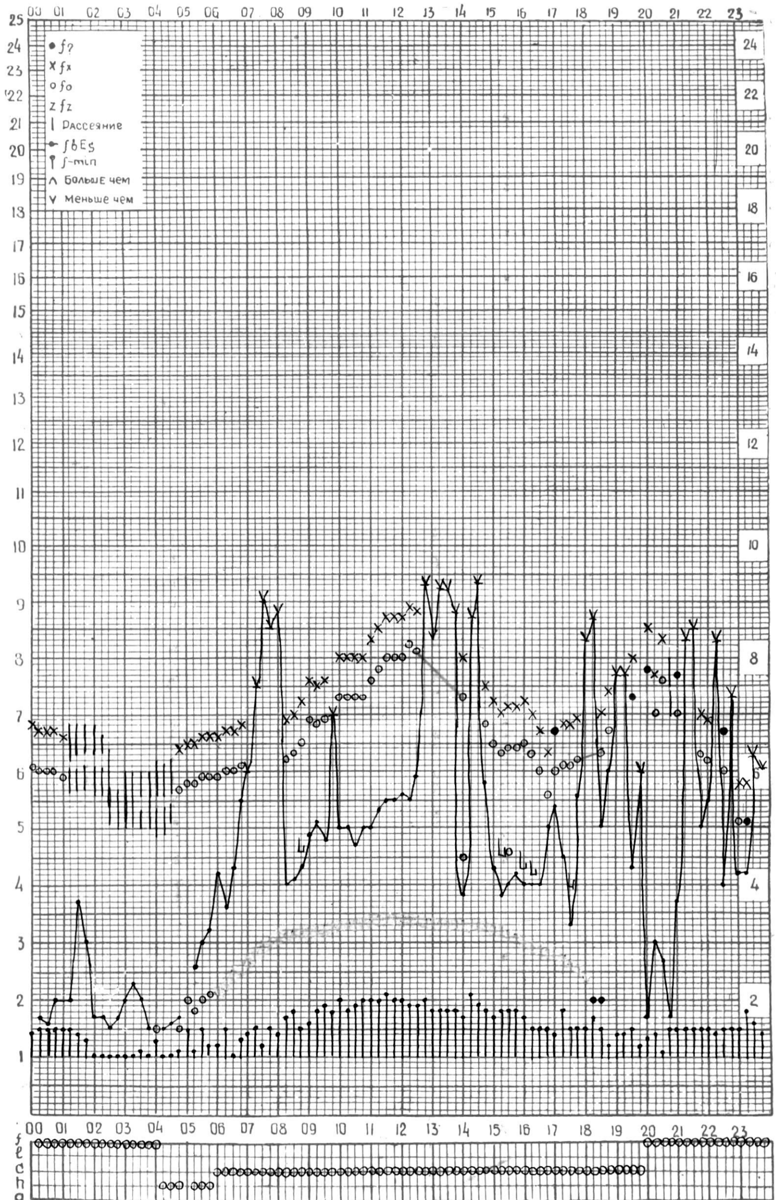
СТАНЦИЯ ТБИЛИСИ F—ГРАФИК ИОНОСФЕРНЫХ ДАННЫХ, ДАТА 5 ИЮНЯ, 1974
