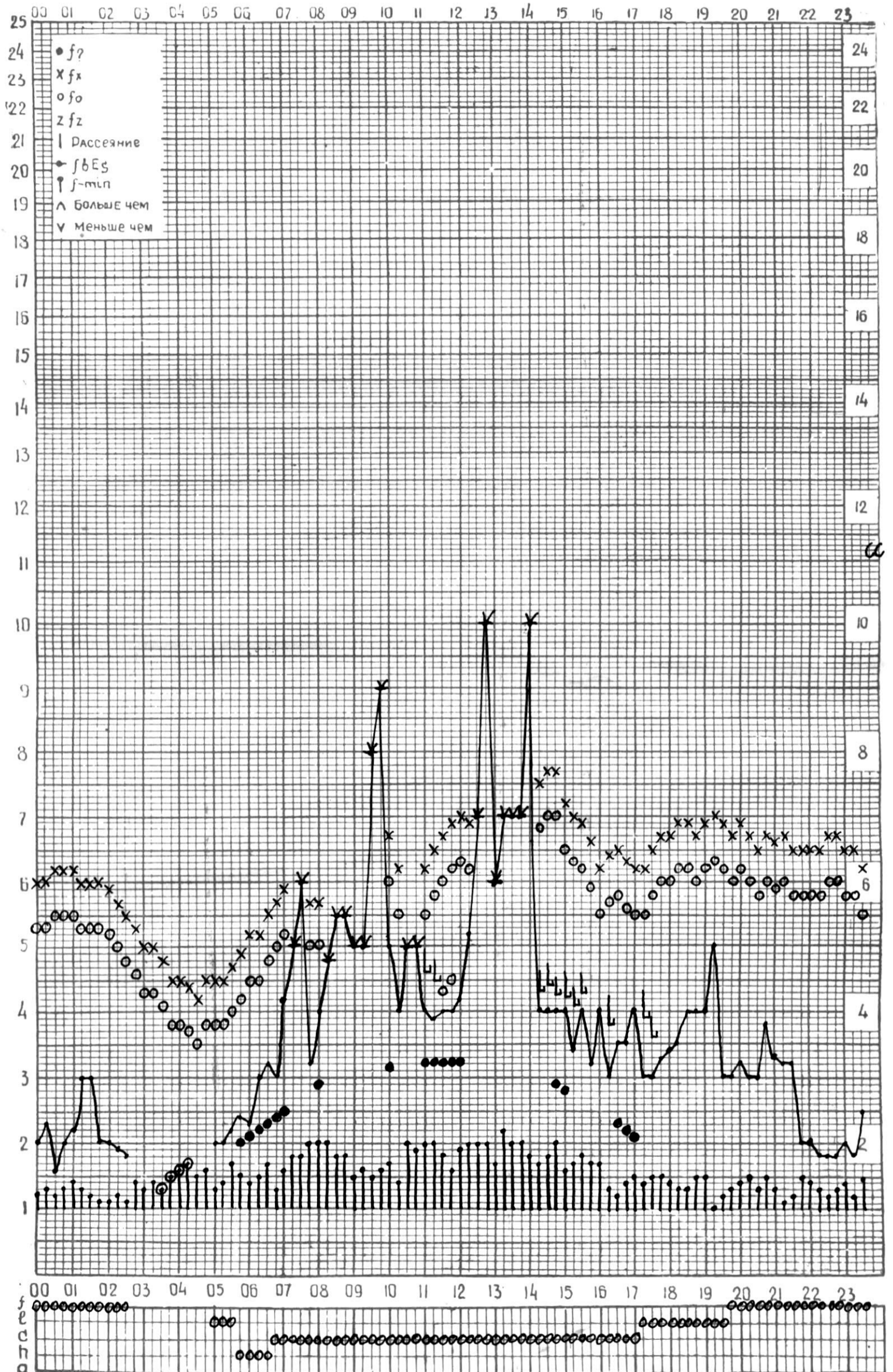
СТАНЦИЯ ТБИЛИСИ F-ГРАФИК ИОНОСФЕРНЫХ ДАННЫХ, ДАТА 15 ИЮНЯ, 1974
