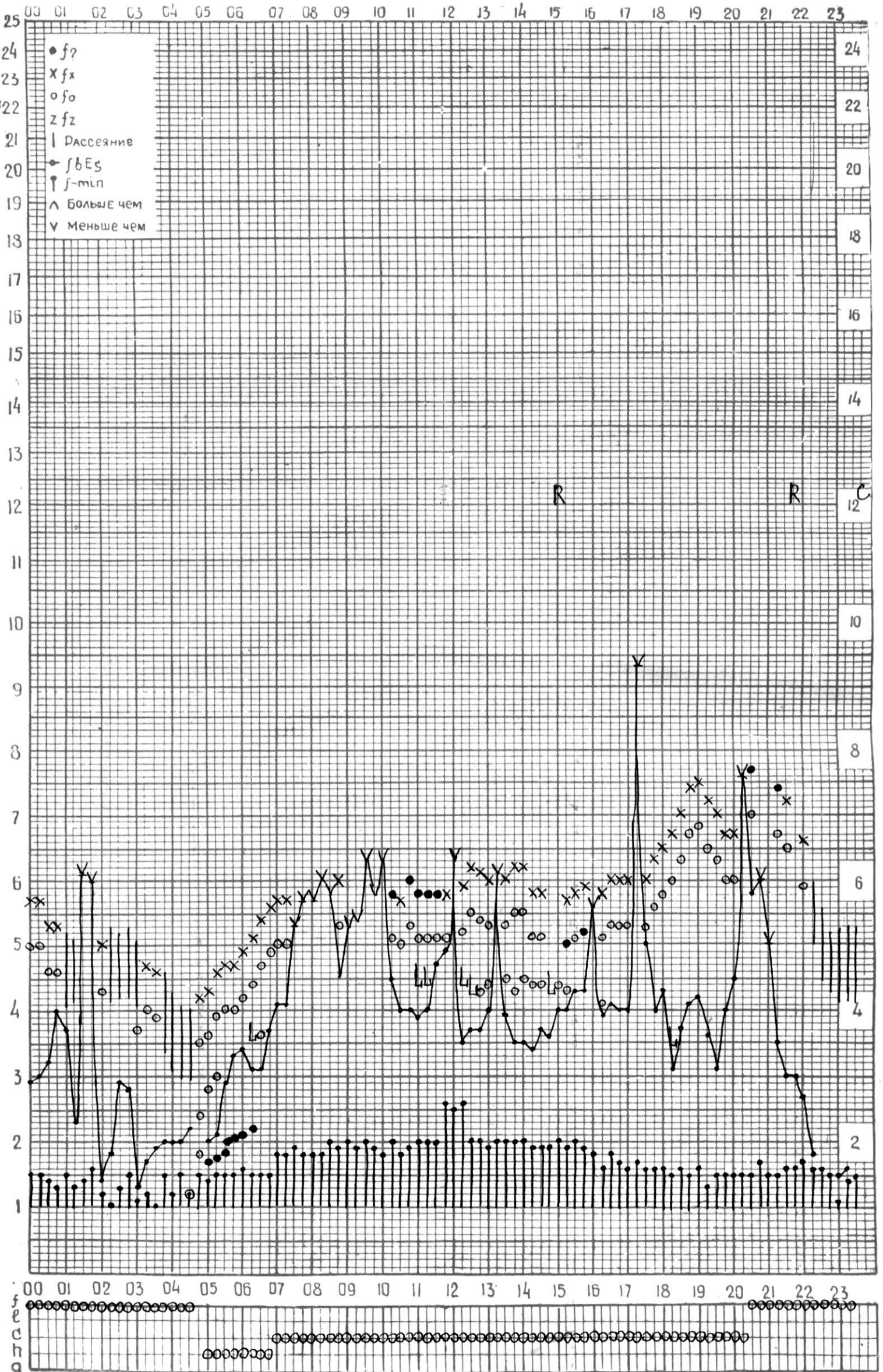
СТАНЦИЯ ТБИЛИСИ F-ГРАФИК ИОНОСФЕРНЫХ ДАННЫХ, ДАТА 29 ИЮНЯ, 1974
