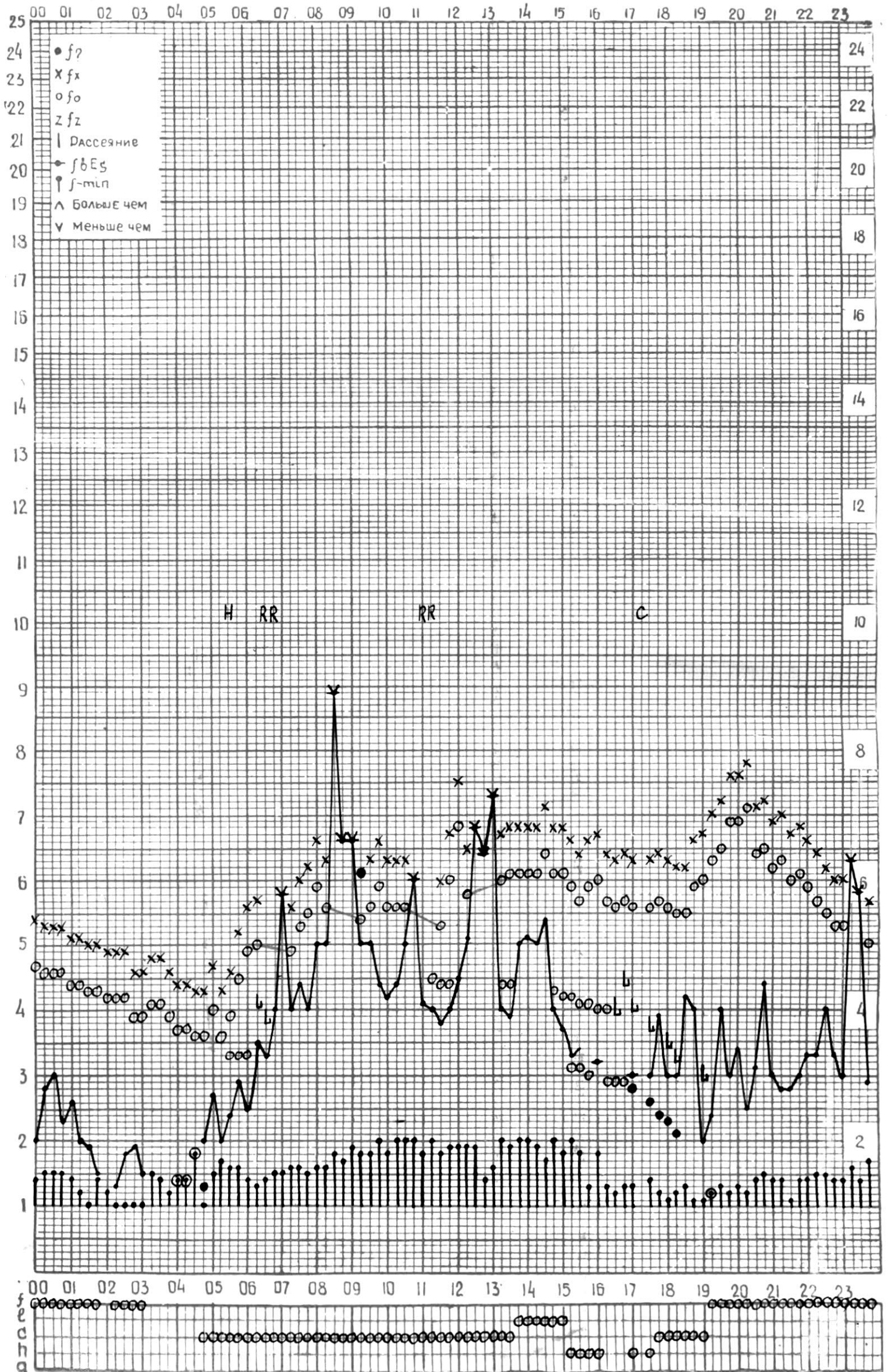
СТАНЦИЯ ТБИЛИСИ F-ГРАФИК ИОНОСФЕРНЫХ ДАННЫХ, ДАТА 28 ИЮНЯ, 1974
