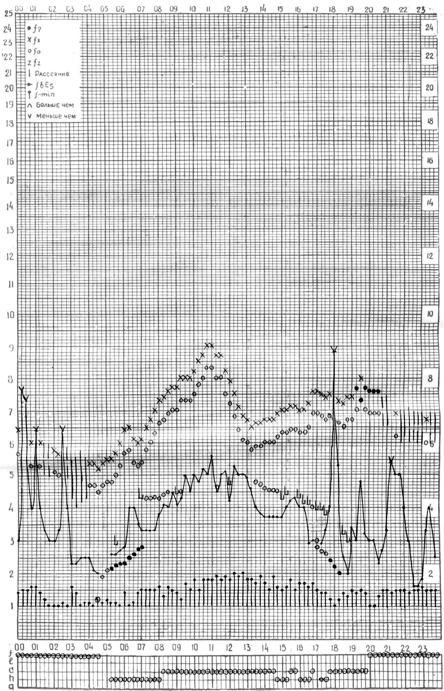
СТАНЦИЯ ТБИЛИСИ F-ГРАФИК ИОНОСФЕРНЫХ ДАННЫХ, ДАТА 9 ИЮНЯ, 1974
