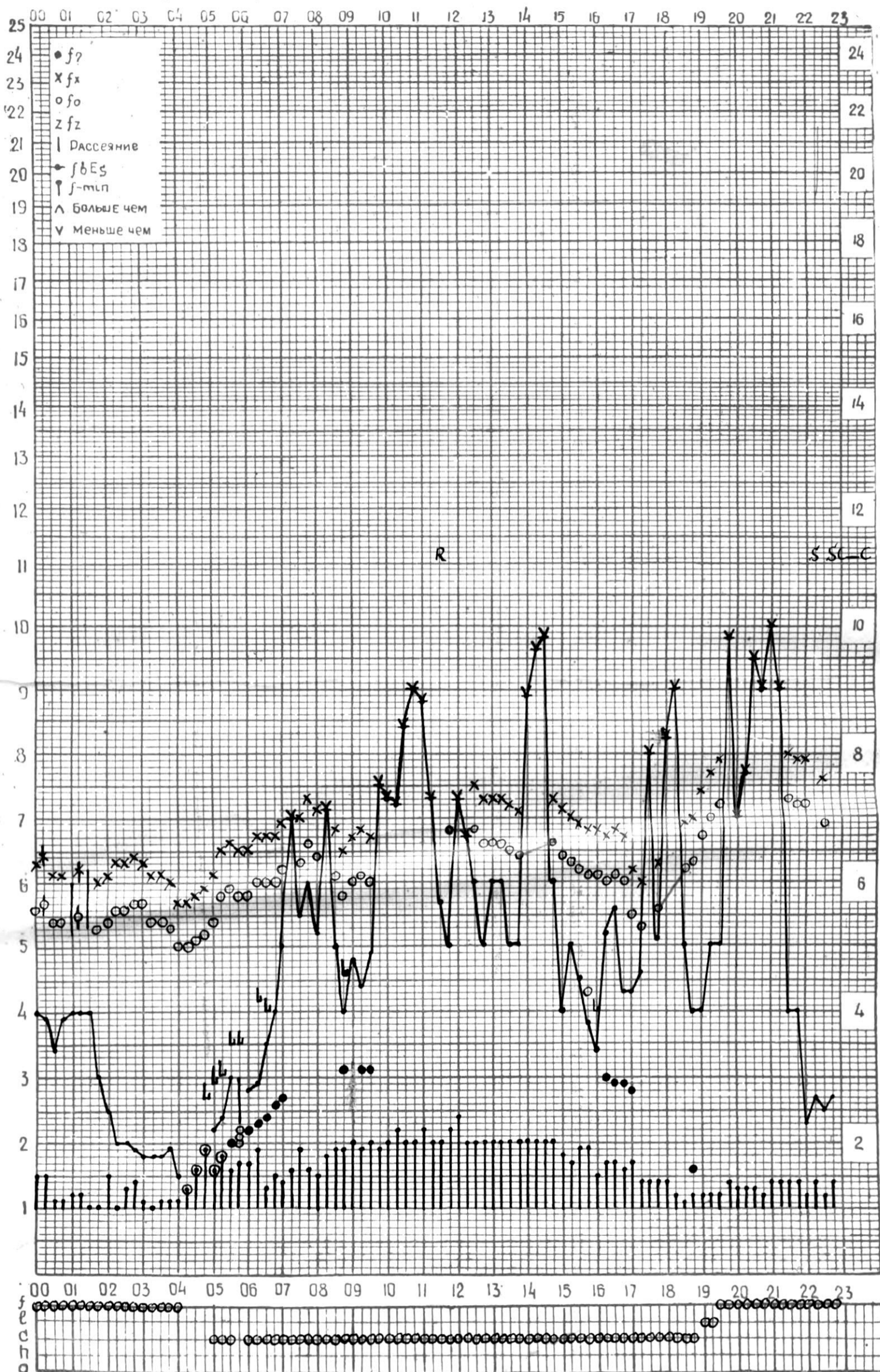
СТАНЦИЯ ТБИЛИСИ F—ГРАФИК ИОНОСФЕРНЫХ ДАННЫХ, ДАТА 4 ИЮНЯ, 1974
