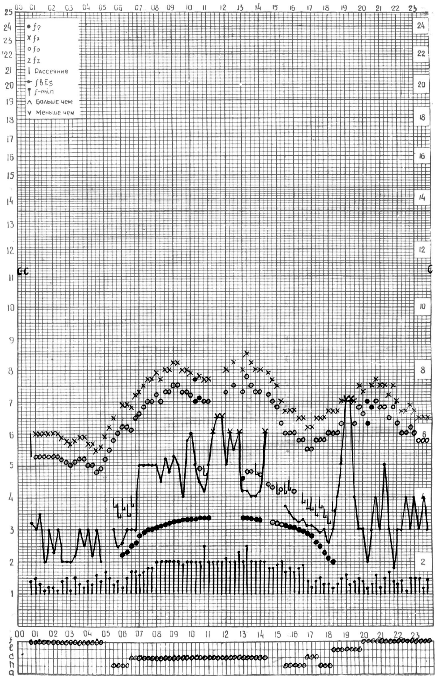
СТАНЦИЯ ТБИЛИСИ F-ГРАФИК ИОНОСФЕРНЫХ ДАННЫХ, ДАТА 7 ИЮНЯ, 1974
