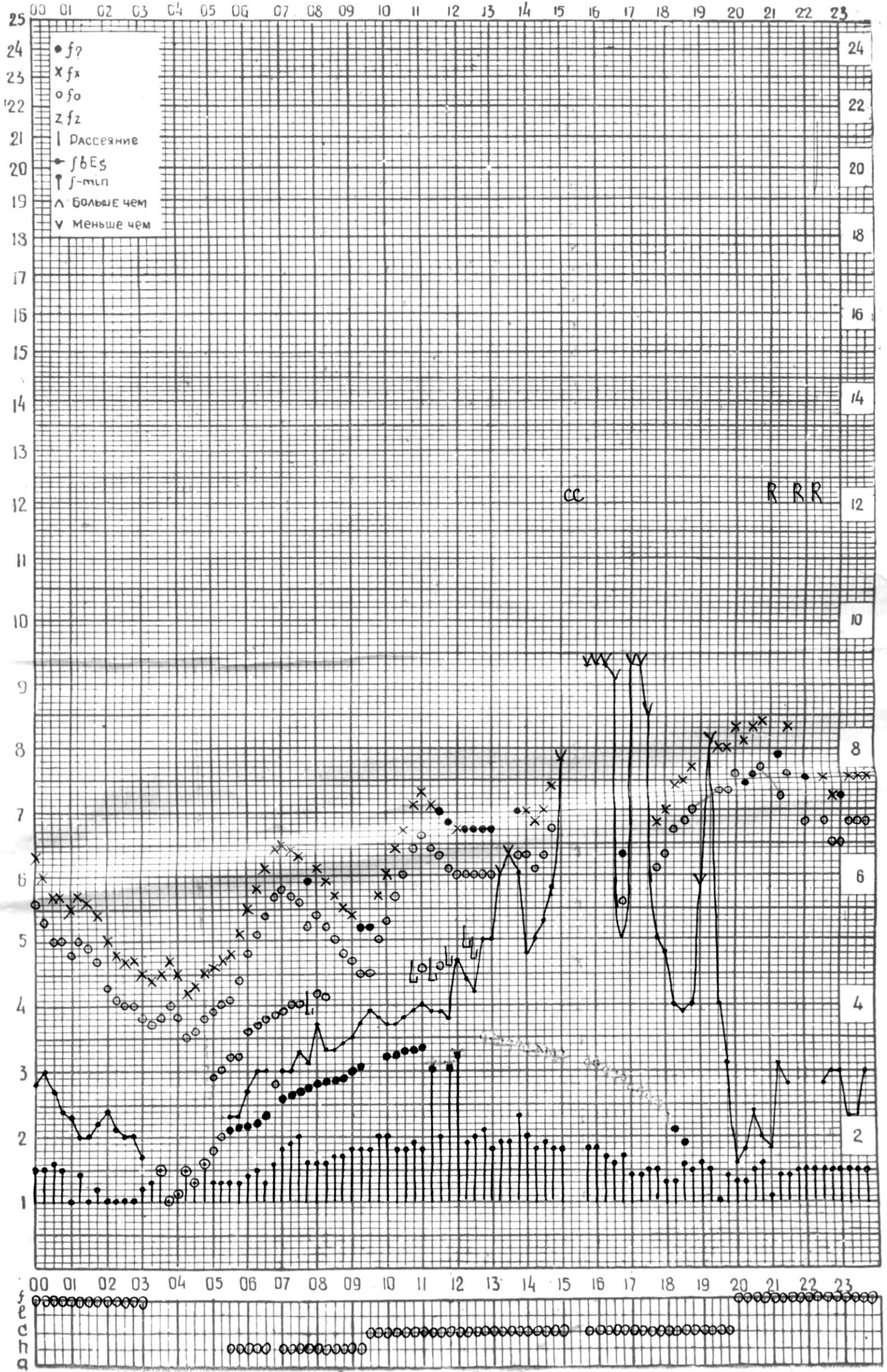
СТАНЦИЯ ТБИЛИСИ F—ГРАФИК ИОНОСФЕРНЫХ ДАННЫХ, ДАТА 1 ИЮНЯ, 1974
