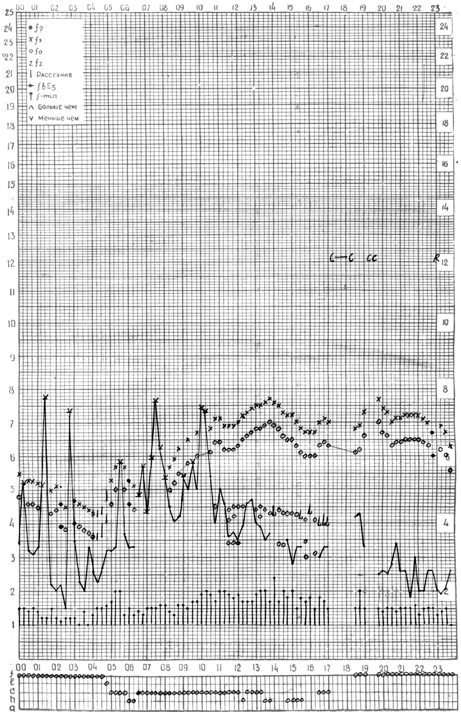
СТАНЦИЯ ТБИЛИСИ F-ГРАФИК ИОНОСФЕРНЫХ ДАННЫХ, ДАТА 14 ИЮНЯ, 1974
