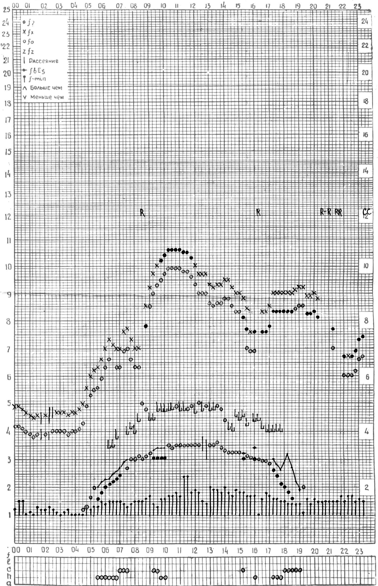
СТАНЦИЯ ТБИЛИСИ F-ГРАФИК ИОНОСФЕРНЫХ ДАННЫХ, ДАТА 4 МАЯ 1974
