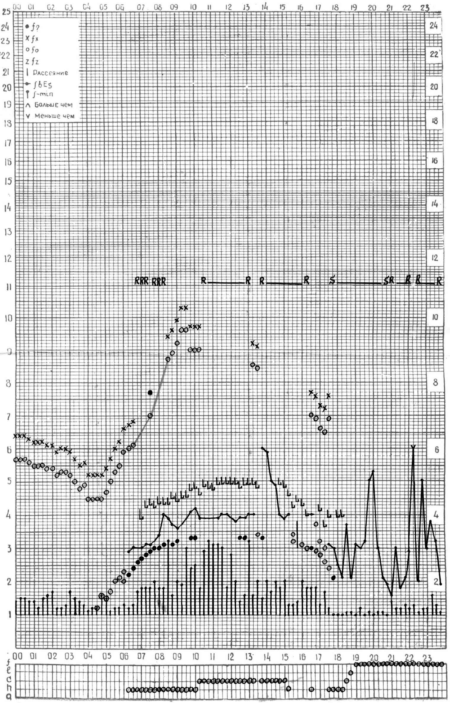
СТАНЦИЯ ТБИЛИСИ F-ГРАФИК ИОНОСФЕРНЫХ ДАННЫХ, ДАТА 7 МАЯ, 1974
