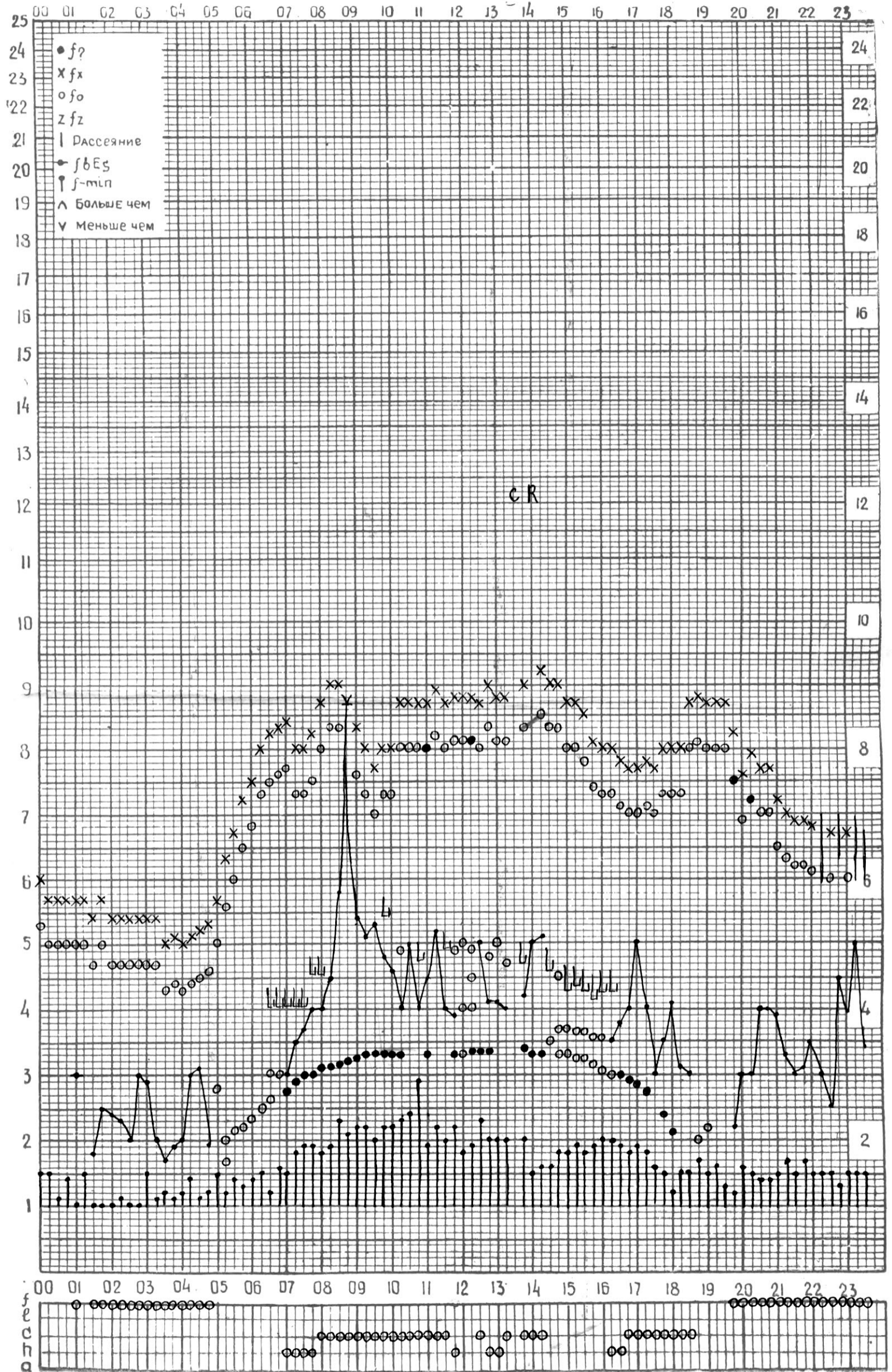
СТАНЦИЯ ТБИЛИСИ F-ГРАФИК ИОНОСФЕРНЫХ ДАННЫХ, ДАТА 12 МАЯ, 1974
