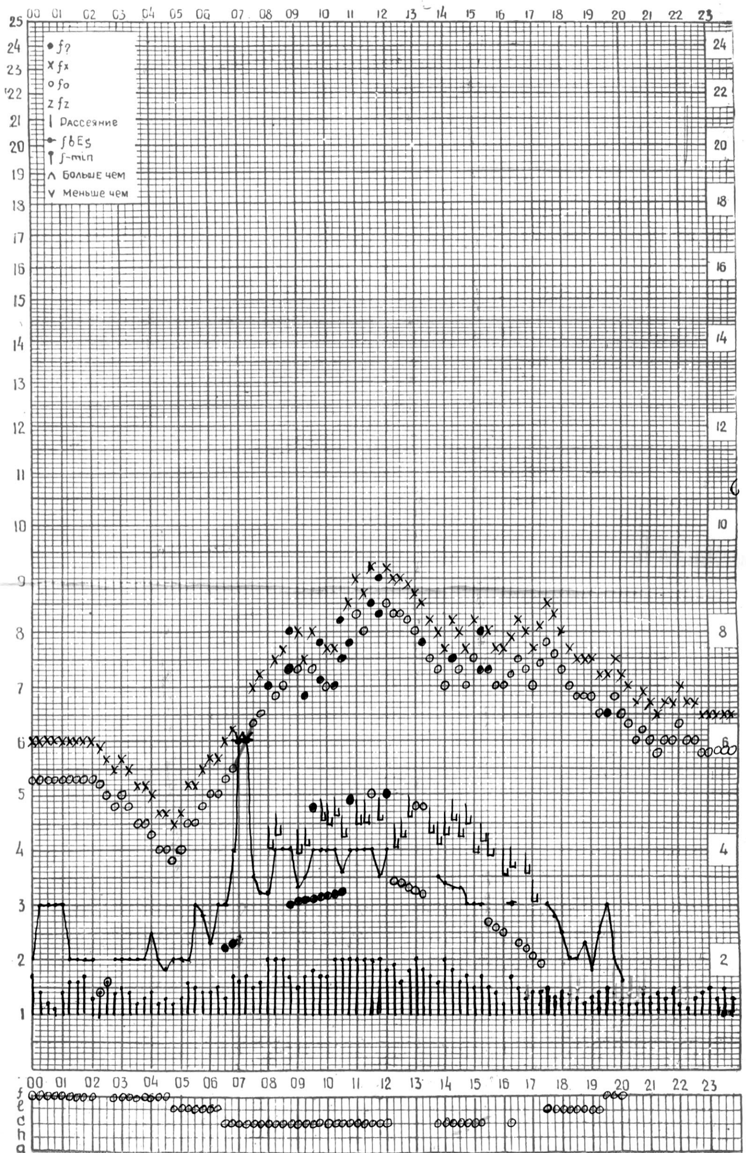
СТАНЦИЯ ТБИЛИСИ F-ГРАФИК ИОНОСФЕРНЫХ ДАННЫХ, ДАТА 6 МАЯ, 1974
