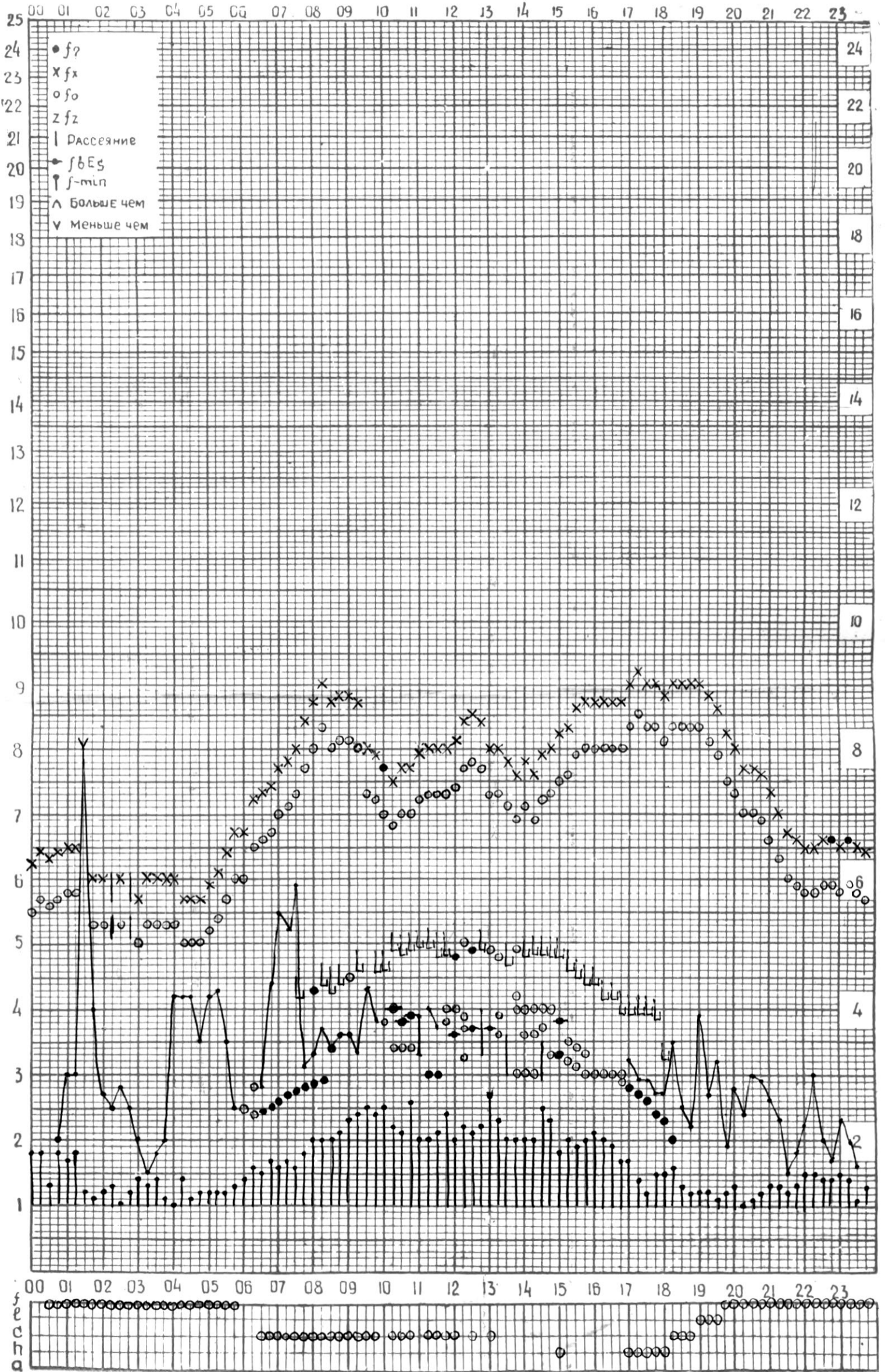
СТАНЦИЯ ТБИЛИСИ F—ГРАФИК ИОНОСФЕРНЫХ ДАННЫХ, ДАТА 11 МАЯ, 1974
