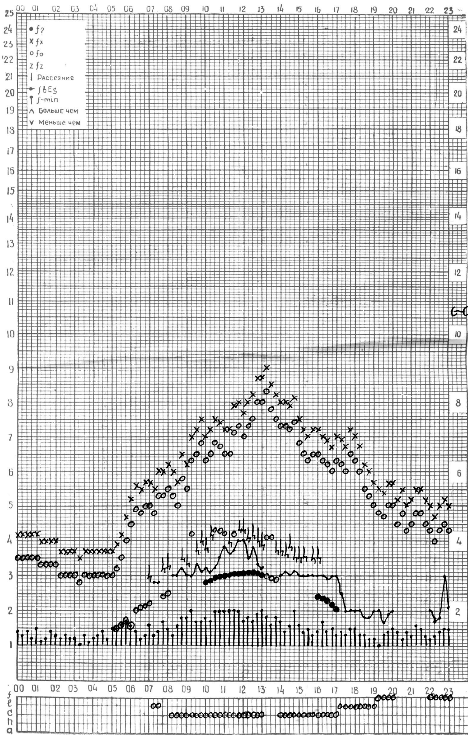
СТАНЦИЯ ТБИЛИСИ F-ГРАФИК ИОНОСФЕРНЫХ ДАННЫХ, ДАТА 31 МАРТА, 1974
