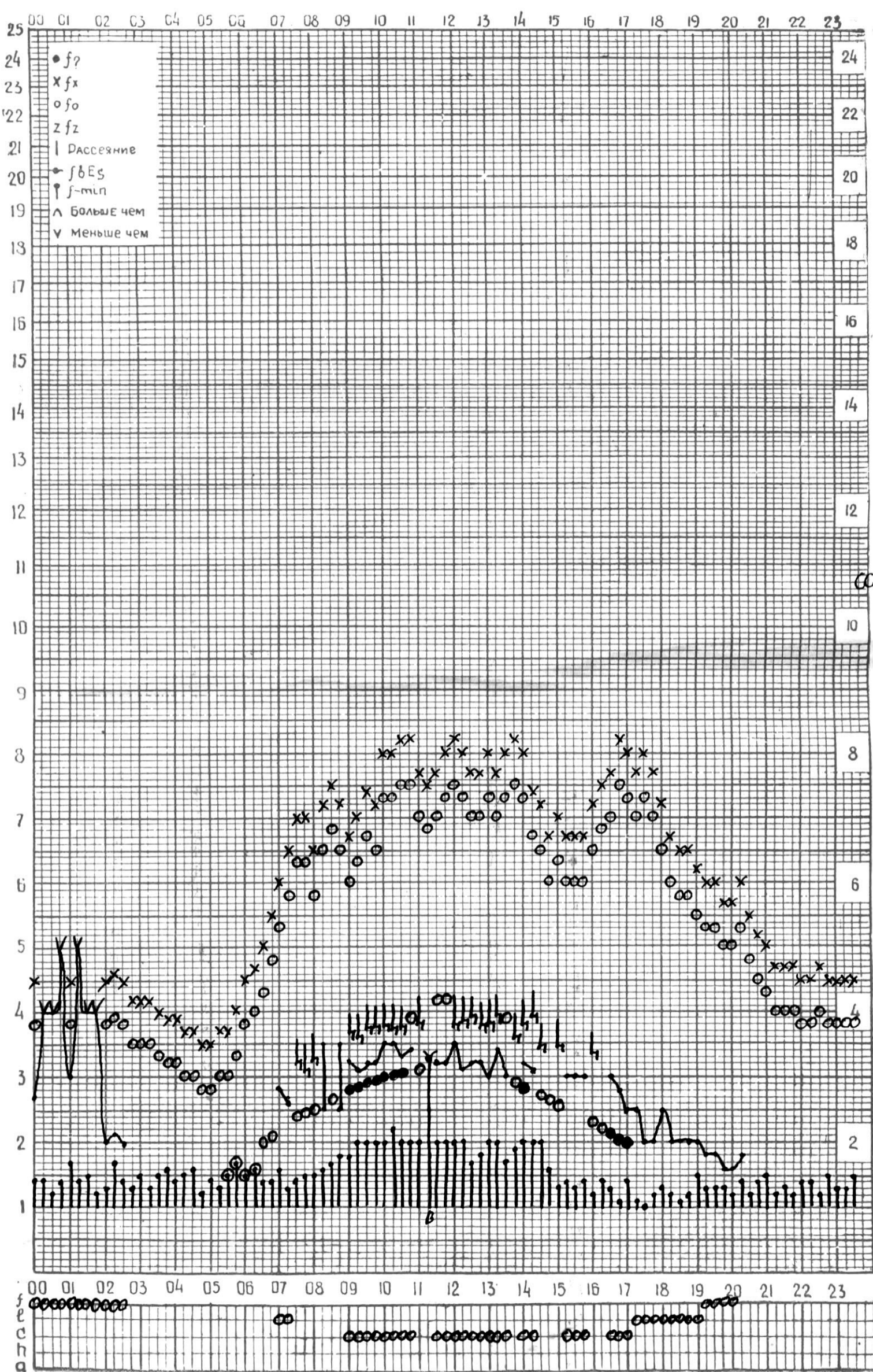
СТАНЦИЯ ТБИЛИСИ F-ГРАФИК ИОНОСФЕРНЫХ ДАННЫХ, ДАТА 27 МАРТА, 1974
