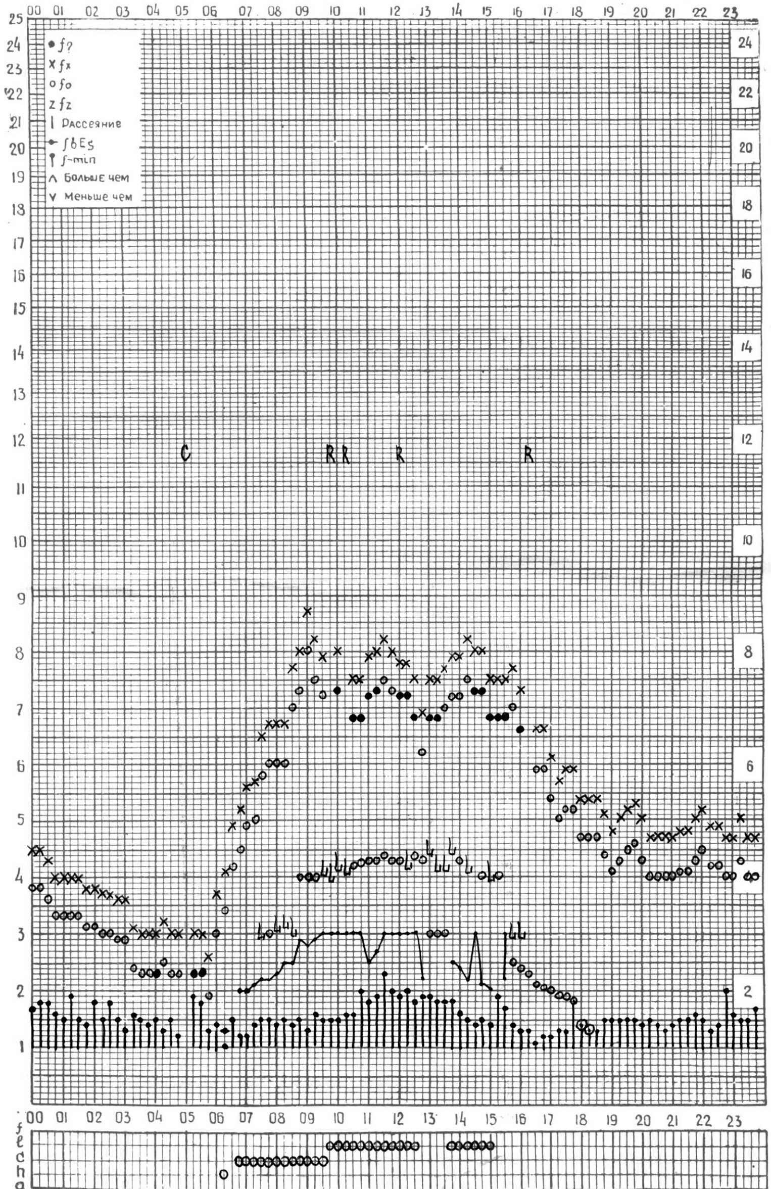
СТАНЦИЯ ТБИЛИСИ F-ГРАФИК ИОНОСФЕРНЫХ ДАННЫХ, ДАТА 10 МАРТА, 1974
