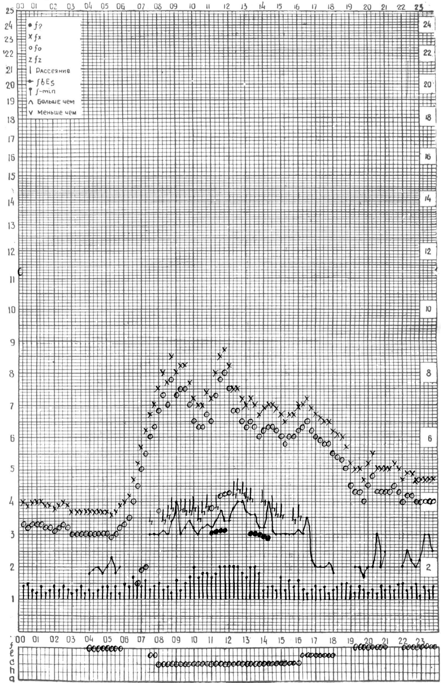
СТАНЦИЯ ТБИЛИСИ F-ГРАФИК ИОНОСФЕРНЫХ ДАННЫХ, ДАТА 7 МАРТА, 1924
