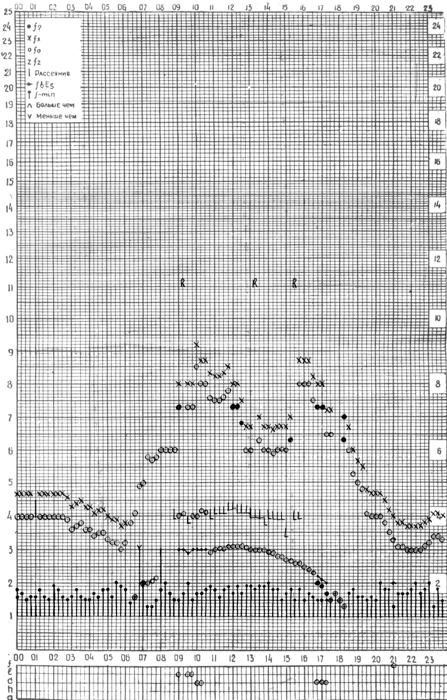
СТАНЦИЯ ТБИЛИСИ F-ГРАФИК ИОНОСФЕРНЫХ ДАННЫХ, ДАТА 6 МАРТА, 1974
