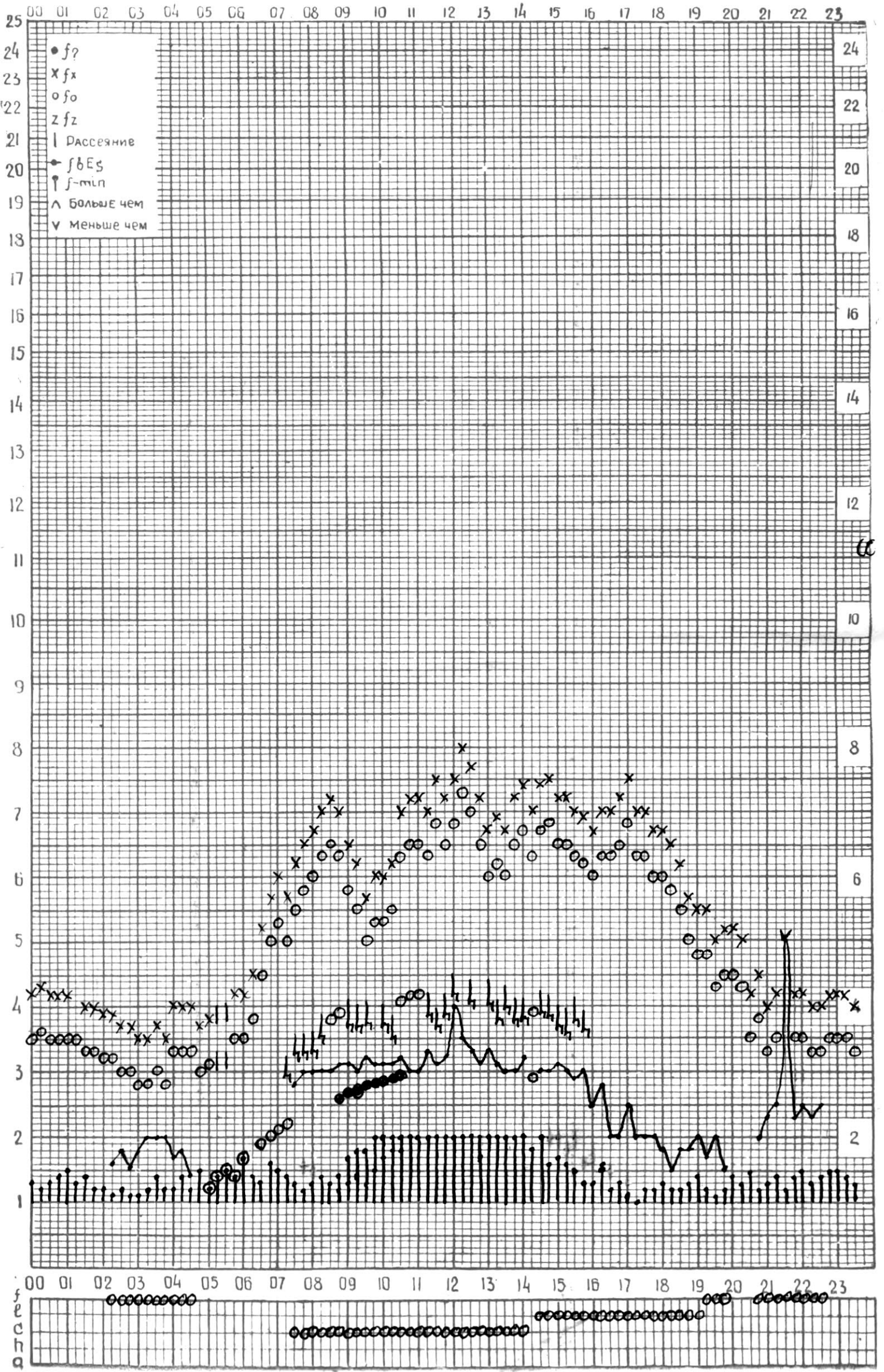
СТАНЦИЯ ТБИЛИСИ F-ГРАФИК ИОНОСФЕРНЫХ ДАННЫХ, ДАТА 23 МАРТА, 1974
