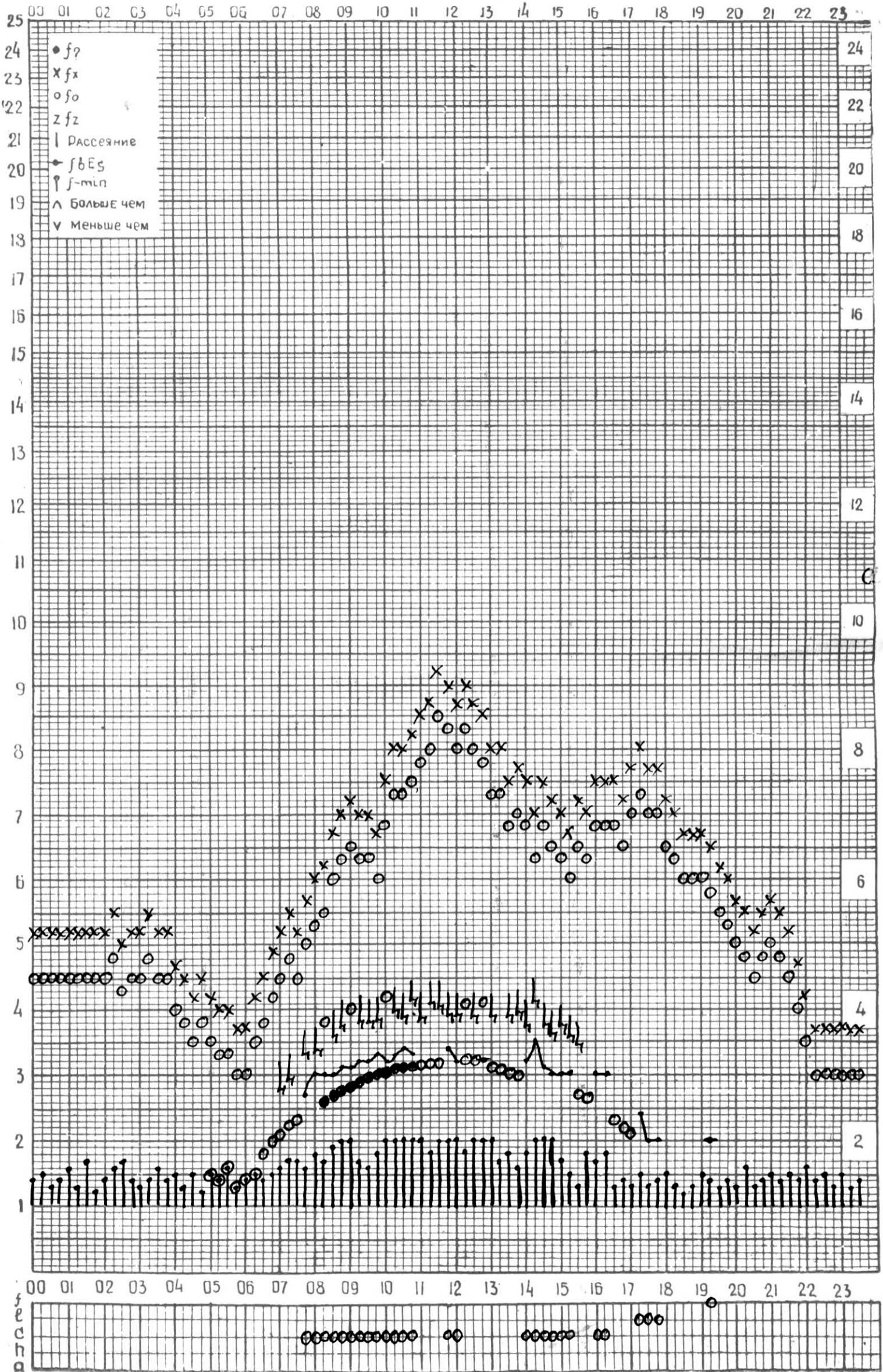
СТАНЦИЯ ТБИЛИСИ F-ГРАФИК ИОНОСФЕРНЫХ ДАННЫХ, ДАТА 15 МАРТА 1974
