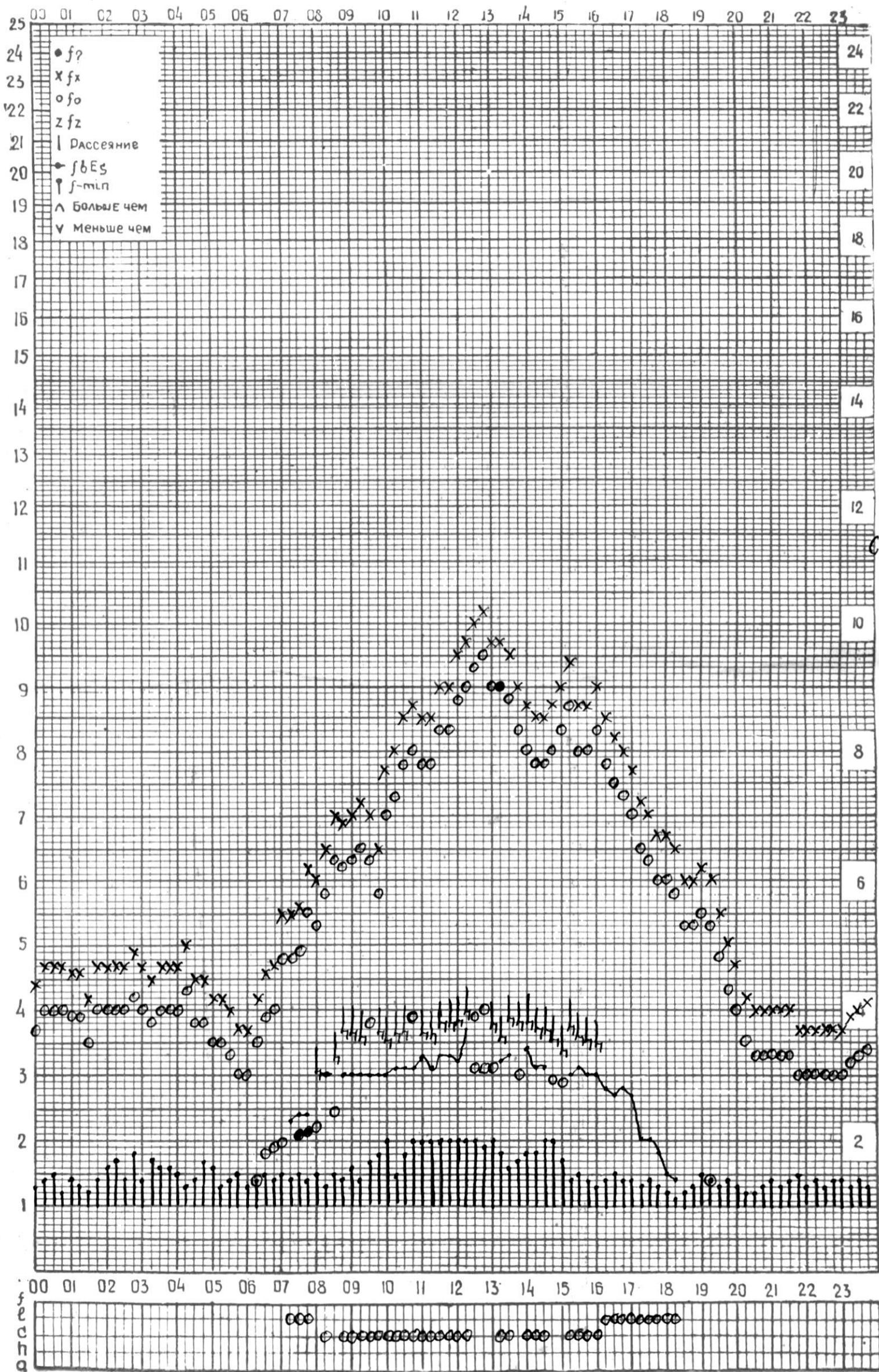
СТАНЦИЯ ТБИЛИСИ F-ГРАФИК ИОНОСФЕРНЫХ ДАННЫХ, ДАТА 11 МАРТА, 1974
