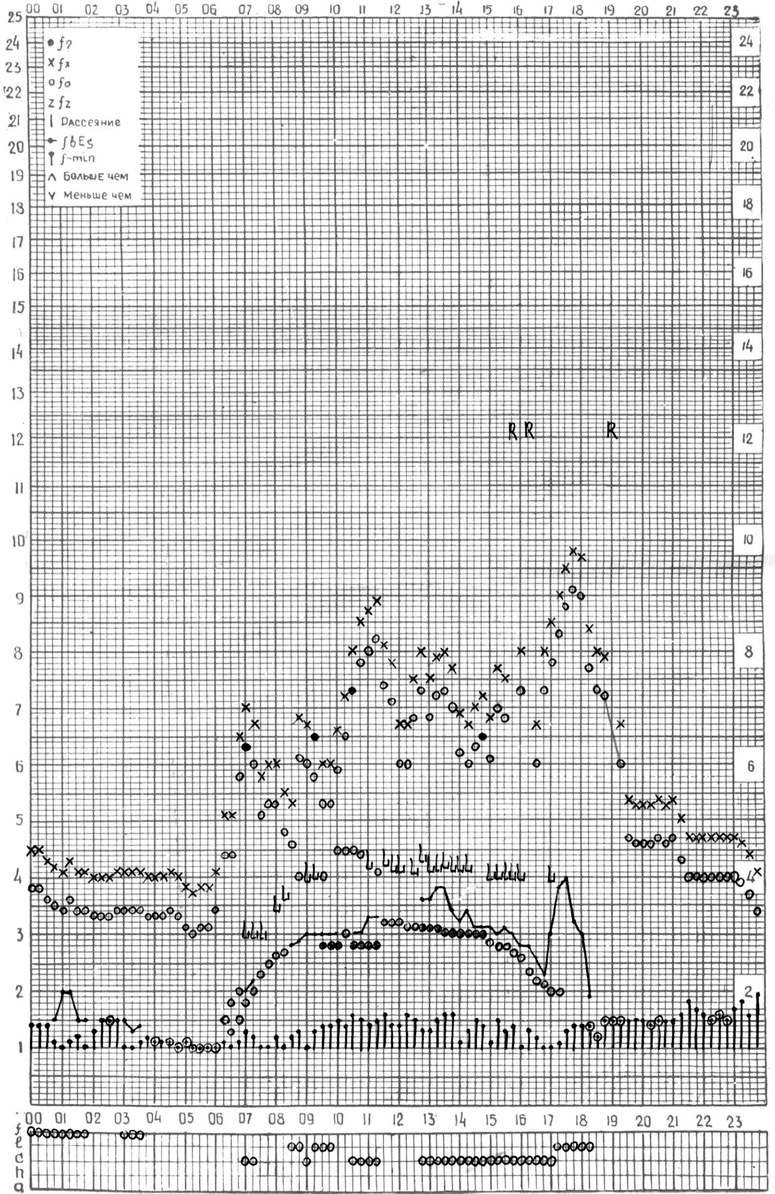
СТАНЦИЯ ТБИЛИСИ F—ГРАФИК ИОНОСФЕРНЫХ ДАННЫХ, ДАТА 21 МАРТА, 1974
