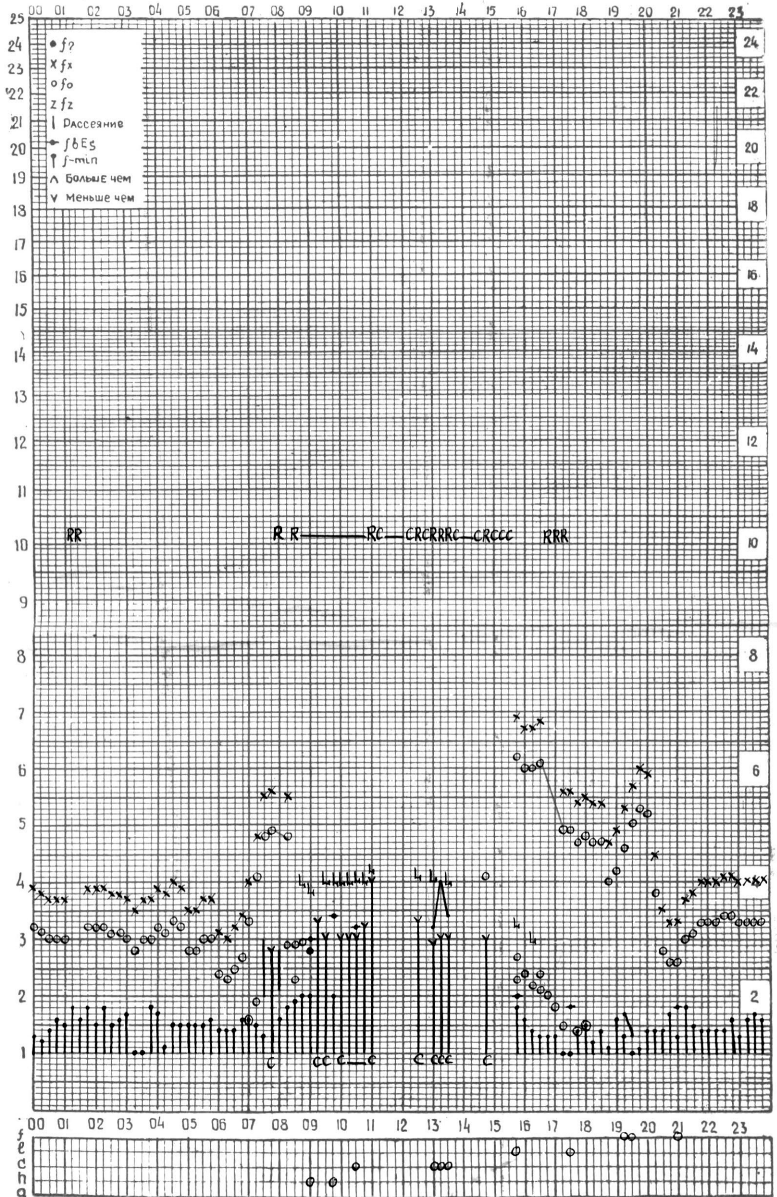
СТАНЦИЯ ТБИЛИСИ F-ГРАФИК ИОНОСФЕРНЫХ ДАННЫХ, ДАТА 11 ФЕВРАЛЯ 1974 Г
