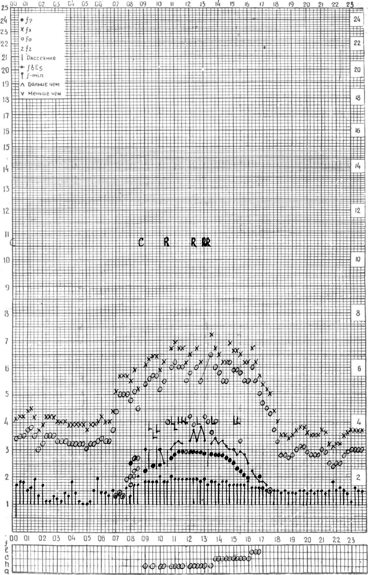
СТАНЦИЯ ТБИЛИСИ F-ГРАФИК ИОНОСФЕРНЫХ ДАННЫХ, ДАТА 6 ФЕВРАЛЯ 1974Г
