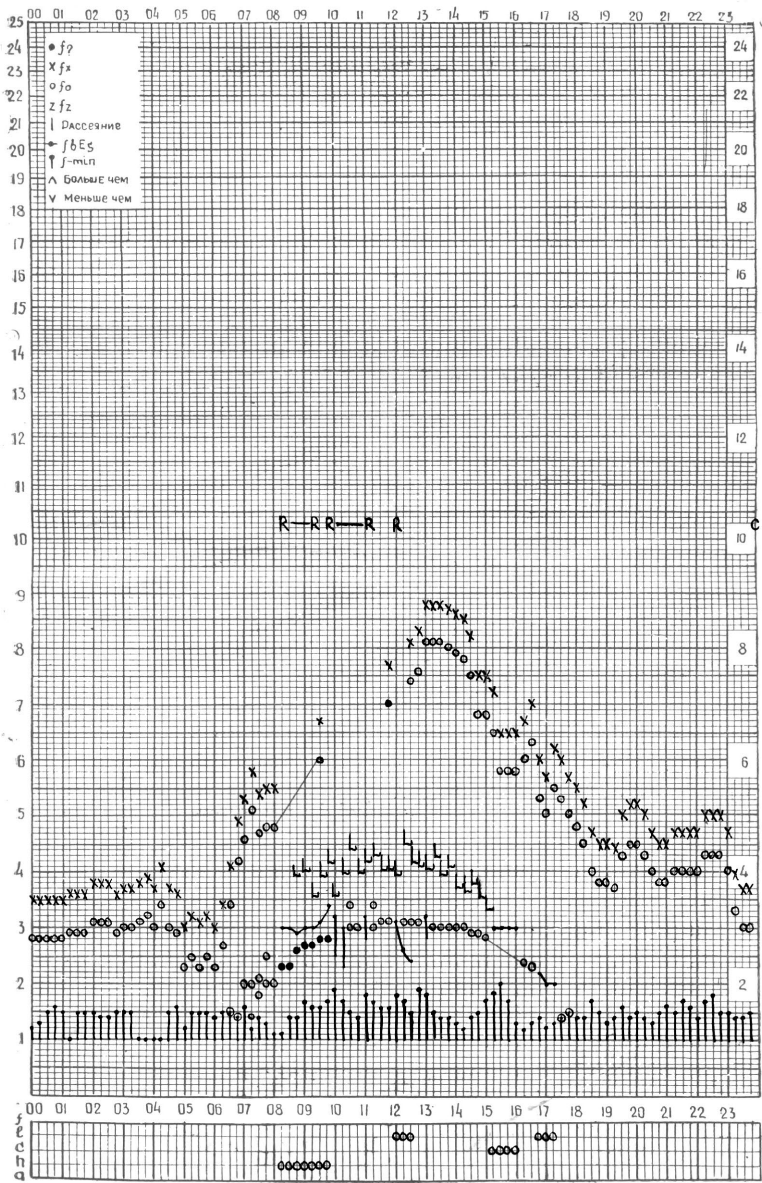
СТАНЦИЯ ТБИЛИСИ F-ГРАФИК ИОНОСФЕРНЫХ ДАННЫХ, ДАТА 23 ФЕВРАЛЯ 1974 Г
