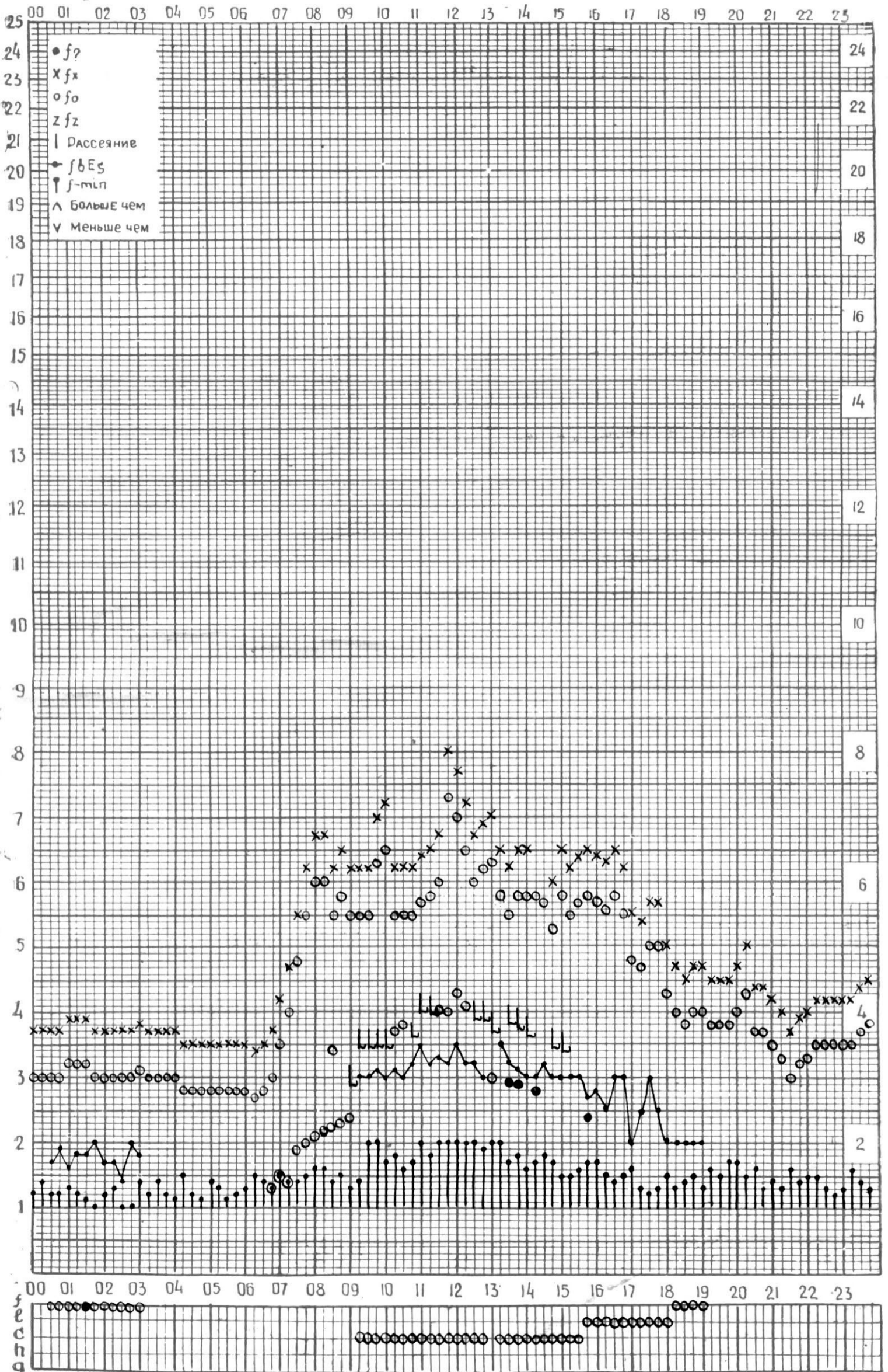
СТАНЦИЯ ТБИЛИСИ F—ГРАФИК ИОНОСФЕРНЫХ ДАННЫХ, ДАТА 7 ФЕВРАЛЯ 1974 Г
