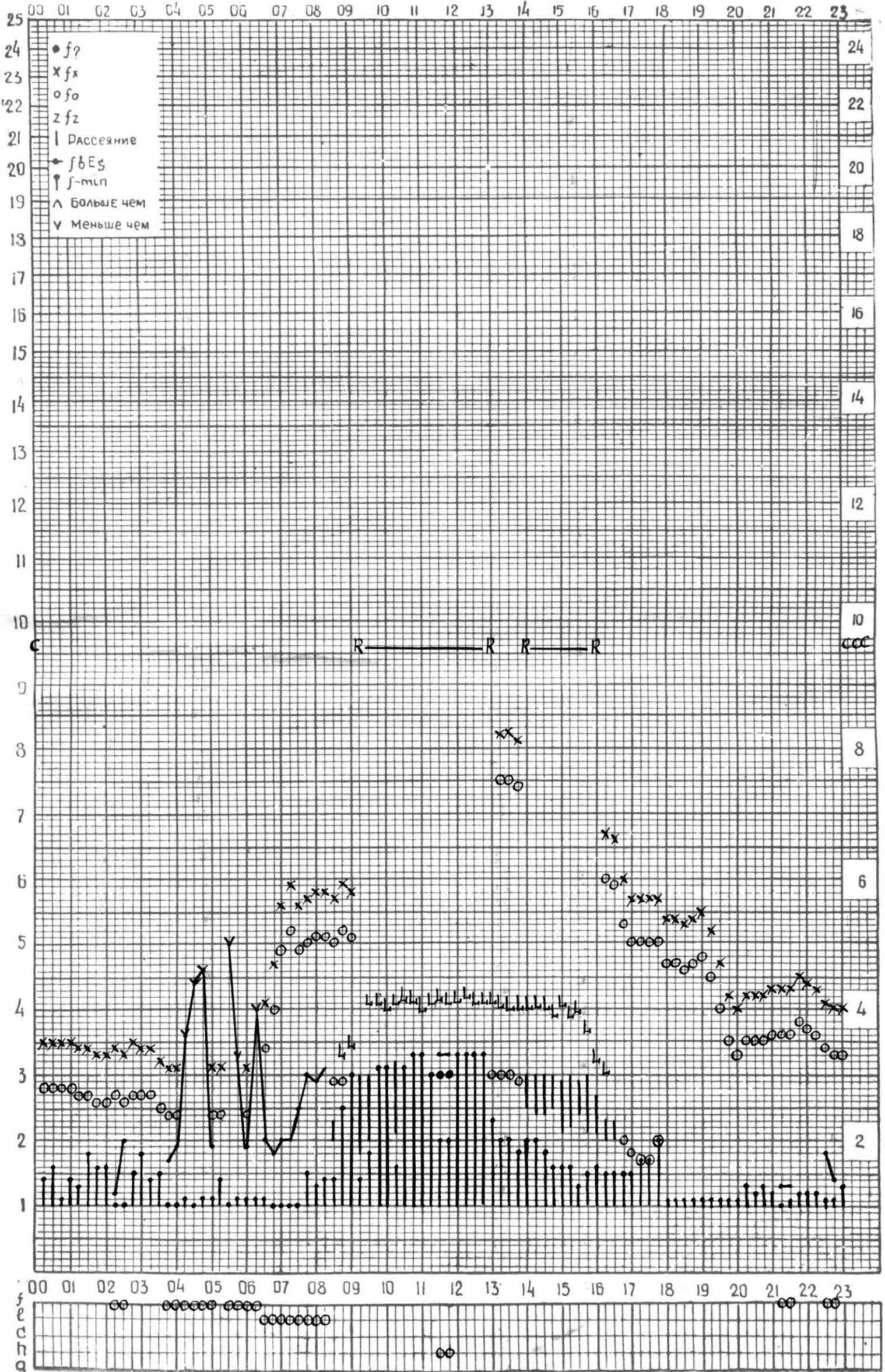
СТАНЦИЯ ТБИЛИСИ F-ГРАФИК ИОНОСФЕРНЫХ ДАННЫХ, ДАТ 28 ФЕВРАЛЯ 1974 Г
