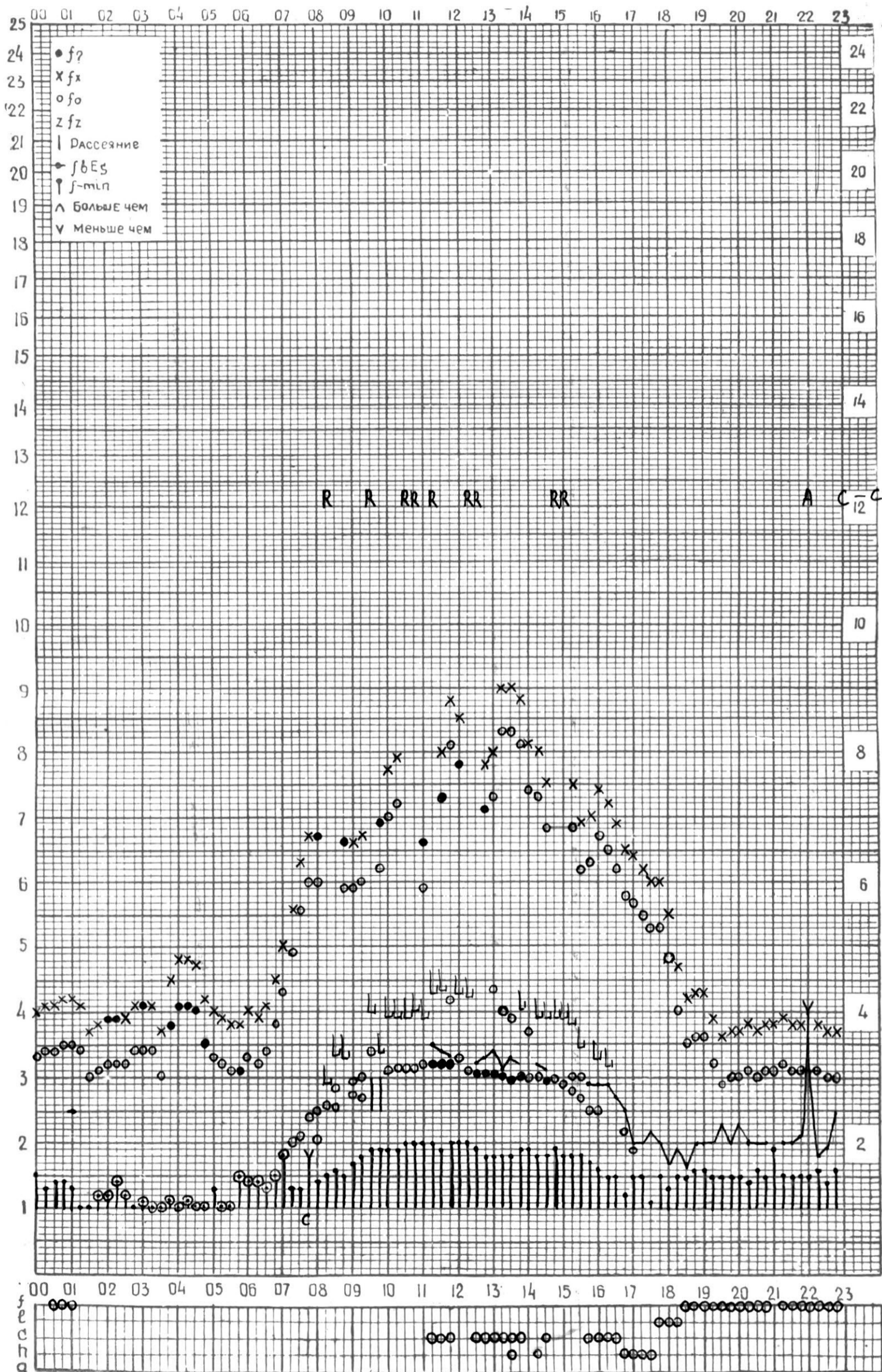
СТАНЦИЯ ТБИЛИСИ F-ГРАФИК ИОНОСФЕРНЫХ ДАННЫХ, ДАТА 25 ФЕВРАЛЯ 1974 Г
