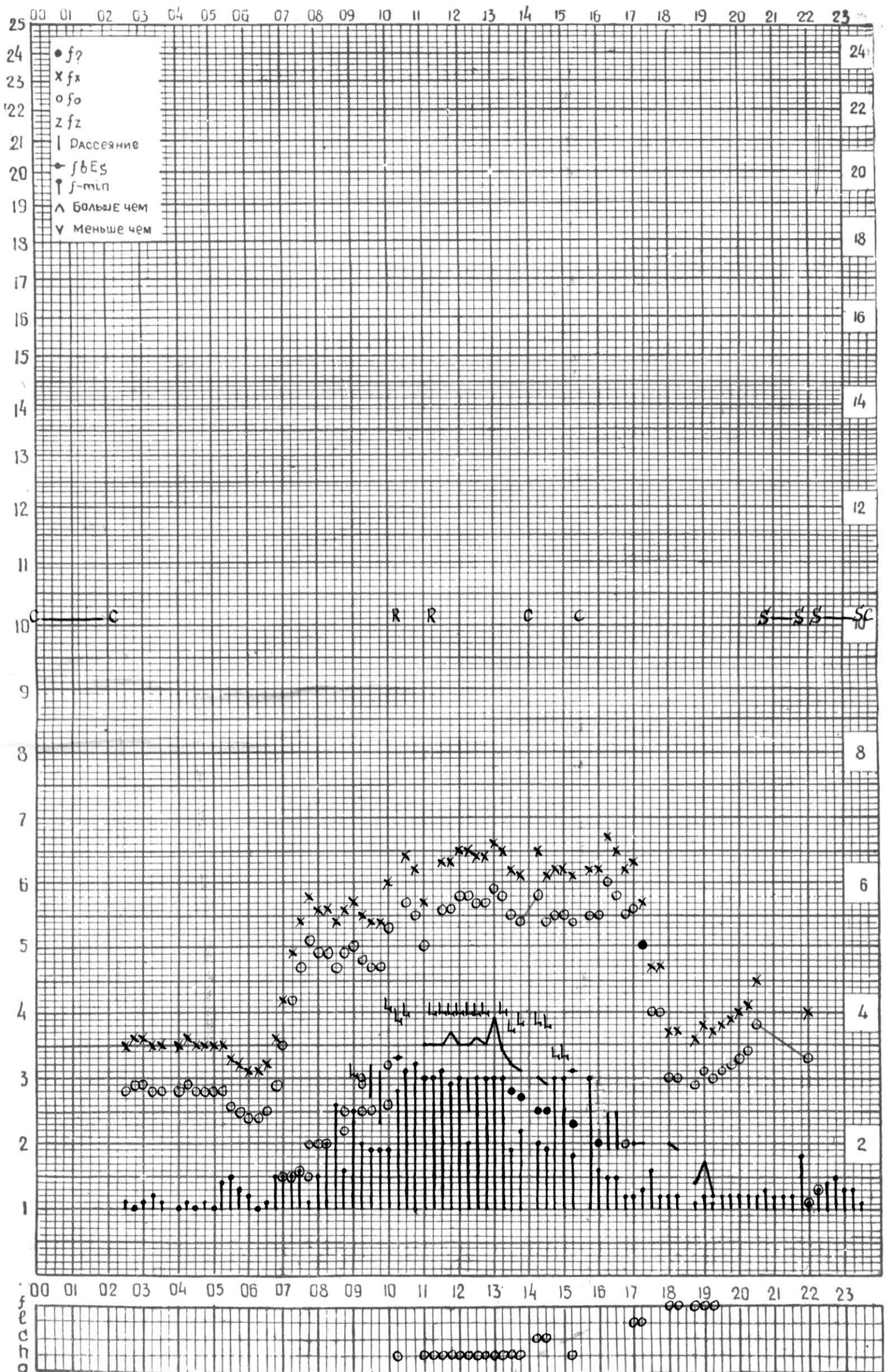
СТАНЦИЯ ТБИЛИСИ F-ГРАФИК ИОНОСФЕРНЫХ ДАННЫХ, ДАТА 4 ФЕВРАЛЯ 1974Г
