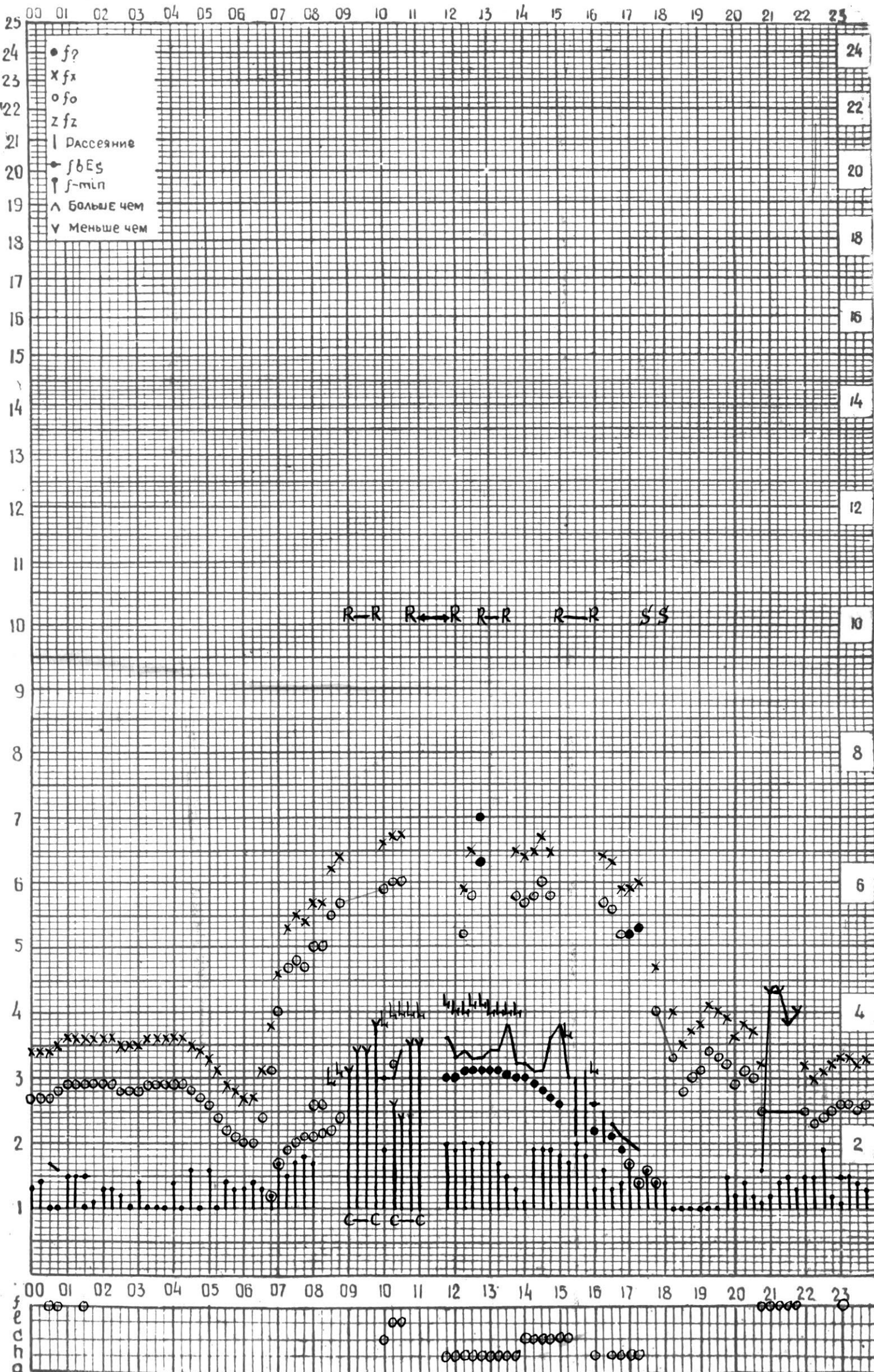
СТАНЦИЯ ТБИЛИСИ F-ГРАФИК ИОНОСФЕРНЫХ ДАННЫХ, ДАТА 15 ФЕВРАЛЯ 1974 Г
