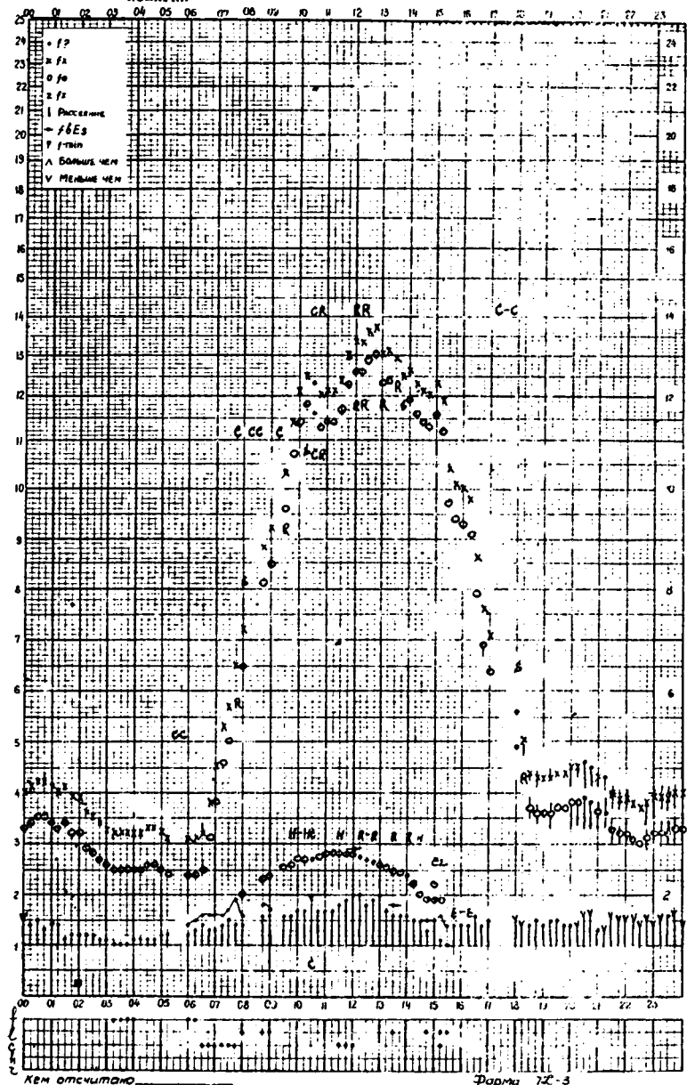
Время 30°E станция Москва f-график ионосферных данных дата 2 декабря 1959г. ИЗМИРАН
