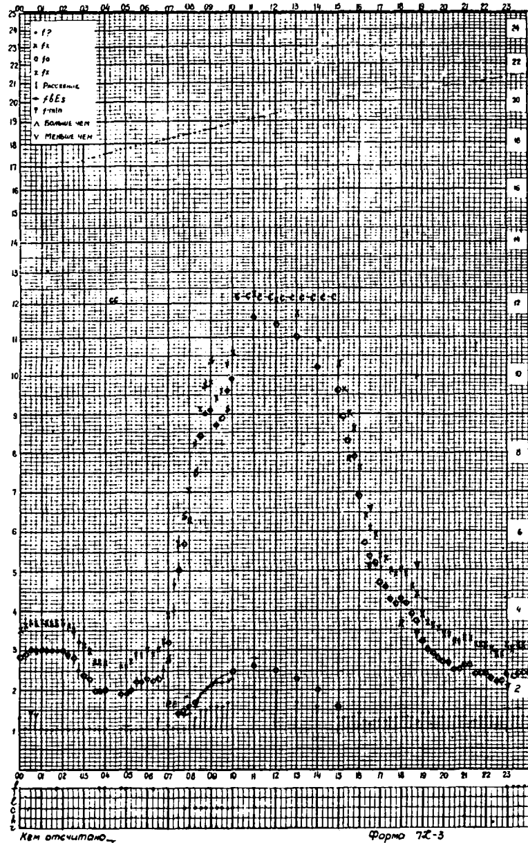
Время 30°E станция Москва f-график ионосферных данных дата 17 декабря 1959г. ИЗМИРАН
