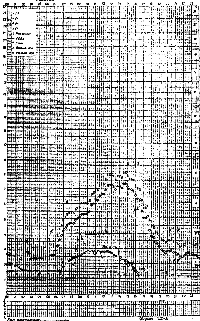
Время 30°E станция Москва f-график ионосферных данных дата 3 ноября 1959г. ИЗМИРАН
