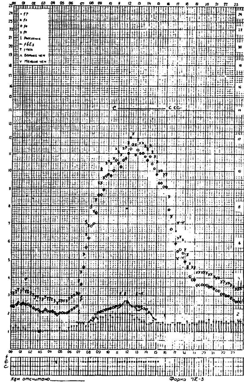
Время 30°E станция Москва f-график ионосферных данных дата 18 декабря 1959г. ИЗМИРАН
