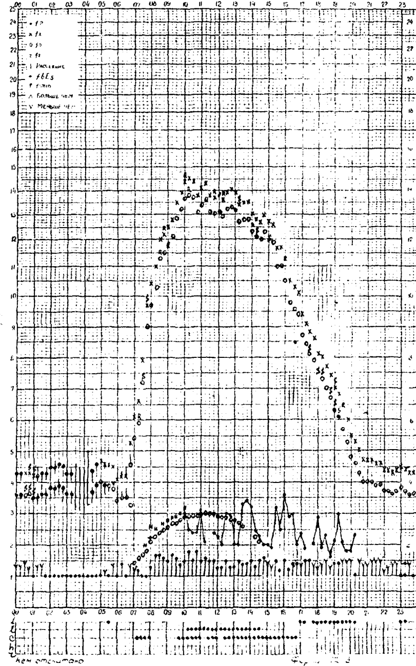
Москва время 30°E станция НИЗМИР f-график ионосферных данных дата 1 декабря 1958г
