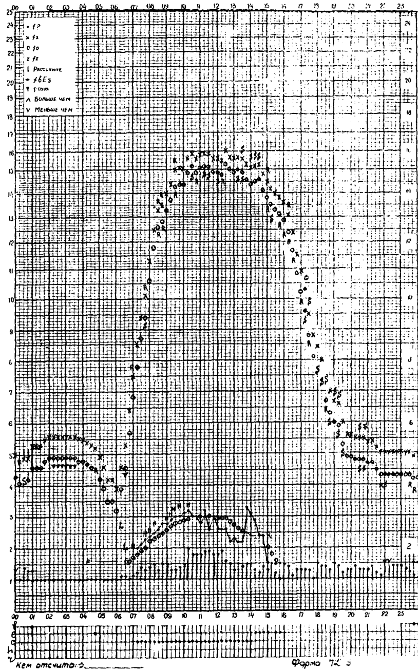
Модель 30° станция Низмид f- график ионосферных данных дата 18 ноября 1958г.
