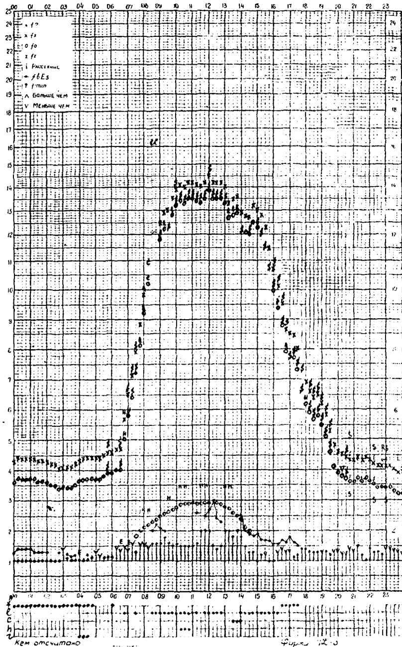
Москва время 30°E станция НИЗМИР f-график ионосферных данных дата 2 декабря 1958г
