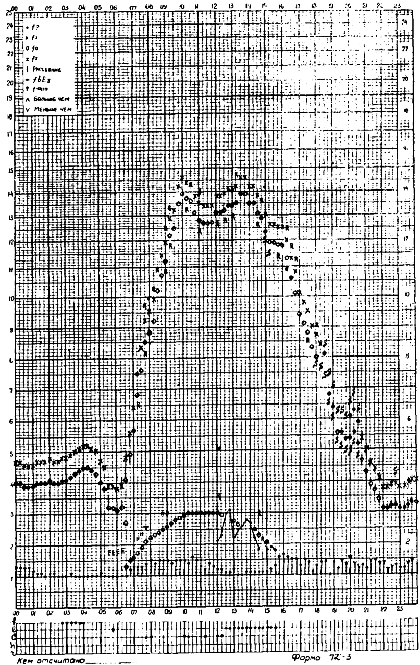
Москва станция НИЗМИР f-график ионосферных данных время 30°E дата 22 ноября 1958г
