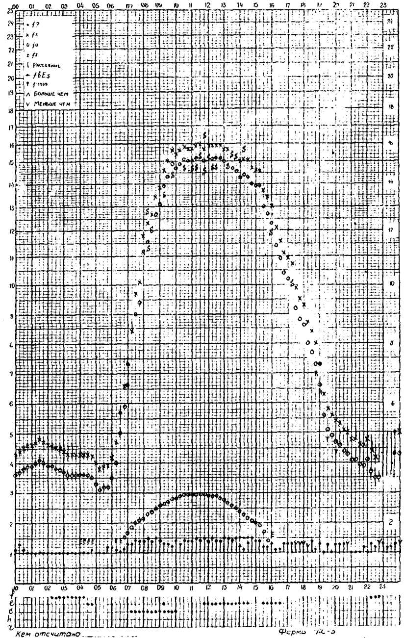
Модель 30° станция Низмид f- график ионосферных данных дата 17 ноября 1958г.
