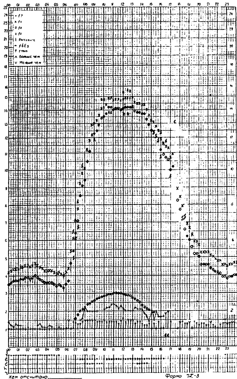
Москва станция НИЗМИР f-график ионосферных данных время 30°E дата 21 ноября 1958г
