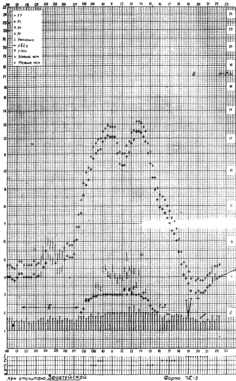
Время 75°E станция Дам-Виа f-график ионосферных данных дата 15 декабря 1959г.
