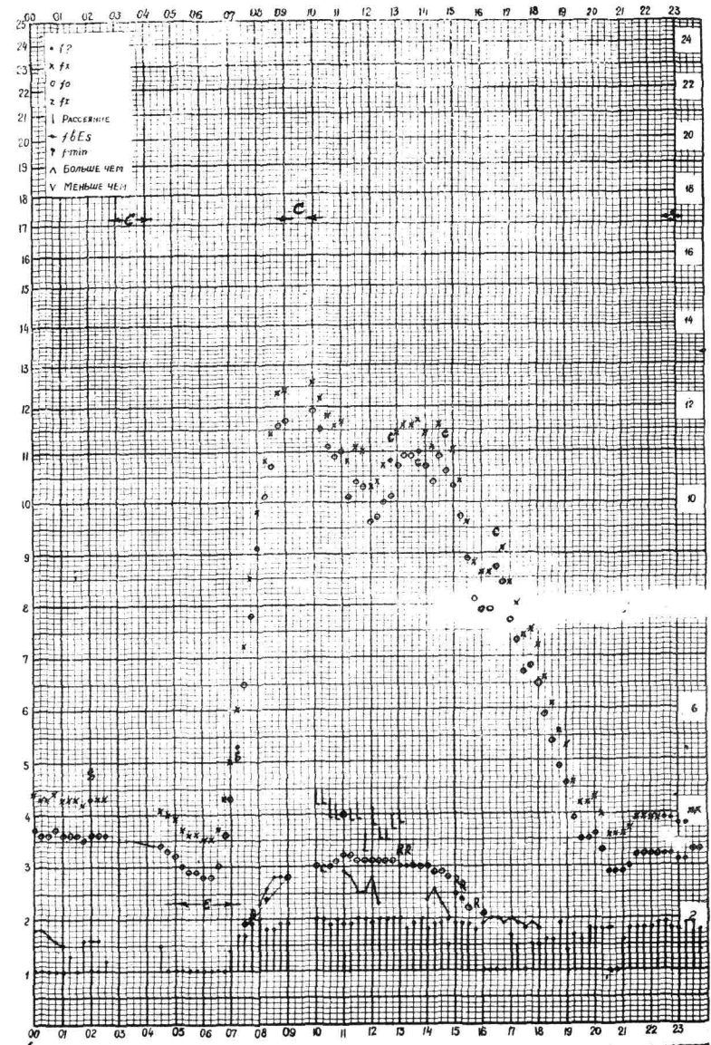
Время 75°E станция Алма-Ата f-график ионосферных данных дата 20 декабря 1959
