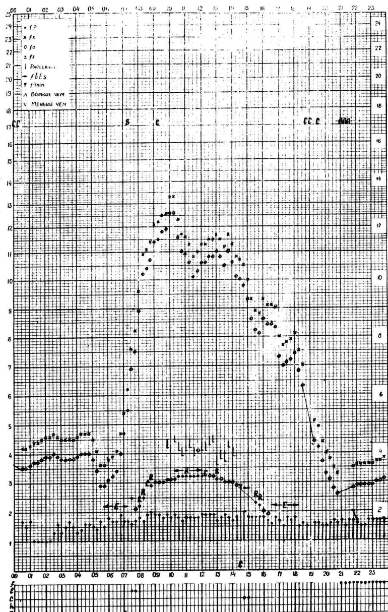
станция Алма-Ата - график ионосферных данных дата 21 декабря 1959. ВРЕМЯ 75°E
