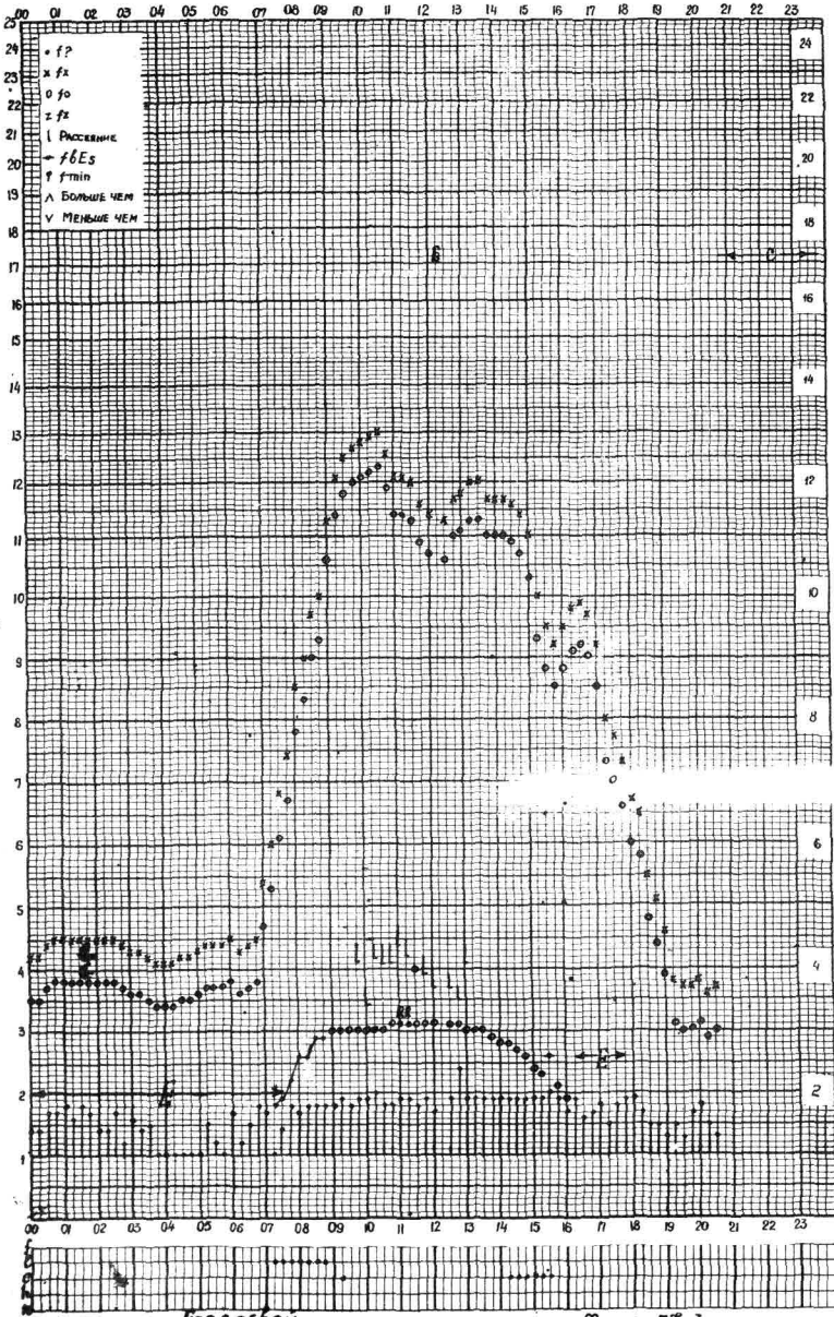
Время 75°E станция Алма-Ата f-график ионосферных данных дата 19 декабря 1959
