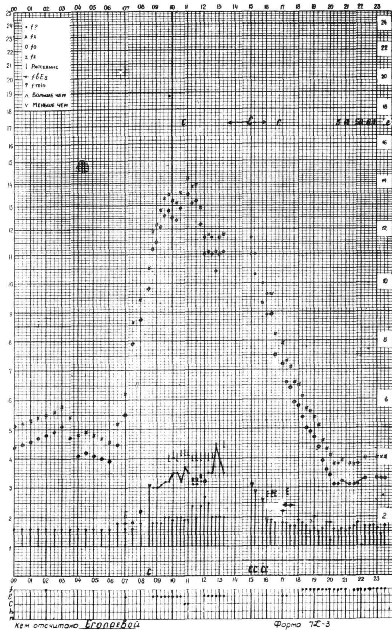
Время 75°E станция Дам-Виа f-график ионосферных данных дата 16 декабря 1959г.
