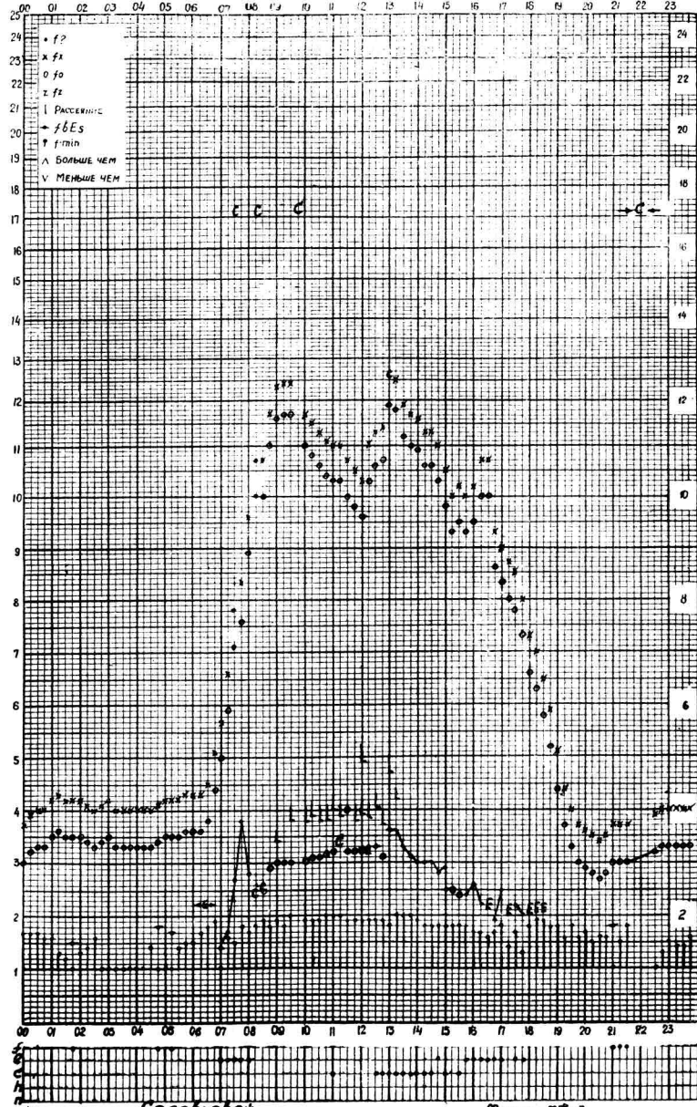
станция Алма-Ата - график ионосферных данных дата 22 декабря 1959.
