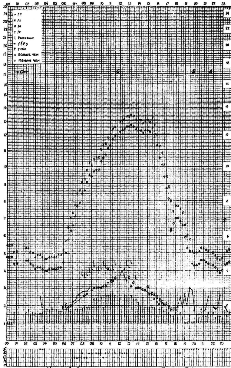
станция Алма-Ата - график ионосферных данных дата 4 ноября 1959 Время 75°E
