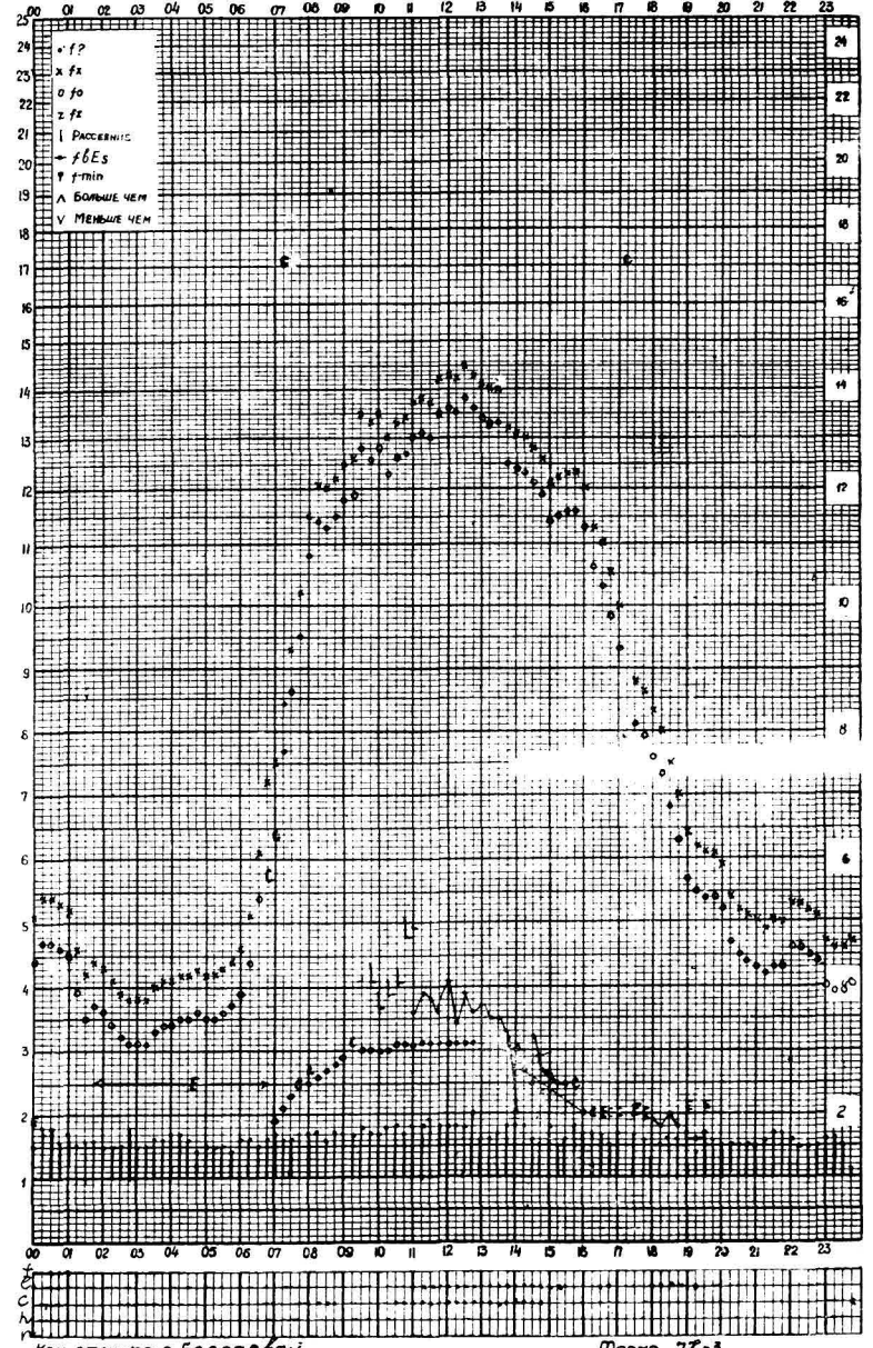
станция Алма-Ата f-график Время 75°E ионосферных данных дата 22 ноября 1959г
