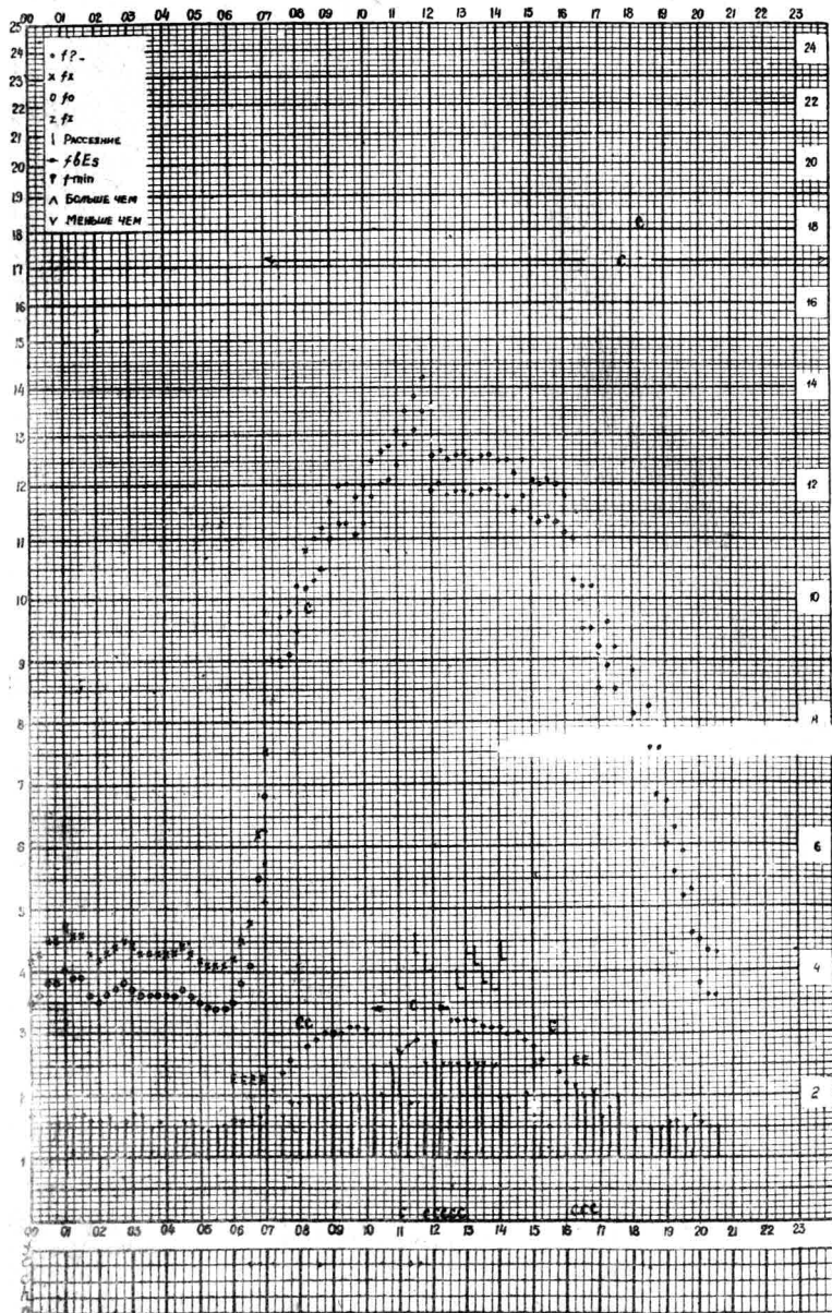
Время 75°E станция Алма-Ата f-график ионосферных данных дата 25 ноября 1959г.
