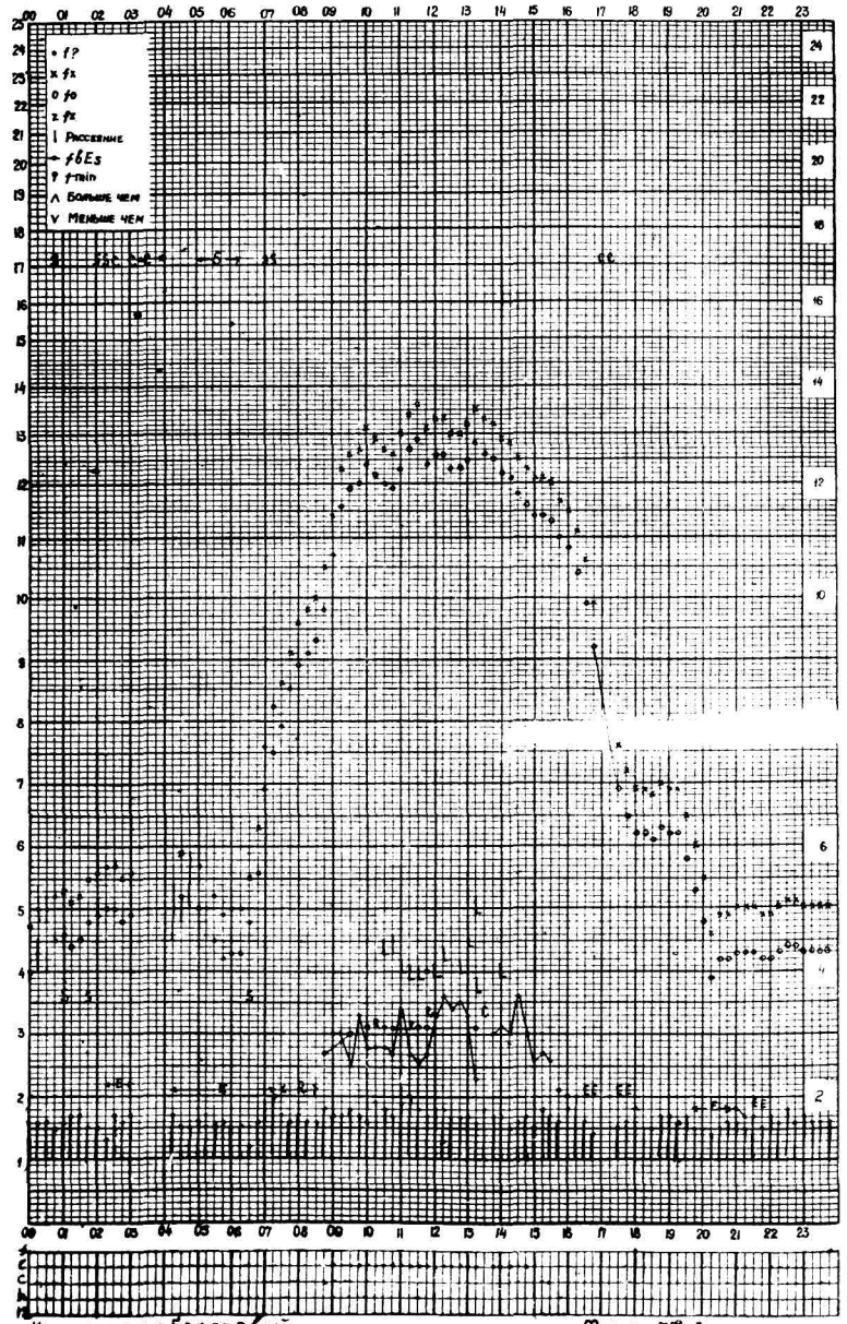
станция Алма-Ата f-график Время 75°E ионосферных данных дата 21 ноября 1959г
