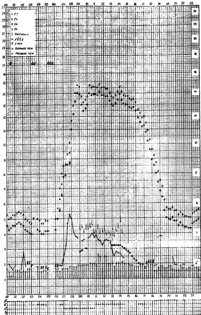
станция Алма-Ата - график ионосферных данных дата 3 ноября 1959 Время 75°E
