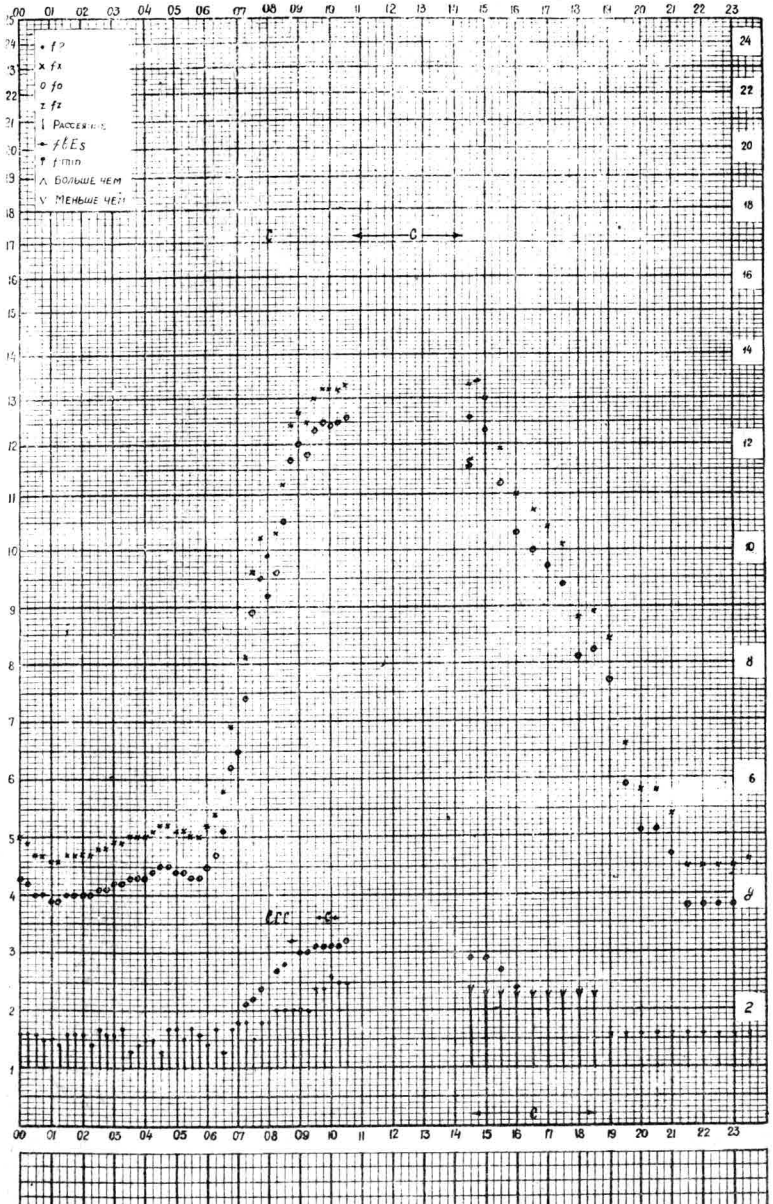
Время 75°E станция Алма-Ата f-график ионосферных данных дата 26 ноября 1959г.
