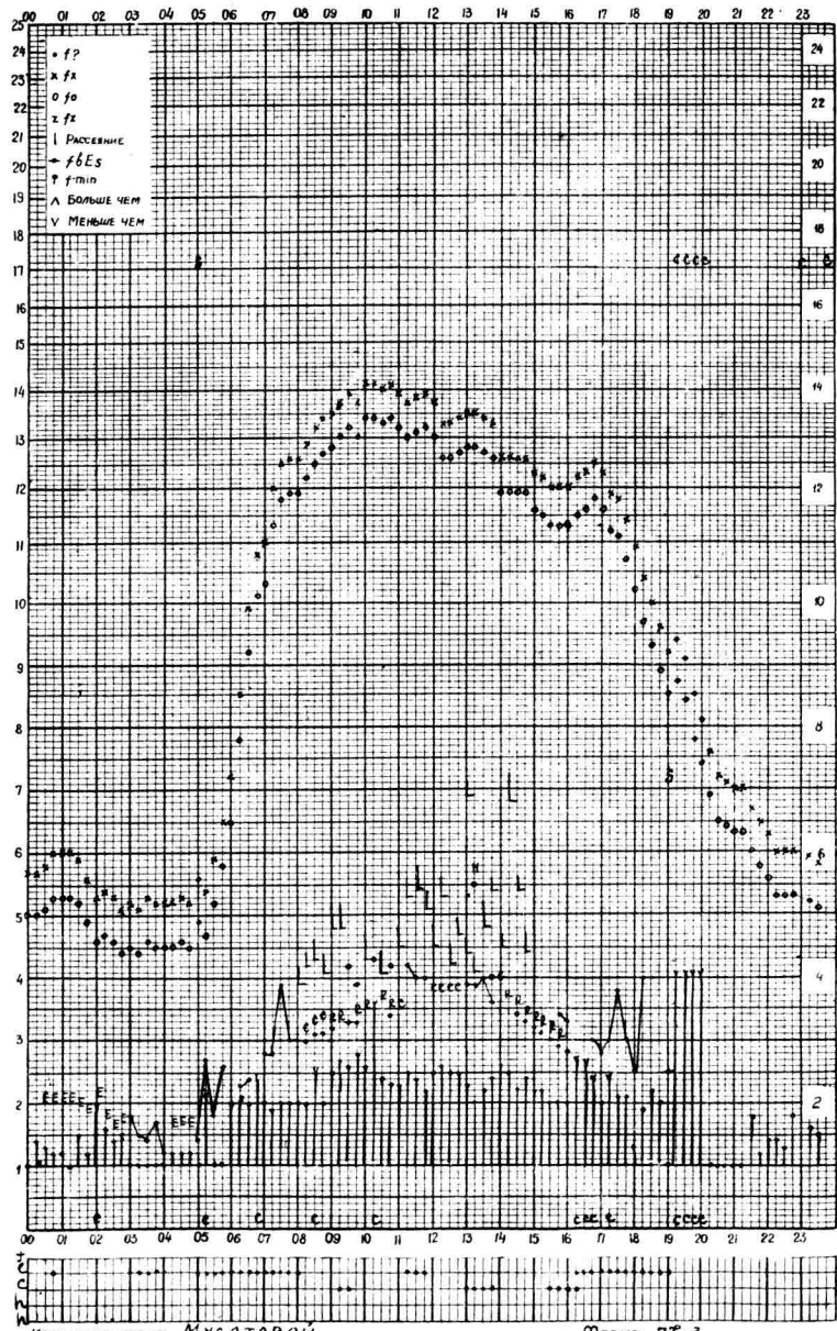
Время 75°E станция Алма-Ата - график ионосферных данных дата 7 ОКТЯБРЯ 1959г.
