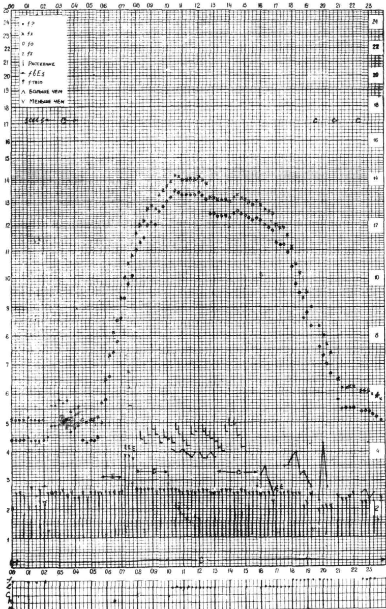
Время 75°E станция Алма-Ата - график ионосферных данных дата 17 октября 1959
