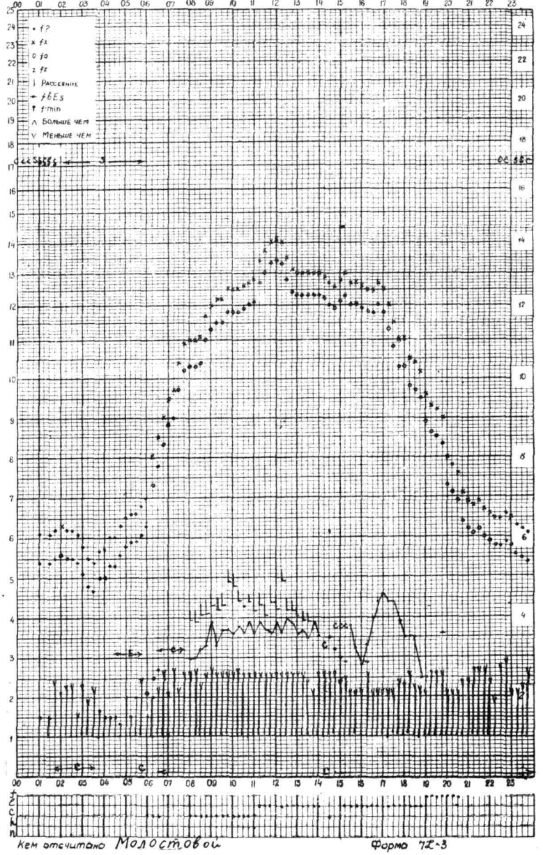
Время 75°E станция Алма-Ата - график ионосферных данных дата 18 октября 1959
