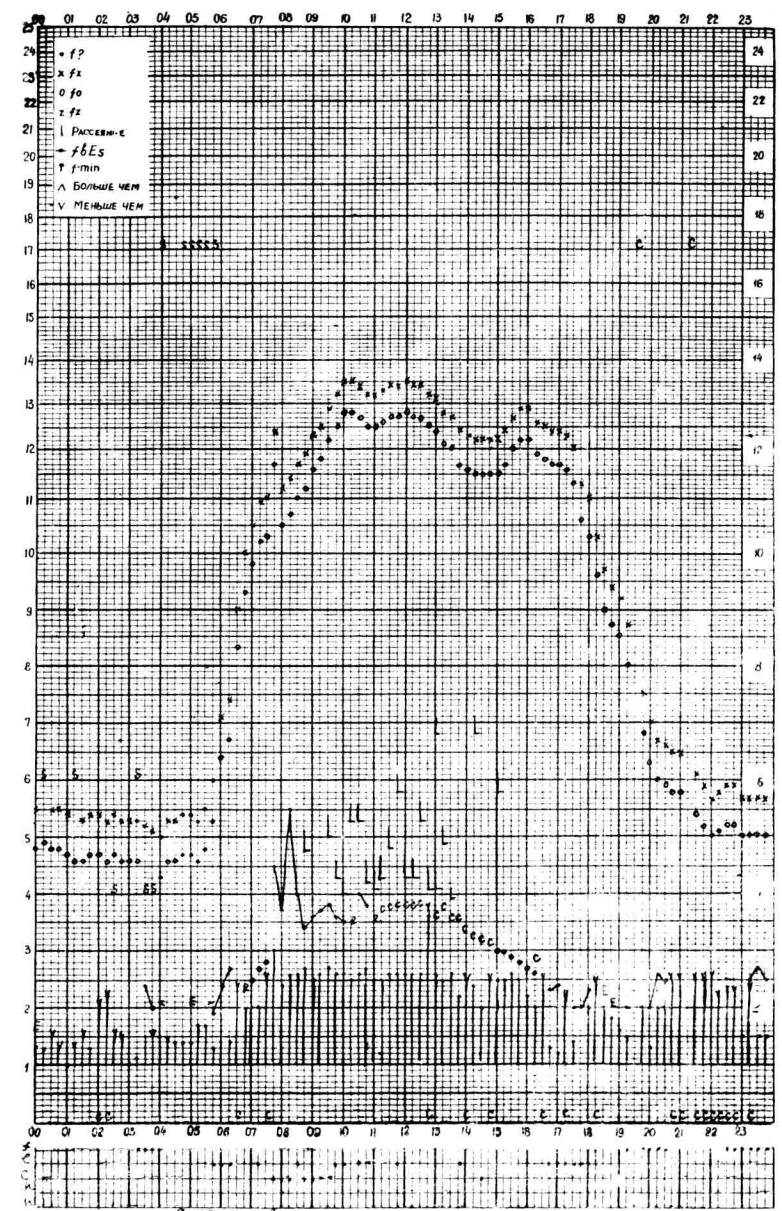
Время 75°E станция Алма-Ата - график ионосферных данных дата 8 ОКТЯБРЯ 1959г.
