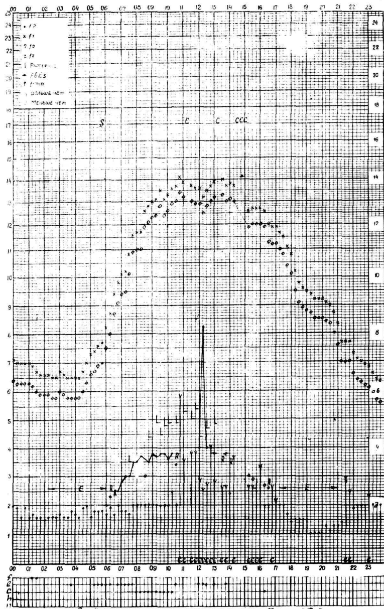
станция Дана-Ата f-график Время 75°E ионосферных данных дата 2 октября 1959
