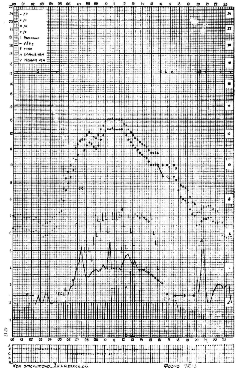
Время 75°E станция Алма-Ата f-график ионосферных данных дата 2 СЕНТЯБРЯ 1959г.
