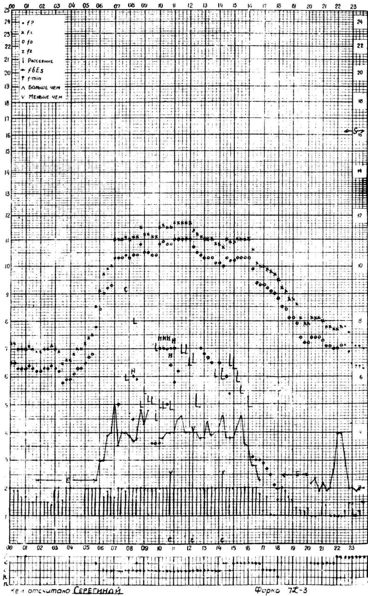
Время 75°E станция Алма-Ата f-график ионосферных данных дата 1 СЕНТЯБРЯ 1957г.
