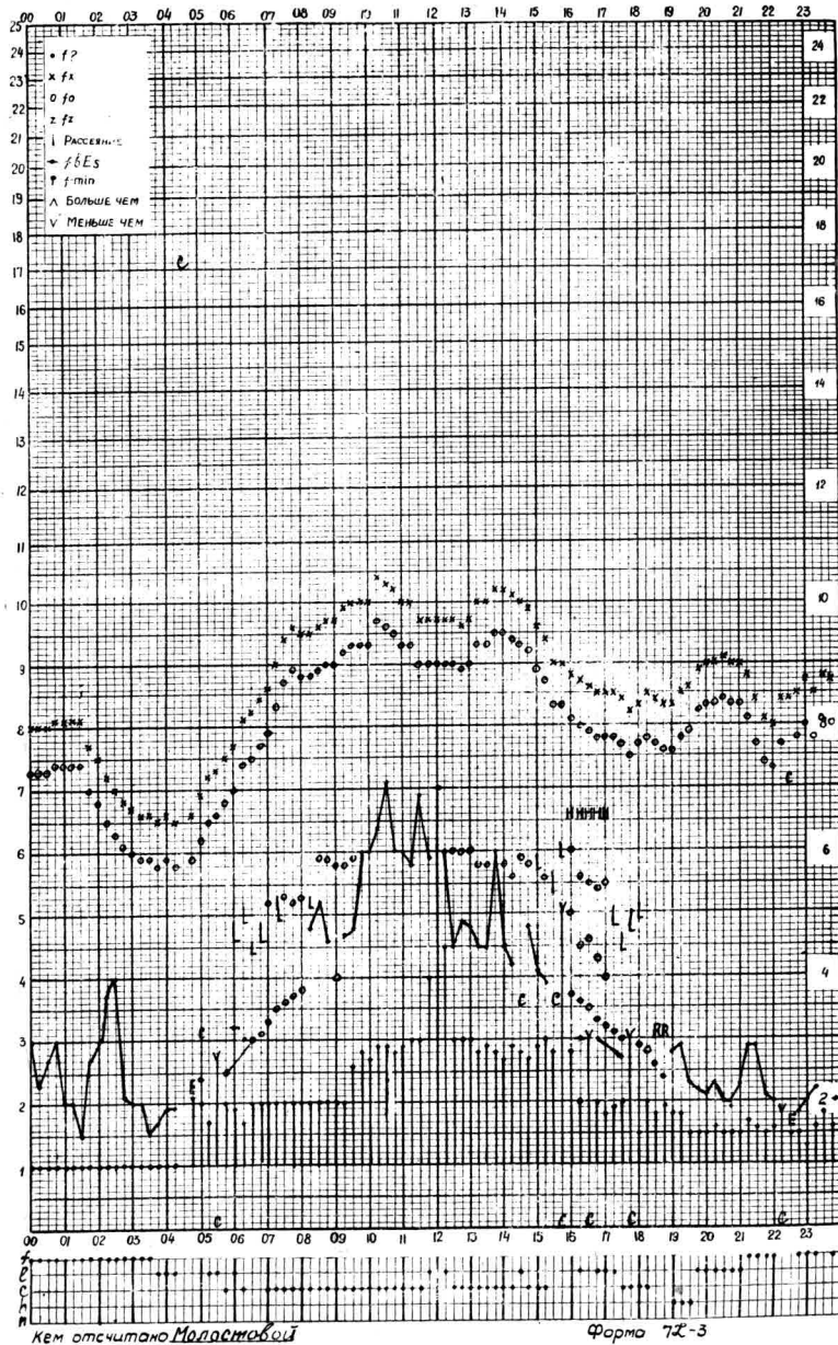
Время 75°E станция Алма-Ата f-график ионосферных данных дата 13 июля 1959г.
