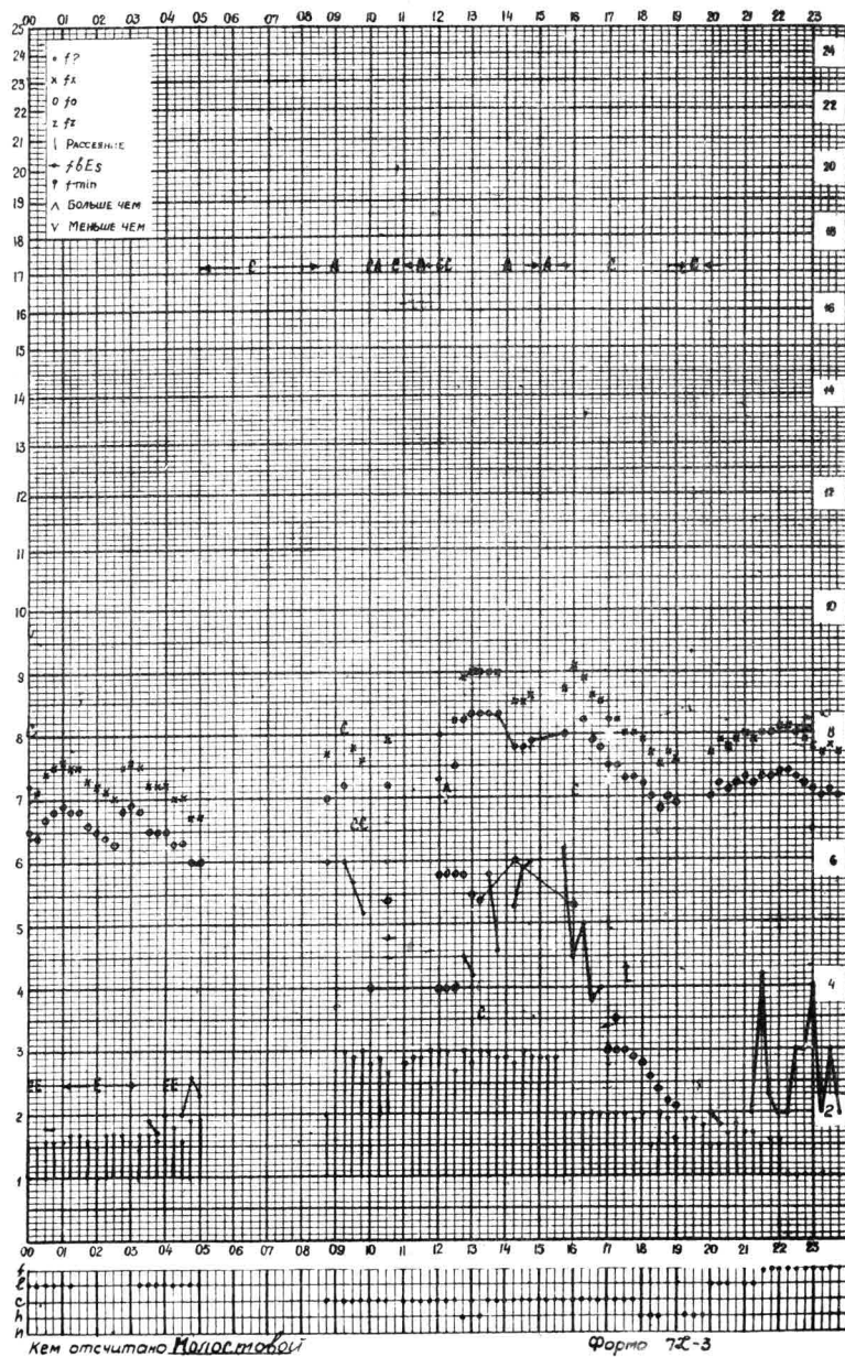
Время 75°E станций Алма-Ата f-график ионосферных данных дата 12 июля 1959г.
