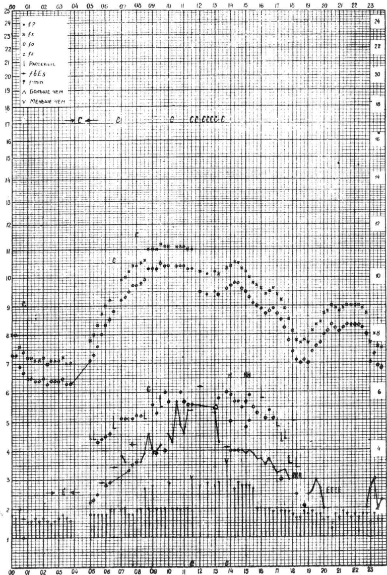
Время 75°E станция Влма-Ата f- график ионосферных данных дата 9 июля 1959г.
