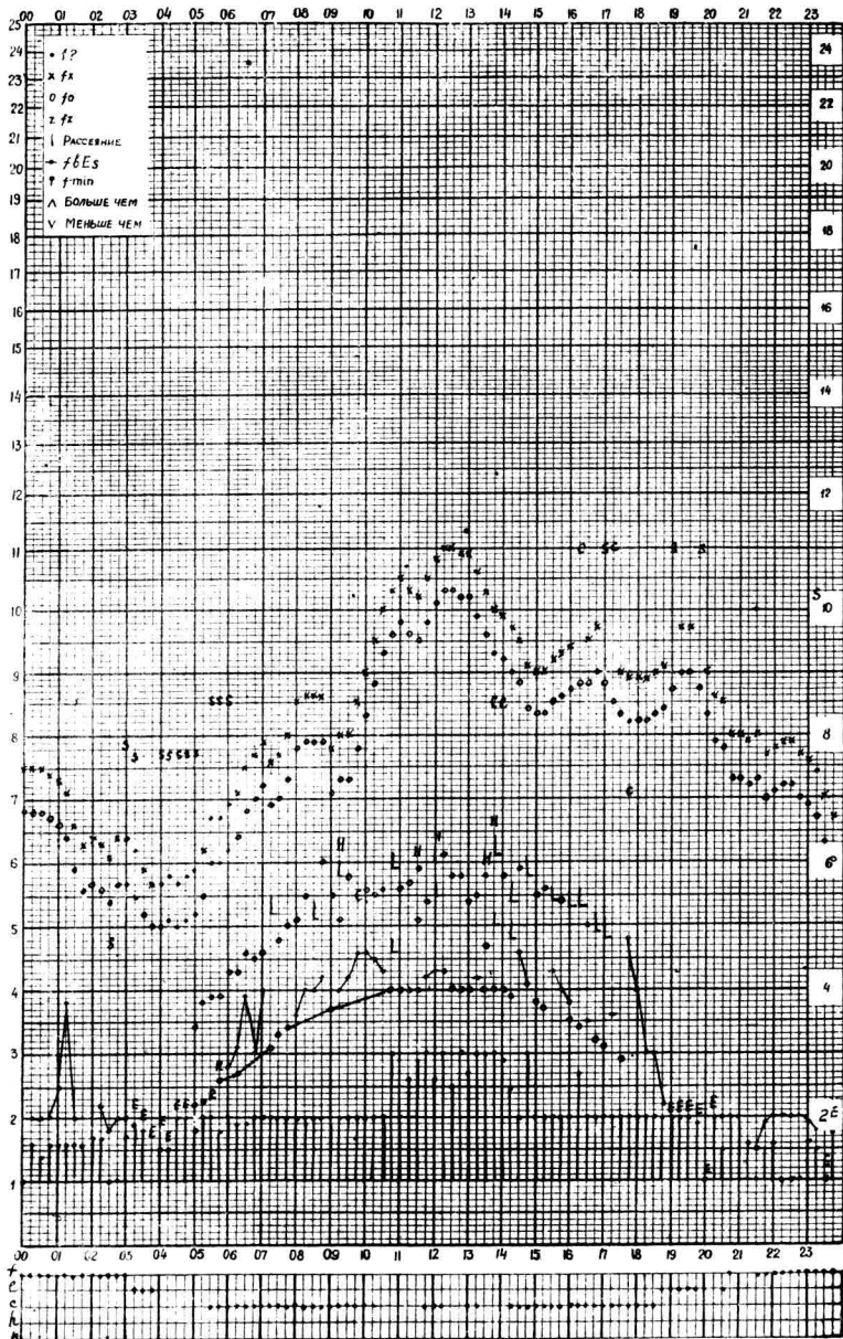
Время 75°E станция Алма-Ата - график ионосферных данных дата 25 июля 1959г.
