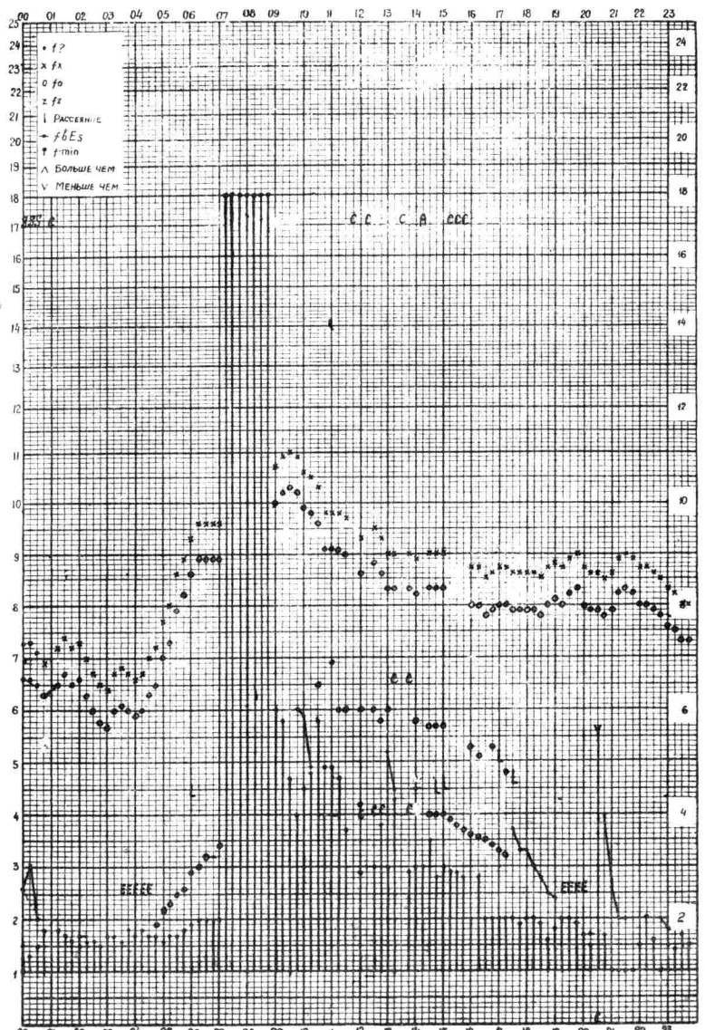
Время 75°E станция Влма-Ата f- график ионосферных данных дата 10 июля 1959г.
