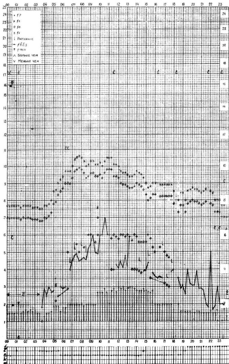
Время 75°E станций Алма-Ата f-график ионосферных данных дата 11 июля 1959г.
