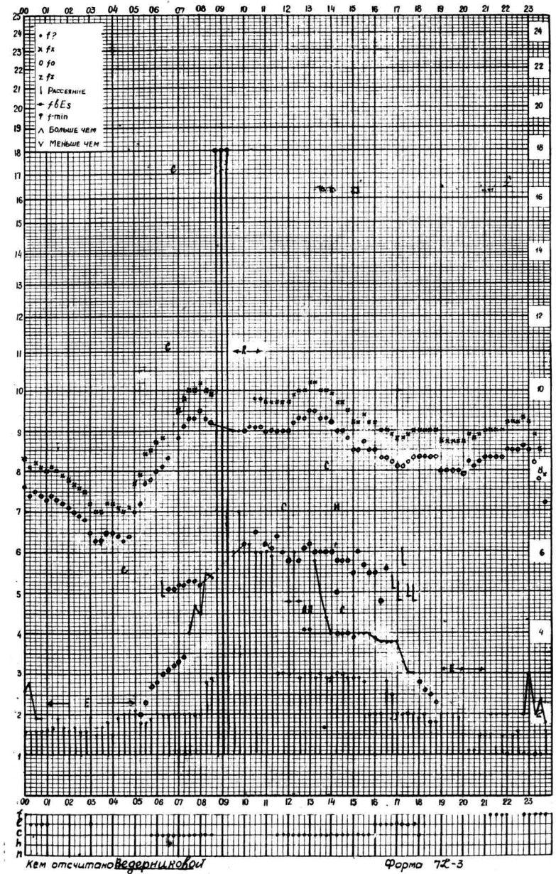
Время 75°E станция Алма-Ата f-график ионосферных данных дата 14 июля 1959г.
