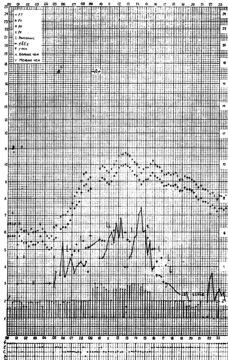
Время 75°E станция Алма-Ата - график ионосферных данных дата 26 июля 1959г.
