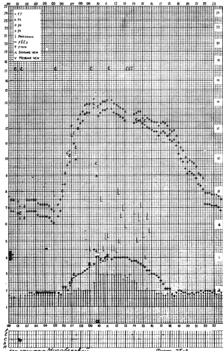
Время 75°E станция вама-аиаф- график ионосферных данных дата 20 Марта 1959г.
