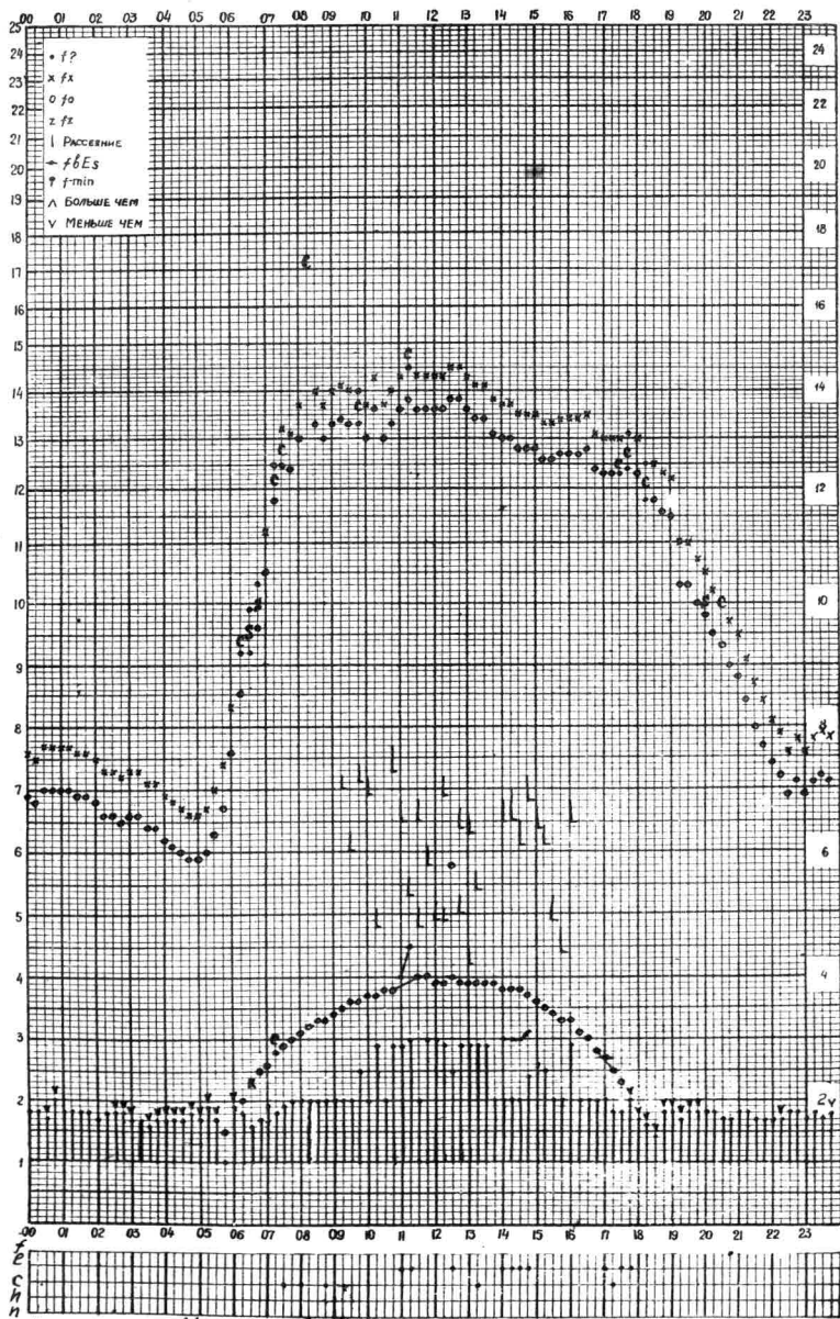
Время 75°E станция вама-аиаф- график ионосферных данных дата 19 Марта 1959г.
