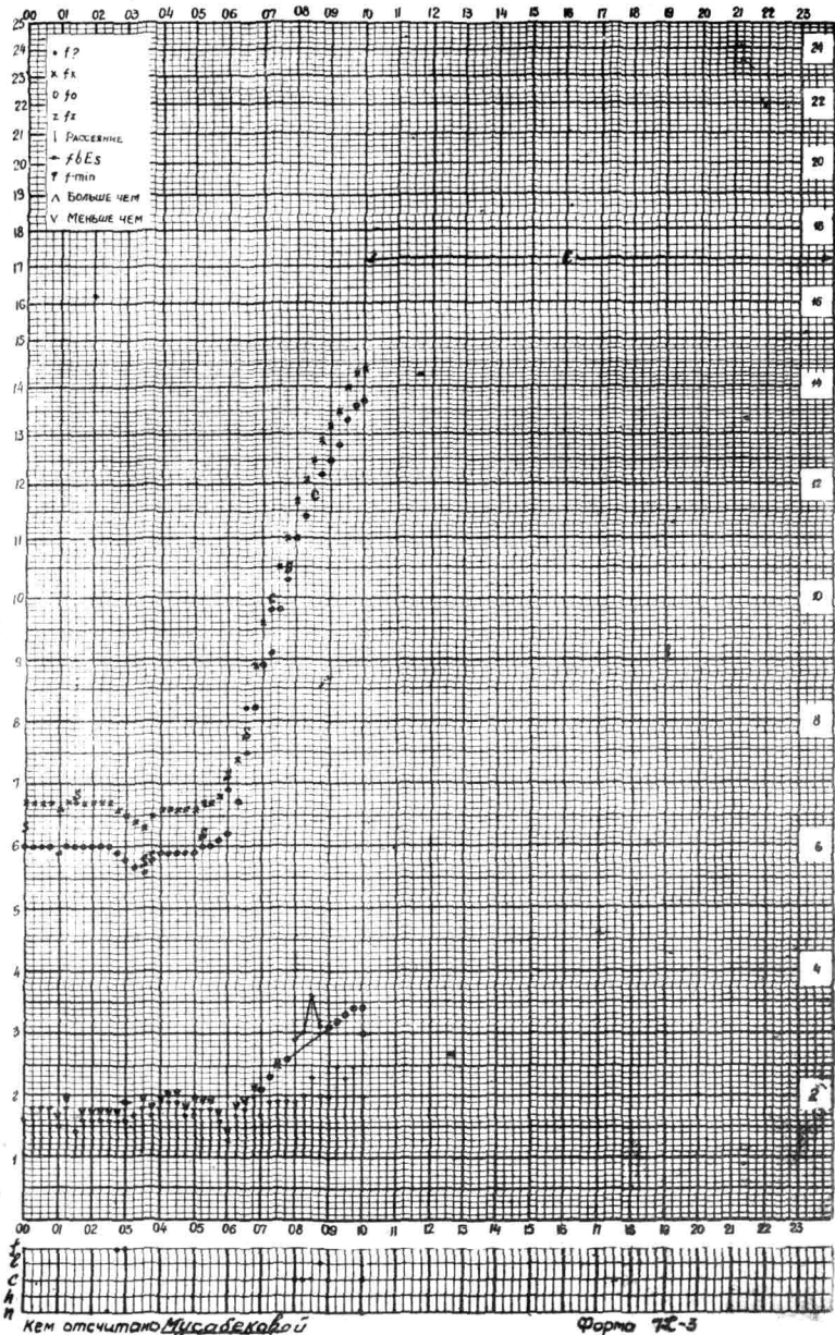
Время 75°E станция Алма-Ата f-график ионосферных данных дата 3 Марта 1959г.
