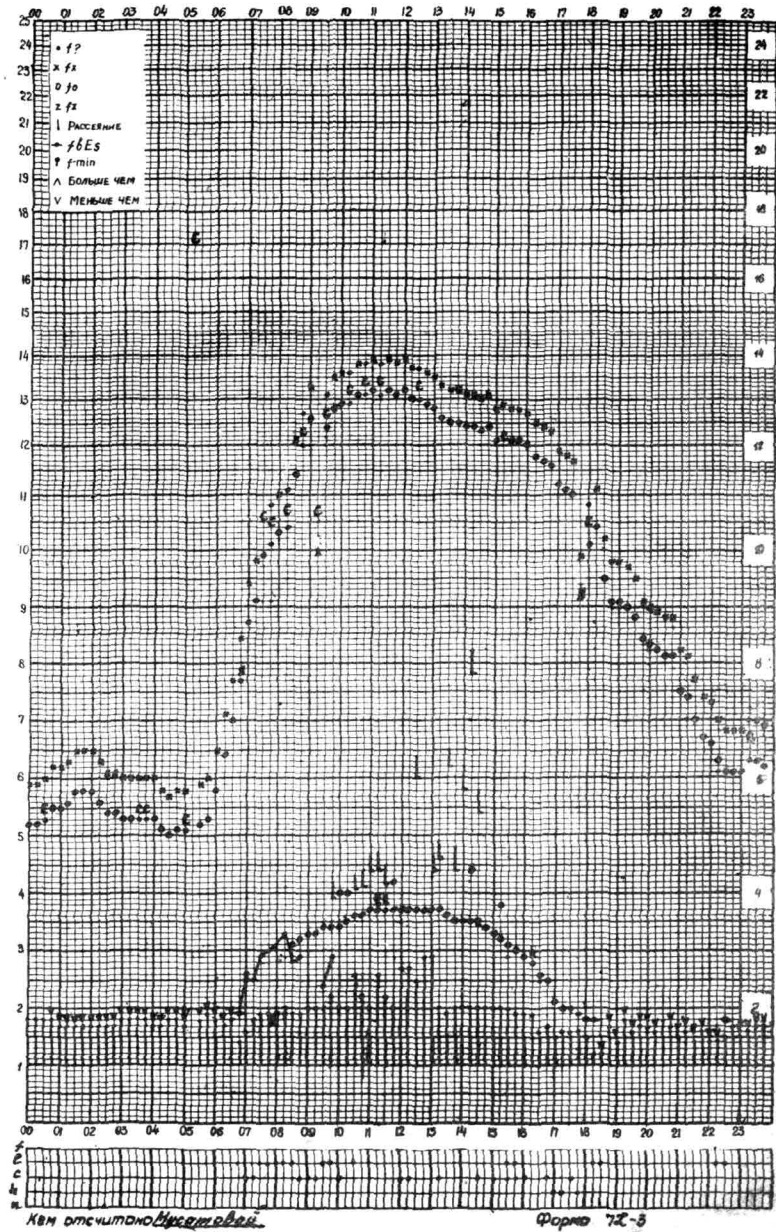
Время 75°E станция Алма-Ата f-график ионосферных данных дата 4 Марта 1959г.
