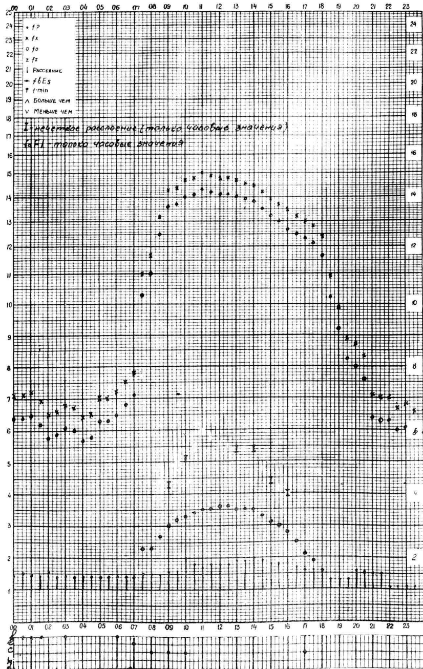
Время 75°E станция Анна-Аста f-график ионосферных данных дата 9 февраля 1958
