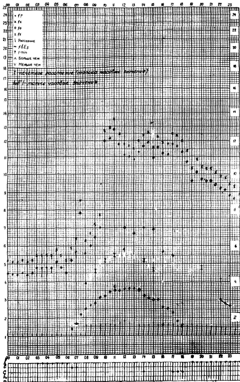
станция Алма-Ата - график ионосферных данных дата 11 февраля 1968
