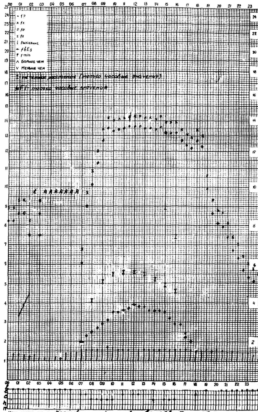
Время 75°E станция Алма-Ата - график ионосферных данных дата 12 февраля 1968
