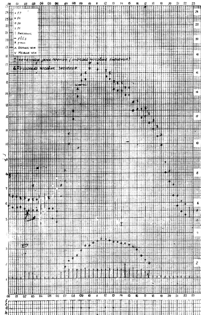
Время 75°E станция Анна-Аста f-график ионосферных данных дата 10 февраля 1958
