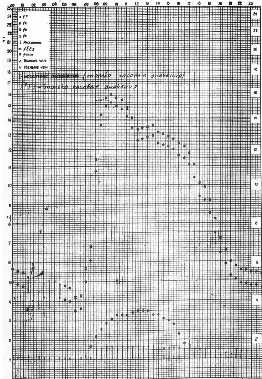
Время t \pm \epsilon станция Алма-Ата - график ионосферных данных дата 7 января 1958
