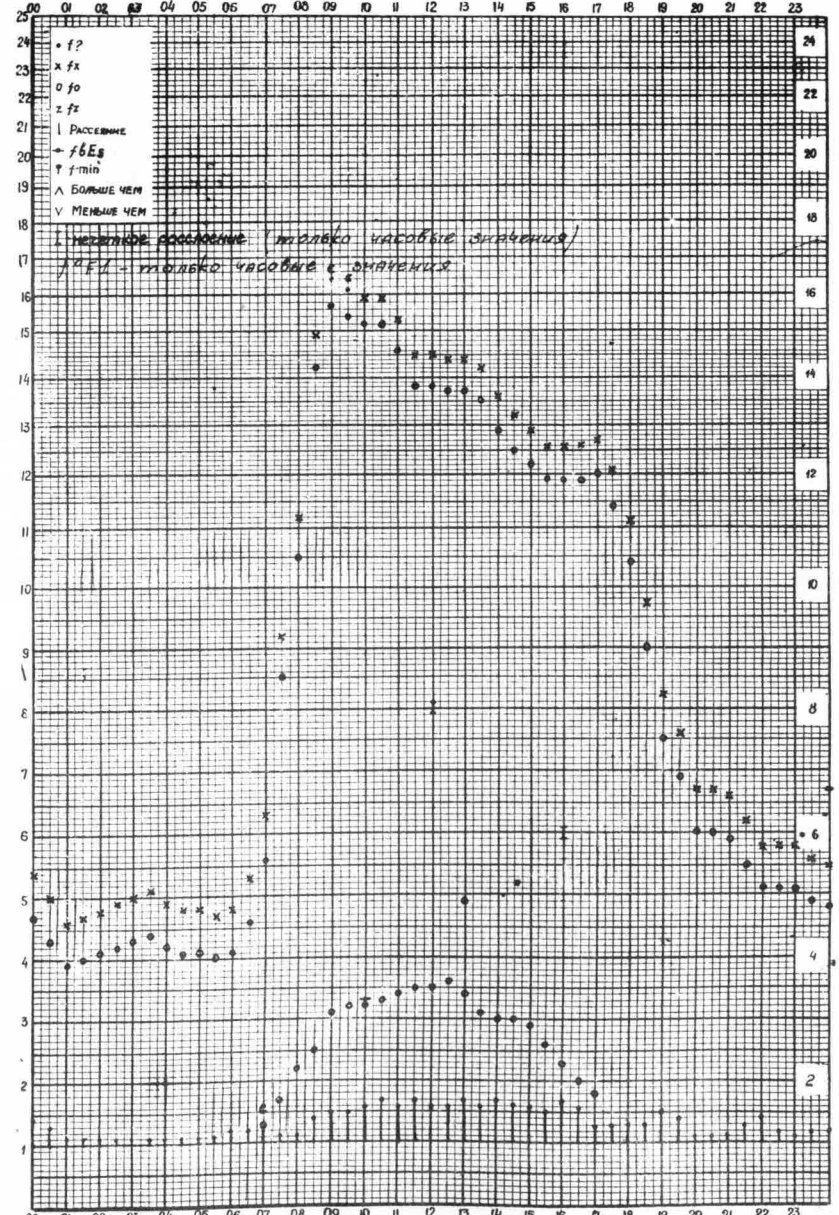
Время t \pm \epsilon станция Алма-Ата - график ионосферных данных дата 8 января 1958
