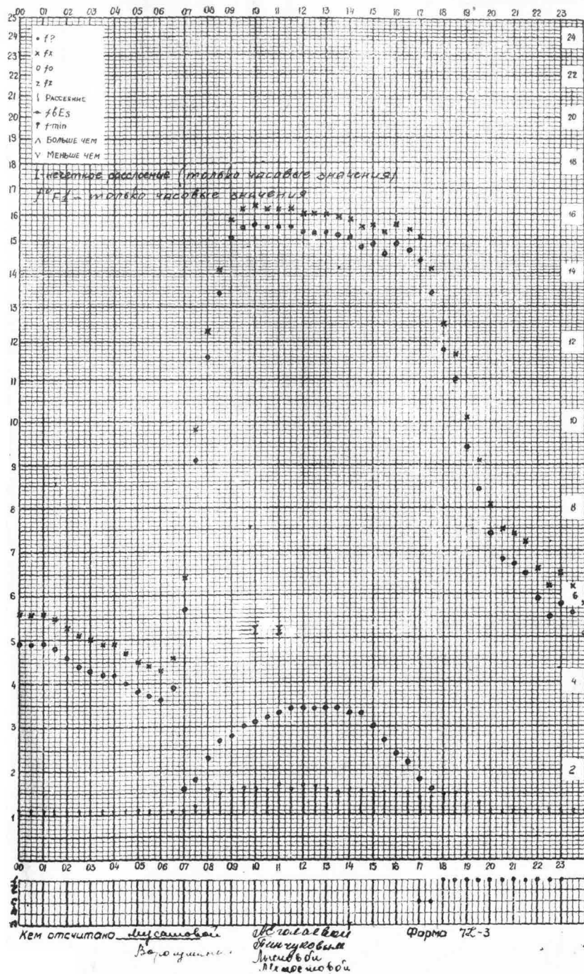
Время \lambda 5^{\circ} E станция Алма-Ата - график ионосферных данных дата 10 января 1958
