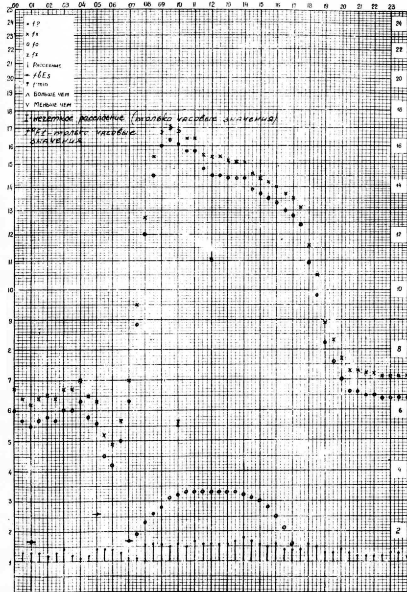
станция Амь-Ата - график ионосферных данных дата 22 января 1958
