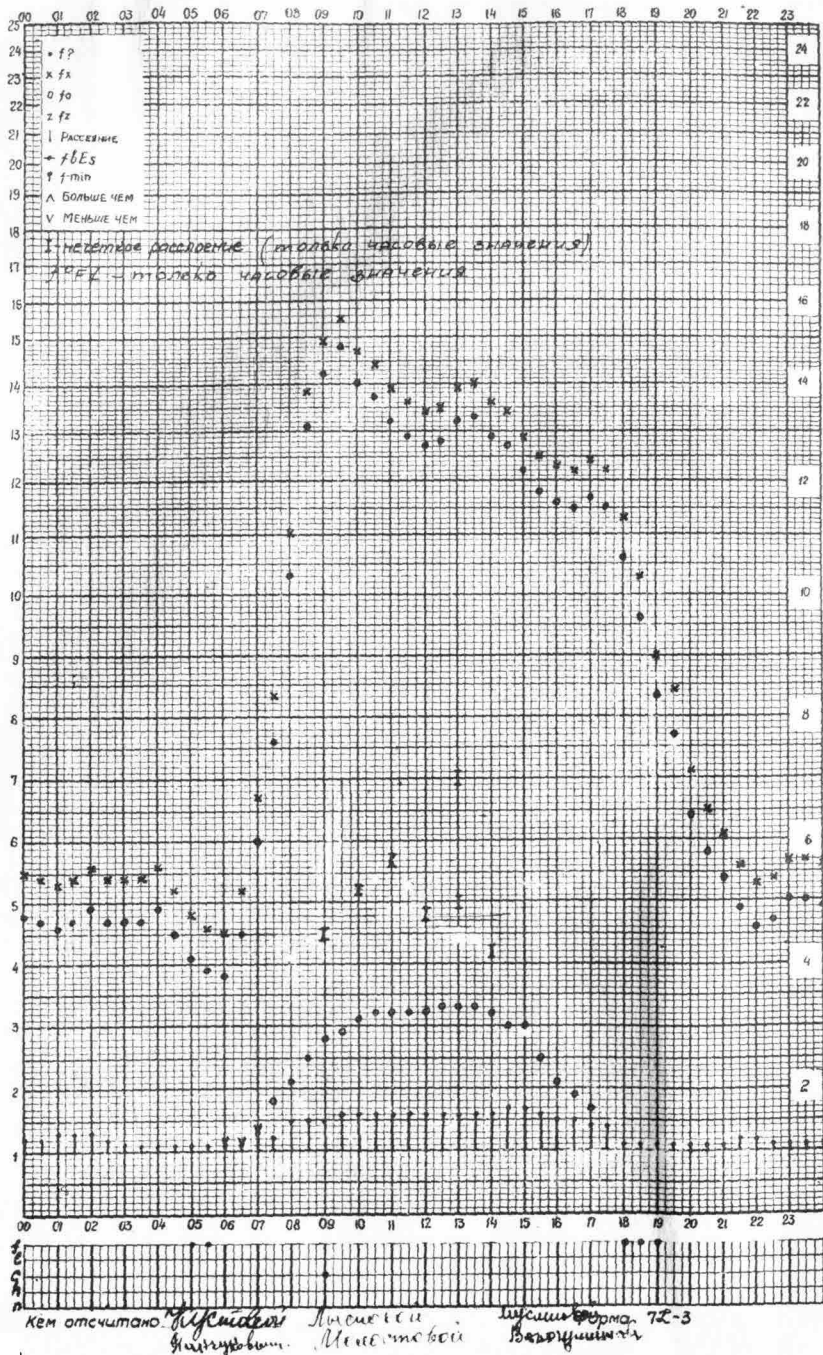
станция Алма-Ата - график ионосферных данных дата 9 января 1958 Время \lambda 5^{\circ} E
